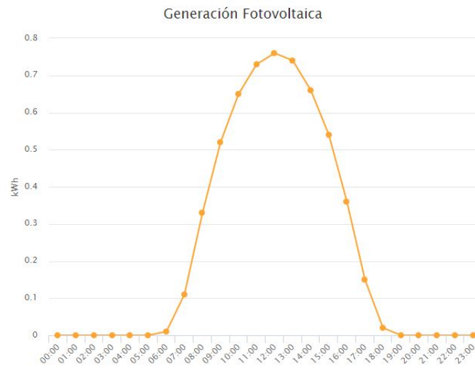
Figura 4.17: Ciclos medios de potencia de un sistema fotovoltaico durante un día
