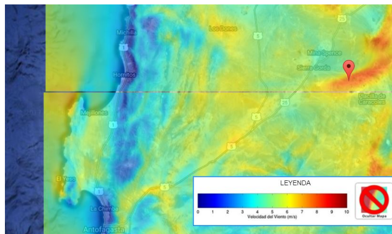
Figura 4.13: Disponibilidad de Recurso Eólico.
