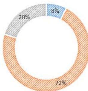
Figura 4.1: Participación por tipo de combustible en la capacidad de generación de la zona.
