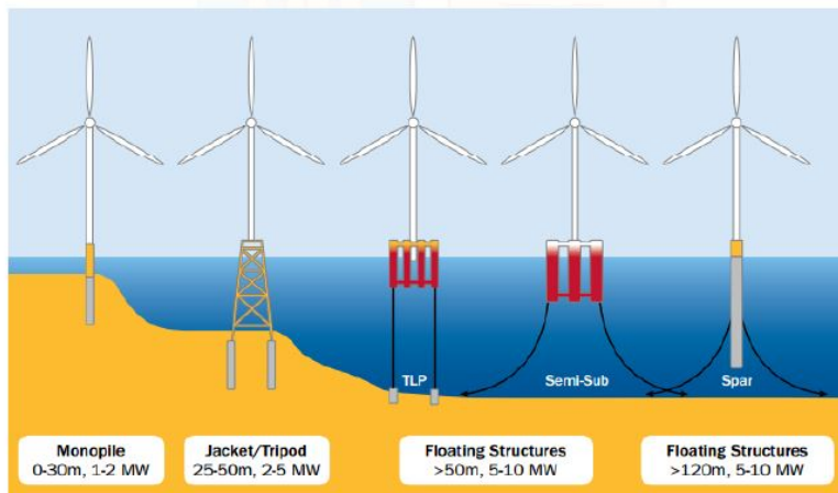
Figura 2.28: Potencia y profundidad recomendada para cada cimentación
