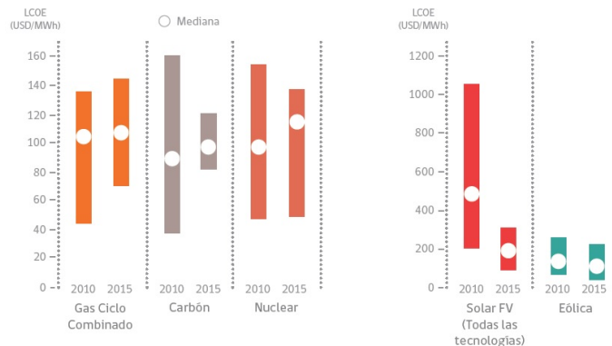
Figura 2.5: Costos Proyectados Distintos Tipos de Energía
