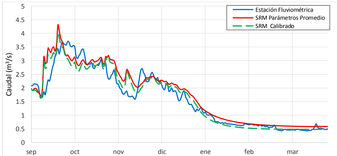
Gráfico 6.37: Caudales diarios medidos y simulados ( \text{m}^3/\text{s} ) –2000 -2001
