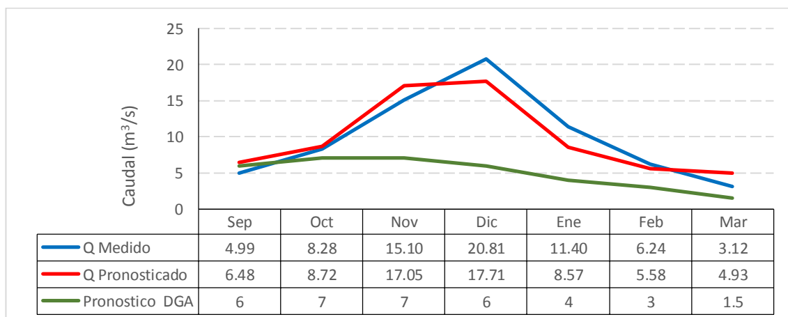
Gráfico 7.56: Caudal medido, pronosticado SRM y DGA Año 2015 con Actualización en Octubre – Río Putaendo en Resguardo los Patos
