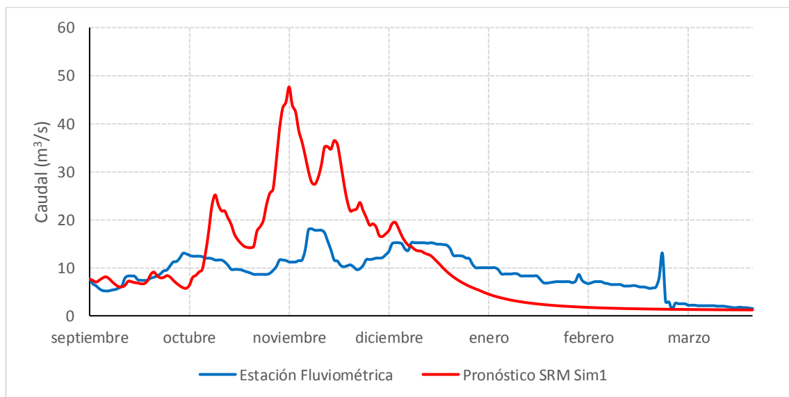
Gráfico 7.39: Pronostico de Caudales Año 2016 – Río Putaendo en Resguardo los Patos
