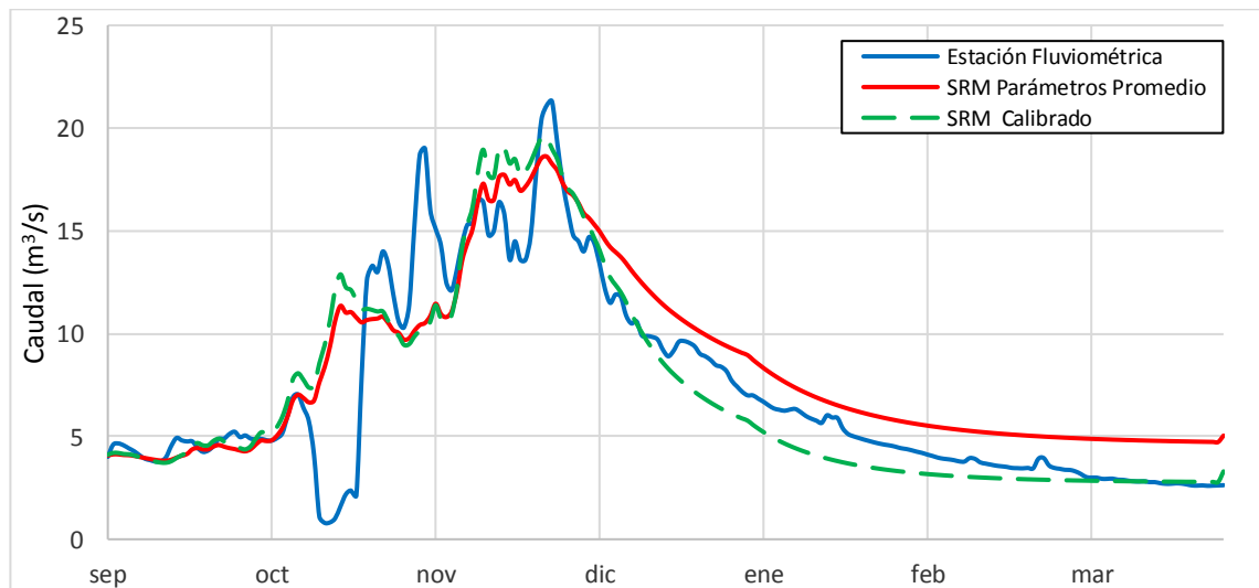
Gráfico 6.29: Caudales diarios medidos y simulados ( \text{m}^3/\text{s} ) –2003 -2004
