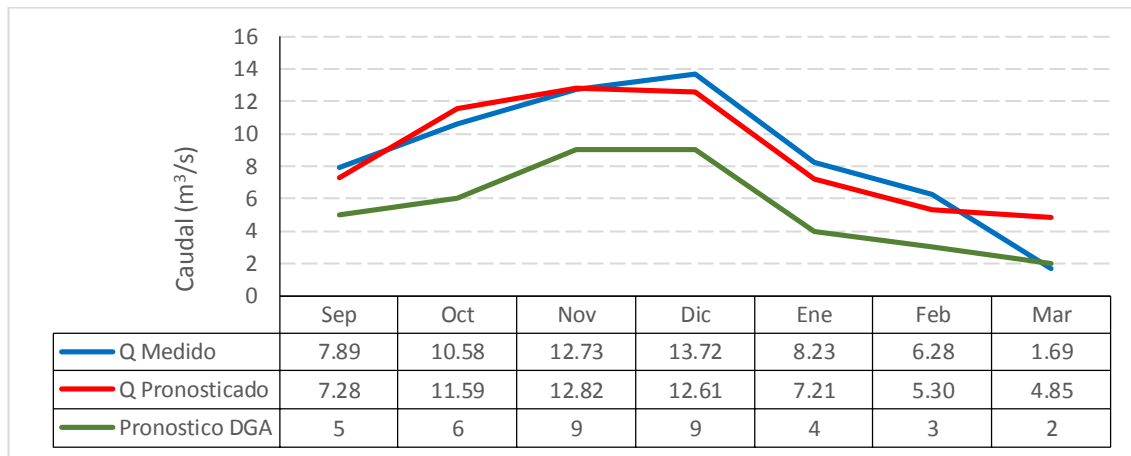
Gráfico 7.72: Caudal medido, pronosticado SRM y DGA Año 2016 con Actualización en Noviembre – Río Putaendo en Resguardo los Patos
