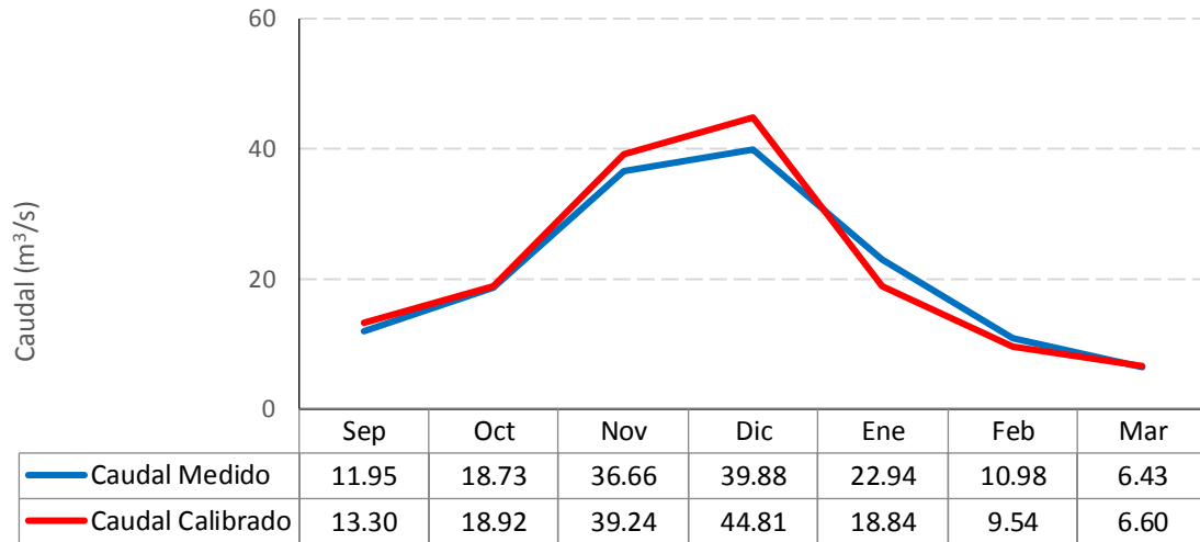
Gráfico 6.2: Caudales mensuales medidos y simulados (m 3 /s) - Cuenca Putaendo en Resguardo Los Patos (2002-2003)
