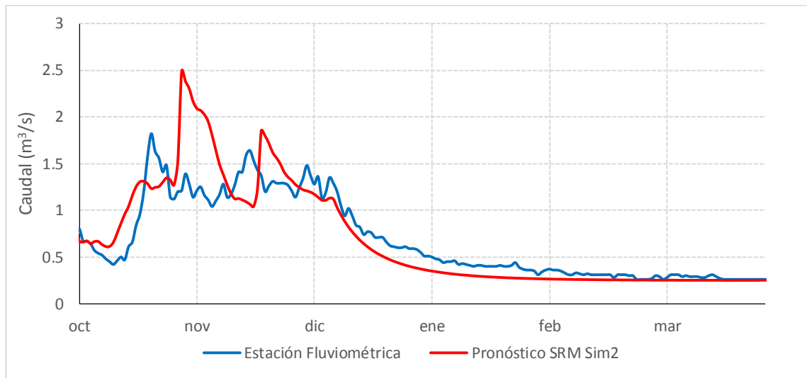
Gráfico 7.62: Pronóstico de Caudales con actualización en Octubre Año 2015 – Estero Pocuro en el Sifón
