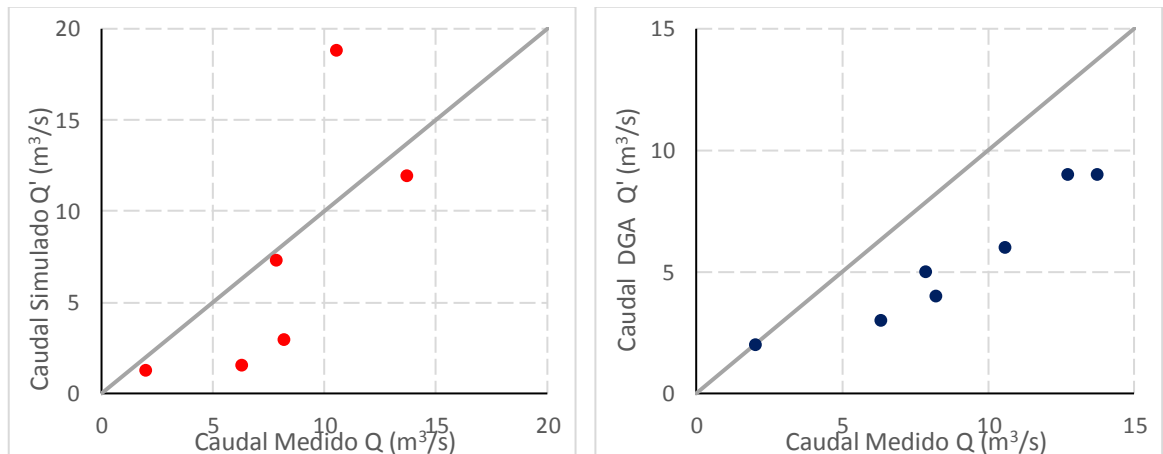
Gráfico 7.45: Comparativa entre Valores medidos en estación Fluviométrica, pronóstico SRM y pronóstico de la DGA – Primera Simulación Año 2016
