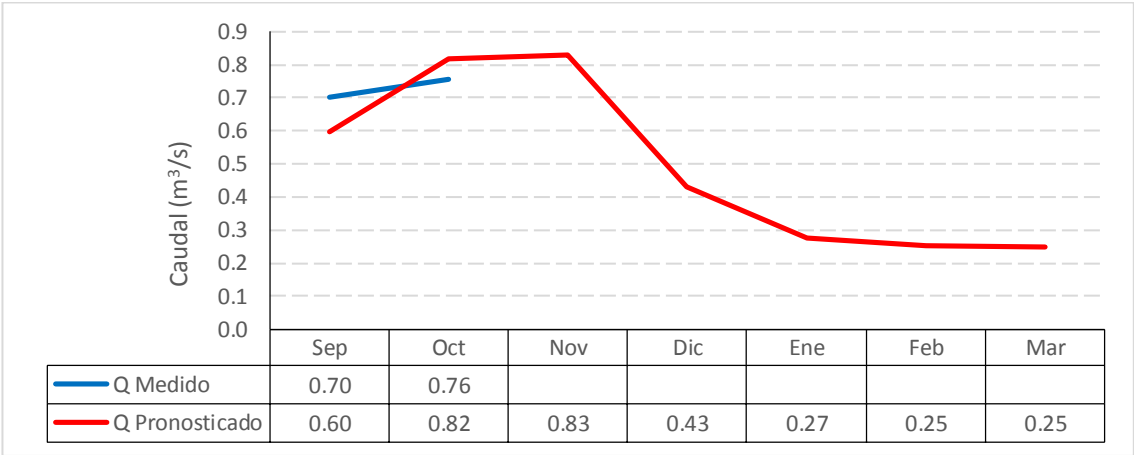
Gráfico 7.66: Caudal medido y pronosticado SRM Año 2016 con Actualización en Octubre – Estero Pocuro en el Sifón
