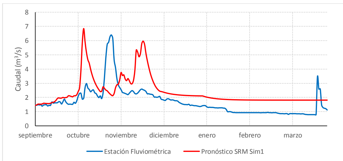
Gráfico 7.37: Pronostico de Caudales Año 2014 – Río Putaendo en Resguardo los Patos
