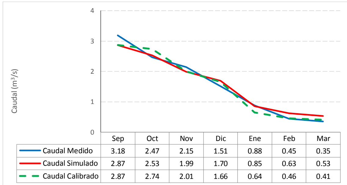
Gráfico 6.40: Caudales mensuales ( m^3/s ) – 2002 -2003
