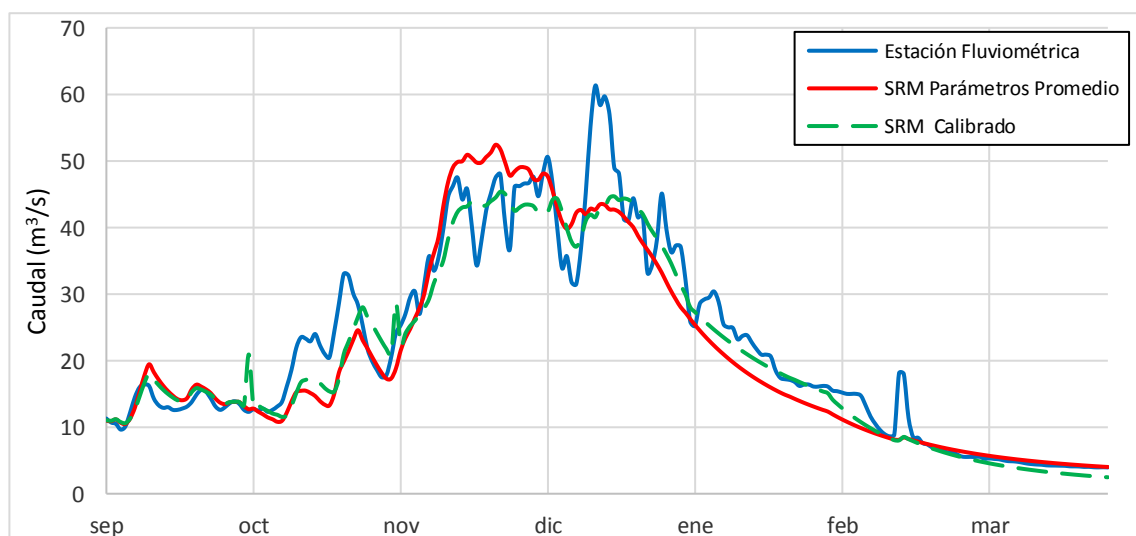
Gráfico 6.27: Caudales diarios medidos y simulados ( m^3/s ) –2005 -2006
