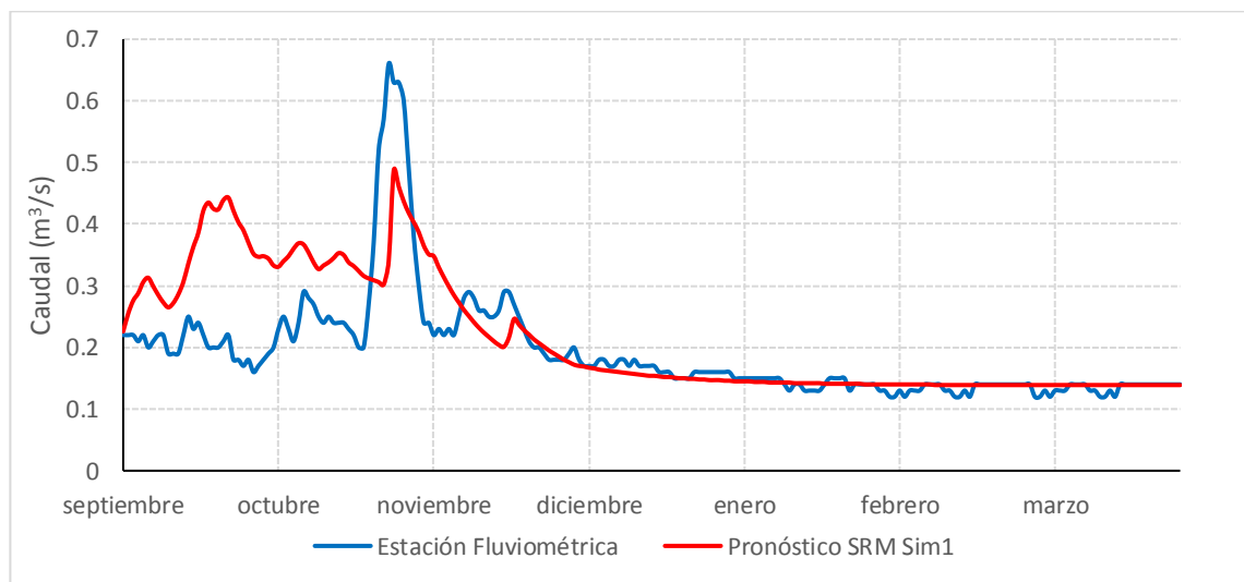
Gráfico 7.46: Pronostico de Caudales Año 2014 – Estero Pocuro en el Sifón
