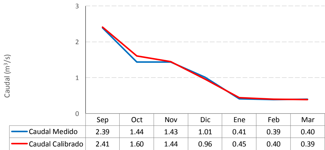
Gráfico 6.20: Caudales mensuales medidos y simulados (m3/s) - Cuenca Pocuro en el Sifón (2009-2010)
