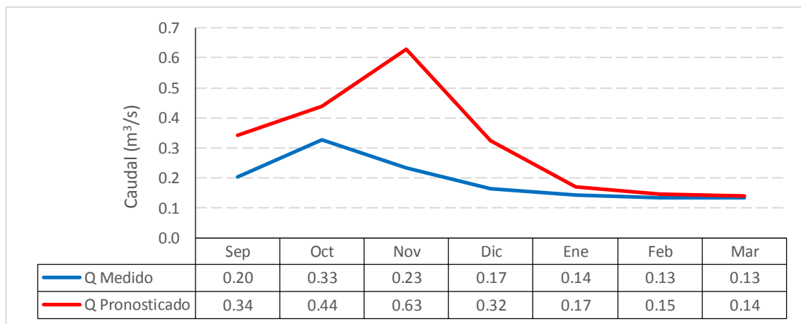
Gráfico 7.64: Caudal medido y pronosticado SRM Año 2014 con Actualización en Octubre – Estero Pocuro en el Sifón
