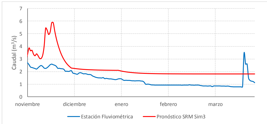
Gráfico 7.67: Pronóstico de Caudales con actualización en Noviembre Año 2014 – Río Putaendo en Resguardo los Patos
