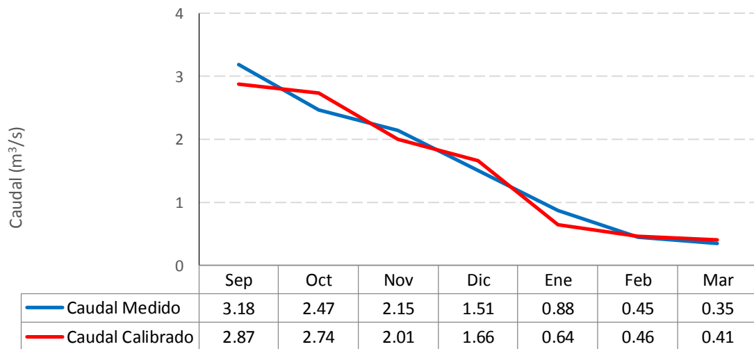
Gráfico 6.16: Caudales mensuales medidos y simulados (m 3 /s) - Cuenca Pocuro en el Sifón (2002-2003)
