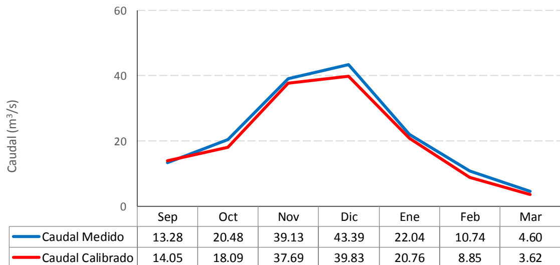
Gráfico 6.4: Caudales mensuales medidos y simulados (m 3 /s) - Cuenca Putaendo en Resguardo Los Patos (2005-2006)
