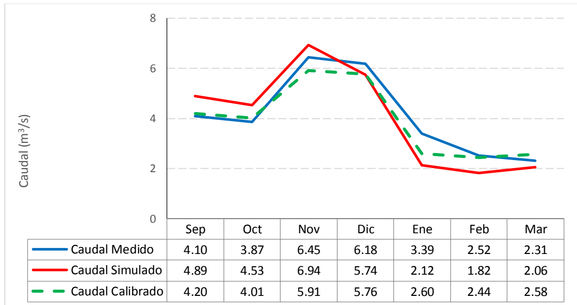
Gráfico 6.34: Caudales mensuales ( m^3/s ) –2004 -2011
