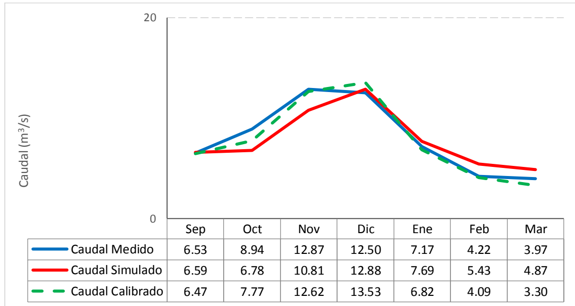
Gráfico 6.32: Caudales mensuales ( \text{m}^3/\text{s} ) –2009 -2010
