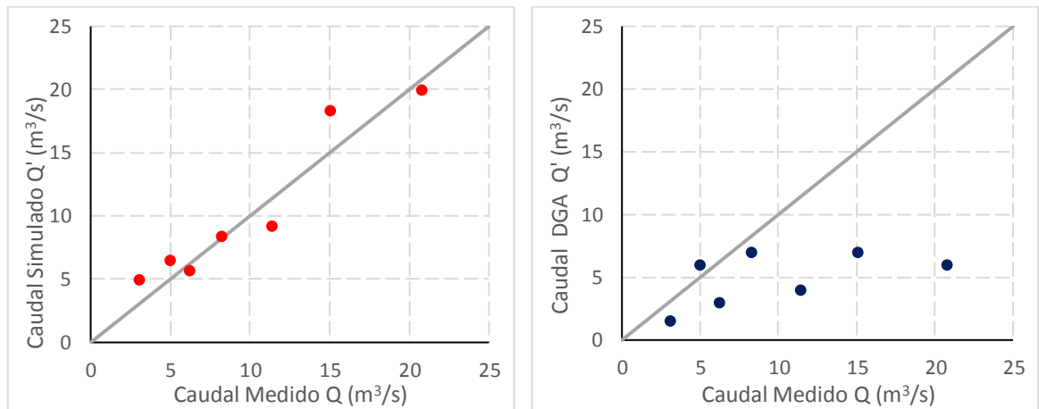
Gráfico 7.44: Comparativa entre Valores medidos en estación Fluviométrica, pronóstico SRM y pronóstico de la DGA – Primera Simulación Año 2015
