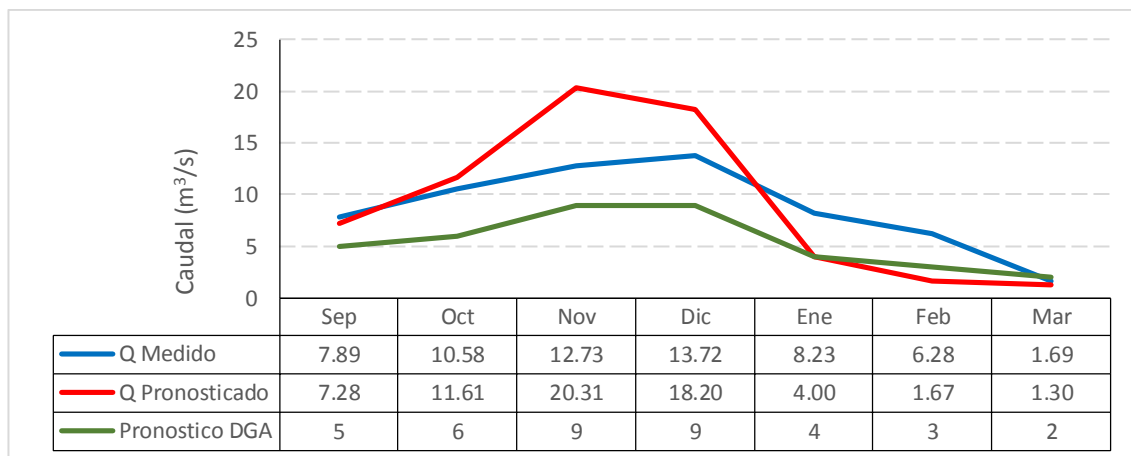
Gráfico 7.57: Caudal medido, pronosticado SRM y DGA Año 2016 con Actualización en Octubre – Río Putaendo en Resguardo los Patos
