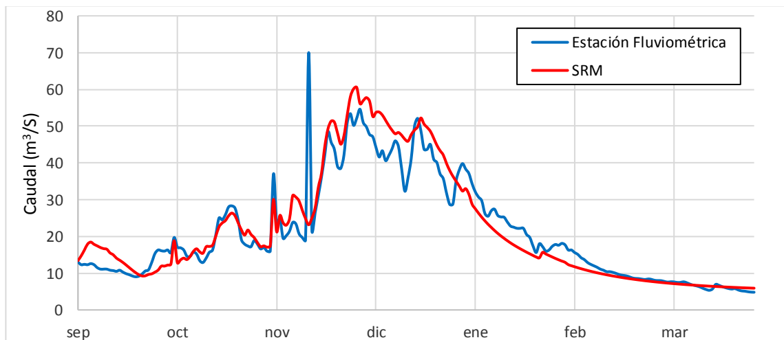
Gráfico 6.1: Caudales diarios medidos y simulados ( \text{m}^3/\text{s} ) - Cuenca Putaendo en Resguardo Los Patos (2002-2003)
