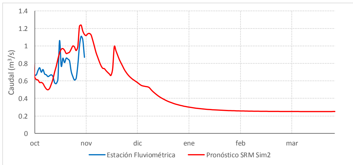
Gráfico 7.63: Pronóstico de Caudales con actualización en Octubre Año 2016 – Estero Pocuro en el Sifón
