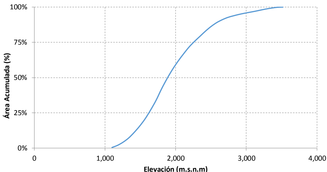
Gráfico 3.2: Curva Hipsométrica - Cuenca Estero Pocuro en Sifón
