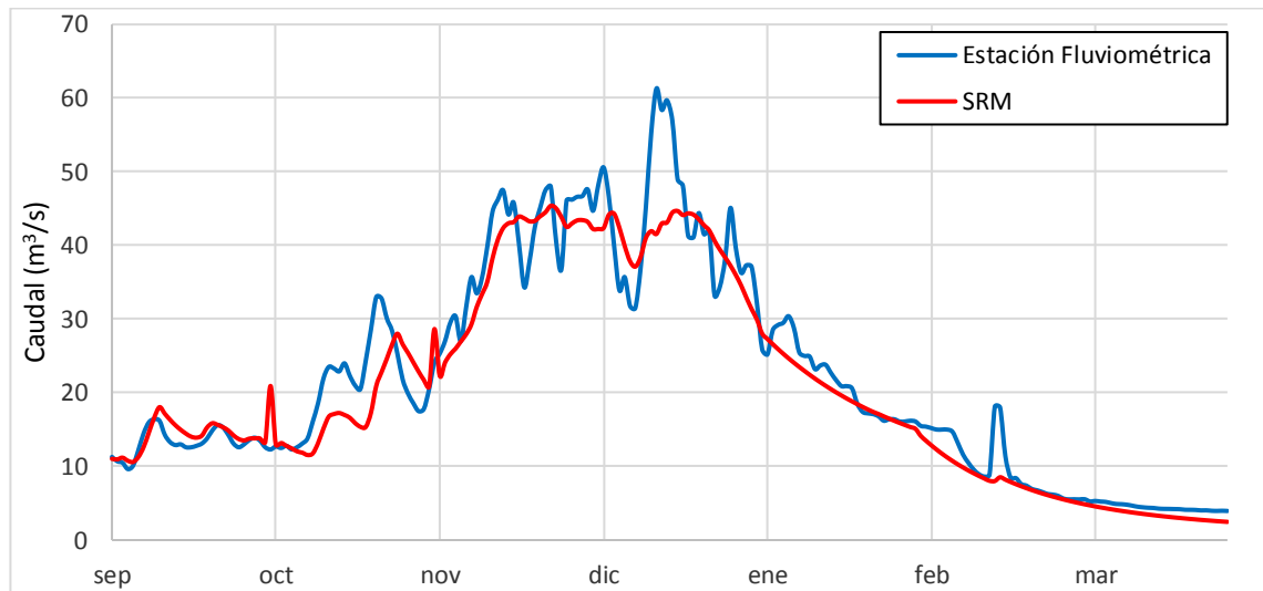
Gráfico 6.3: Caudales diarios medidos y simulados (m 3 /s) - Cuenca Putaendo en Resguardo Los Patos (2005-2006)
