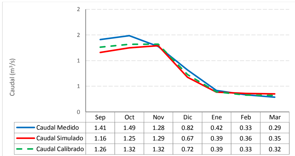
Gráfico 6.42: Caudales mensuales ( m^3/s ) –2001 -2002
