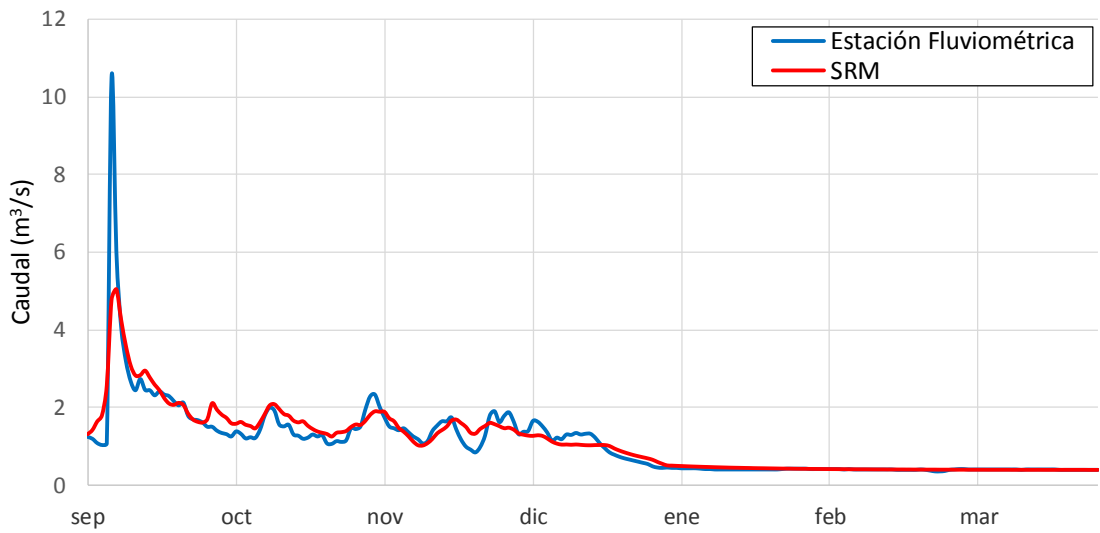
Gráfico 6.19: Caudales diarios medidos y simulados (m3/s) - Cuenca Pocuro en el Sifón (2009-2010)
