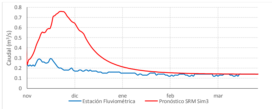
Gráfico 7.76: Pronóstico de Caudales con actualización en Noviembre Año 2014 – Estero Pocuro en el Sifón
