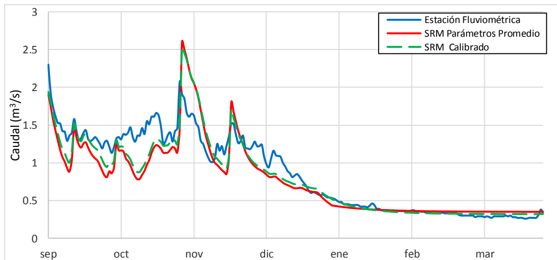
Gráfico 6.41: Caudales diarios medidos y simulados ( \text{m}^3/\text{s} ) –2001 -2002
