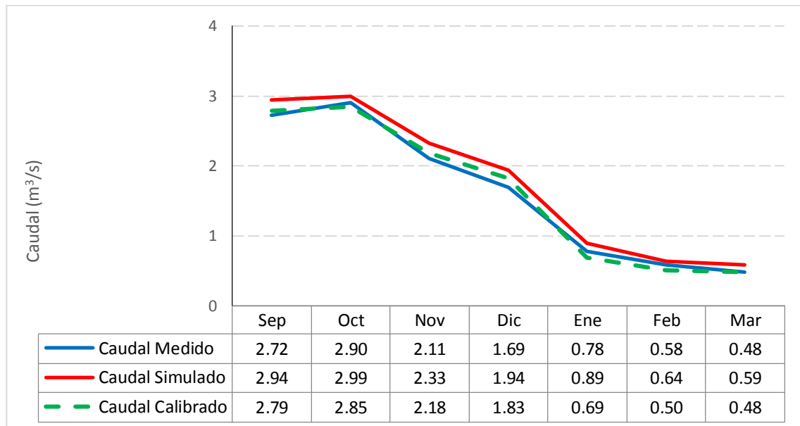
Gráfico 6.38: Caudales mensuales ( m^3/s ) –2000 -2001
