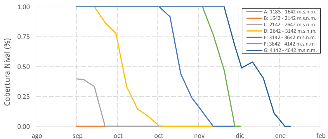
Gráfico 5.4: Cobertura Nival por bandas ciclo de deshielo año 2002 – Cuenca del Río Putaendo en Resguardo los Patos
