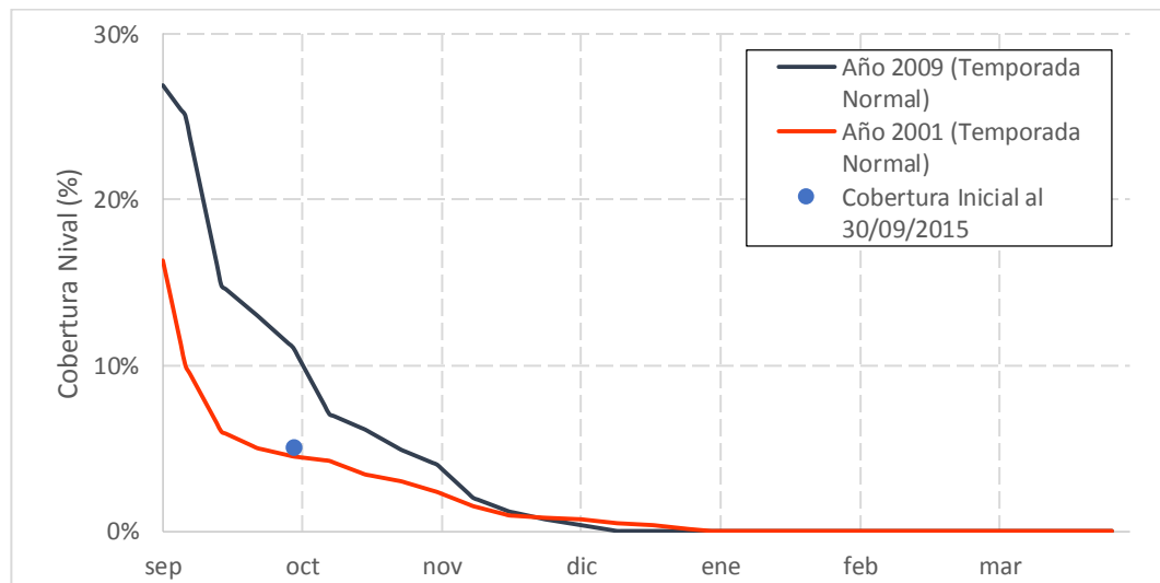
Gráfico 7.26: Cobertura Inicial Octubre 2015 y Cobertura de años Normales – Estero Pocuro en Sifón
