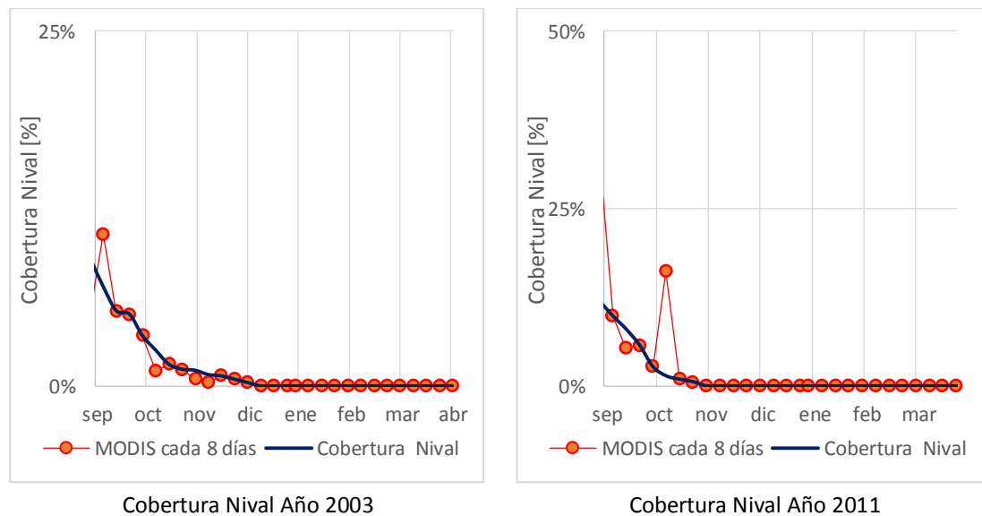
Gráfico 5.7: Cobertura Nival ciclo de deshielo Temporada Seca – Cuenca del Estero Pocuro en Sifón
