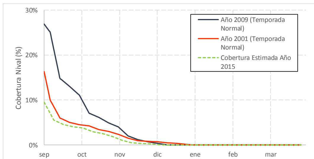
Gráfico 7.23: Cobertura pronosticada Septiembre Año 2015 – Estero Pocuro en Sifón
