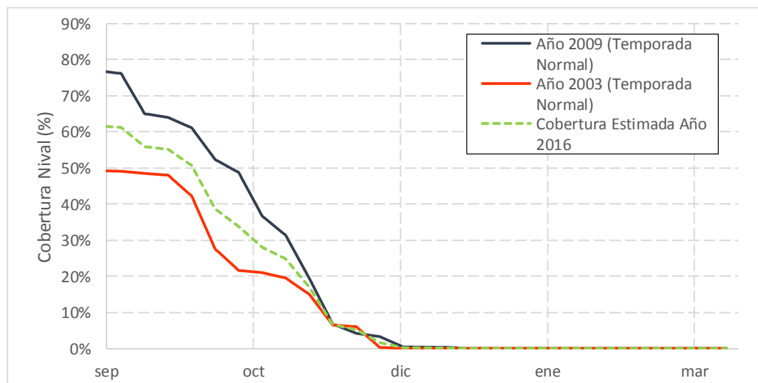
Gráfico 7.6: Cobertura pronosticada Septiembre Año 2016 – Río Putaendo en Resguardo los Patos
