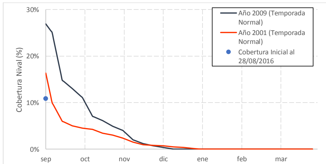
Gráfico 7.21: Cobertura Inicial Año 2016 y Cobertura de años Normales – Estero Pocuro en Sifón
