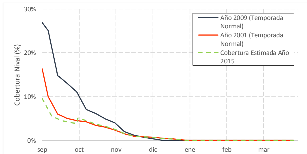
Gráfico 7.32: Cobertura Actualizada Octubre Año 2015 – Estero Pocuro en Sifón
