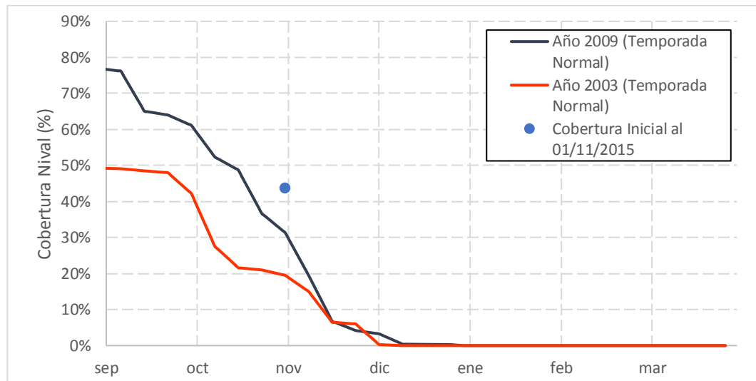
Gráfico 7.11: Cobertura Inicial Noviembre 2015 y Cobertura de años Normales – Río Putaendo en Resguardo los Patos
