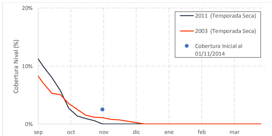
Gráfico 7.28: Cobertura Inicial Noviembre 2014 y Cobertura de años Normales – Estero Pocuro en Sifón
