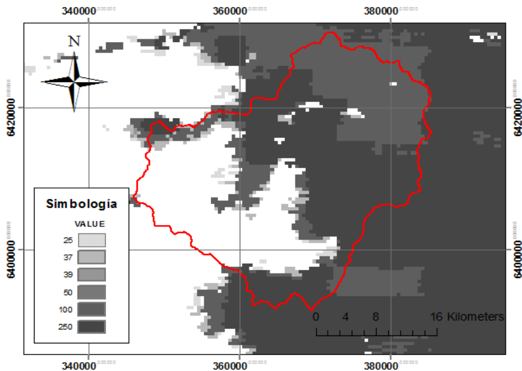
Figura 5.3: MOD10A2 Cobertura 8 días Putaendo Resguardo los Patos 14/09/2002
