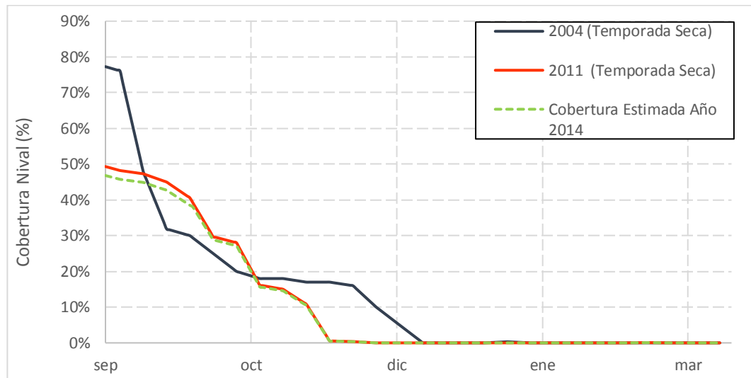
Gráfico 7.13: Cobertura Actualizada Octubre Año 2014 – Río Putaendo en Resguardo los Patos
