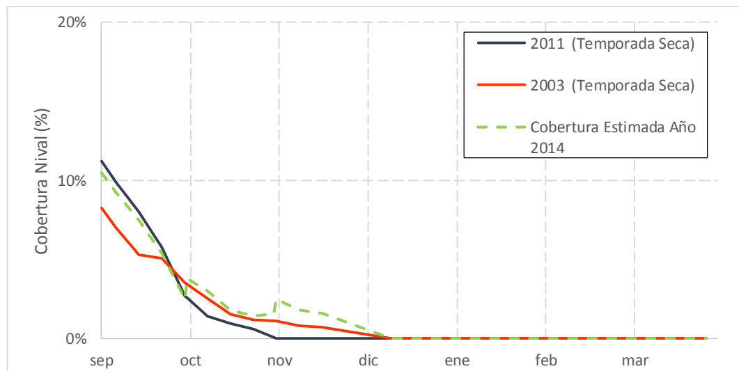
Gráfico 7.34: Cobertura Actualizada Noviembre Año 2014 – Estero Pocuro en Sifón
