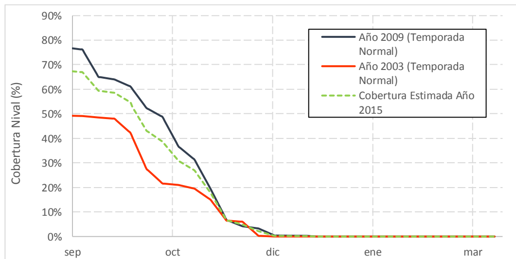
Gráfico 7.14: Cobertura Actualizada Octubre Año 2015 – Río Putaendo en Resguardo los Patos
