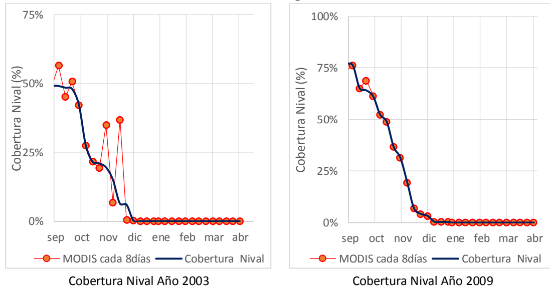
Gráfico 5.2: Cobertura Nival ciclo de deshielo Temporada Normal – Cuenca del Río Putaendo en Resguardo los Patos
