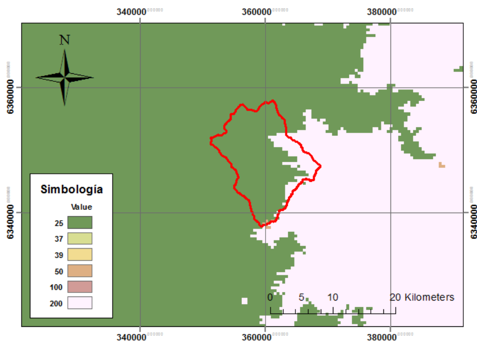
Figura 5.2: MOD10A2 Cobertura máxima Pocuro en Sifón 14/09/2002
