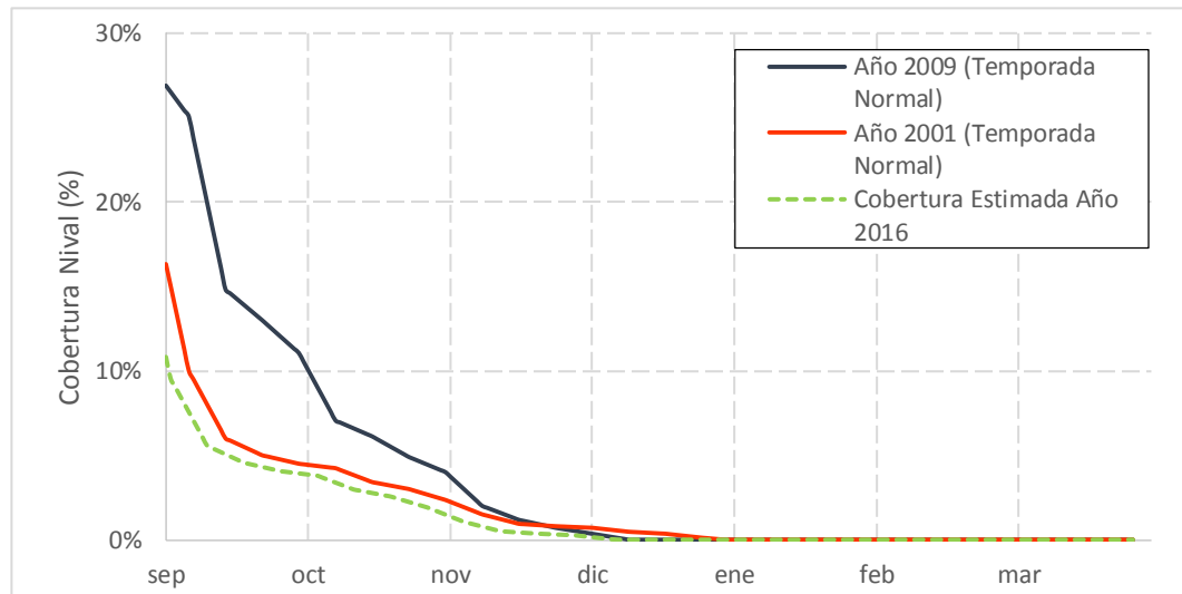
Gráfico 7.24: Cobertura pronosticada Septiembre Año 2016 – Estero Pocuro en Sifón
