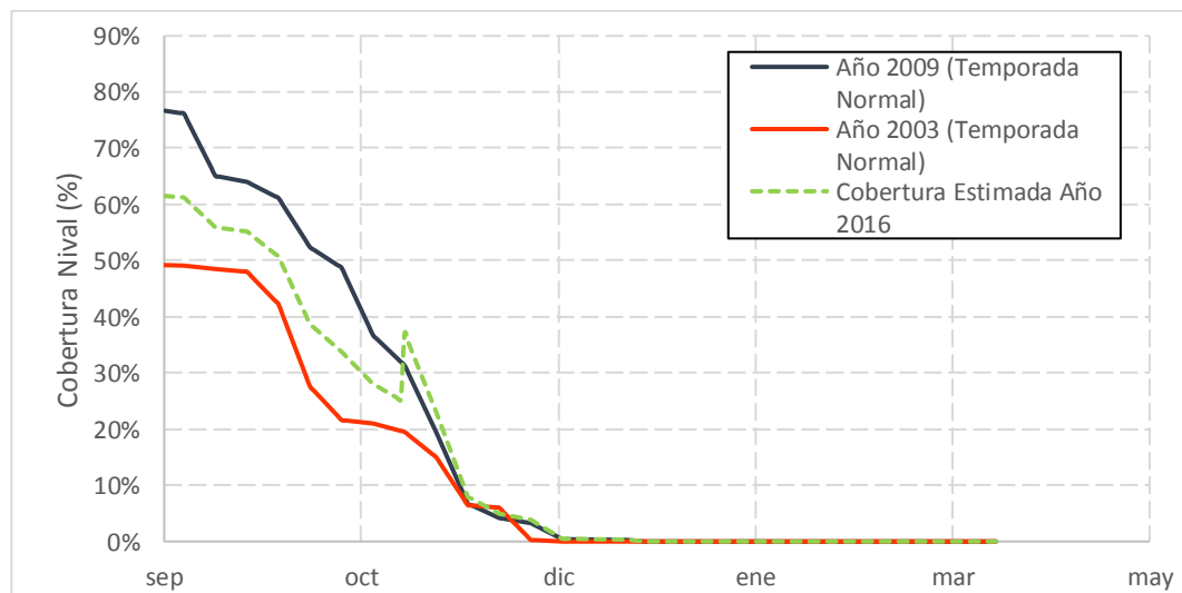
Gráfico 7.18: Cobertura Actualizada Noviembre Año 2016 – Río Putaendo en Resguardo los Patos
