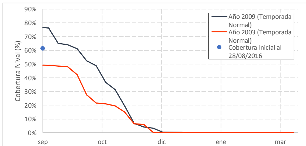
Gráfico 7.3: Cobertura Inicial Año 2016 y Cobertura de años Normales – Río Putaendo en Resguardo los Patos
