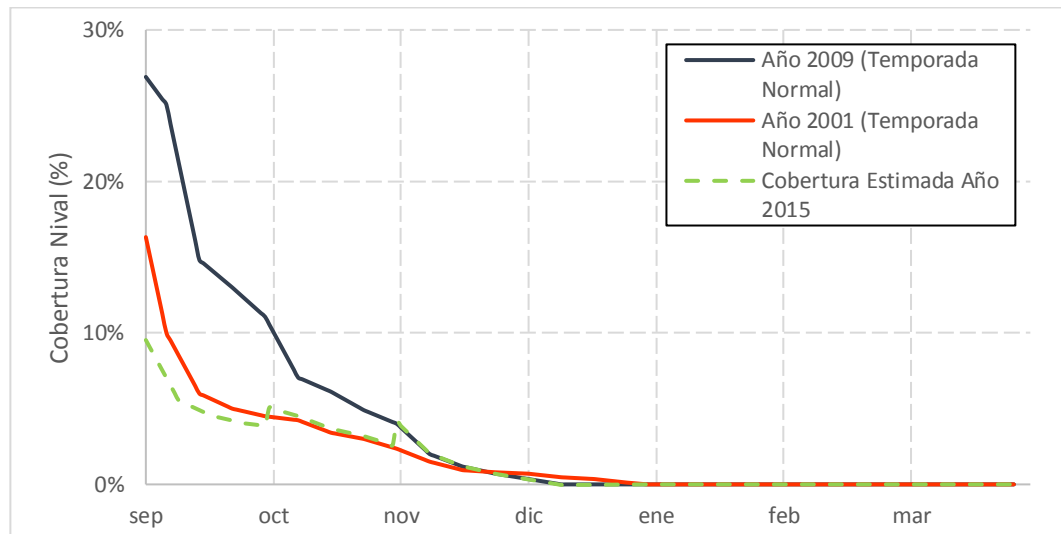
Gráfico 7.35: Cobertura Actualizada Noviembre Año 2015 – Estero Pocuro en Sifón
