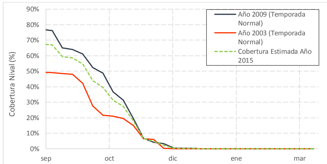
Gráfico 7.5: Cobertura pronosticada Septiembre Año 2015 – Río Putaendo en Resguardo los Patos
