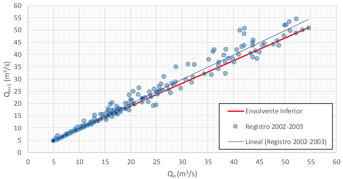
Figura 6.3: Caudales Q_n frente Q_{n+1} E.F. Putaendo en Resguardo los Patos - Determinación del coeficiente de recesión
