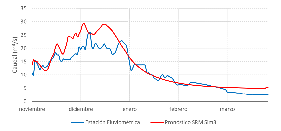
Gráfico 7.68: Pronóstico de Caudales con actualización en Noviembre Año 2015 – Río Putaendo en Resguardo los Patos
