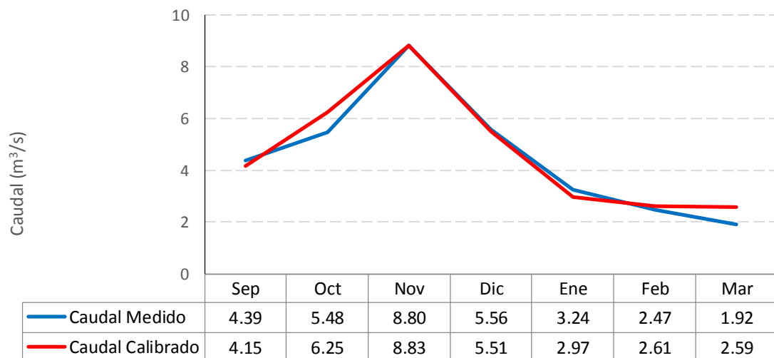
Gráfico 6.12: Caudales mensuales medidos y simulados (m 3 /s) - Cuenca Putaendo en Resguardo Los Patos (2011-2012)
