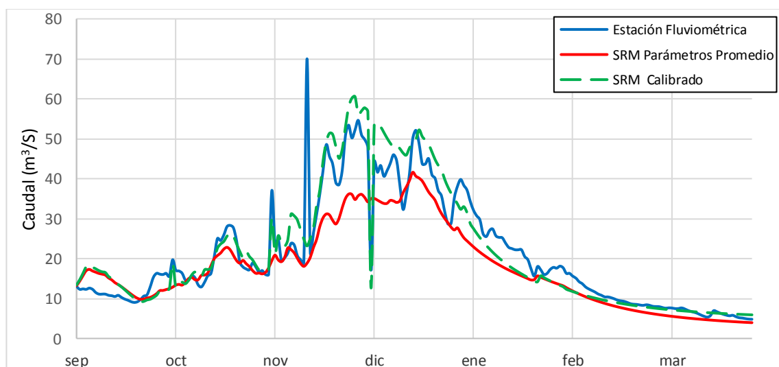
Gráfico 6.25: Caudales diarios medidos y simulados ( \text{m}^3/\text{s} ) –2002 -2003
