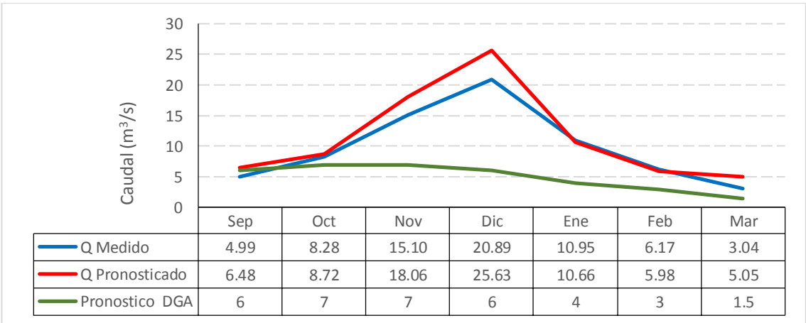
Gráfico 7.71: Caudal medido, pronosticado SRM y DGA Año 2015 con Actualización en Noviembre – Río Putaendo en Resguardo los Patos
