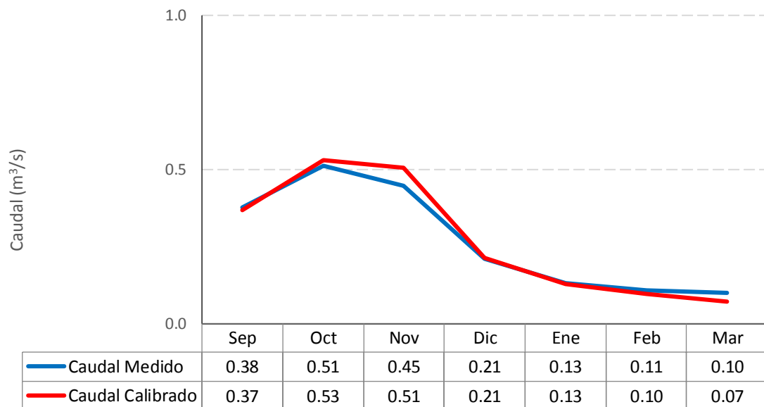
Gráfico 6.22: Caudales mensuales medidos y simulados (m 3 /s) - Cuenca Pocuro en el Sifón (2003-2004)
