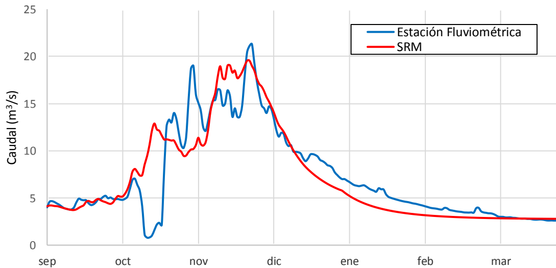
Gráfico 6.5: Caudales diarios medidos y simulados ( \text{m}^3/\text{s} ) - Cuenca Putaendo en Resguardo Los Patos (2003-2004)
