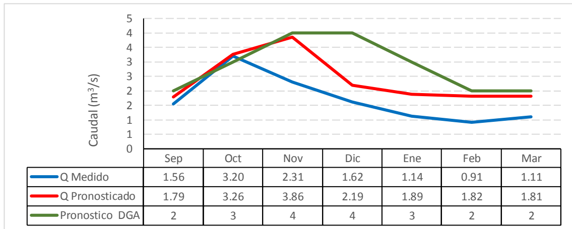
Gráfico 7.40: Caudal medido, pronosticado SRM y DGA Año 2015 – Río Putaendo en Resguardo los Patos
