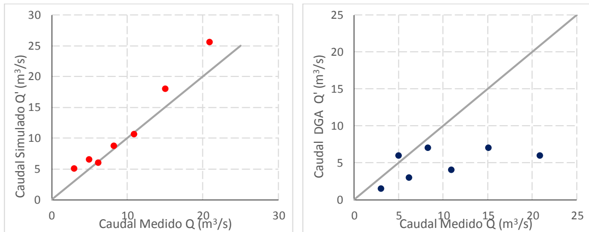
Gráfico 7.74: Comparativa entre Valores medidos en estación Fluviométrica, pronóstico SRM y pronóstico de la DGA – Tercera Simulación Año 2015
