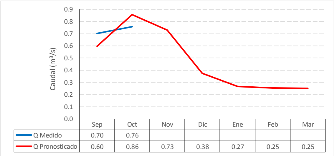
Gráfico 7.51: Caudal medido y pronosticado SRM Año 2016 – Estero Pocuro en el Sifón
