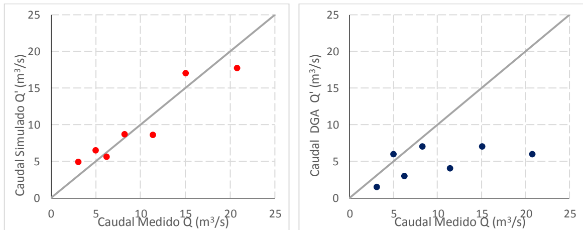
Gráfico 7.59: Comparativa entre Valores medidos en estación Fluviométrica, pronóstico SRM y pronóstico de la DGA – Segunda Simulación Año 2015
