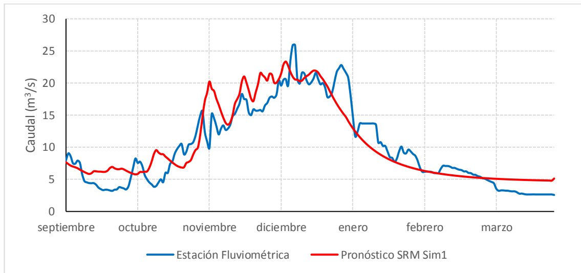
Gráfico 7.38: Pronostico de Caudales Año 2015 – Río Putaendo en Resguardo los Patos
