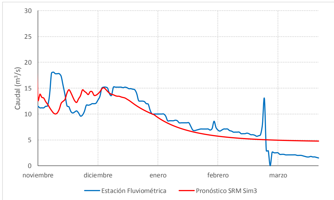
Gráfico 7.69: Pronóstico de Caudales con actualización en Noviembre Año 2016 – Río Putaendo en Resguardo los Patos
