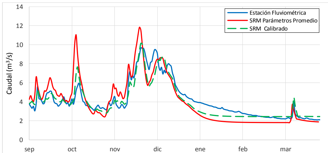
Gráfico 6.33: Caudales diarios medidos y simulados ( \text{m}^3/\text{s} ) –2004 -2011
