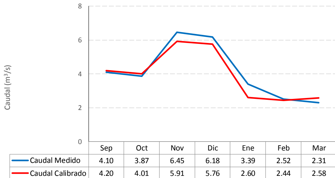
Gráfico 6.10: Caudales mensuales medidos y simulados (m 3 /s) - Cuenca Putaendo en Resguardo Los Patos (2004-2005)
