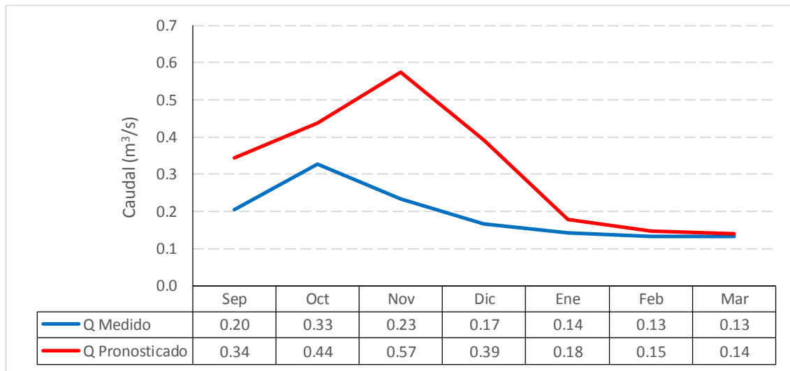
Gráfico 7.79: Caudal medido y pronosticado SRM Año 2014 con Actualización en Noviembre – Estero Pocuro en el Sifón
