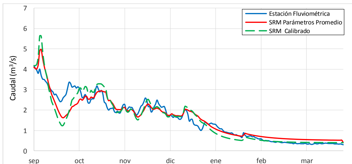
Gráfico 6.39: Caudales diarios medidos y simulados ( m^3/s ) –2002 -2003
