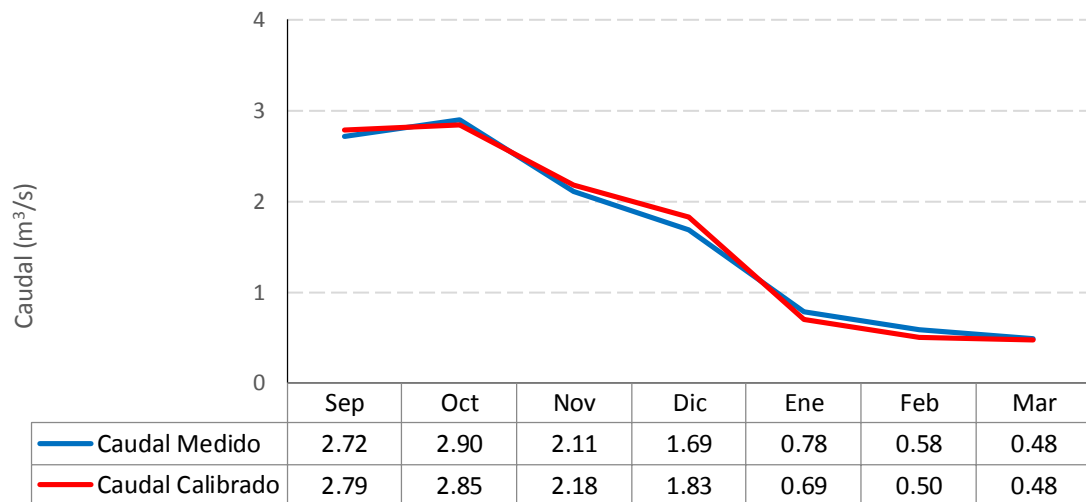
Gráfico 6.14: Caudales mensuales medidos y simulados (m 3 /s) - Cuenca Pocuro en el Sifón (2000-2001)
