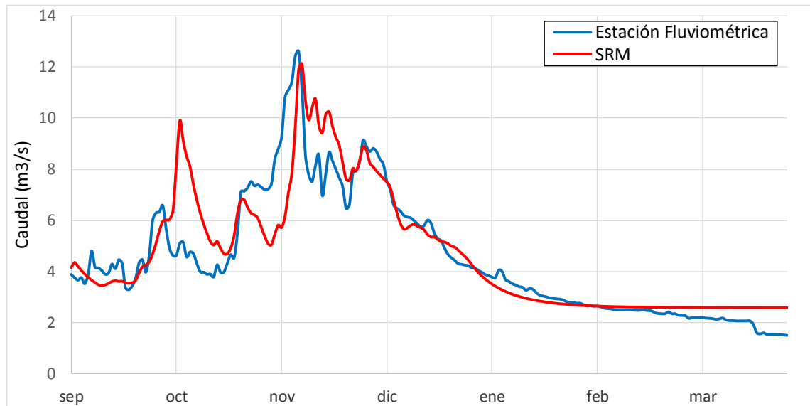
Gráfico 6.11: Caudales diarios medidos y simulados (m 3 /s) - Cuenca Putaendo en Resguardo Los Patos (2011-2012)
