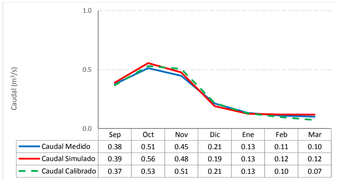
Gráfico 6.46: Caudales mensuales ( m^3/s ) – 2003 -2004
