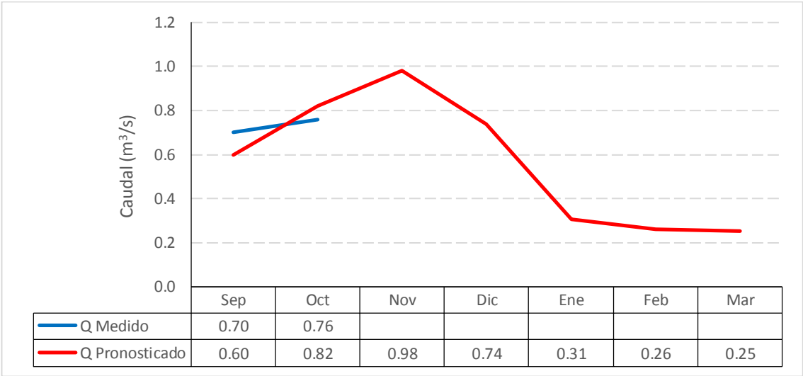
Gráfico 7.81: Caudal medido y pronosticado SRM Año 2016 con Actualización en Noviembre – Estero Pocuro en el Sifón
