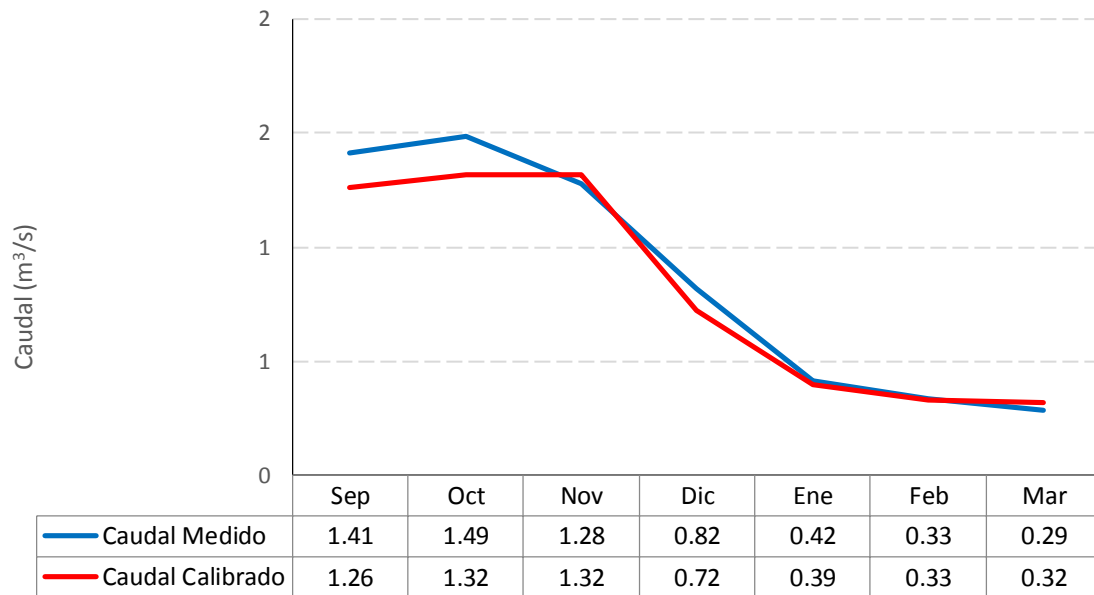
Gráfico 6.18: Caudales mensuales medidos y simulados (m 3 /s) - Cuenca Pocuro en el Sifón (2001-2002)
