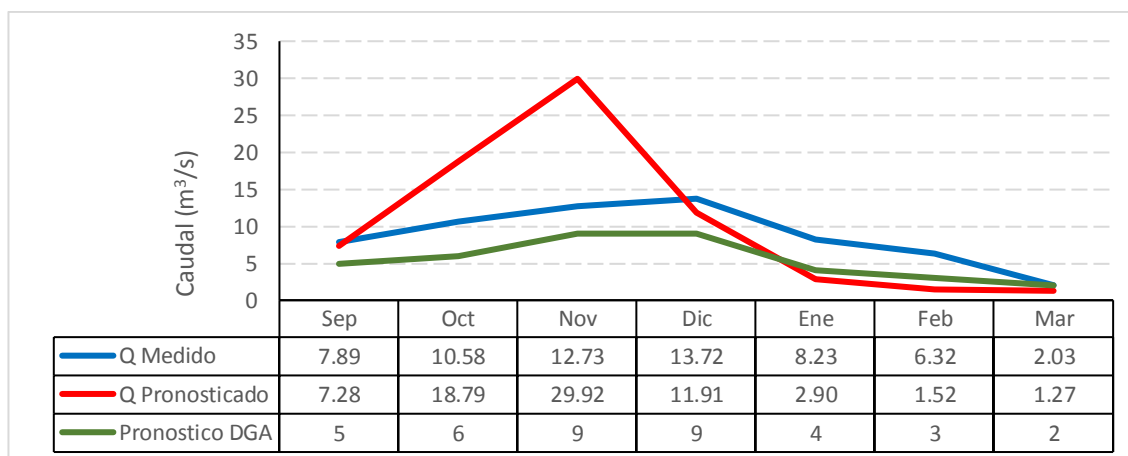
Gráfico 7.42: Caudal medido, pronosticado SRM y DGA Año 2016 – Río Putaendo en Resguardo los Patos
