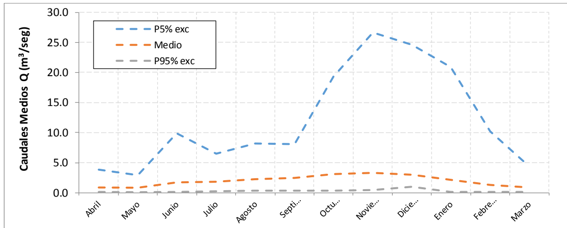
Gráfico 3.4: Curva Variación Estacional - Estero Pocuro en Sifón
