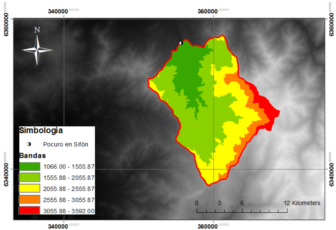
Figura 6.2: Distribución de Bandas Cuenca Pocuro en el Sifón
