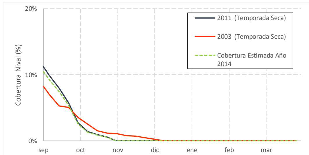
Gráfico 7.22: Cobertura pronosticada Septiembre Año 2015 – Estero Pocuro en Sifón
