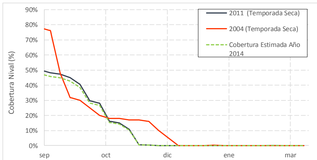
Gráfico 7.4: Cobertura pronosticada Septiembre Año 2014 – Río Putaendo en Resguardo los Patos
