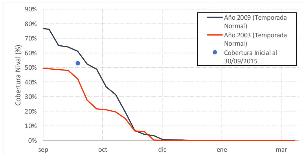
Gráfico 7.8: Cobertura Inicial Octubre 2015 y Cobertura de años Normales – Río Putaendo en Resguardo los Patos
