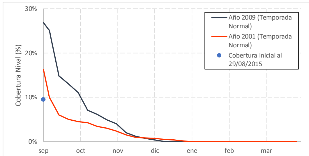
Gráfico 7.20: Cobertura Inicial Año 2015 y Cobertura de años Normales – Estero Pocuro en Sifón
