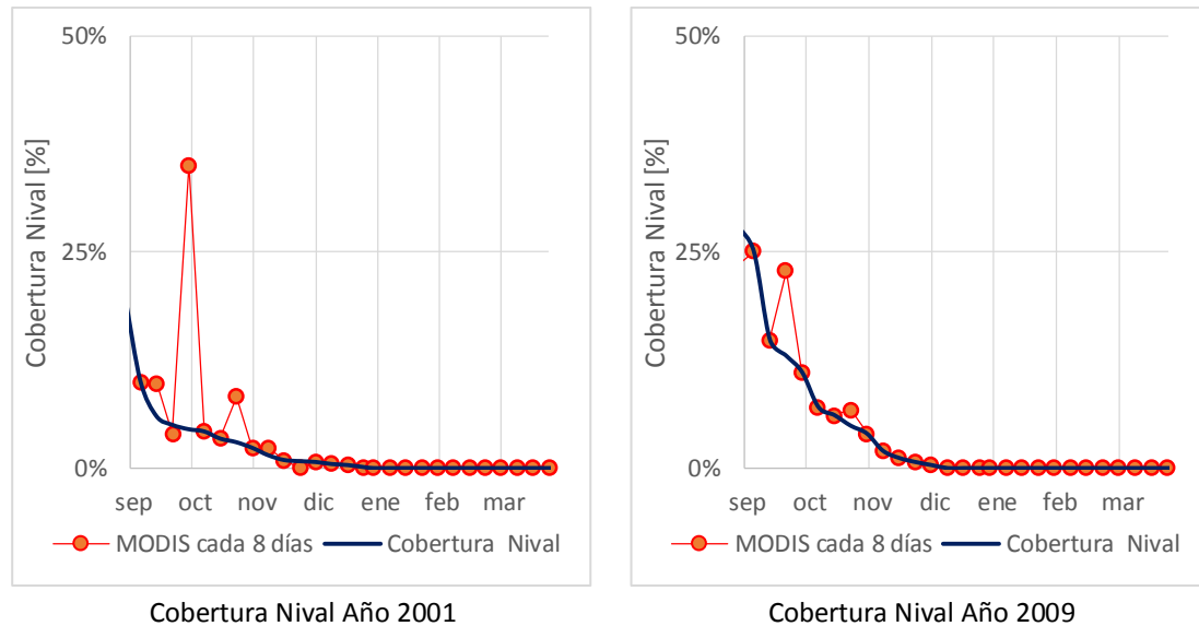
Gráfico 5.6: Cobertura Nival ciclo de deshielo Temporada Normal – Cuenca del Estero Pocuro en Sifón
