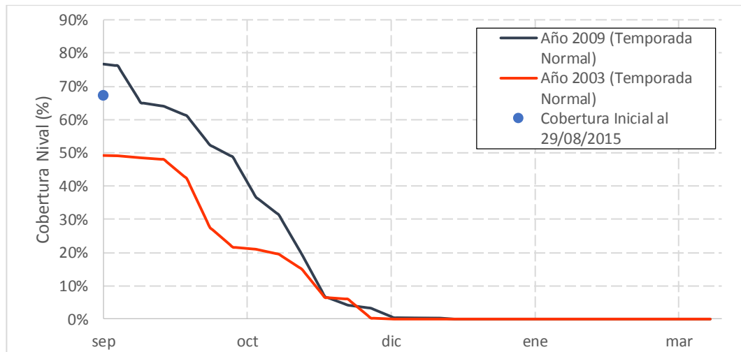
Gráfico 7.2: Cobertura Inicial Año 2015 y Cobertura de años Normales – Río Putaendo en Resguardo los Patos
