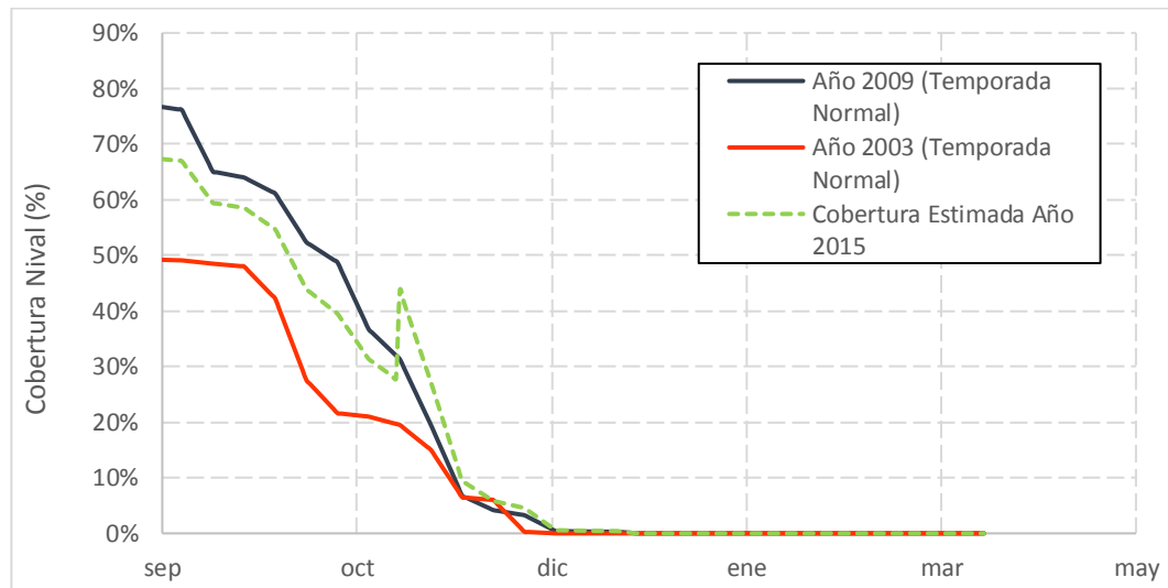
Gráfico 7.17: Cobertura Actualizada Noviembre Año 2015 – Río Putaendo en Resguardo los Patos
