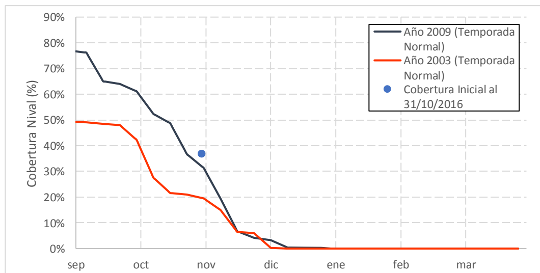
Gráfico 7.12: Cobertura Inicial Noviembre 2016 y Cobertura de años Normales – Río Putaendo en Resguardo los Patos
