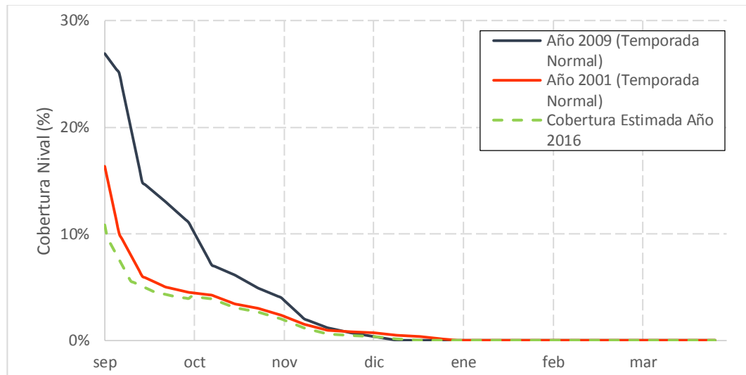
Gráfico 7.33: Cobertura Actualizada Octubre Año 2016 – Estero Pocuro en Sifón
