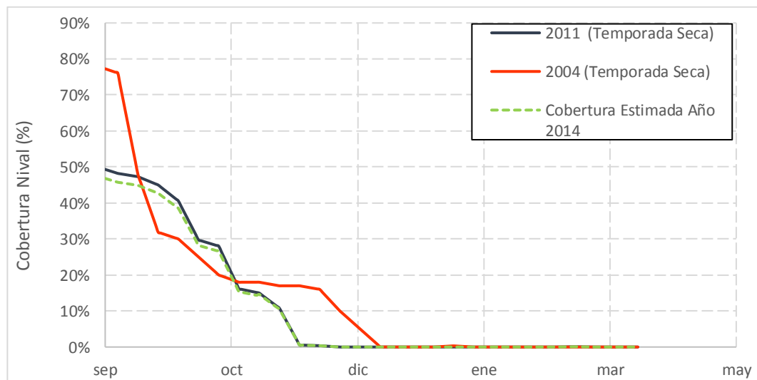
Gráfico 7.16: Cobertura Actualizada Noviembre Año 2014 – Río Putaendo en Resguardo los Patos
