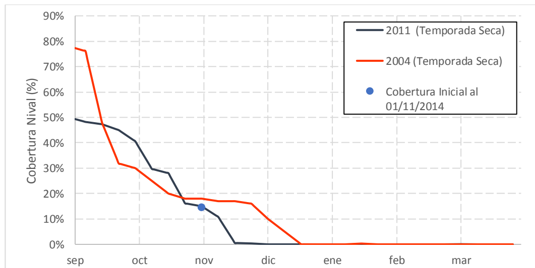
Gráfico 7.10: Cobertura Inicial Noviembre 2014 y Cobertura de años Normales – Río Putaendo en Resguardo los Patos
