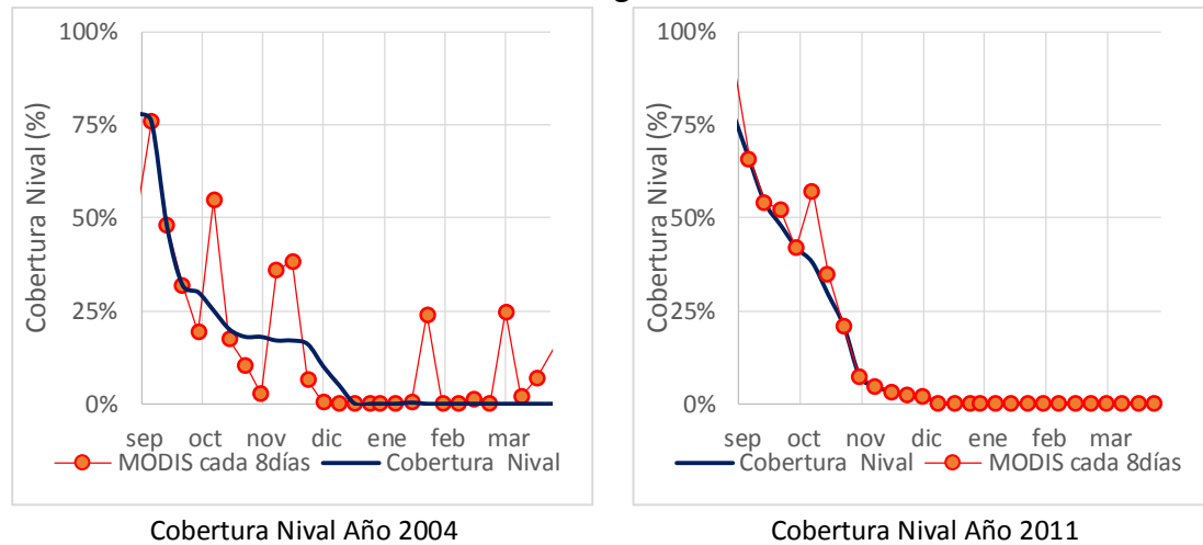
Gráfico 5.3: Cobertura Nival ciclo de deshielo Temporada Seca – Cuenca del Río Putaendo en Resguardo los Patos
