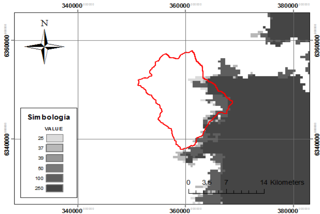
Figura 5.4: MOD10A2 Cobertura 8 días Pocuro en Sifón 14/09/2002
