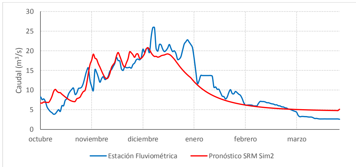
Gráfico 7.53: Pronóstico de Caudales con actualización en Octubre Año 2015 – Río Putaendo en Resguardo los Patos
