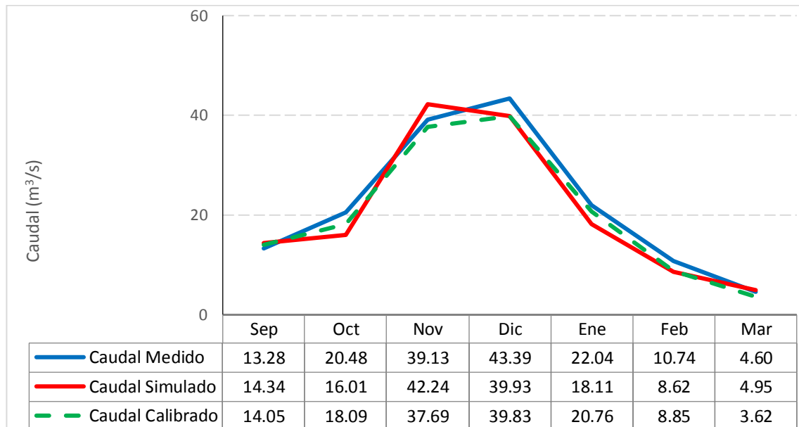
Gráfico 6.28: Caudales mensuales ( \text{m}^3/\text{s} ) –2005 -2006
