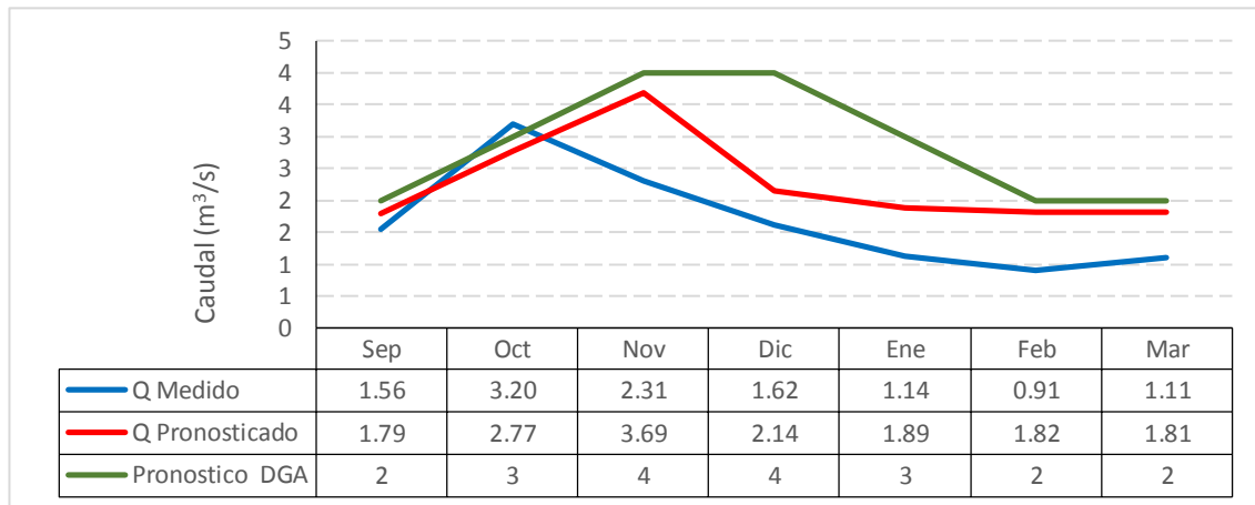
Gráfico 7.55: Caudal medido, pronosticado SRM y DGA Año 2014 con Actualización en Octubre – Río Putaendo en Resguardo los Patos
