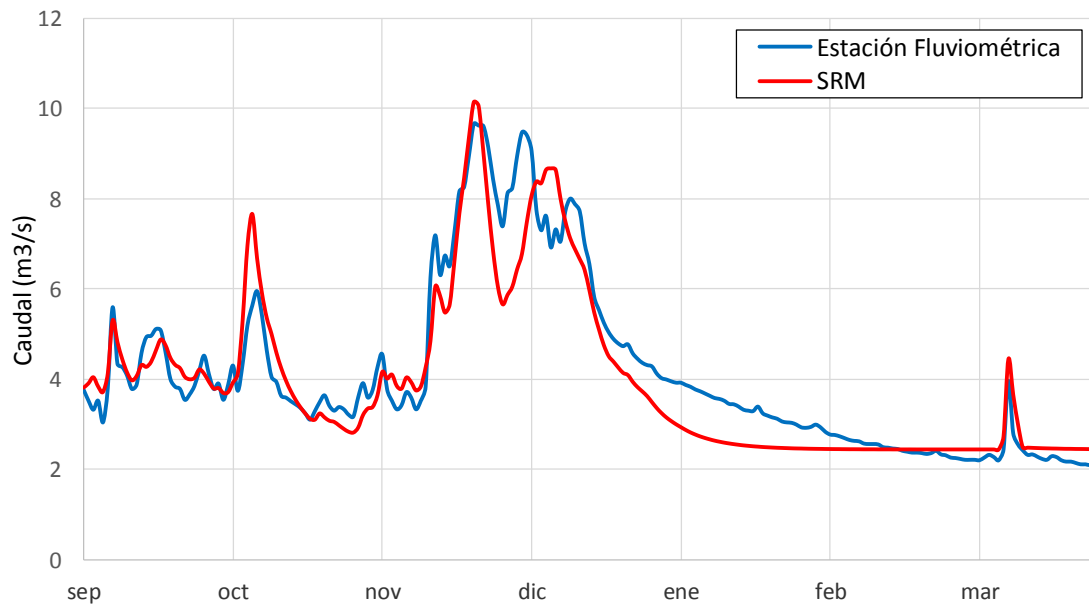
Gráfico 6.9: Caudales diarios medidos y simulados ( \text{m}^3/\text{s} ) - Cuenca Putaendo en Resguardo Los Patos (2004-2005)
