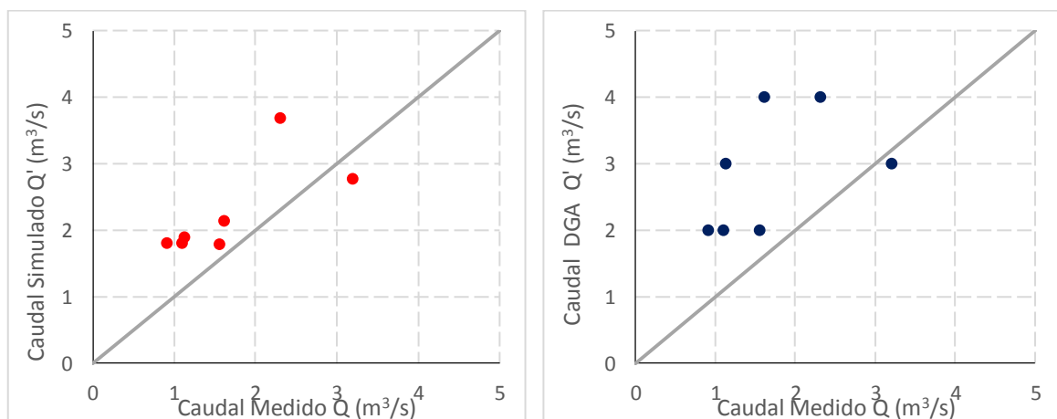
Gráfico 7.58: Comparativa entre Valores medidos en estación Fluviométrica, pronóstico SRM y pronóstico de la DGA – Segunda Simulación Año 2014
