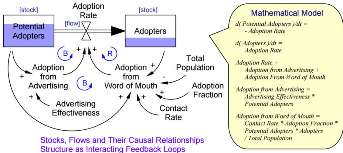
Figura 3.1 Representación clásica de los elementos y las relaciones de un modelo de Sistema Dinámico. (Borshchev & Filippov, 2004)
