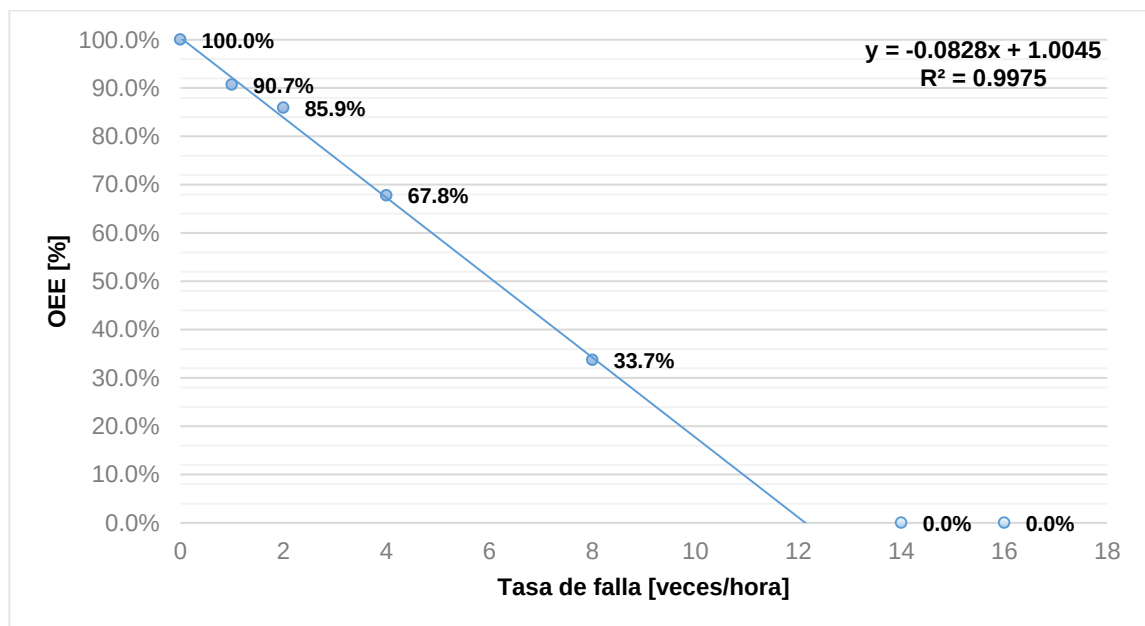
Figura 8.2. Análisis de sensibilidad del OEE al variar la tasa de falla de la cuadrilla de Enfierradura
