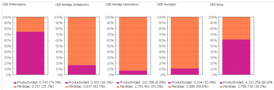
Figura 9.3. OEE de las cuadrillas y grúa con valores nominales
