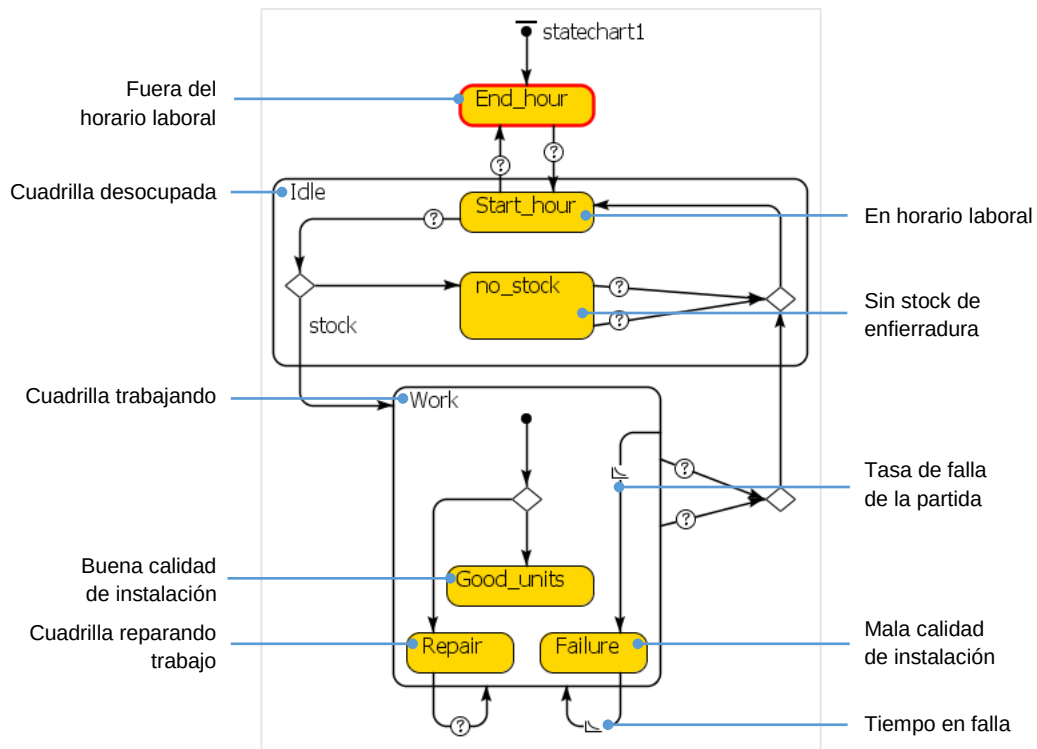
Figura 7.2. Diagrama de estado de la cuadrilla de enfierradura. (en Anylogic)
