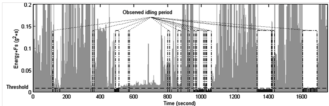
Figura 3.10. Comparación de los períodos de ocio entre la observación (cuadro de puntos) y el análisis energético de las señales de vibración (barras grises oscuro). (Ahn, Lee, & Peña-Mora, 2012)
