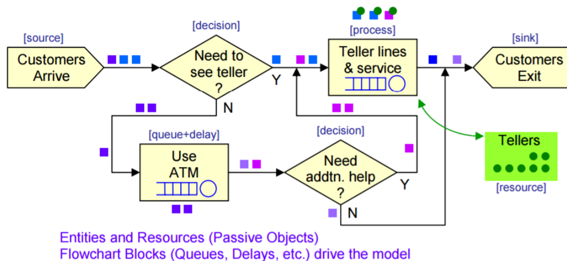
Figura 3.2. Representación de los elementos y las relaciones de un modelo de Eventos Discretos. (Borshchev & Filippov, 2004)
