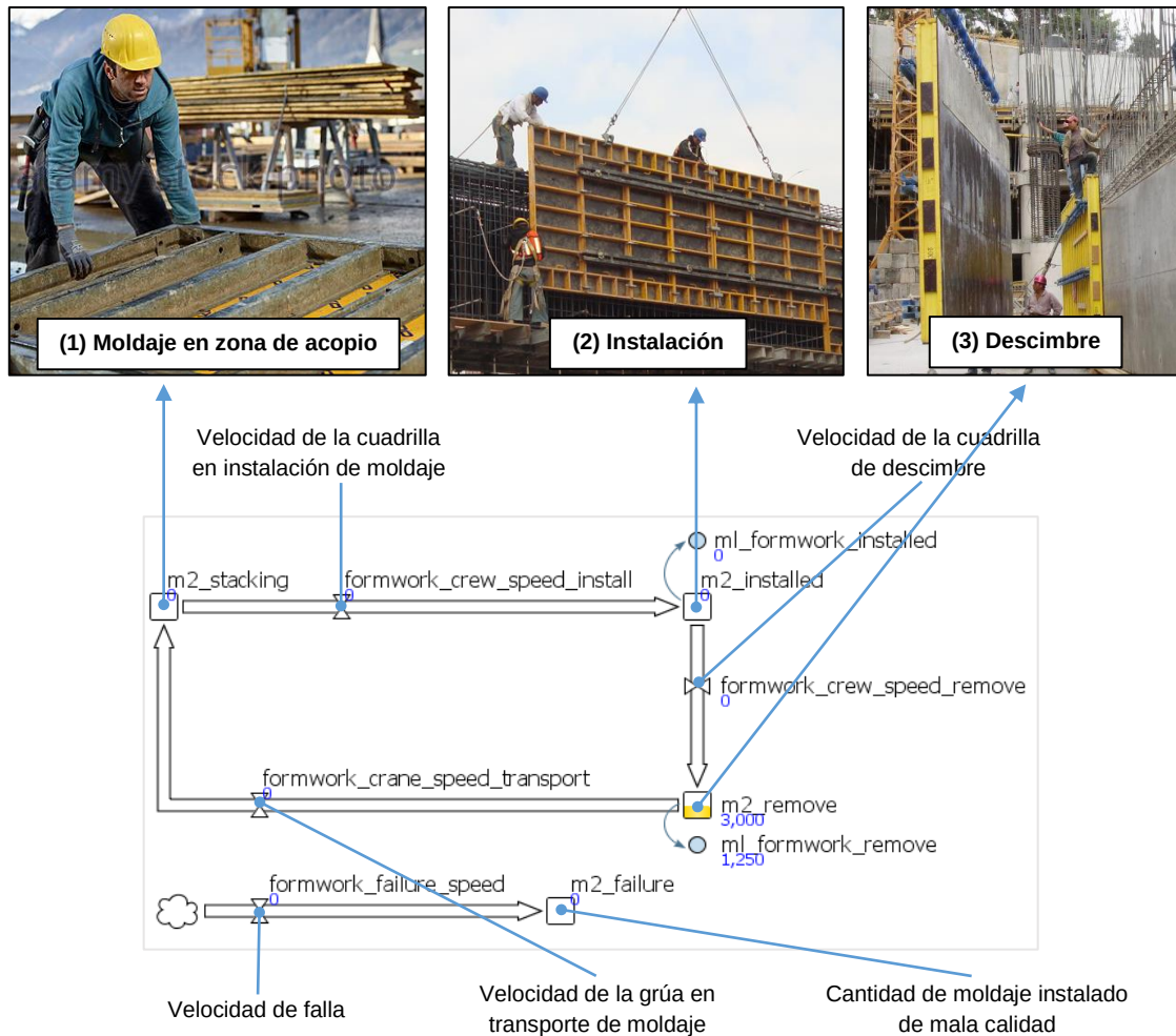
Figura 7.3. Diagrama Forrester de la partida de moldaje y sus elementos. (en Anylogic)
