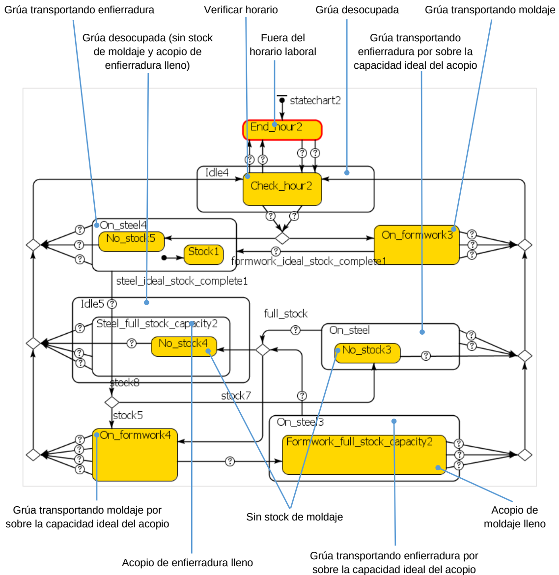
Figura 7.10. Diagrama de estado del tercer comportamiento de la grúa. (en Anylogic)
