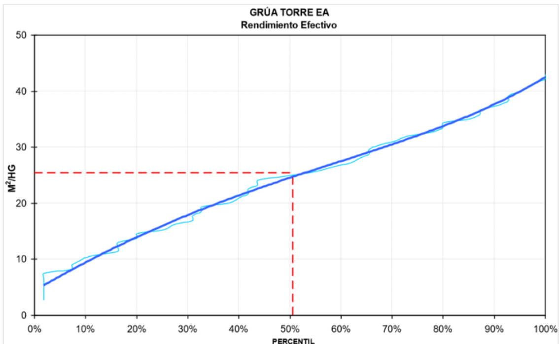
Figura 7.14. Gráfico Benchmarking de rendimientos de la grúa para Edificación en Altura. (CALIBRE, 2013)
