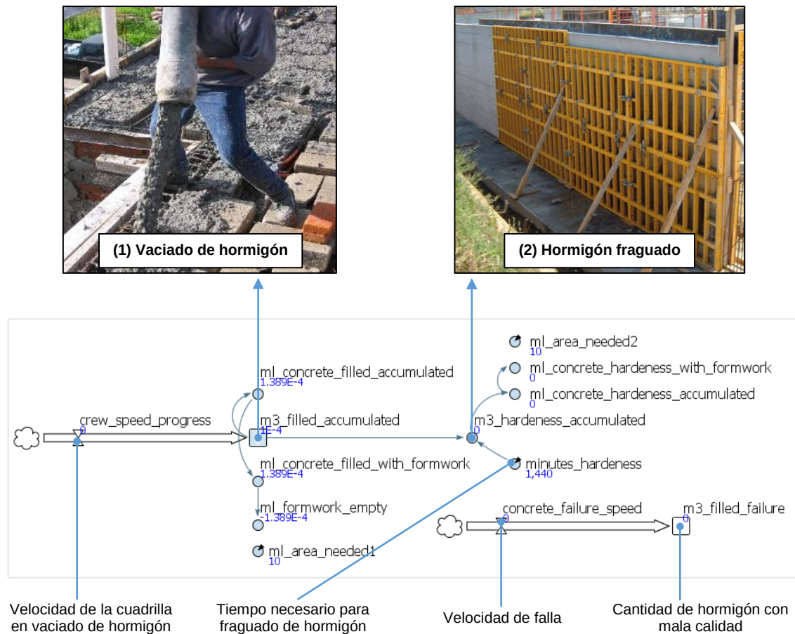
Figura 7.6. Diagrama Forrester de la partida de hormigonado. (en Anylogic)
