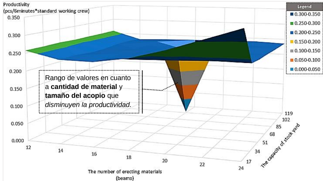
Figura 3.7. Resultados visuales del análisis de sensibilidad. (WoonSeong et al., 2016)
