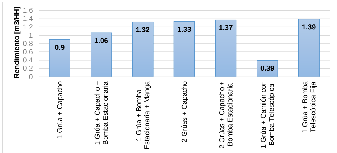
Figura 7.12. Gráfico del rendimiento de vaciado del hormigón según metodología. (CDT, 2013)
