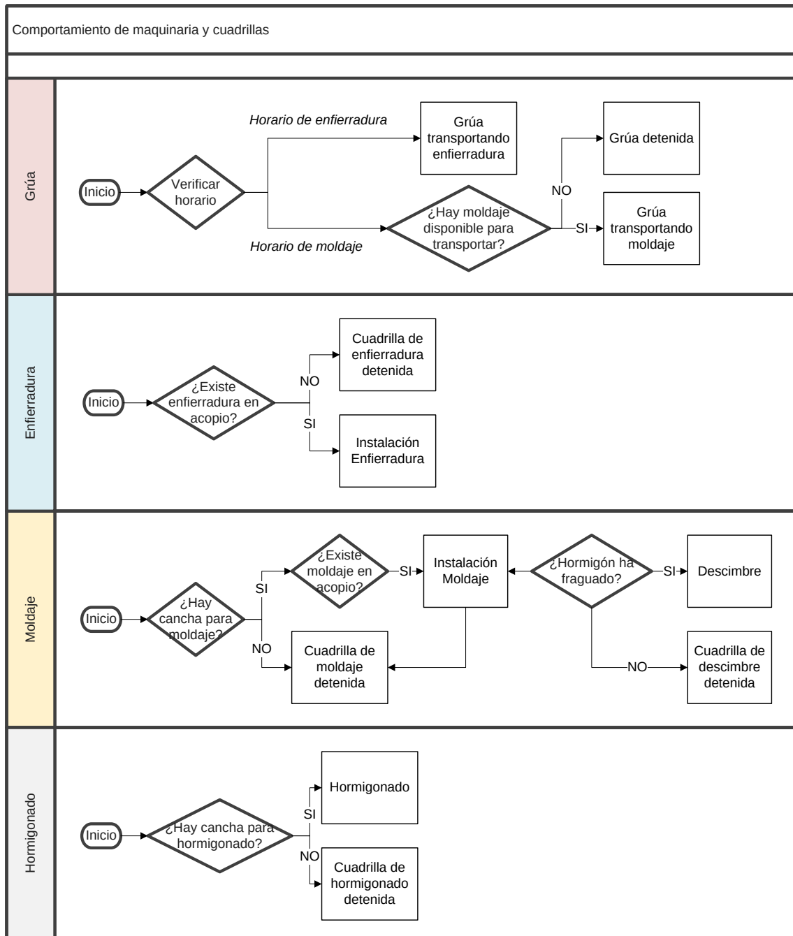
Figura 6.3. Diagrama de flujo del comportamiento de la grúa y de las cuadrillas de enfierradura, moldaje y hormigonado.
