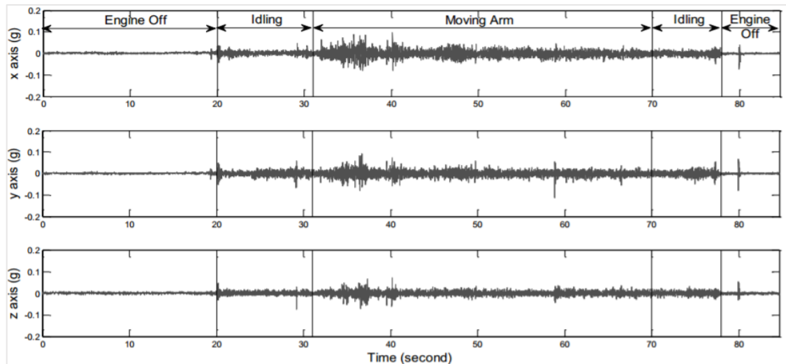
Figura 3.9. Señal de vibración en los ejes x,y,z. (Ahn, Lee, & Peña-Mora, 2012)
