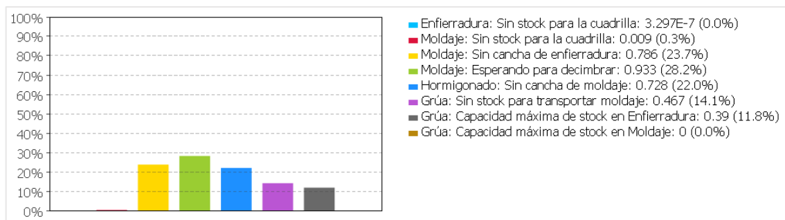
Figura 9.1. Uso del tiempo en actividades que representan pérdidas para el sistema con valores nominales
