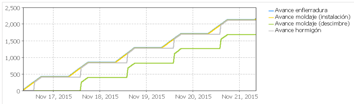
Figura 9.2. Avance de las partidas de obra gruesa con valores nominales
