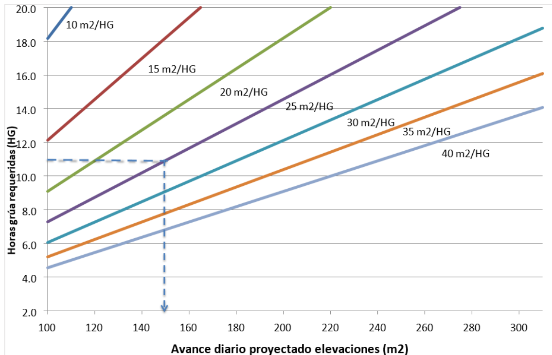
Figura 7.15. Gráfico rendimientos, según utilización de grúa. 55% en moldaje, 1 grúa. (CDT, 2013)
