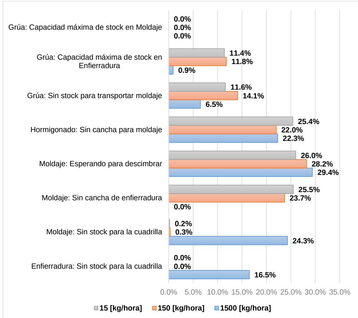
Figura 9.6. Evaluación de los desperdicios del sistema al variar el rendimiento máximo de la cuadrilla de enfierradura
