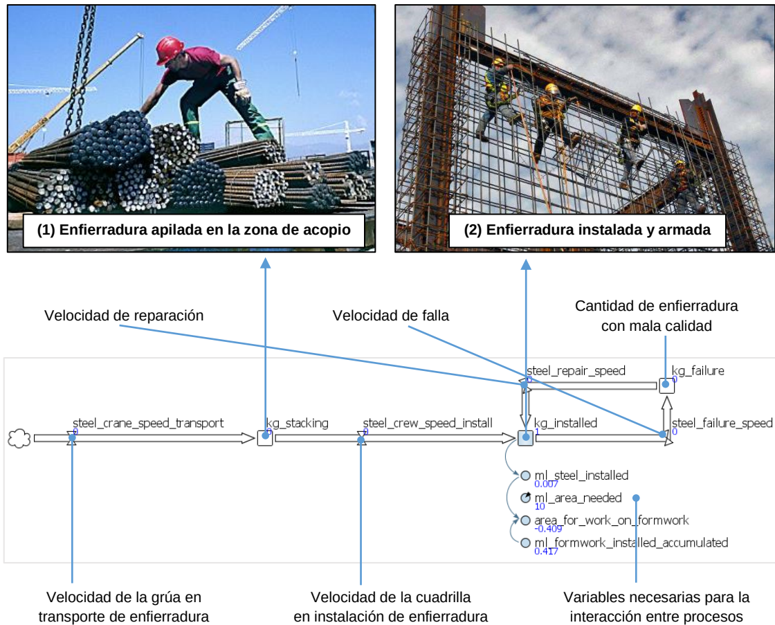
Figura 7.1. Diagrama Forrester del proceso de enfierradura y sus elementos. (en Anylogic)
