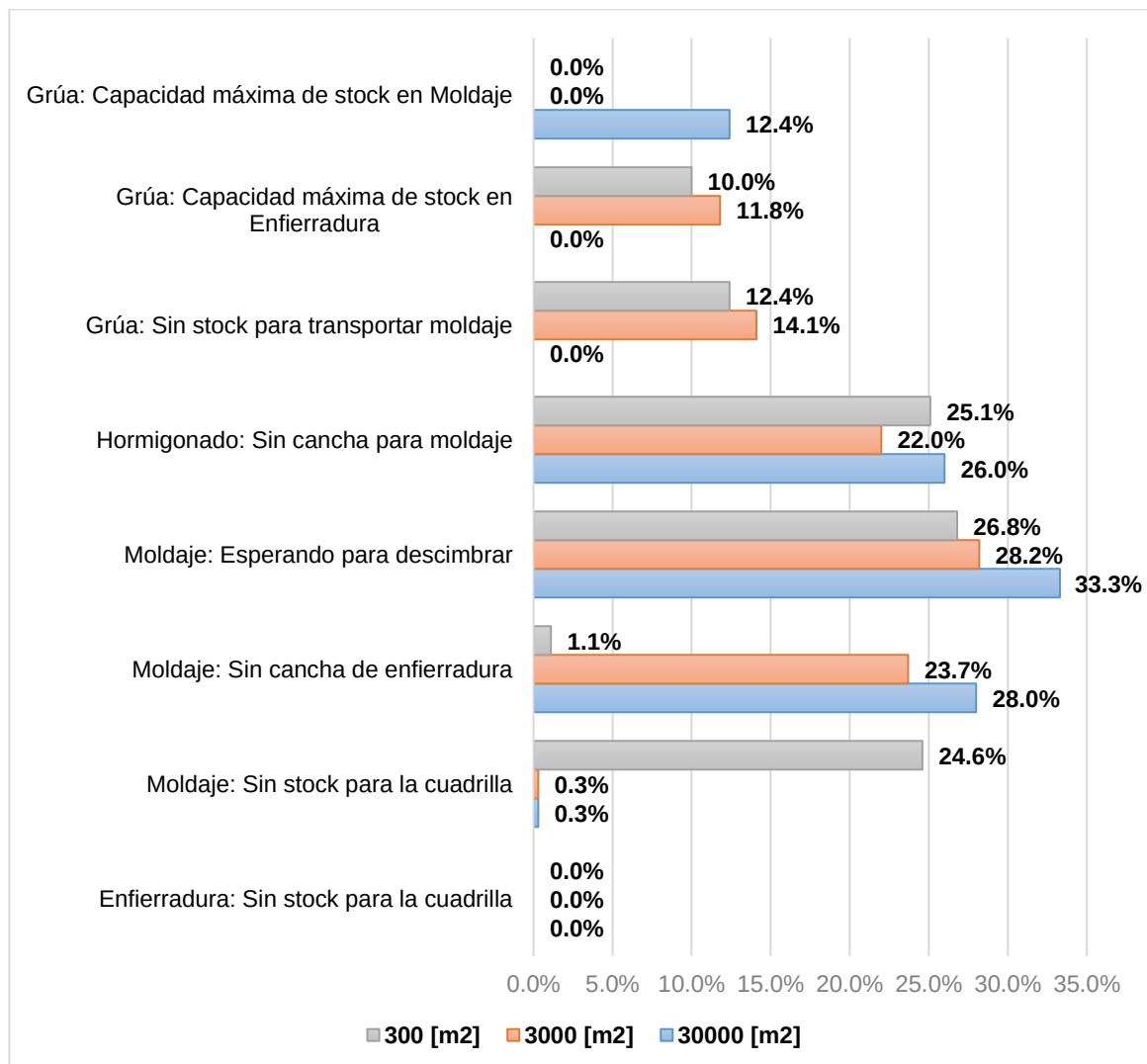
Figura 9.5. Evaluación de los desperdicios del sistema al variar la cantidad de moldaje en obra
