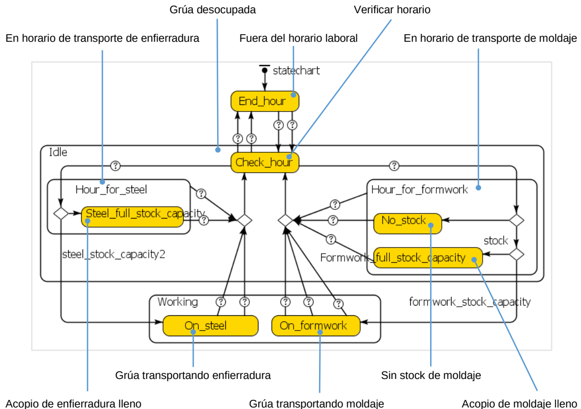
Figura 7.8. Diagrama de estado del primer comportamiento de la grúa. (en Anylogic)
