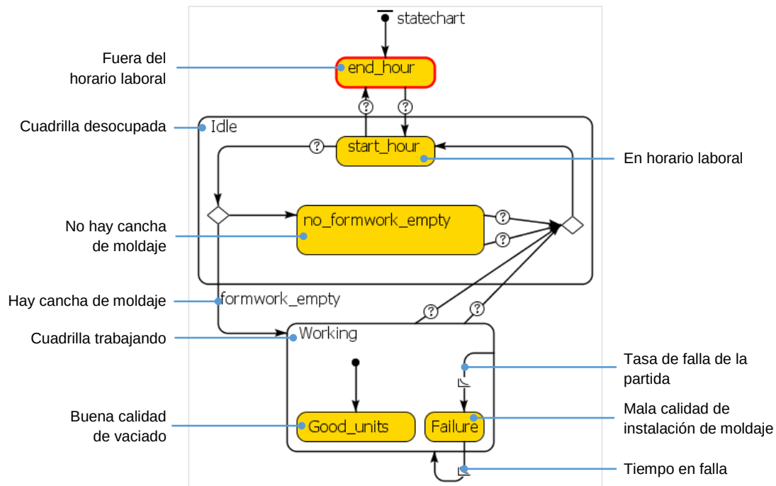
Figura 7.7. Diagrama de estado de la cuadrilla de hormigonado. (en Anylogic)
