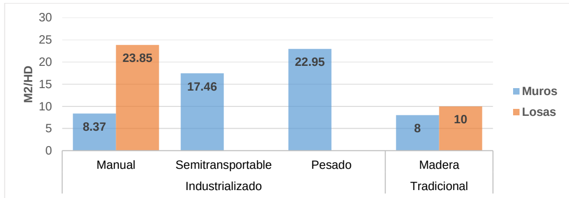
Figura 7.11. Gráfico del rendimiento de la partida de moldaje por tipología. (CDT, 2013)
