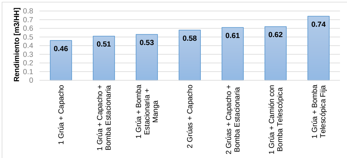
Figura 7.13. Gráfico del rendimiento real de vaciado del hormigón según metodología. (CDT, 2013)
