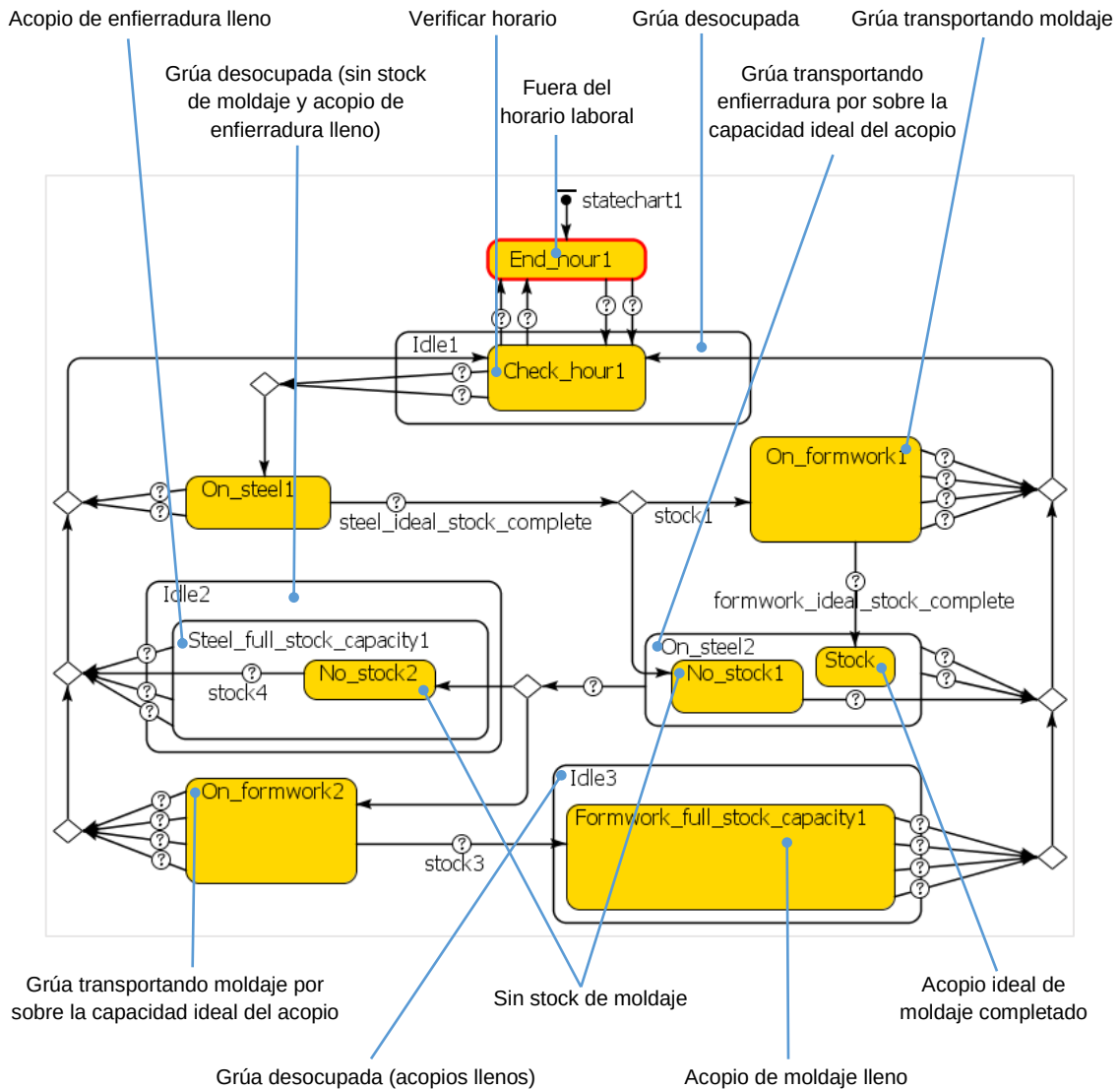
Figura 7.9. Diagrama de estado del segundo comportamiento de la grúa. Software Anylogic
