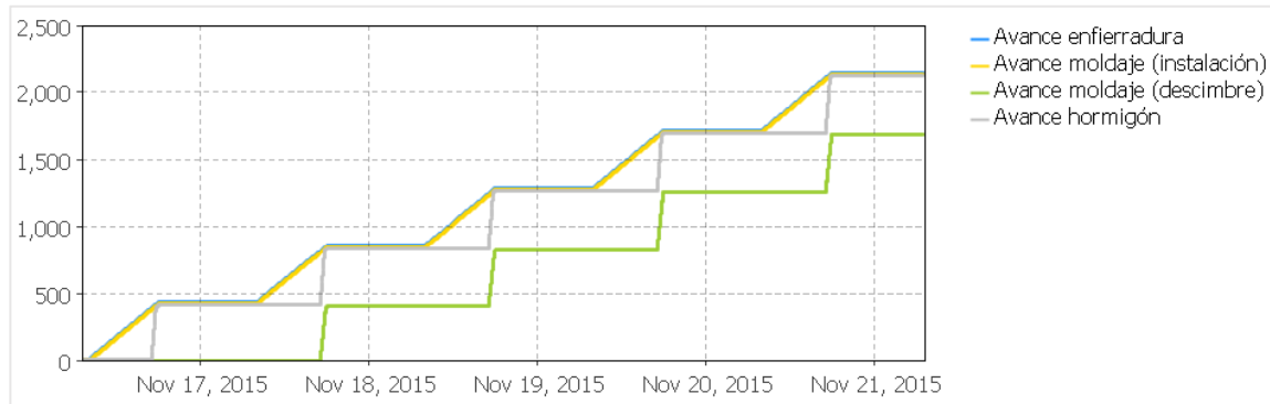
Figura 8.3. Gráfico del avance las distintas partidas de la etapa de obra gruesa simuladas en Anylogic.
