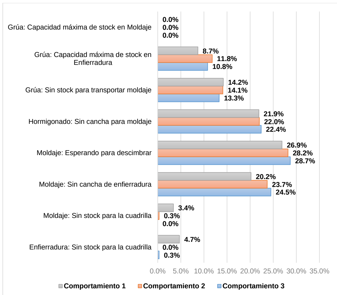
Figura 9.4. Comparación de los desperdicios del proceso según el comportamiento que desempeña la grúa
