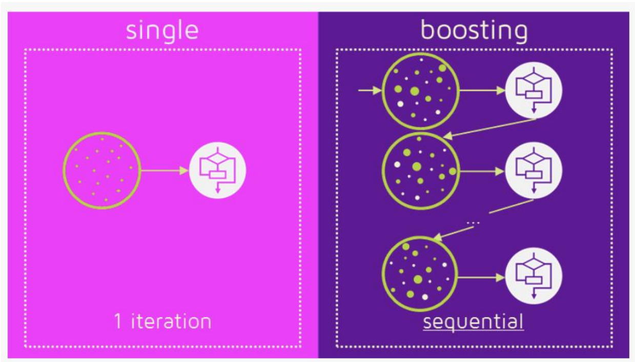
Ilustración 5: Ejemplo de Árbol de Decisión Potenciado
