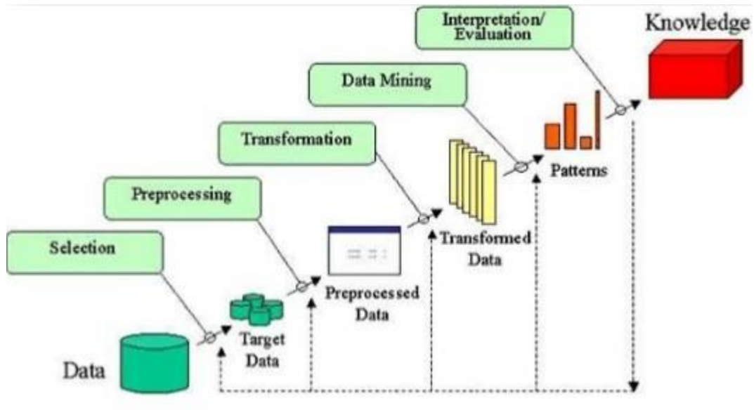
Ilustración 1:Proceso KDD
