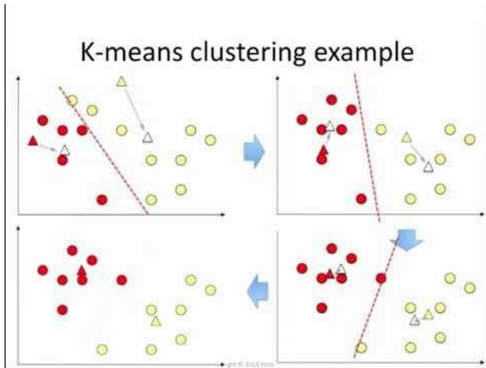
Ilustración 2: Modelo K-Medias
