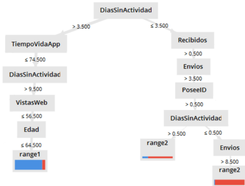
Ilustración 13: Muestra del Árbol de Decisión
