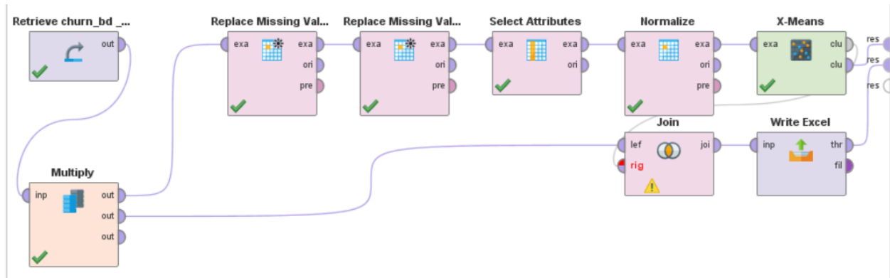
Ilustración 11: Modelo de Clasificación
