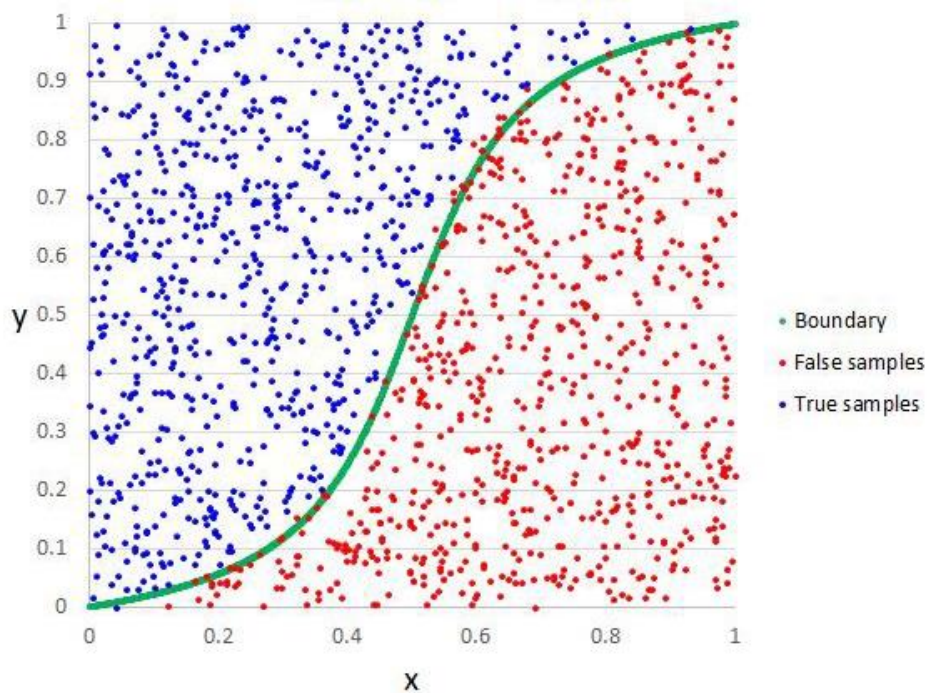
Ilustración 6: Ejemplo de Regresión Logística
