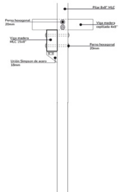
Unión sector impuro
