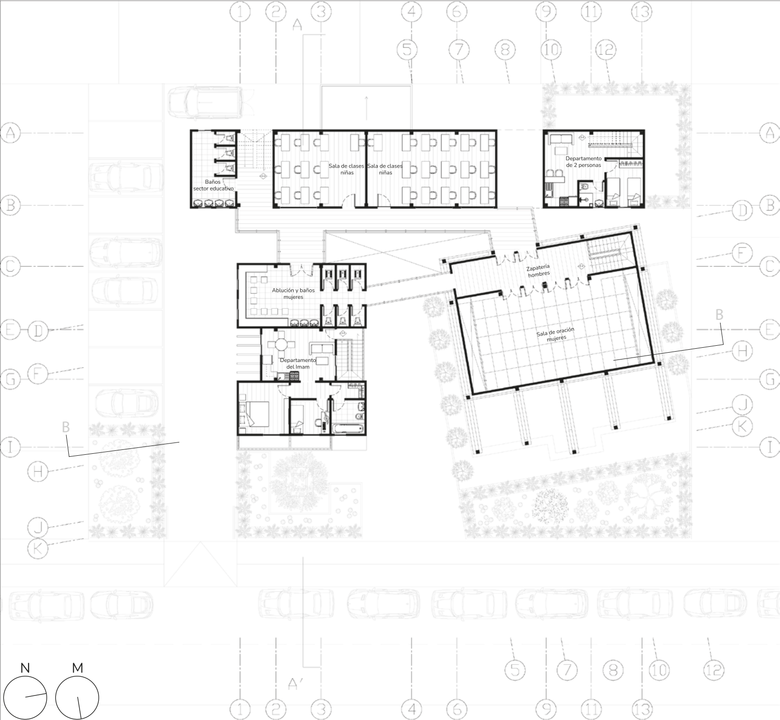
Planta nivel °2 escala 1:250. Elaboración propia
