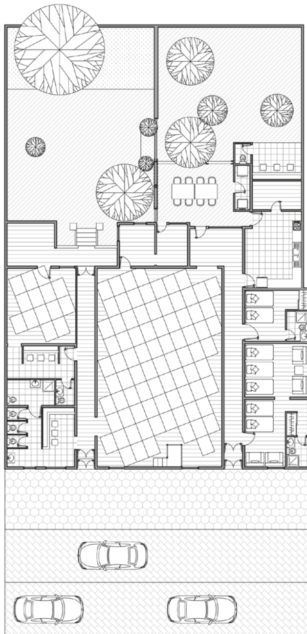
Planta en proceso de construcción (2024). Autoría propia
