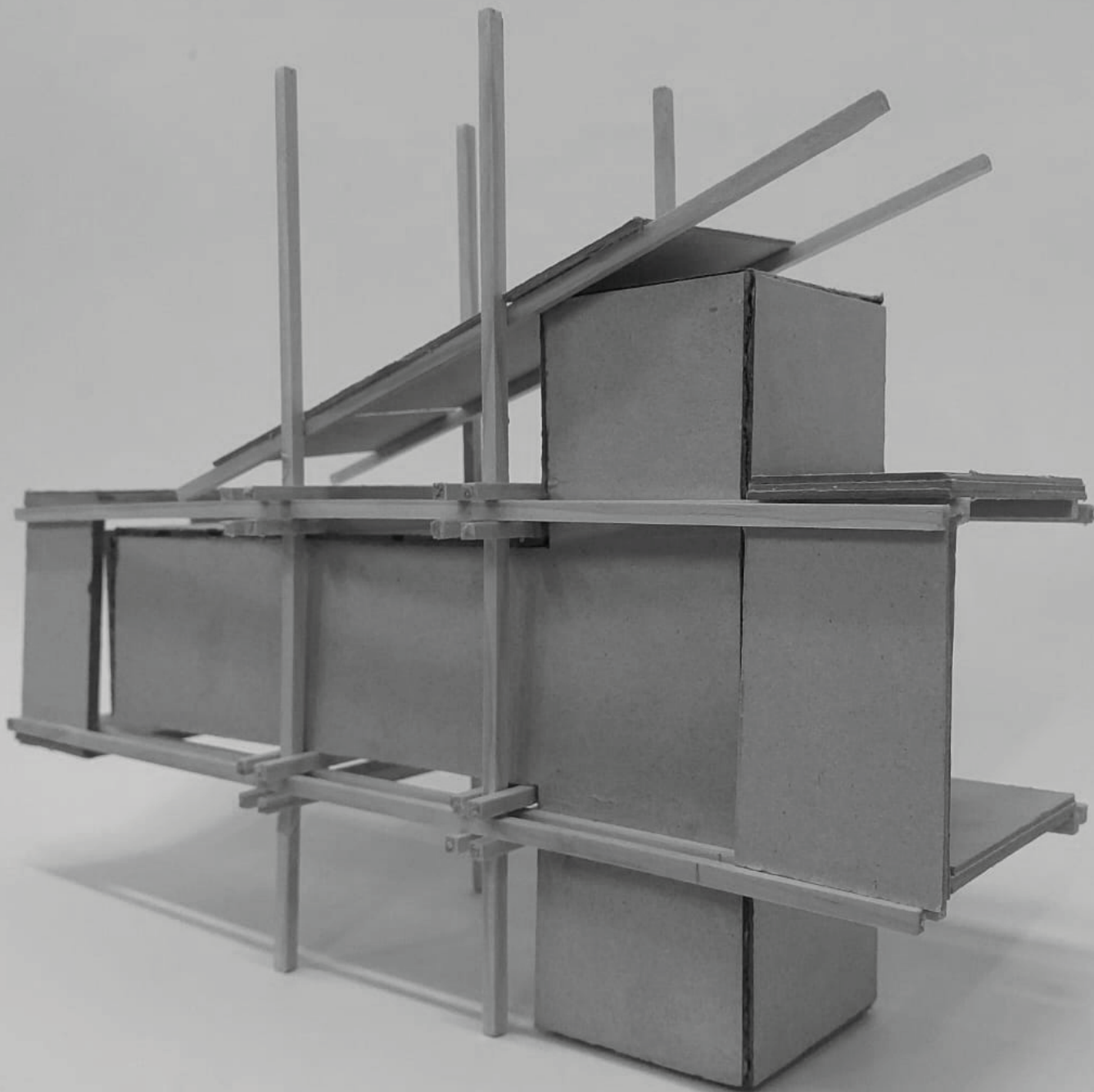
Imagen de modelo detalle con palos de madera y cartón piedra (Sector puro). Autoría propia
