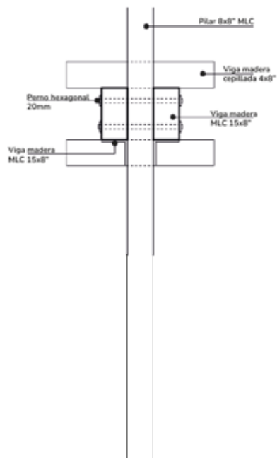
Unión sector puro
