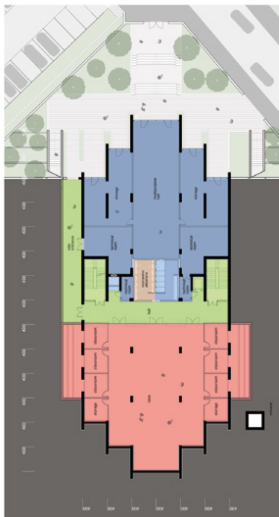
Planta nivel 1
