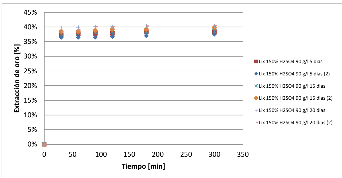
Figura 36. Curva de extracción de oro vs tiempo, para distintos tiempos de pretratamiento químico, 150% consumo de ácido en la etapa de pretratamiento y lixiviación a 90 [g/l] de concentración de cloruro.
