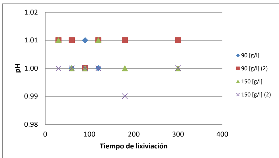
Figura 40. Variación de pH en el tiempo de lixiviación.
