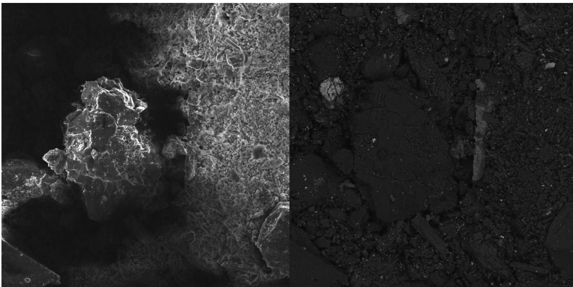
Figura 52. Imagen obtenida a 500X para un ripio obtenido por lixiviación, a la izquierda la morfología de las partículas mientras que a la derecha la imagen obtenida por cambios de densidades.
