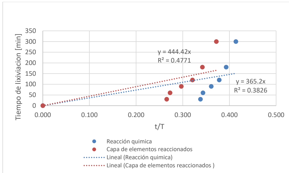
Figura 50. Tiempo de lixiviación vs t/T obtenido mediante el modelo cinético del núcleo sin reaccionar para la extracción del oro.
