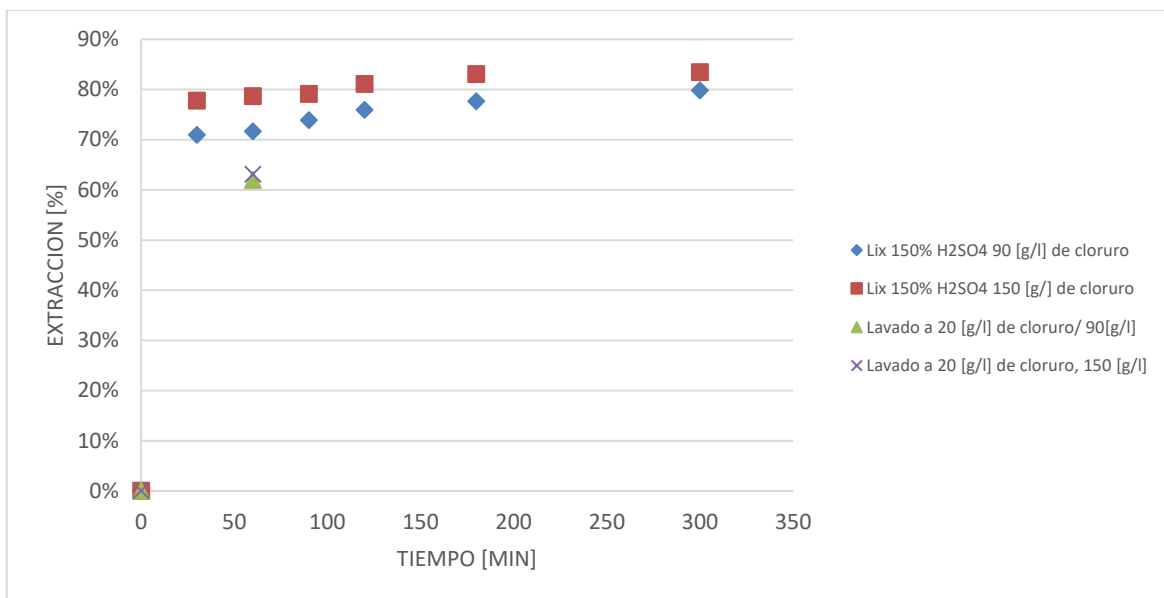
Figura 39. Curva de extracción de plata promedio de los duplicados realizados vs tiempo, para 10 días de pretratamiento, 150% consumo de ácido, lixiviación a 90 y 150 [g/l].
