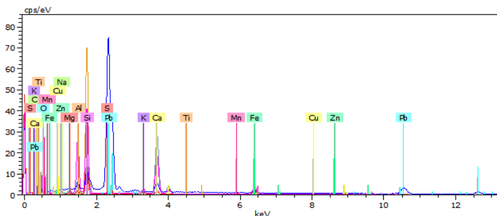
Figura 45 Espectrograma obtenido para la ventana de puntos analizados, donde se verifican los elementos presentes en los puntos seleccionados.
