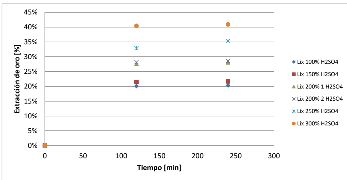
Figura 30. Curva de extracción de oro vs tiempo, 10 días de pretratamiento, lixiviación a 50 [g/l] de concentración de cloruro y distintos consumos de ácido en etapa de pretratamiento.
