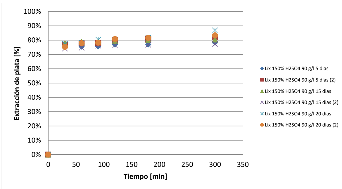
Figura 37. Curva de extracción de plata vs tiempo, para distintos tiempos de pretratamiento químico, 150% consumo de ácido en la etapa de pretratamiento y lixiviación a 90 [g/l] de concentración de cloruro.
