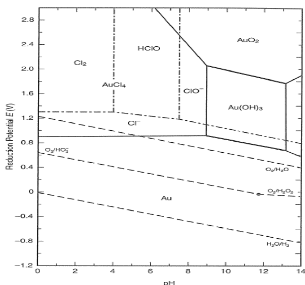
Figura 10. Diagrama Pourbaix para el sistema Au-Cl-H 2 O, a 25°C. [10]
