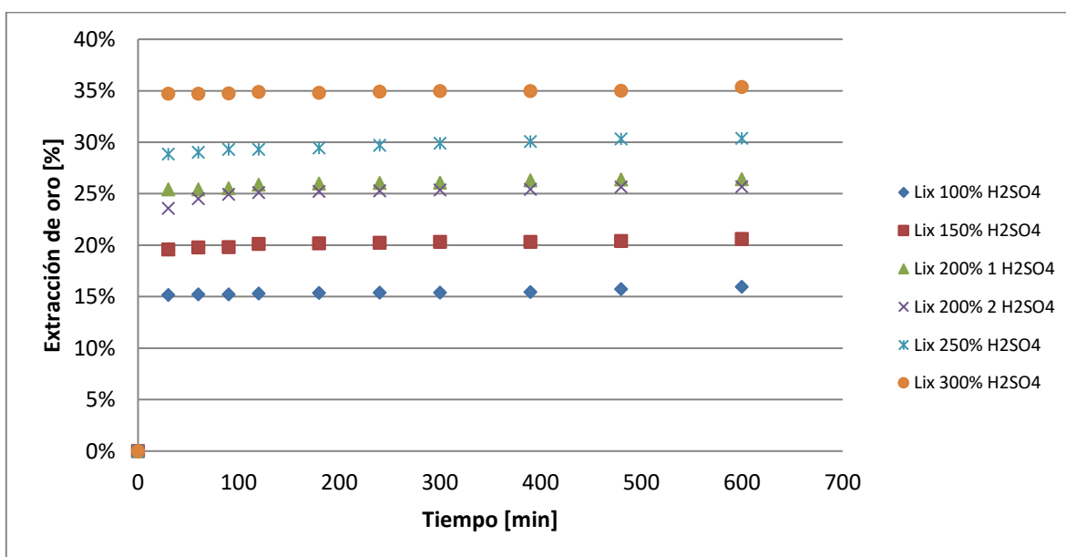
Figura 28. Curva de extracción de oro vs tiempo, 10 días de pretratamiento, lixiviación a 10 [g/l] de concentración de cloruro y distintos consumos de ácido en etapa de pretratamiento.
