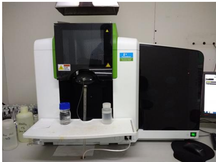
Figura 23. Espectrofotómetro de absorción atómica utilizado para lectura de iones en soluciones acuosas.
