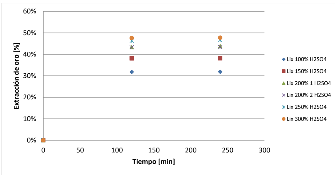
Figura 32. Curva de extracción de oro vs tiempo, 10 días de pretratamiento, lixiviación a 90 [g/l] de concentración de cloruro y distintos consumos de ácido en etapa de pretratamiento.
