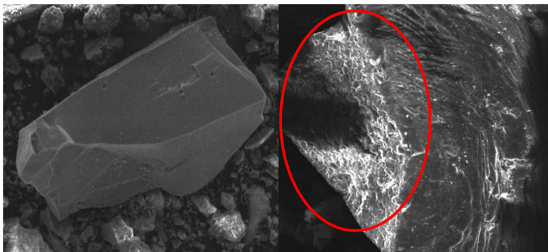
Figura 46. Morfología de una partícula a 698X presente en el mineral de cabeza a la izquierda, a la derecha a 700X se verifica en rojo el inicio de formación de porosidades alrededor de una partícula.
