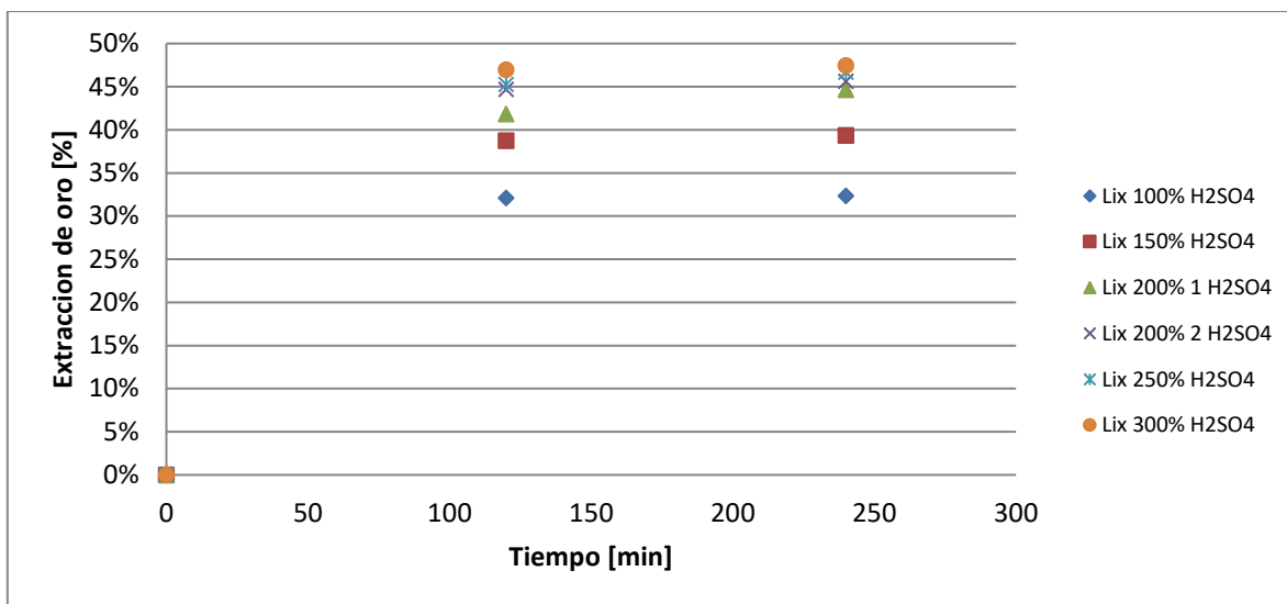
Figura 34. Curva de extracción de oro vs tiempo, 10 días de pretratamiento, lixiviación a 120 [g/l] de cloruro en solución y distintos consumos de ácido en etapa de pretratamiento.
