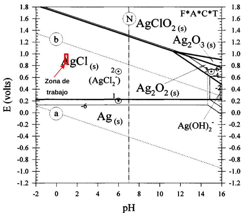
Figura 42. Diagrama de pourbaix a 25 °C y a concentración 1 [m] de \text{Cl}^- , se incluye la zona de trabajo obtenida mediante las variaciones de Eh y pH en el proceso de lixiviación.
