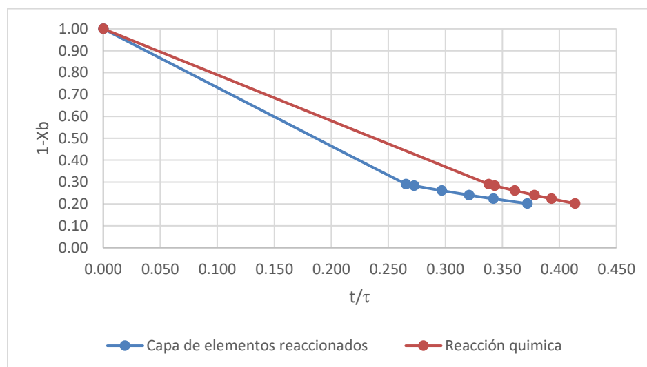
Figura 48. Progreso de la reacción de una sola panícula de plata esférica con el fluido circundante medido en función del tiempo necesario para la conversión completa.
