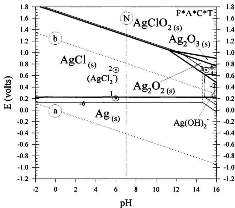
Figura 12. Diagrama de pourbaix a 25 °C y a concentración 1 [m] de Cl - , para el sistema Ag-Cl-H 2 O.[17]
