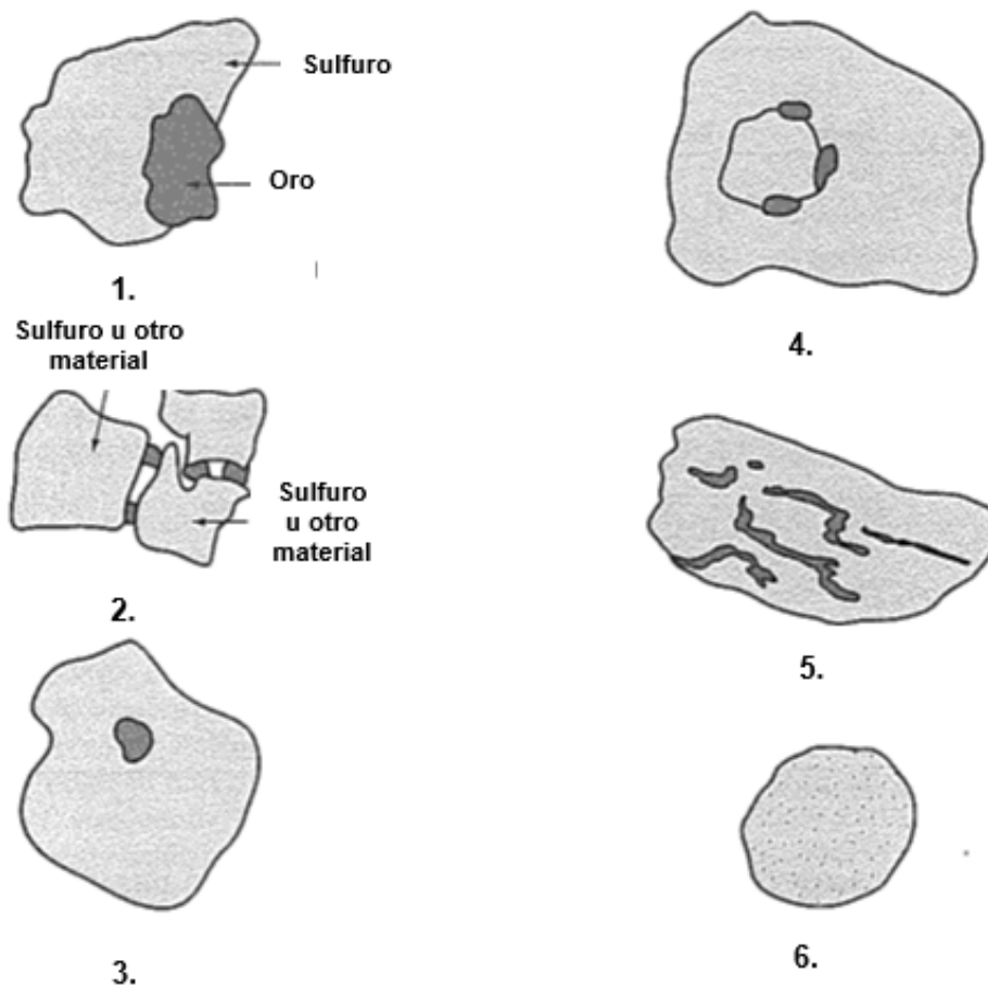
Figura 1. Representación esquemática de asociaciones de oro con minerales sulfurados.
