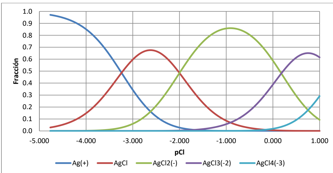
Figura 13. Diagrama de distribución para las especies de plata y cloruro formadas a 25°C y distintas concentraciones de cloruro.
