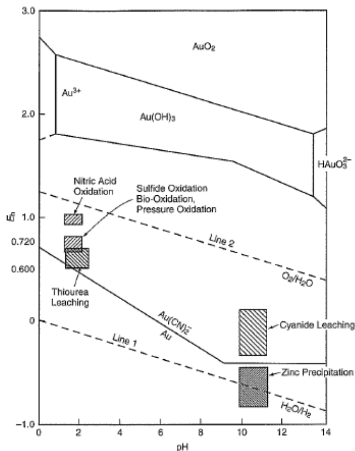
Figura 3. Rangos Eh-pH empleados en procesos industriales de extracción de oro.
