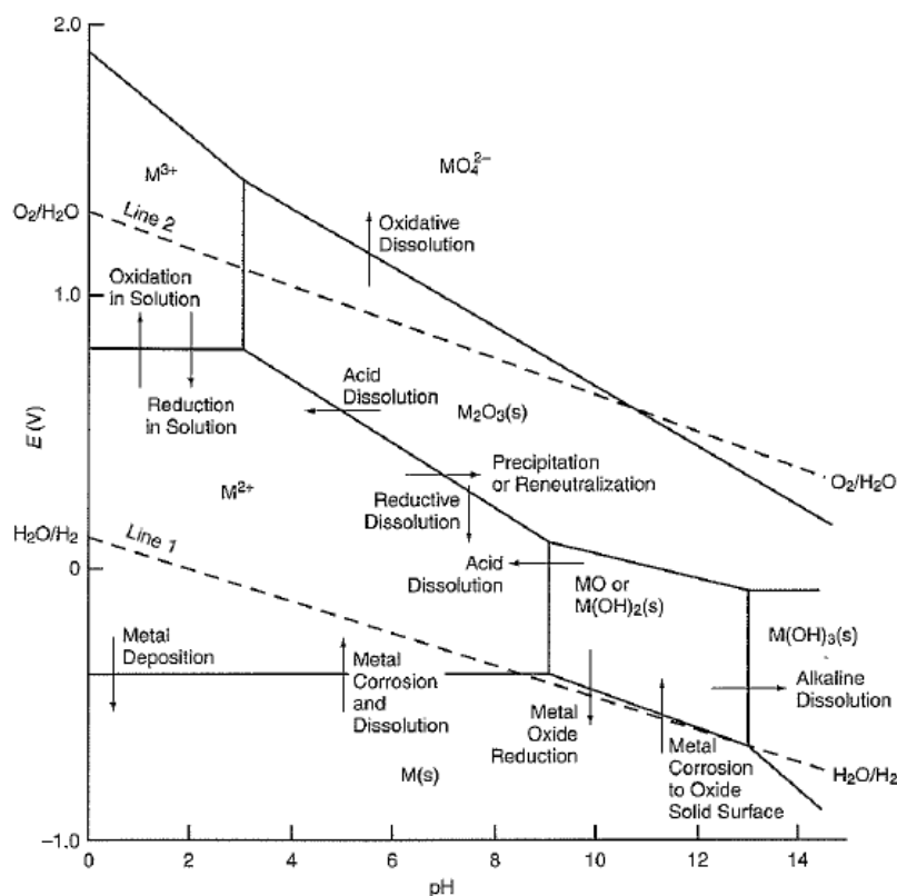
Figura 2. Ejemplo esquemático de un diagrama EH-pH para un sistema metal-agua, a 25°C.
