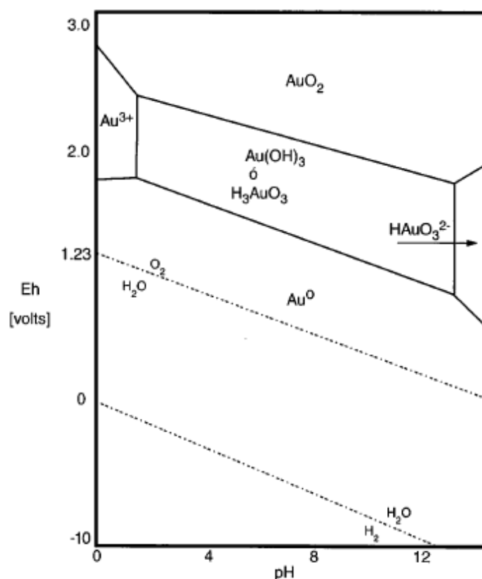
Figura 4. Diagrama Eh/pH oro y agua a 25°C, en concentraciones límite de especies a 10^{-4} molar. [5]
