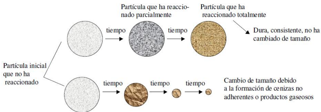
Figura 6. Diferentes tipos de comportamientos de partículas reactiva sólidas. [22]
