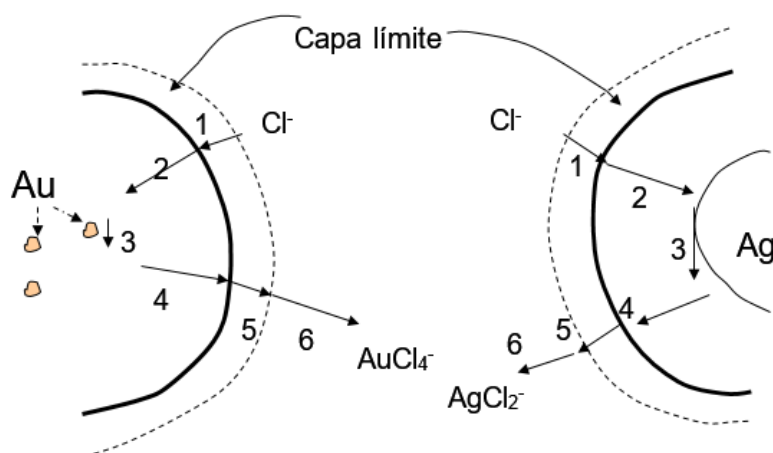
Figura 5. Representación esquemática de las etapas de una reacción química heterogénea.
