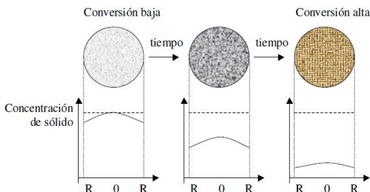
Figura 7. Esquematización del modelo de conversión progresiva. [22]
