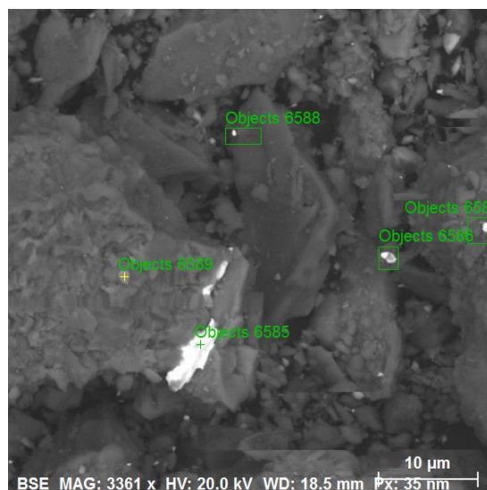
Figura 44. Puntos de análisis seleccionados a 3361X para un ripio obtenido por lixiviación a 90 [g/l] de cloruro, 150% consumo de ácido y 10 días de pretratamiento.
