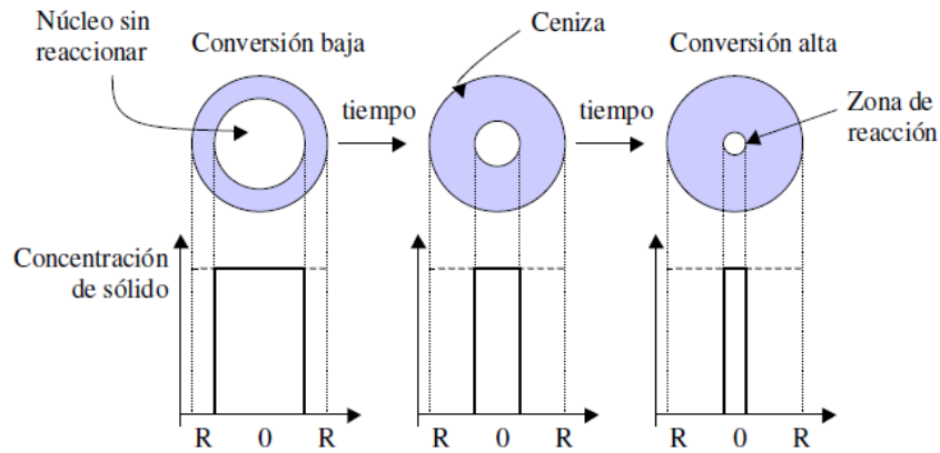
Figura 8. Esquematización del modelo del núcleo sin reaccionar. [8]
