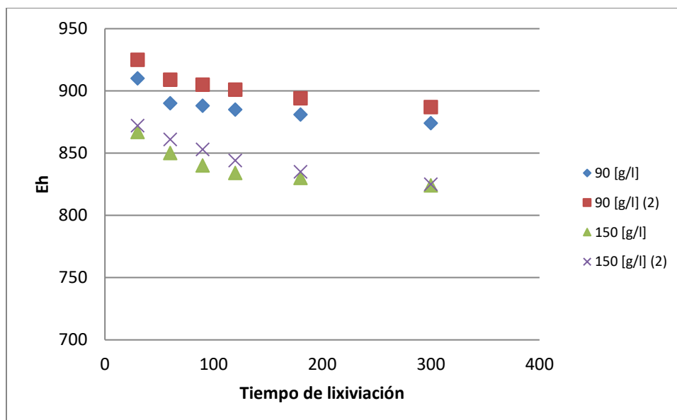
Figura 41. Variación de Eh en el tiempo de lixiviación.
