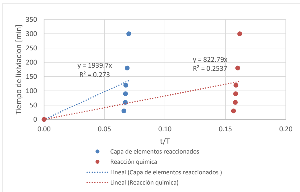
Figura 49. Tiempo de lixiviación vs t/T obtenido mediante el modelo cinético del núcleo sin reaccionar para la extracción del oro.
