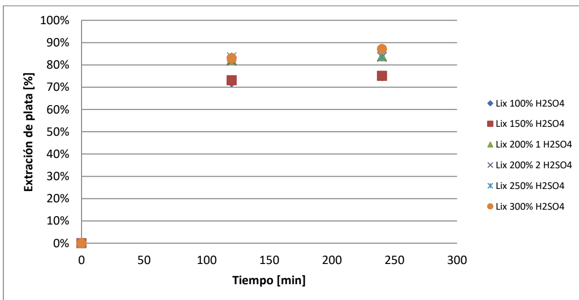
Figura 35. Curva de extracción de plata vs tiempo, 10 días de pretratamiento y lixiviación a 120 [g/l].
