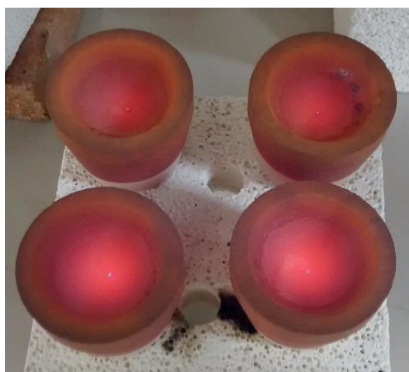
Figura 18. Copelas retiradas del horno, se puede apreciar botón de doré.
