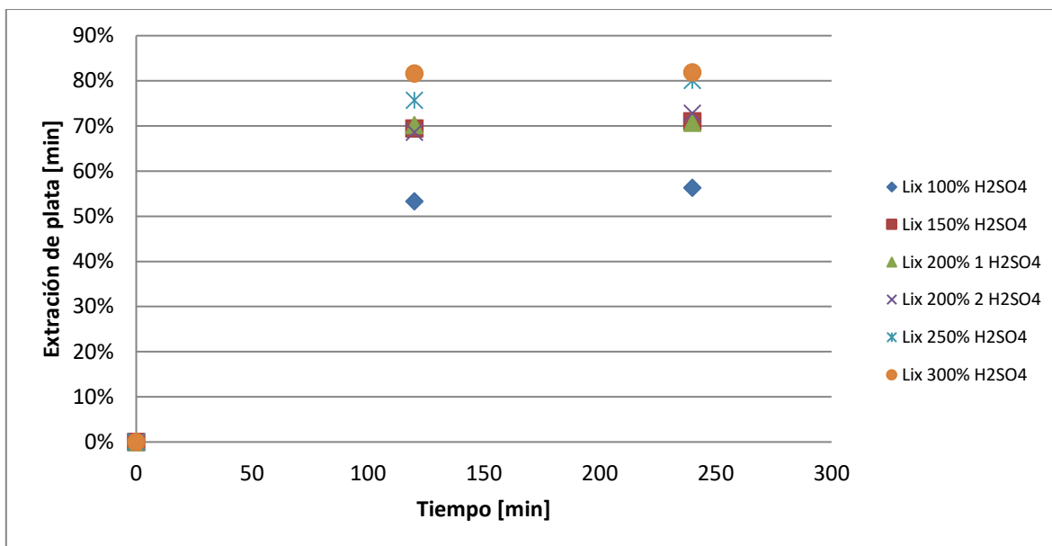
Figura 31. Curva de extracción de plata vs tiempo, 10 días de pretratamiento, lixiviación a 50 [g/l] de concentración de cloruro y distintos consumos de ácido en etapa de pretratamiento.
