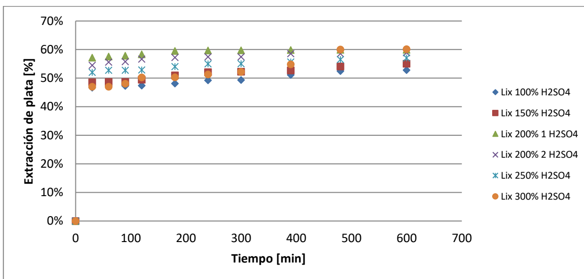
Figura 29. Curva de extracción de plata vs tiempo, 10 días de pretratamiento, lixiviación a 10 [g/l] de concentración de cloruro y distintos consumos de ácido en etapa de pretratamiento.
