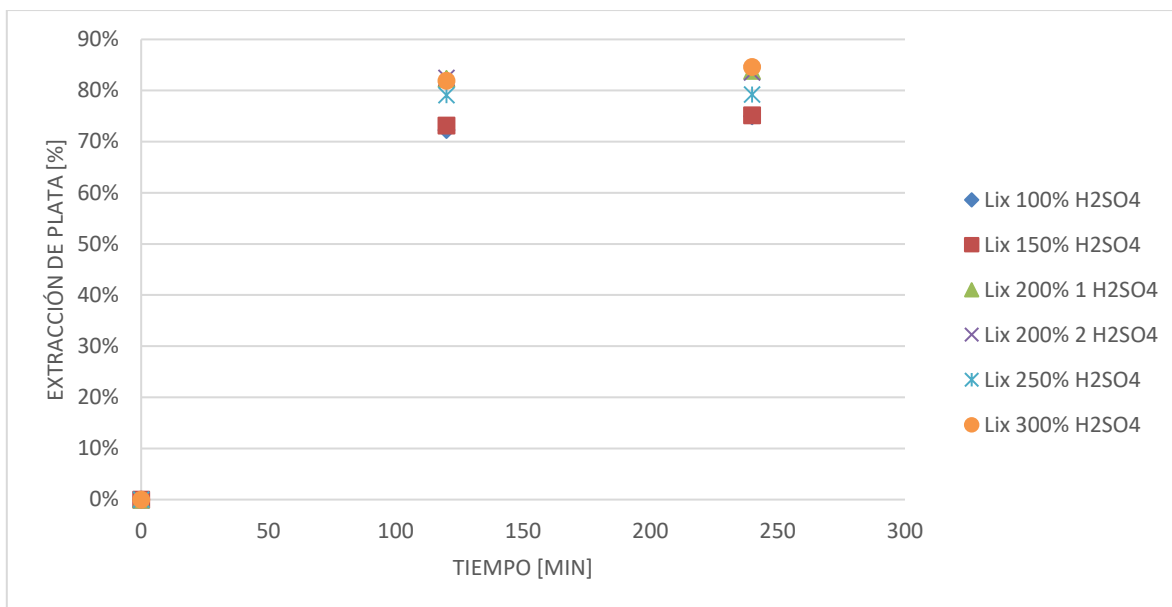
Figura 33. Curva de extracción de plata vs tiempo, 10 días de pretratamiento, lixiviación a 90 [g/l] de concentración de cloruro y distintos consumos de ácido en etapa de pretratamiento.
