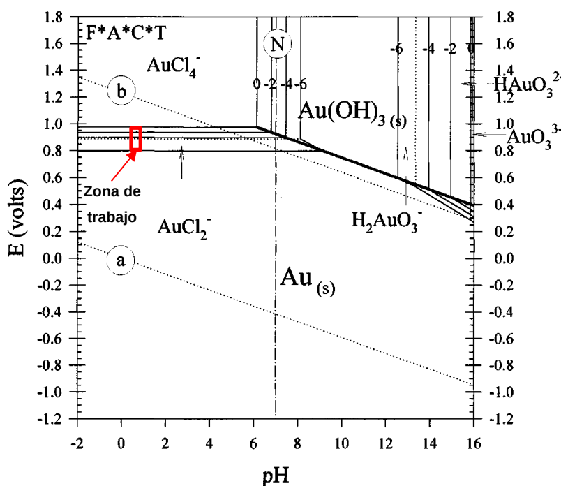
Figura 43. Diagrama de pourbaix para el sistema Au-Cl-H 2 O a 25 °C, a concentración 1 [m] de \text{Cl}^- y concentraciones de Au a 10^{-6} , 10^{-4} , 10^{-2} y 1 [m], se incluye la zona de trabajo obtenida mediante las variaciones de Eh y pH en el proceso de lixiviación.
