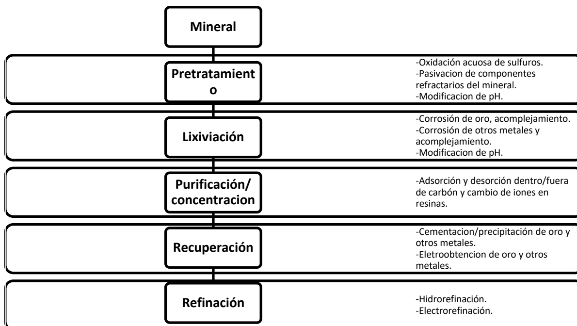
Figura 9. Diagrama de bloques del proceso de extracción del oro y su tipo de reacciones hidrometalúrgicas asociadas.
