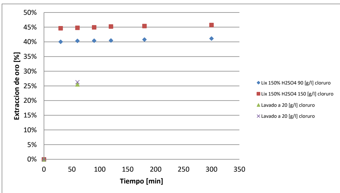
Figura 38. Curva de extracción de oro promedio de los duplicados realizados vs tiempo, para 10 días de pretratamiento, 150% consumo de ácido y lixiviación a 90 y 150 [g/l] de concentración de cloruro en solución lixivante.
