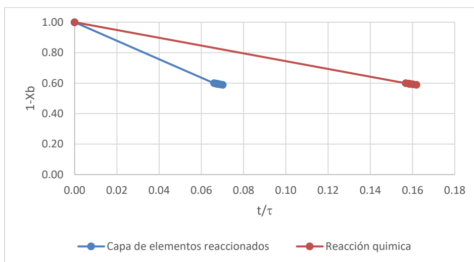
Figura 47. Progreso de la reacción de una sola panícula de oro esférica con el fluido circundante medido en función del tiempo necesario para la conversión completa.
