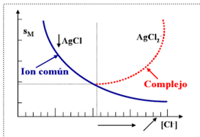
Figura 11. Solubilidad de los complejos de plata ante el aumento en la concentración de cloruro en solución. [21]
