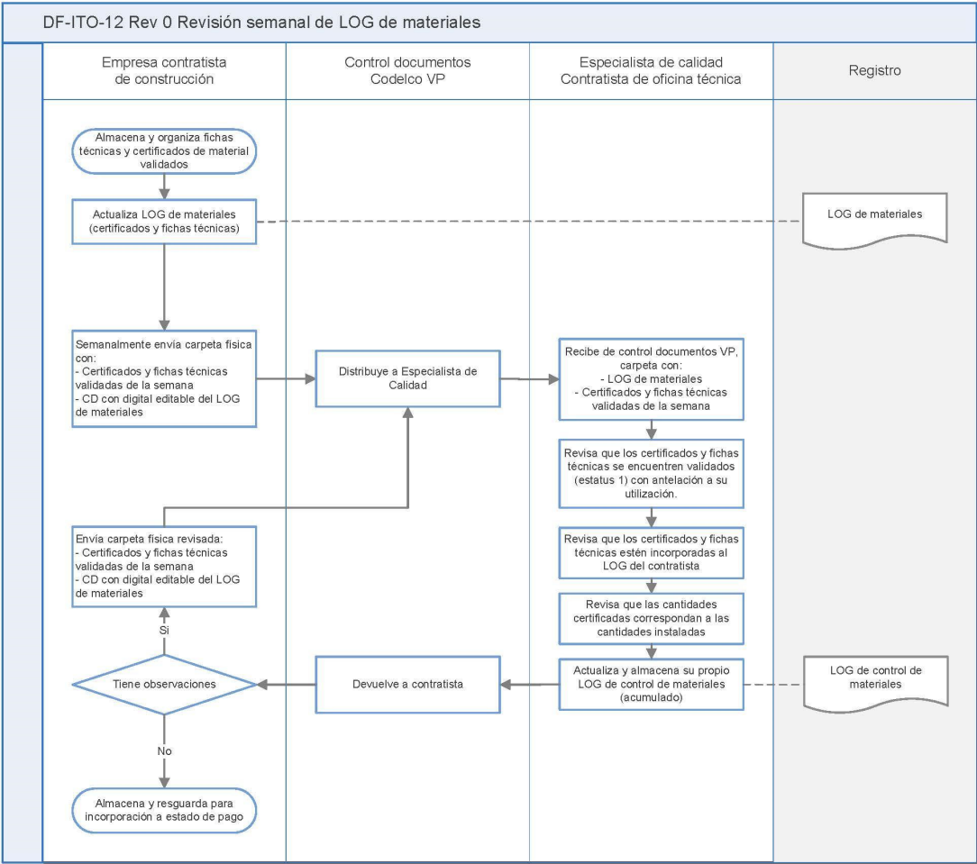
Ilustración 21: Diagrama de flujo – Revisión semanal de LOG de materiales Fuente: Elaboración propia.
