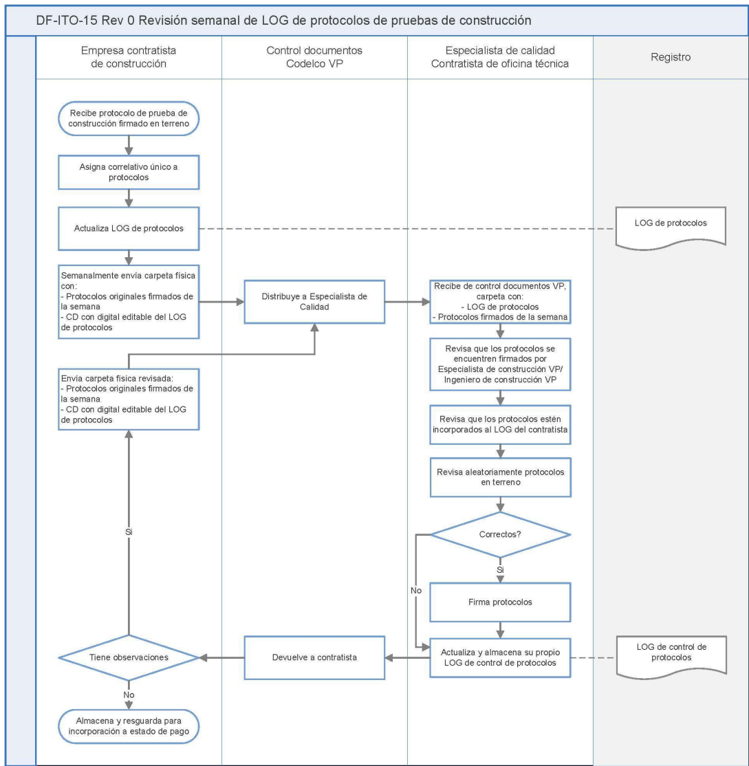
Ilustración 27: Diagrama de flujo – Revisión semanal de LOG de protocolos de pruebas de construcción Fuente: Elaboración propia.
