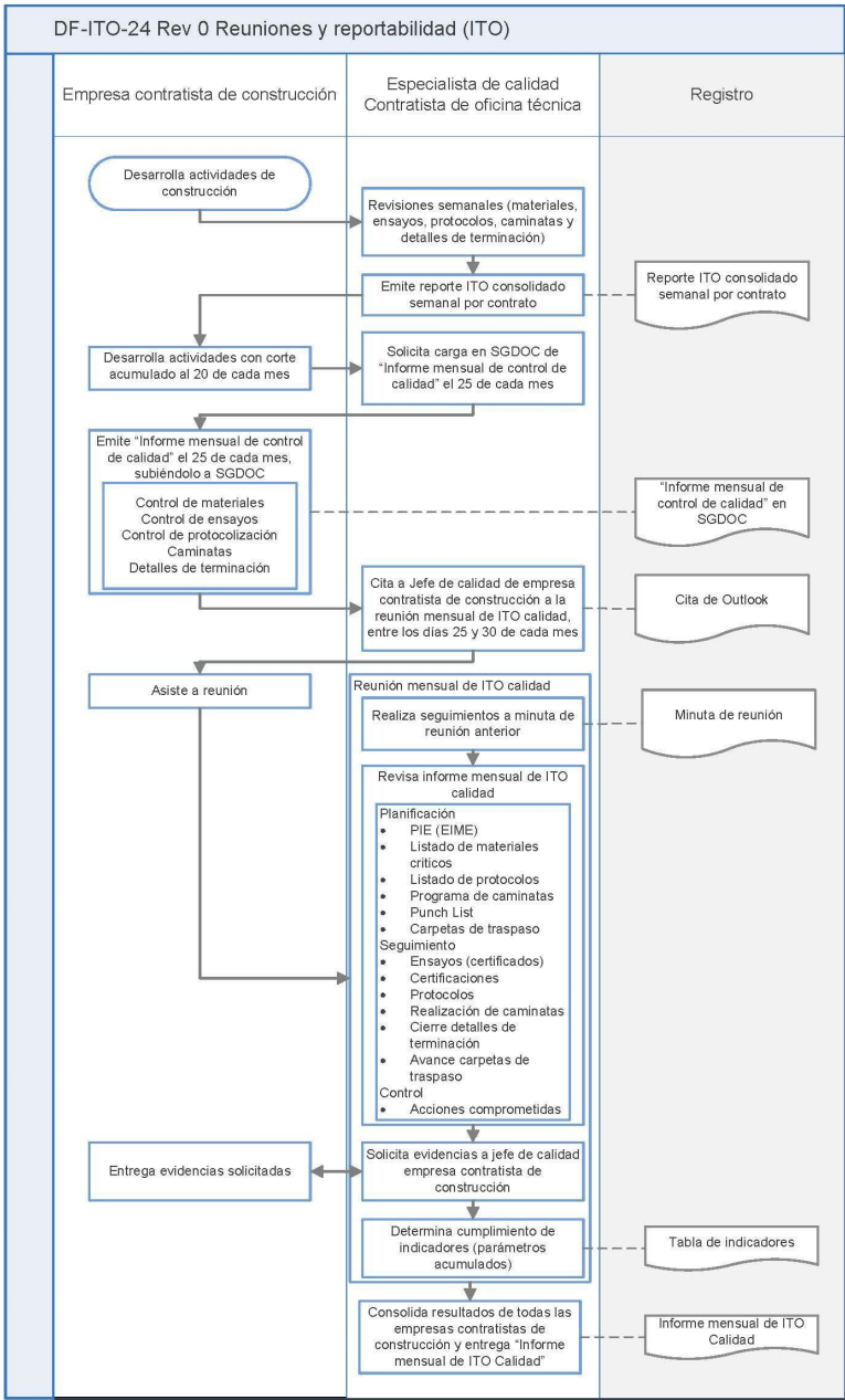
Ilustración 34: Diagrama de flujo – Reuniones y reportabilidad. Fuente: Elaboración propia.
