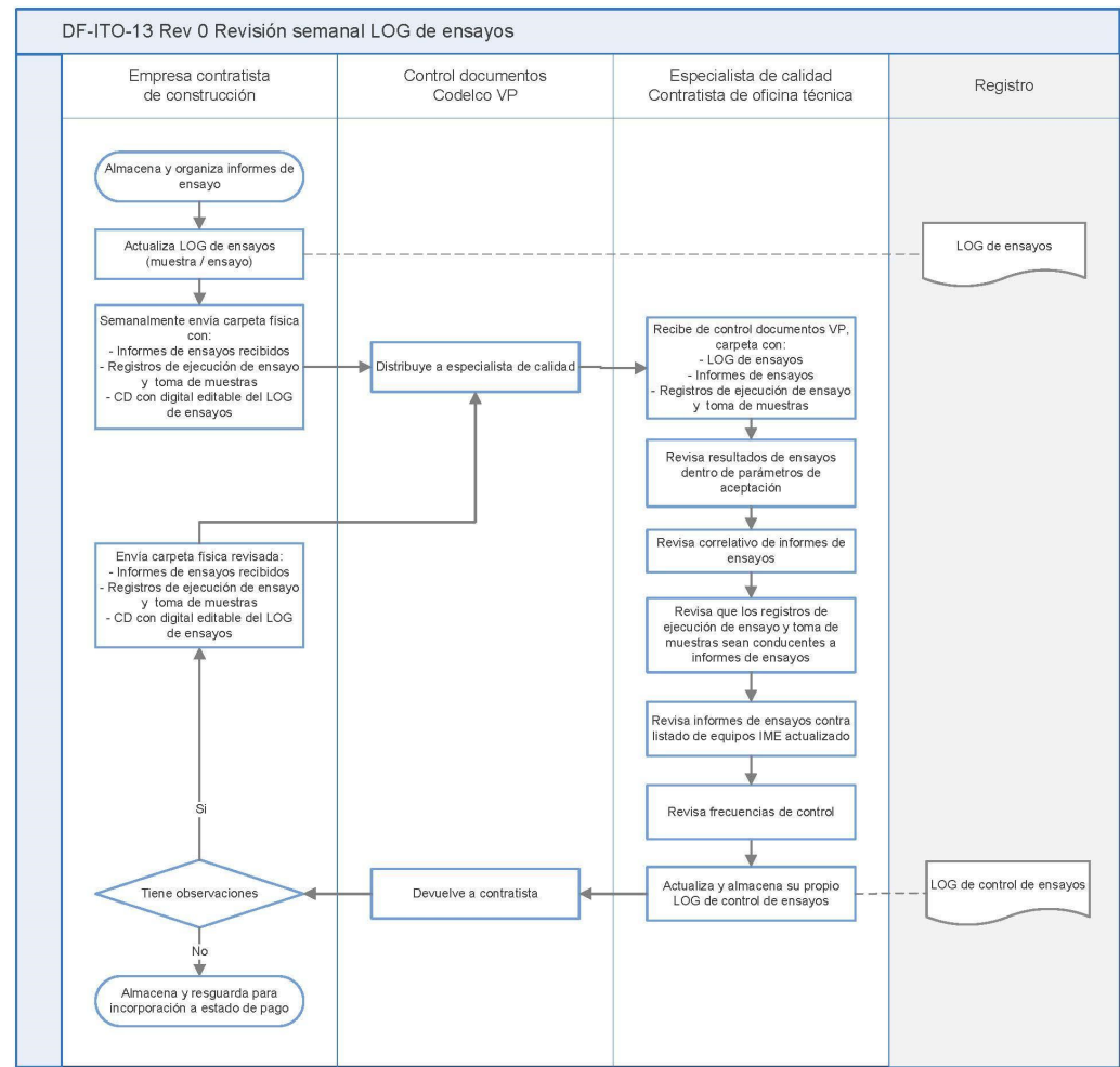
Ilustración 23: Diagrama de flujo – Revisión semanal de LOG de ensayos Fuente: Elaboración propia.
