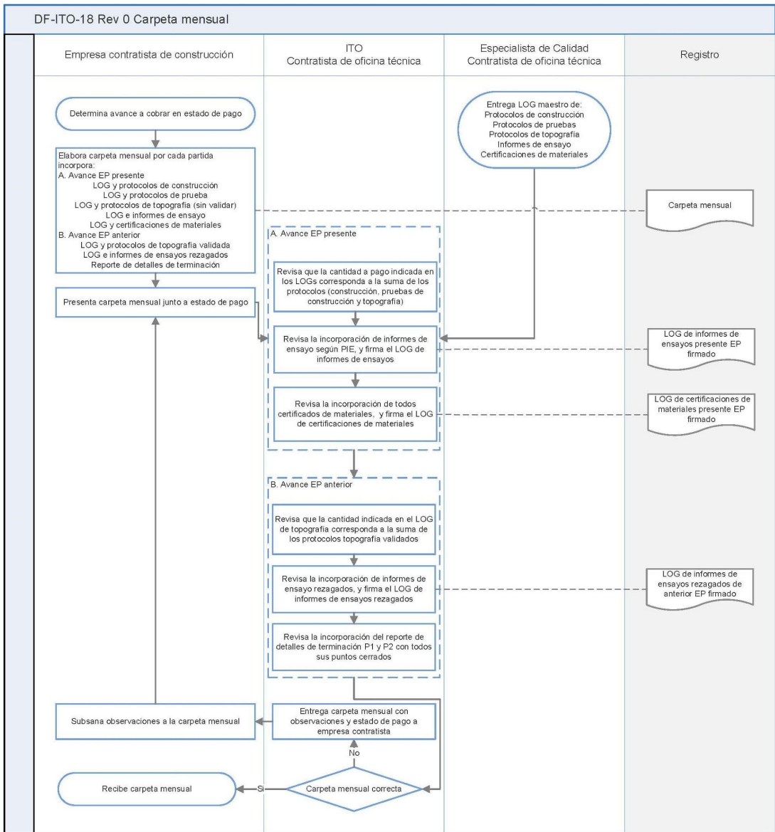
Ilustración 30: Diagrama de flujo – Carpeta mensual Fuente: Elaboración propia.
