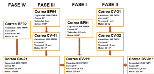
Figura 10: Esquema manejo de materiales Diablo Regimiento.
