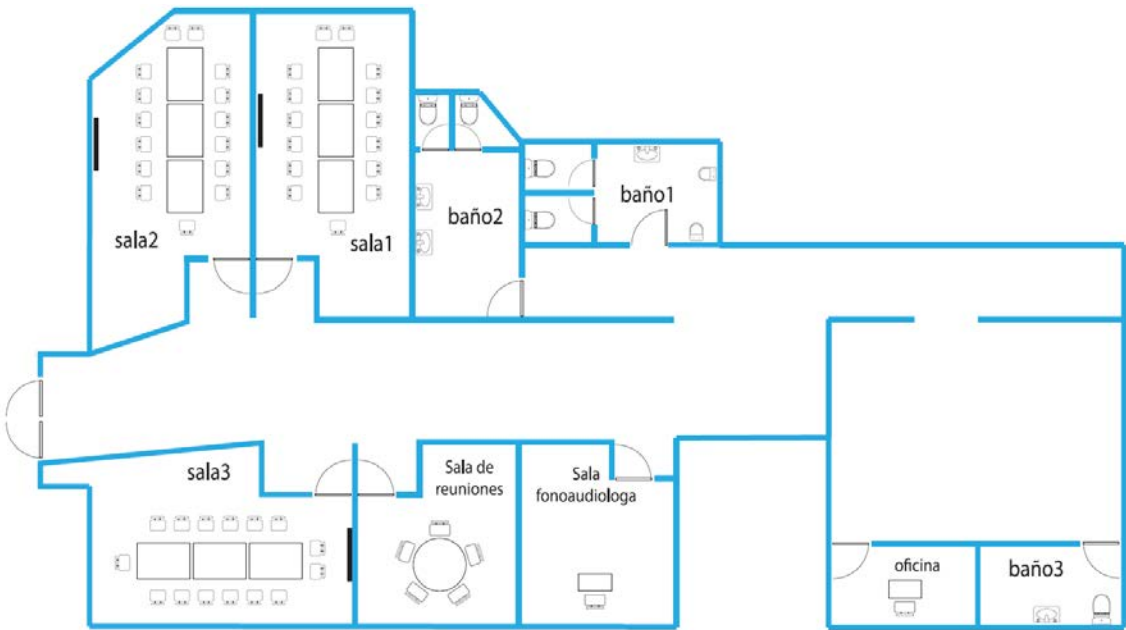
Figura 3-3. Lay Out de la Escuela de Lenguaje
