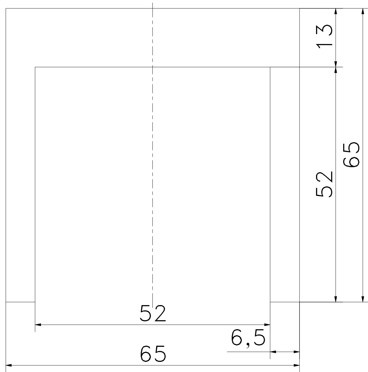
VISTA ALZADO
