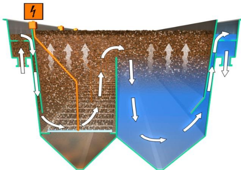
Figura 21: Descripción gráfica del funcionamiento de un equipo de electroflotación para el tratamiento de aguas. Fuente: EnviroChemie GmbH.
