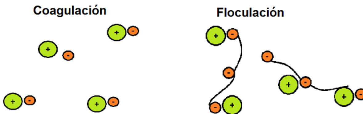
Figura 14: Efectos del proceso de coagulación y floculación. Suponiendo una partícula coloide de carga negativa, se añaden agentes coagulantes para desestabilizar las cargas y minimizar la repulsión entre las partículas. Luego el agente floculante permite crear puentes para aumentar el peso y tamaño de estas.
