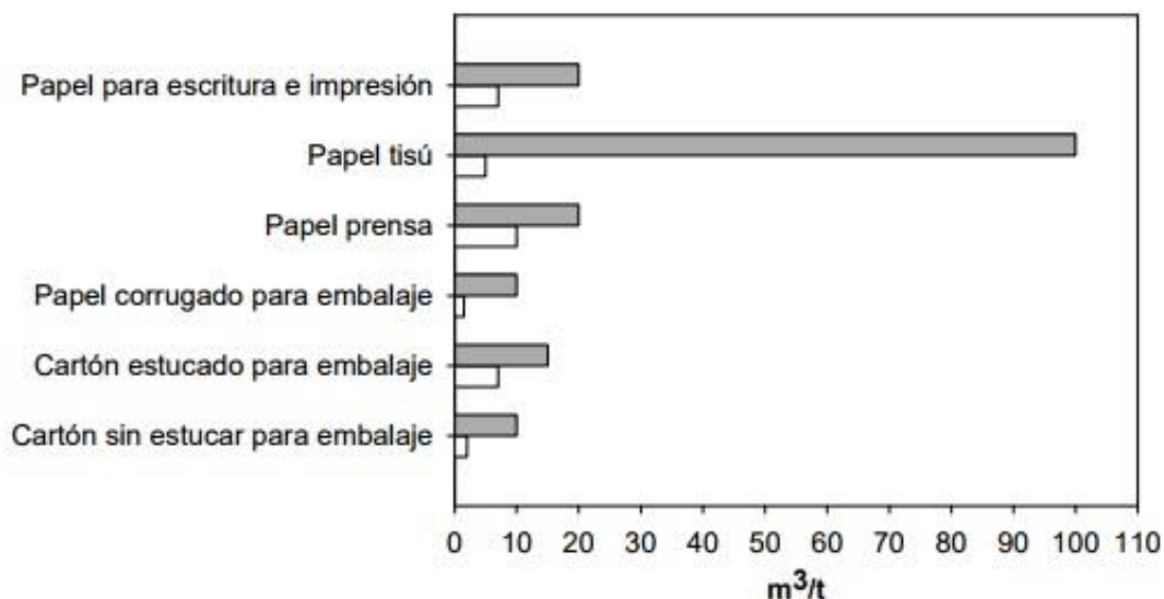
Figura 11: Valores máximos y mínimos de consumo de agua de alimentación por tonelada producida, para algunos productos fabricados a partir de fibra recuperada. Fuente: IPPC, 2006.
