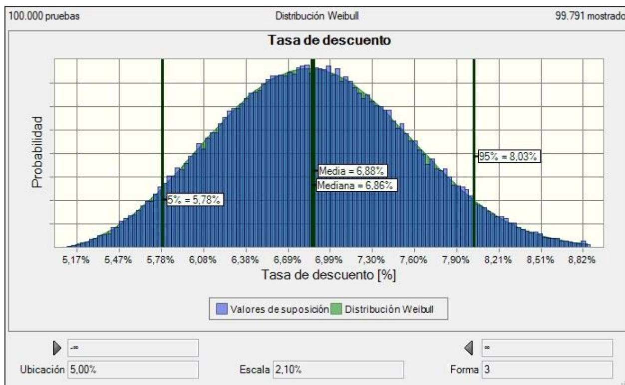
Figura 36: Distribución de probabilidad de la tasa de descuento en base a un financiamiento externo del 60%. Fuente: elaboración propia en base al software Crystal Ball.
