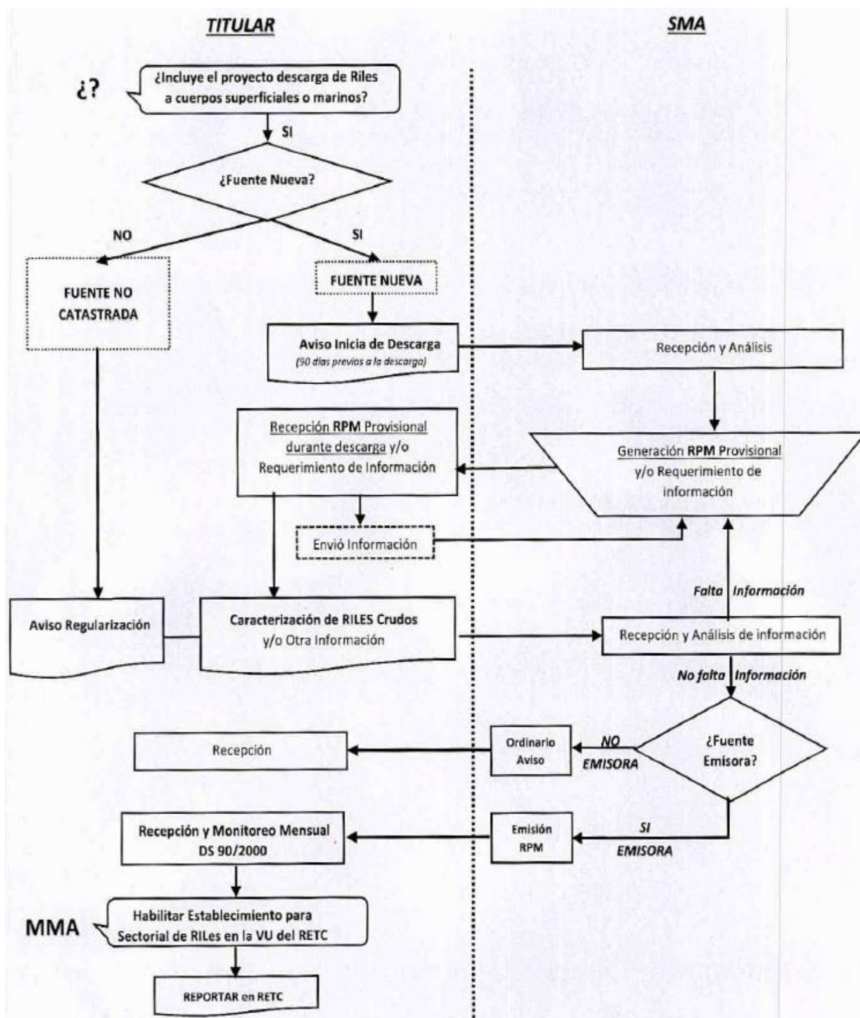
Figura 48: Diagrama de flujo de una RPM. Fuente: SMA, 2015.
