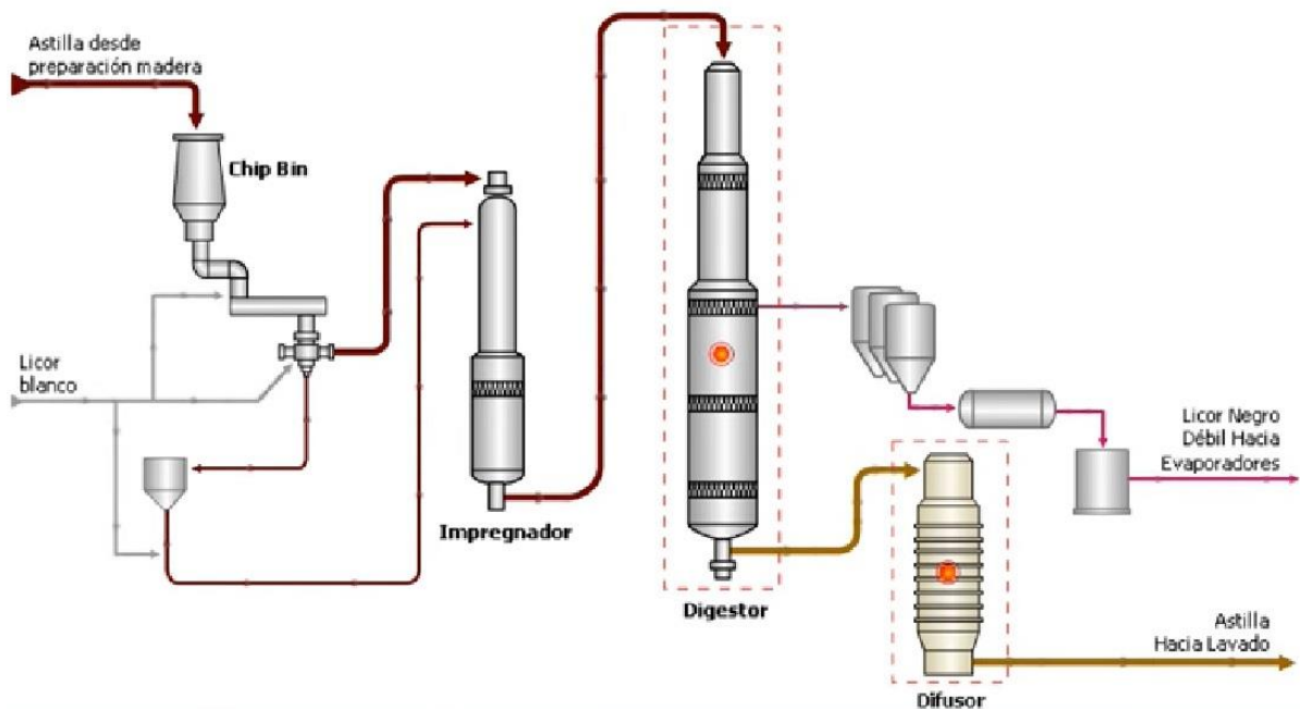
Figura 44: Diagrama de flujo de la fase de digestión. Fuente: Documento bibliográfico Celulosa Arauco 2014.
