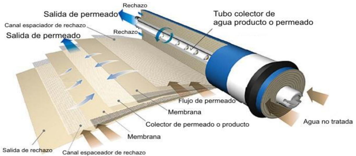
Figura 16: Filtración por membrana de flujo cruzado de tipo dentro-fuera. Fuente: Aquapurif.
