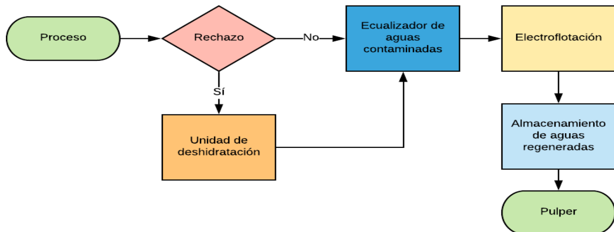
Figura 23: Diagrama de proceso de circuito de regeneración de aguas correspondiente a la sección de preparación pasta. Fuente: elaboración propia.
