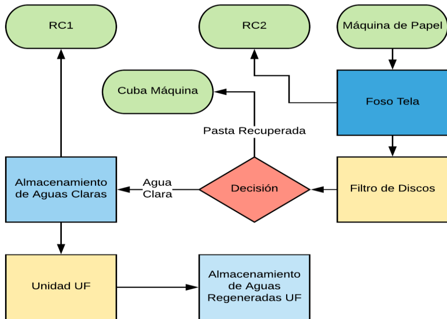
Figura 26: Diagrama de proceso del sistema de regeneración de aguas correspondiente al circuito de la máquina de papel. Fuente elaboración propia.
