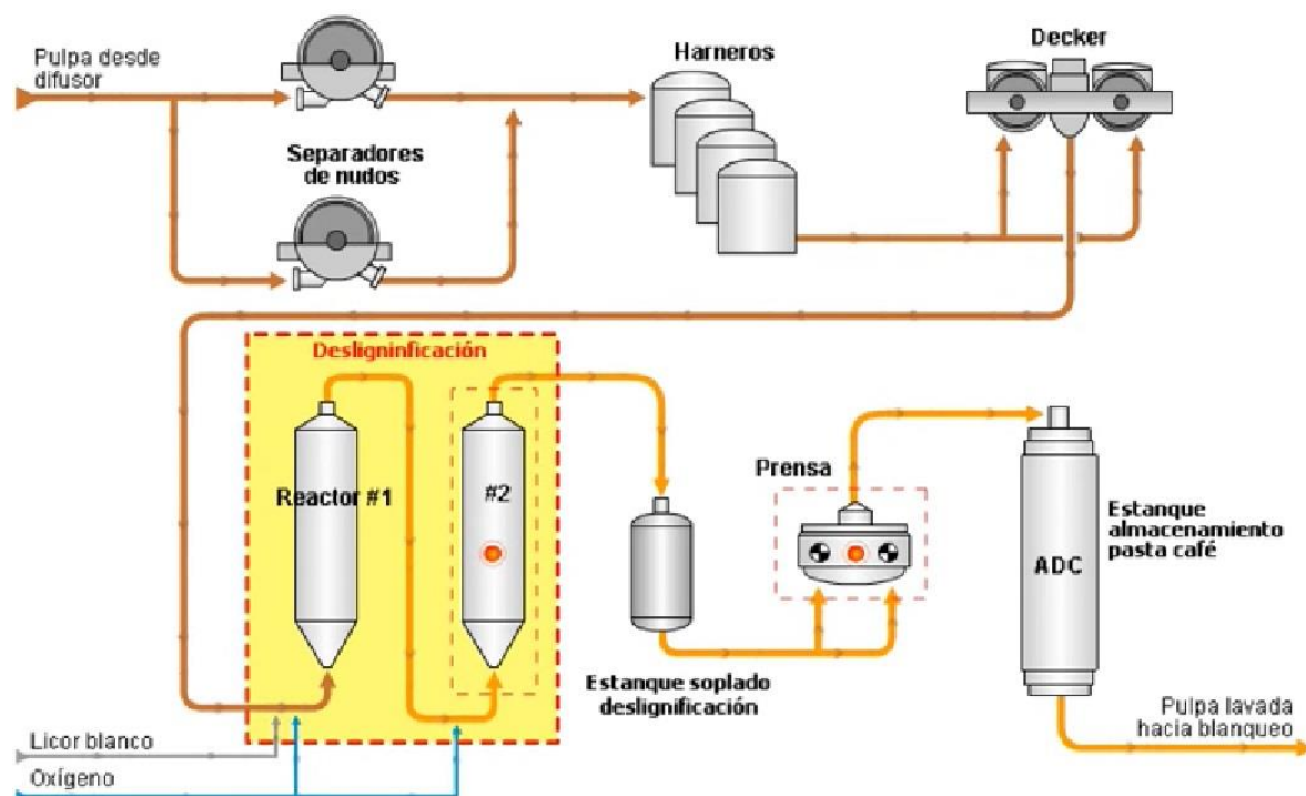
Figura 45: Diagrama de flujo de la fase de clasificación y lavado. Fuente: Documento bibliográfico Celulosa Arauco 2014.
