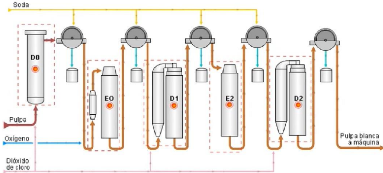
Figura 46: Diagrama de flujo de la fase de blanqueo. Fuente: Documento bibliográfico Celulosa Arauco 2014.
