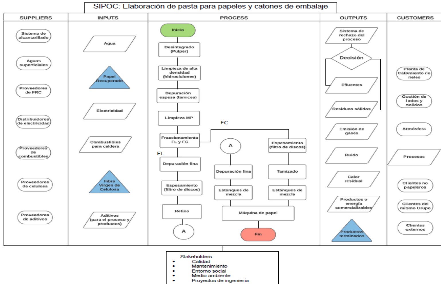
Figura 17: SIPOC del proceso de producción de papeles y cartones a partir de fibra recuperada, con (FC) fibra corta y (FL) fibra larga. Fuente: elaboración propia.
