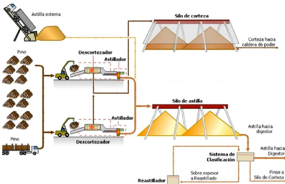
Figura 7:Diagrama de flujo de la fase preparación madera (descortezado y astillado). Fuente: Documento bibliográfico Celulosa Arauco 2014.
