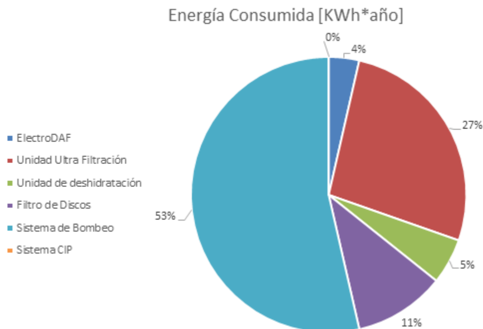
Figura 31: Gráfico circular con el aporte porcentual del consumo de energía de los equipos considerados en el sistema de regeneración. Fuente: elaboración propia.
