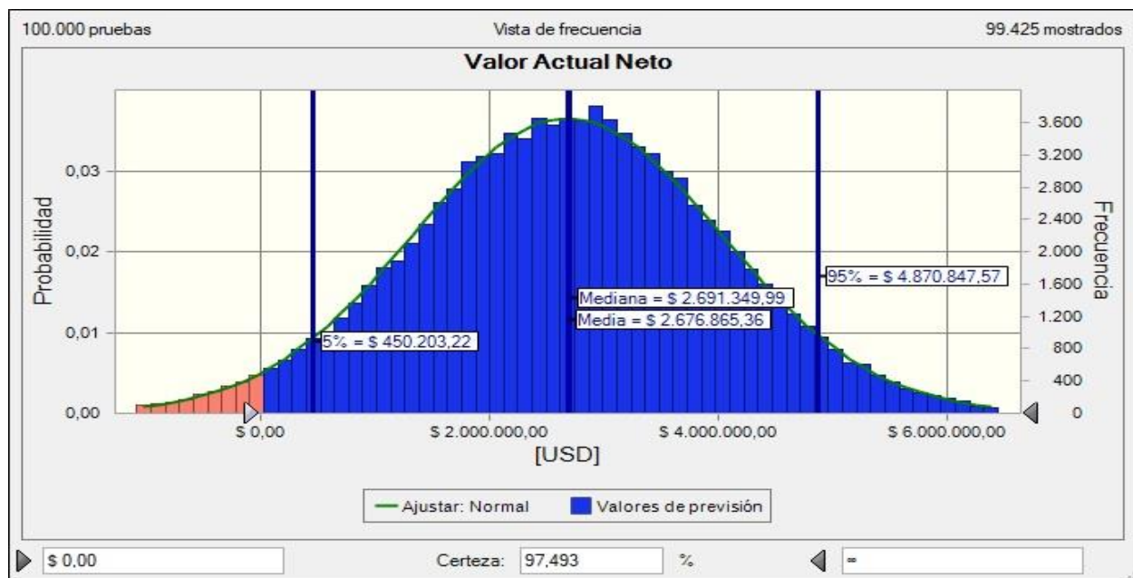
Figura 42: Distribución de probabilidad del Valor Actual Neto con un financiamiento externo del 60%, determinando la certeza para que este sea positivo. Fuente: elaboración propia en base al software Crystal Ball.
