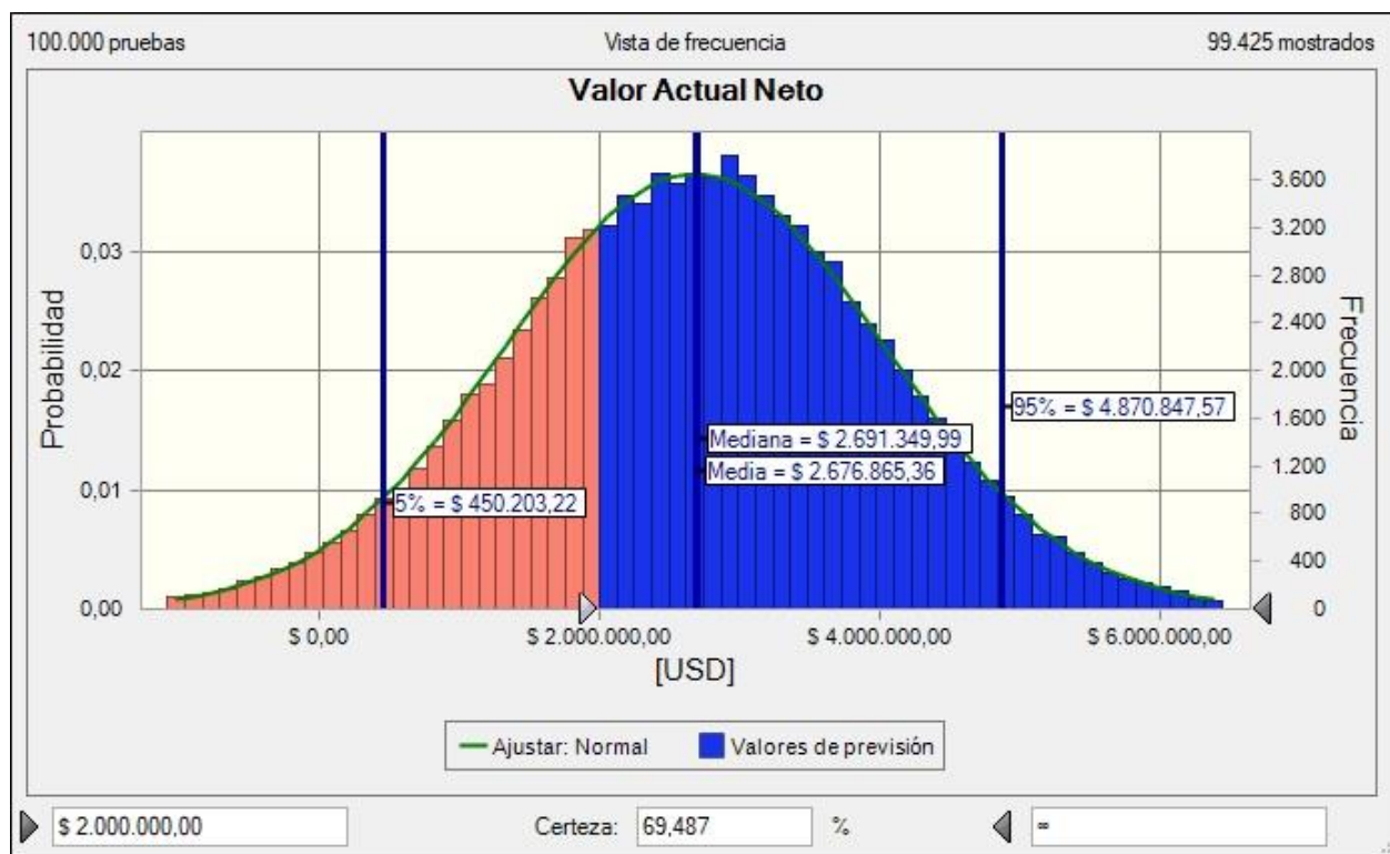
Figura 38: Distribución de probabilidad del Valor Actual Neto con un financiamiento externo del 60%, determinando la certeza para que este sea mayor a 2.000.000 [USD]. Fuente: elaboración propia en base al software Crystal Ball.
