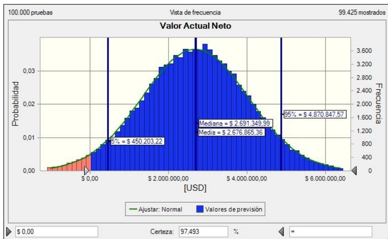
Figura 37: Distribución de probabilidad del Valor Actual Neto con un financiamiento externo del 60%, determinando la certeza para que este sea positivo. Fuente: elaboración propia en base al software Crystal Ball.
