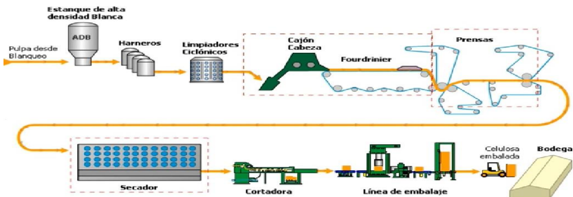
Figura 10: Diagrama de flujo de la máquina de pasta papelera. Fuente: Celulosa Arauco 2014.
