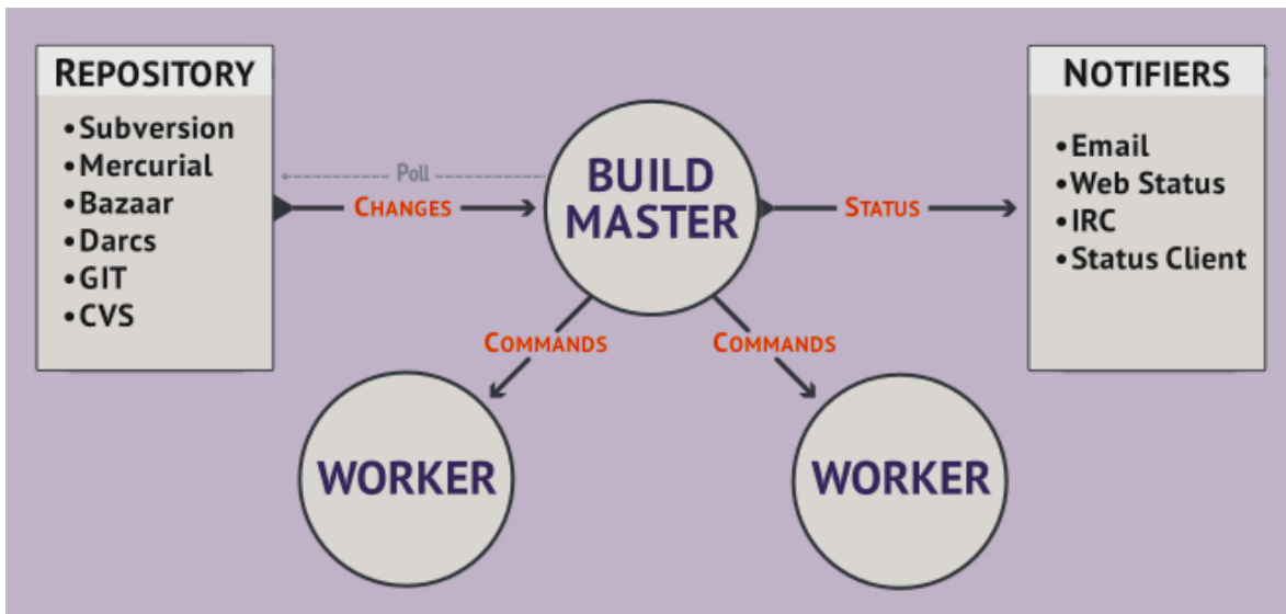
Figura 5: Flujo de trabajo en BuildBot.
