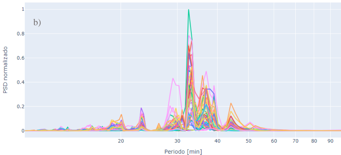
Figura 5-3: Espectro normalizado de los 50 escenarios simulados para a) magnitud Mw 8.6 y b) magnitud Mw 9.2 Bahía Coquimbo.
