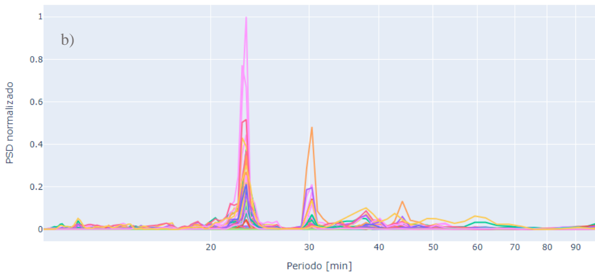
Figura 5-5: Espectro normalizado de los 50 escenarios simulados para a) magnitud Mw 8.6 y b) magnitud Mw 9.2 Bahía Quintero
