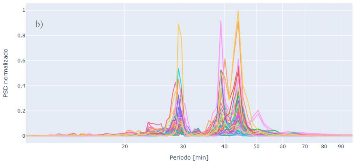
Figura 5-2: Espectro normalizado de los 50 escenarios simulados para a) magnitud Mw 8.6 y b) magnitud Mw 9.2 Bahía Choros.
