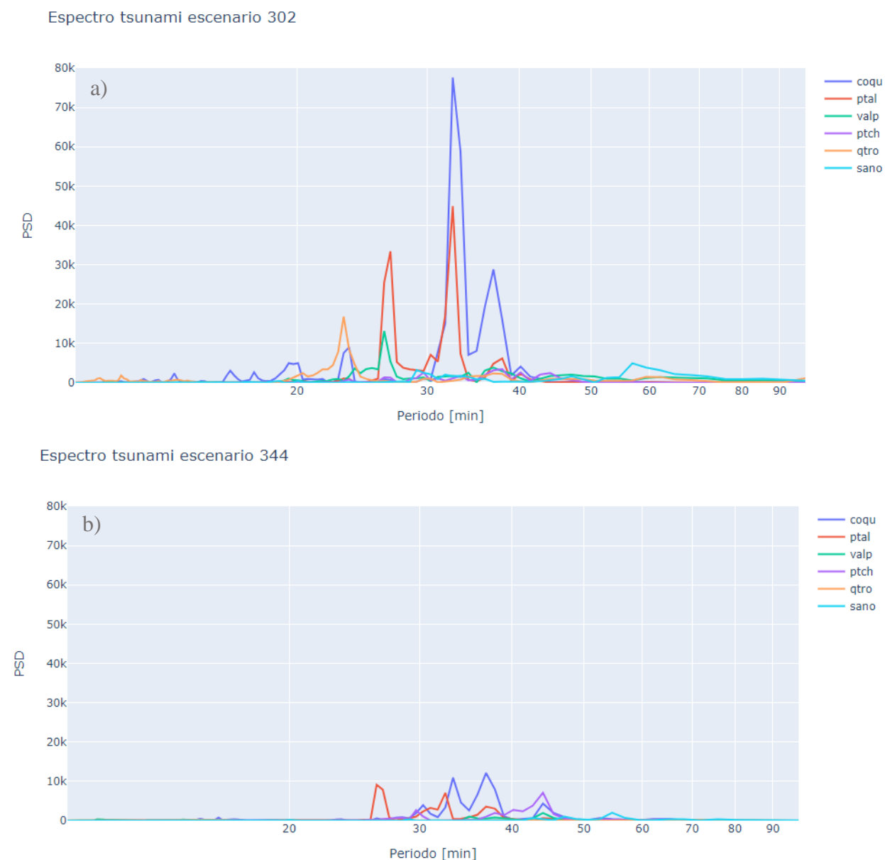
Figura 6-2: Espectro para Coquimbo (coqu), Puerto Aldea (ptal), Valparaíso (valp), Punta de Choros (ptch), Quintero (qtro) y San Antonio (sano) – a) Escenario 302 y b) Escenario 344.
