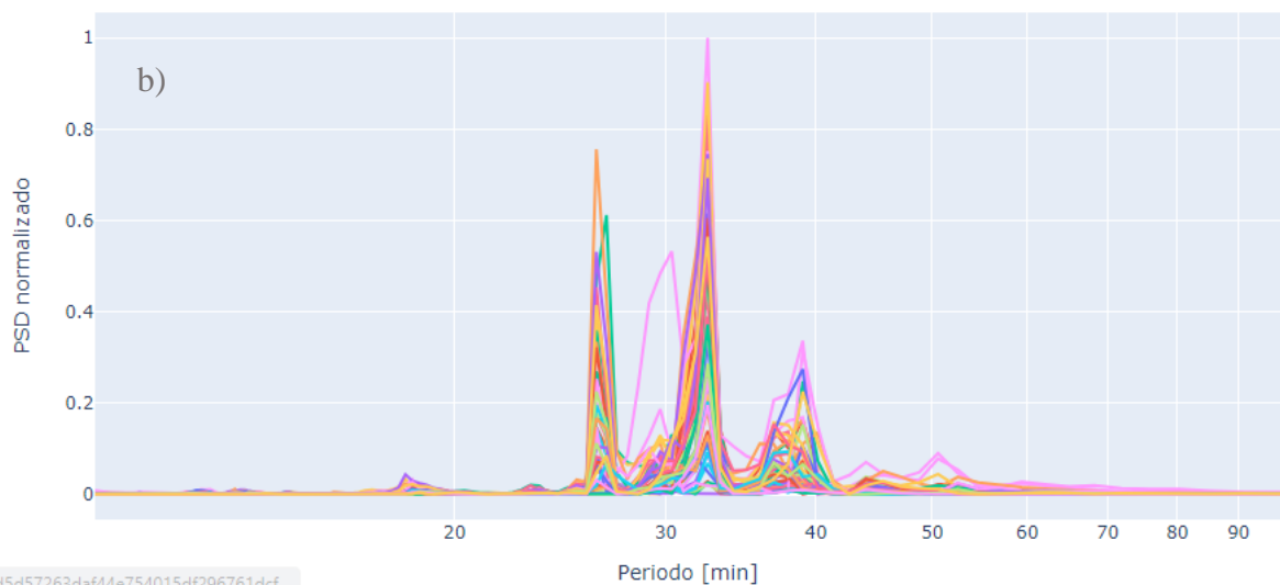
Figura 5-4: Espectro normalizado de los 50 escenarios simulados para a) magnitud Mw 8.6 y b) magnitud Mw 9.2 Bahía Tongoy.
