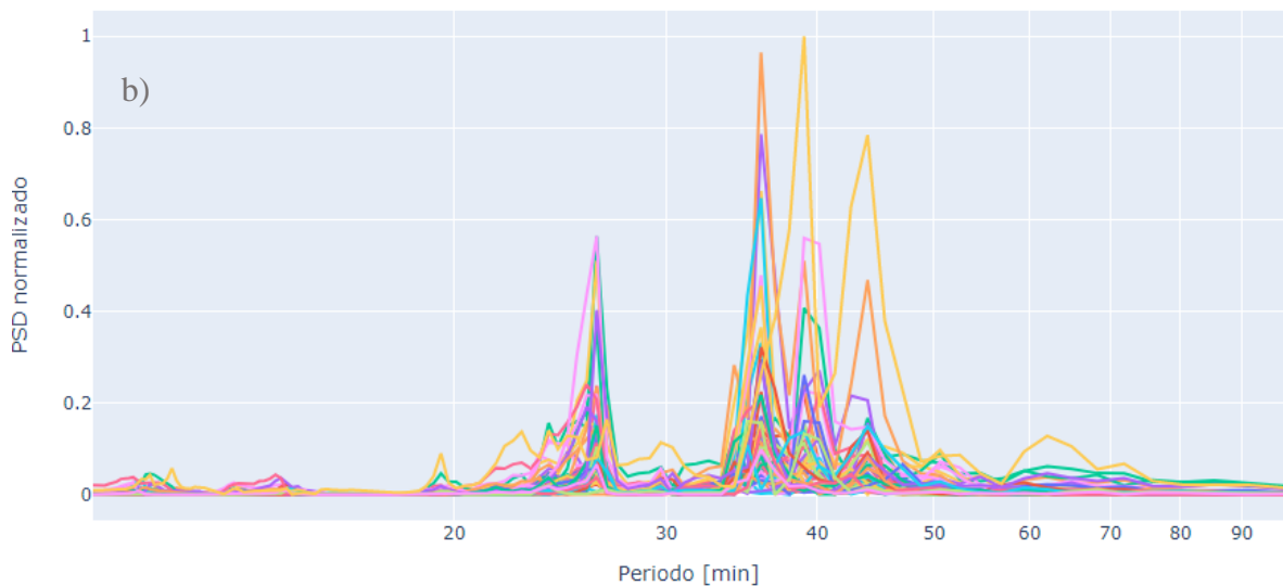
Figura 5-6: Espectro normalizado de los 50 escenarios simulados para a) magnitud Mw 8.6 y b) magnitud Mw 9.2 Bahía Valparaíso.
