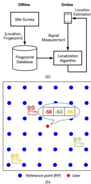
Figura 3.11: (a) Flujo básico de fingerprint. (b) radio-map de un sistema de localización indoor
