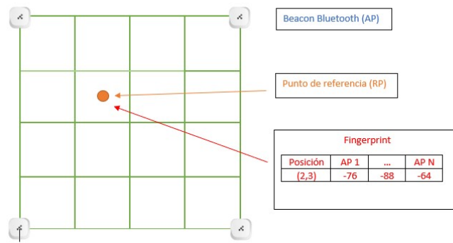
Figura 4.9: Ejemplo de grilla utilizada, con sus puntos de referencia y los Fingerprints leídos, que corresponden a vectores de señales RSSI
