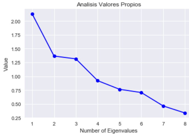
Figura 5.15: Análisis de los valores propios obtenidos a partir de la matriz de covarianza utilizada en el algoritmo PCA (Fuente: Elaboración Propia)
