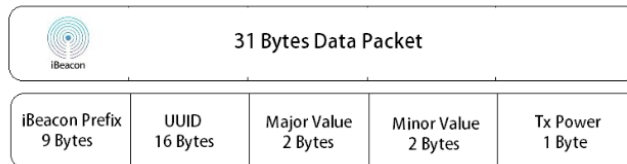
Figura 4.2: Paquete iBeacon realizado por Apple.
