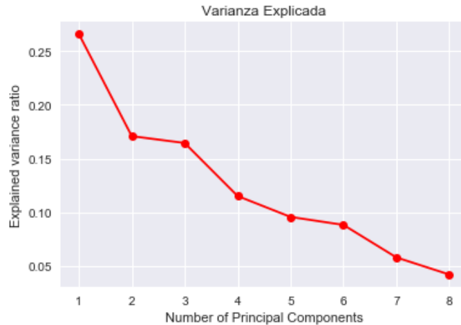
Figura 5.16: Proporción de la varianza explicada respecto a la varianza total para cada componente ordenada por su valor en orden descendente
