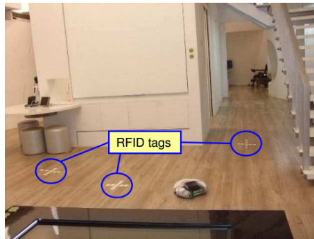
Figura 3.10: Robot que toma automáticamente las características para elaborar el mapeo fingerprint de un determinado lugar.
