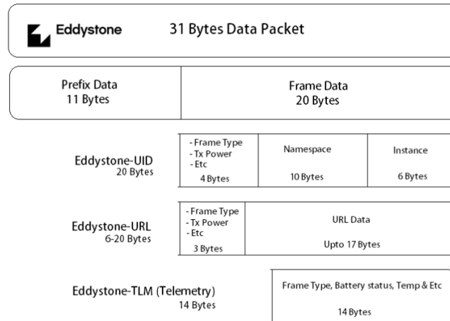
Figura 4.1: Tipos de paquetes Eddystone con su respectivo tamaño.
