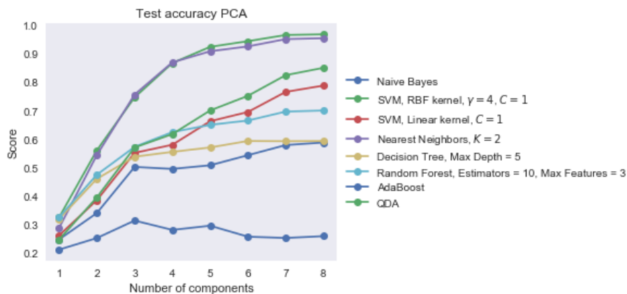
Figura 5.17: Comparativa de resultados obtenidos por los clasificadores utilizando PCA
