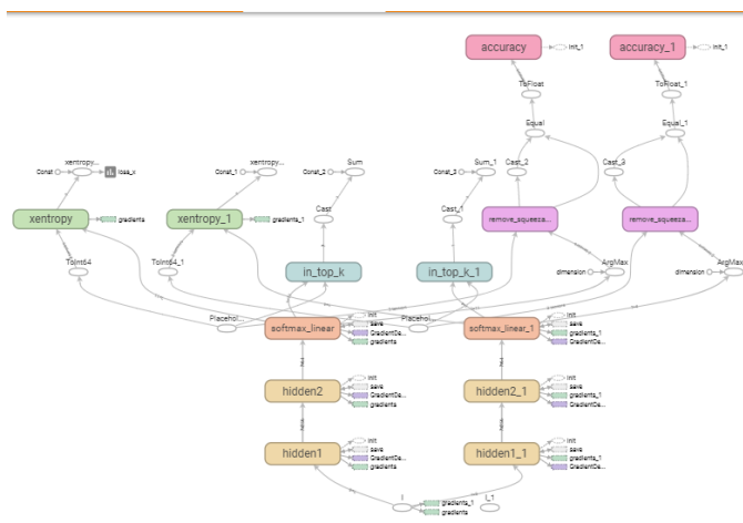
Figura 5.13: Estructura de las redes neuronales construidas. En la figura se muestran ambas, tanto X como Y (Fuente: Elaboración Propia)
