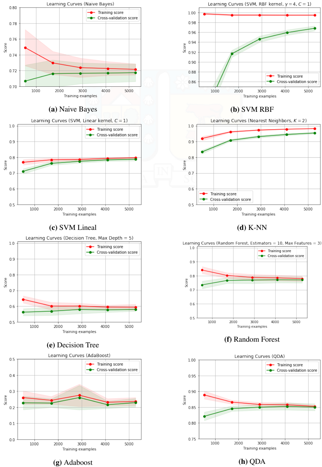
Figura 5.12: Curvas de aprendizajes obtenidas por cada clasificador
