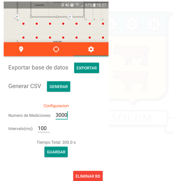
Figura 5.8: Pestaña de configuración de la aplicación Android, donde se puede configurar el tiempo y exportar la base de datos a CSV
