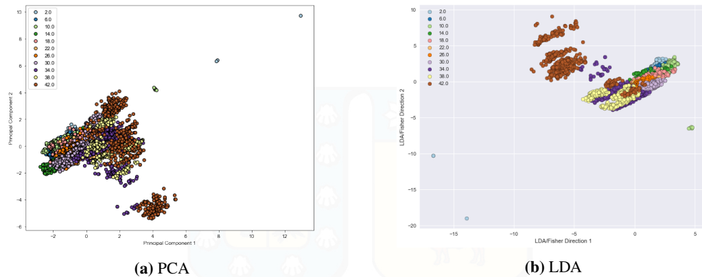
Figura 5.11: Comparativa entre los algoritmos PCA y LDA aplicado a los datos
