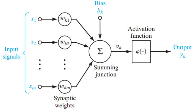
Figura 4.7: Esquema básico de single layer perceptron (Fuente: Syed Danish Ali (2016))
