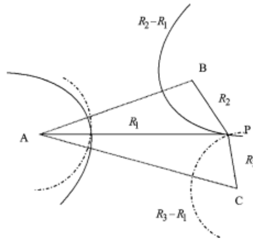
Figura 3.7: Curvas hiperbólicas de TDoA que estiman la posición basado en el tiempo de transmisión.
