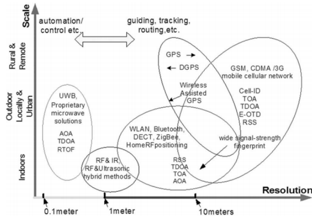
Figura 3.5: Comparativa de distintas tecnologías inalámbricas basado en su resolución y alcance.
