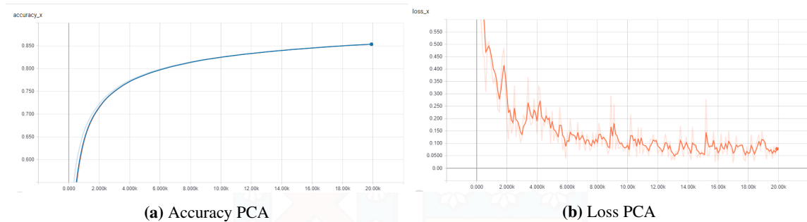
Figura 5.19: Accuracy y Loss(Costo) obtenidos en el entrenamiento de la red neuronal profunda con dos capas ocultas utilizando PCA con 5 componentes principales.
