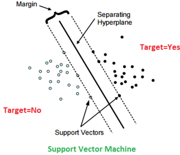
Figura 4.6: Ejemplo SVM en dos dimensiones, en donde se muestran los vectores de soporte y el hiperplano que logra la máxima separación
