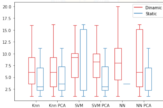
Figura 6.3: Diagrama de cajas para método estático y dinámico
