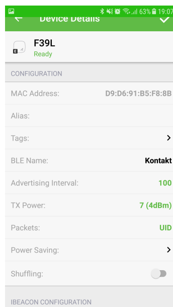
Figura 5.4: Configuración que ejemplifica los valores definidos para TX Power y el intervalo de transmisión (Fuente: Elaboración Propia)
