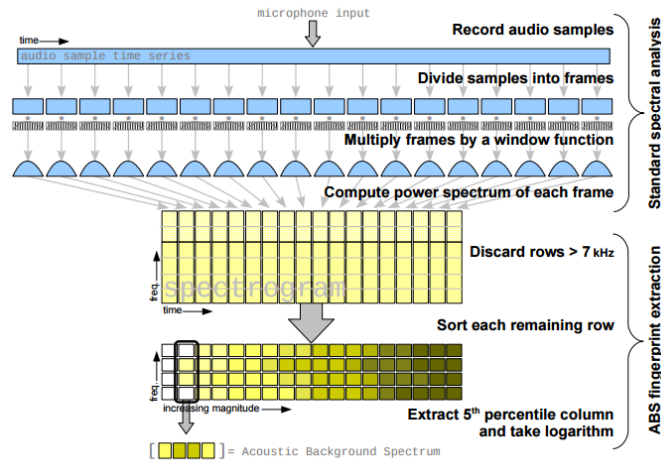
Figura 3.3: Descripción del método ABS con el cual se realiza la obtención del mapeo fingerprint
