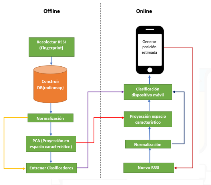
Figura 4.10: Framework desarrollado para resolver el problema de posicionamiento en interiores (Fuente: Elaboración propia)
