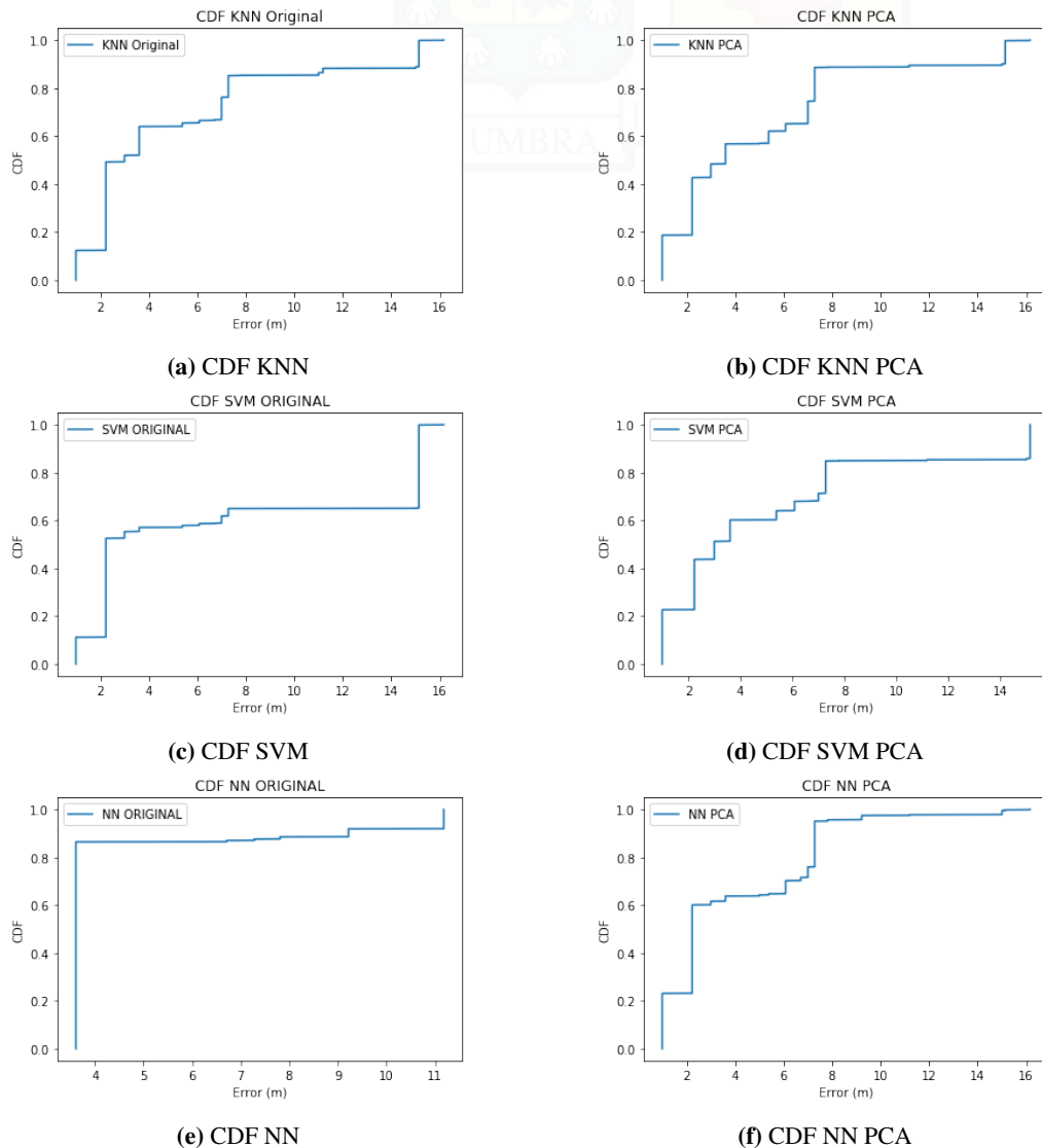
Figura 6.2: Cumulative distribution function para el método estático obtenido utilizando los distintos algoritmos (Fuente: Elaboración Propia)
