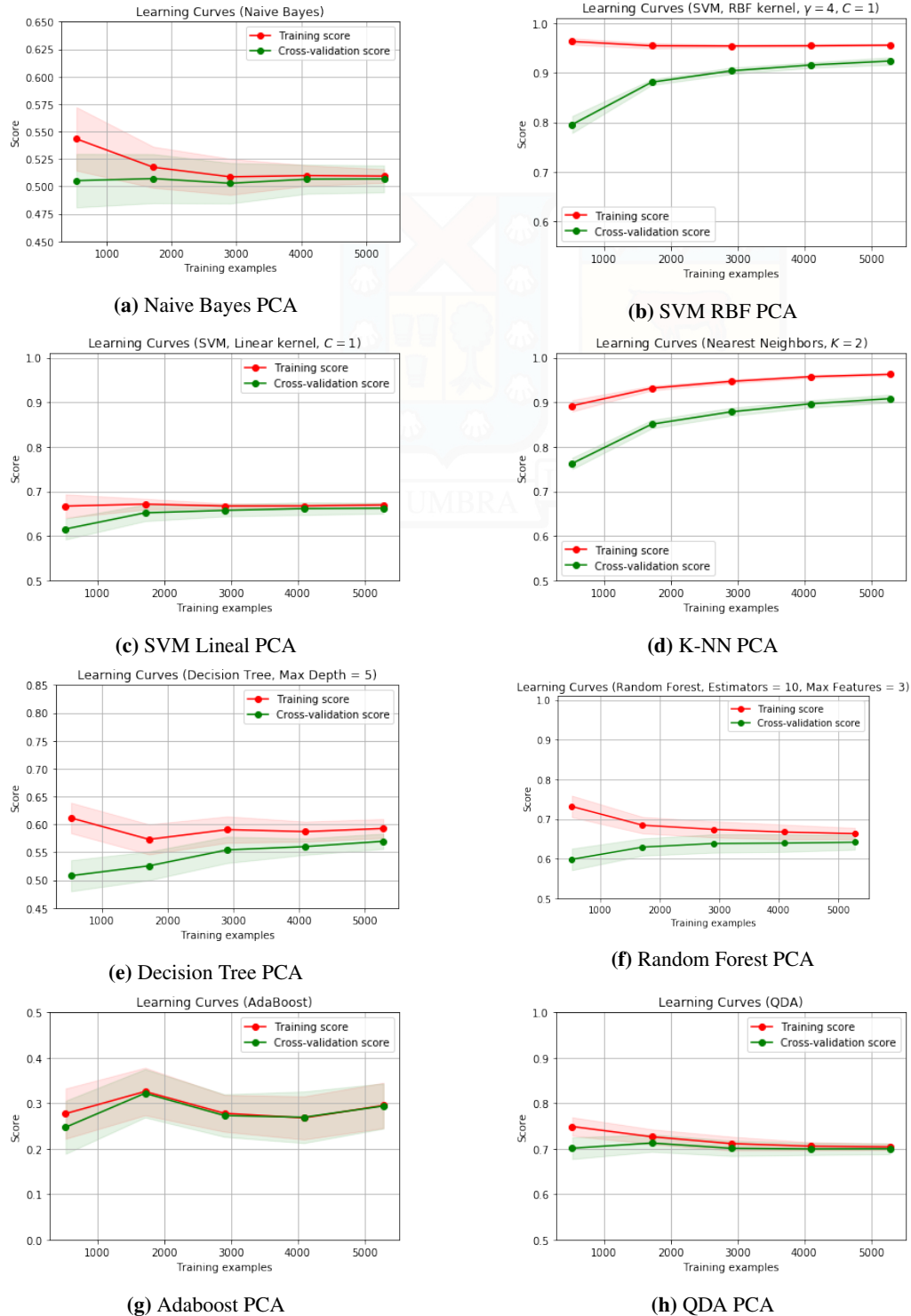
Figura 5.18: Curvas de aprendizajes obtenidas por cada clasificador utilizando PCA con 5 componentes (Fuente: Elaboración Propia)
