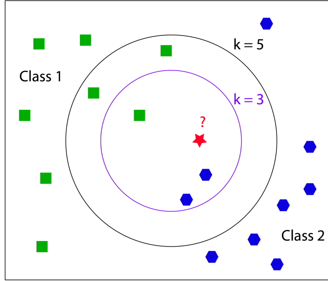
Figura 4.5: Ejemplo de clasificación utilizando k-nn con k = 5 y k = 3
