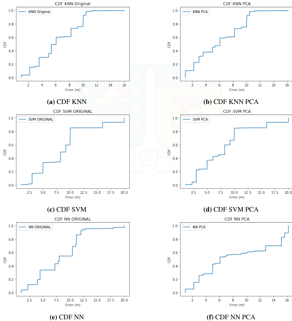
Figura 6.1: Cumulative distribution function para el método dinámico obtenido utilizando los distintos algoritmos (Fuente: Elaboración Propia)
