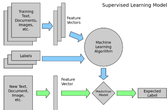
Figura 4.4: Esquema básico del funcionamiento de las técnicas de aprendizaje automático
