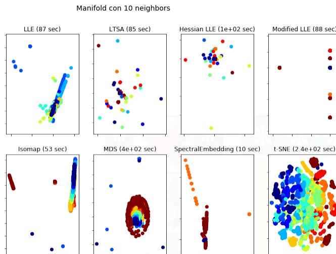
Figura 5.10: Comparación de los diferentes algoritmos Manifold para la reducción de la dimensionalidad con sus respectivos tiempos de ejecución.
