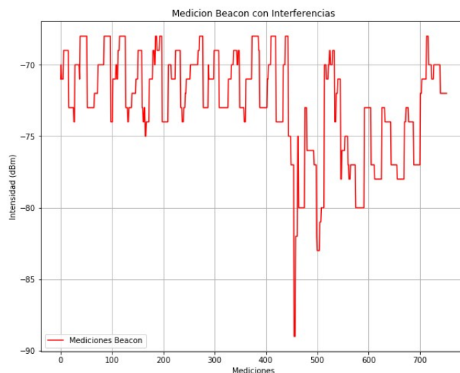
Figura 4.3: Resultados del cambio en la señal producto de una persona caminando delante de la línea entre un Beacon y un teléfono celular receptor (Fuente: Elaboración propia)
