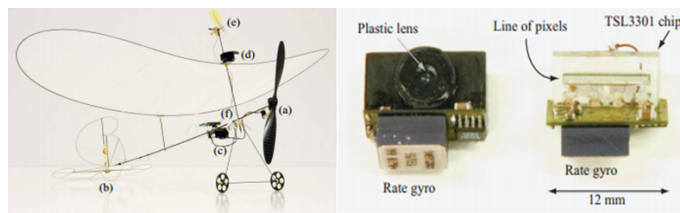
Figura 3.1: Dispositivo volador que toma imágenes de las murallas para detectar los patrones de textura
