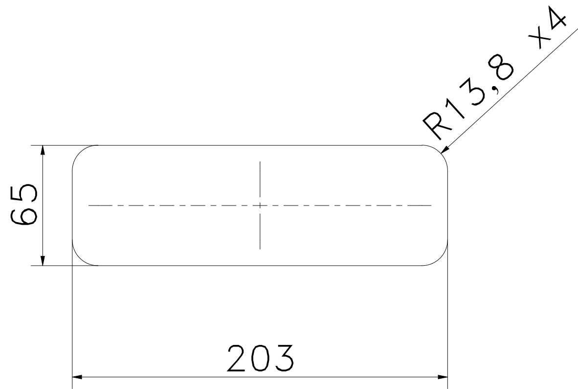
VISTA ALZADO Espesor: 8 mm
