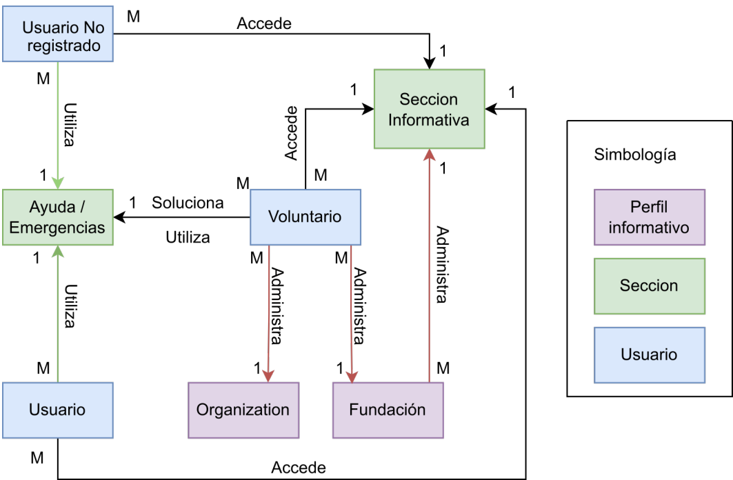
Figura 8: Modelo de Dominio del sistema propuesto
