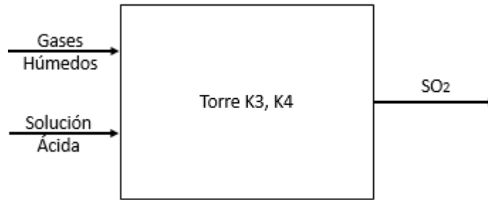
Figura 12: Diagrama EMS, Secado de Gases
