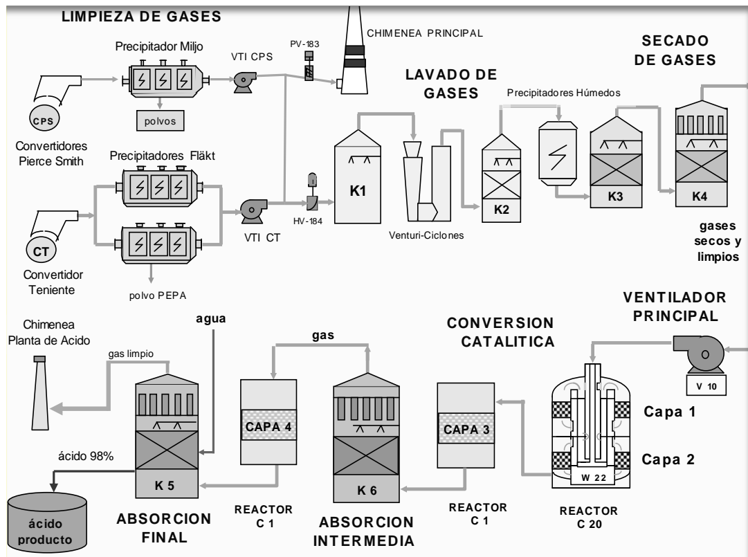
Figura 16: Esquema general de Planta de Ácido
