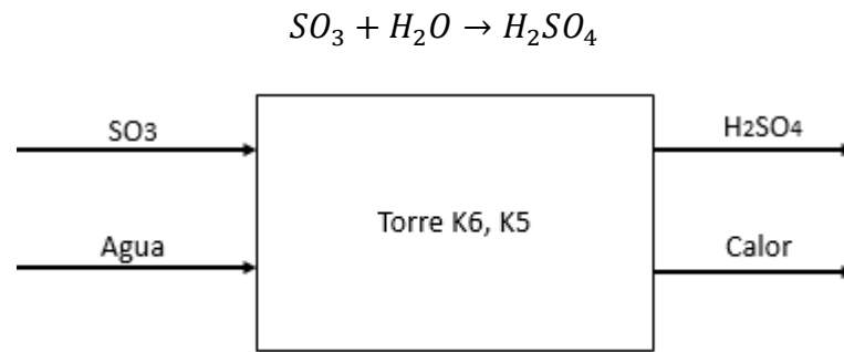
Figura 14: Diagrama EMS, Absorción de SO_3
