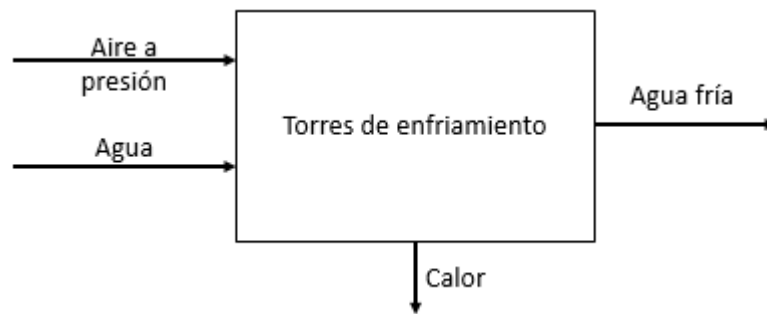
Figura 15: Diagrama EMS, Enfriamiento de agua
