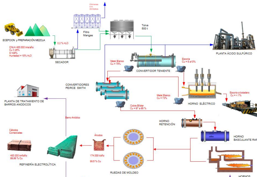
Figura 9: Esquema productivo Codelco División Ventanas
