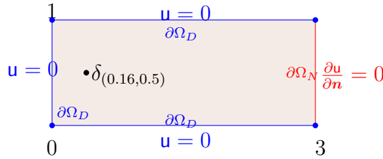
FIGURA 20. Dominio \Omega = (0, 3) \times (0, 1) , para el problema (8.7), de contaminación con fuente Delta de Dirac.
