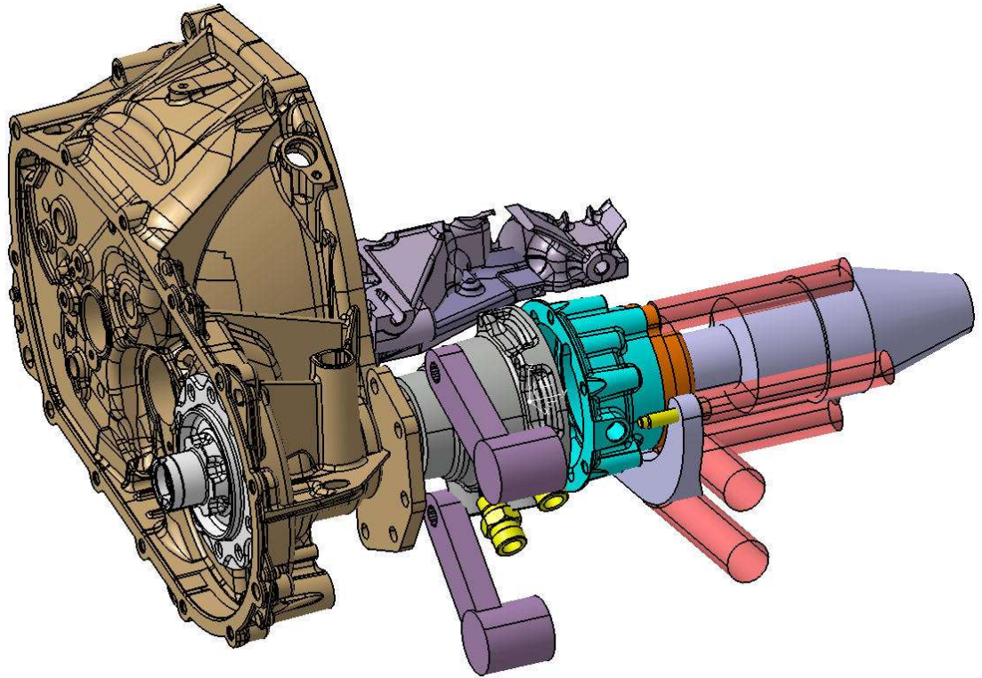
Ilustración 8 Conexión de línea diferencial con bomba de transmisión REF: RENAULT Coercánica
