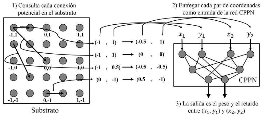
Figura 4.1: Interpretación del patrón geométrico de conectividad de un hipercubo usando \tau -HyperNEAT. Al igual que como funciona el método HyperNEAT (1) cada conexión potencial es consultada para determinar si esta existe, y de existir, cual sería su peso y su retardo asociado. (2) Por cada consulta, la red CPPN toma como entrada las coordenadas de los dos puntos terminales y (3) entrega como salida el peso y el retardo de la conexión entre ellos. Luego de que todas las conexiones han sido determinadas, un patrón de conexiones, pesos y retardos de conexión resultan en función de la geometría del substrato.
