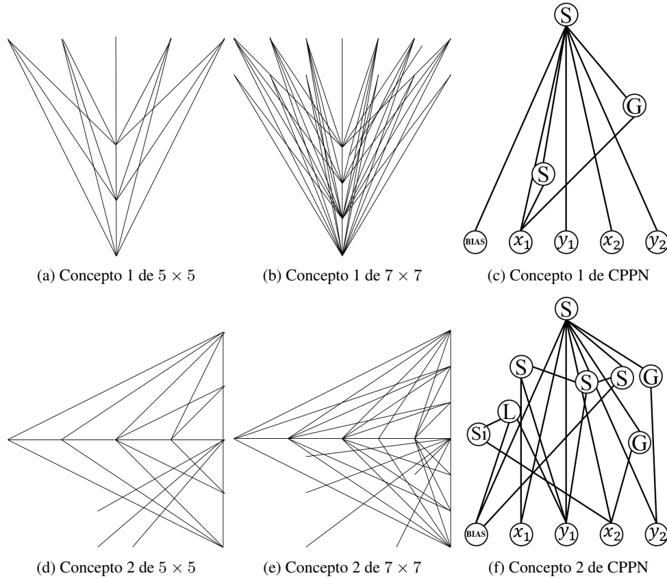
Figura 3.8: Conceptos de conectividad equivalentes en diferentes resoluciones del substrato. Se describen dos conceptos de conectividad generados en el proceso de evolución. La red CPPN que genera el primer concepto a resoluciones de 5 \times 5 (a) y 7 \times 7 (b) es mostrado en (c). La red CPPN en (f) genera de forma similar el segundo concepto en ambas resoluciones (d) y (e). Esta ilustración demuestra que CPPNs representan un concepto matemático en lugar de una sola estructura. Así, la misma red CPPN puede producir patrones con el mismo fundamento conceptual en diferentes resoluciones del substrato en diferente densidad de nodos. Las funciones de activación de las redes CPPN mostradas están denotadas por G para funciones Gaussianas , S para Sigmoides , Si para Senos , y L para Lineales . Imagen adaptada de [1].
