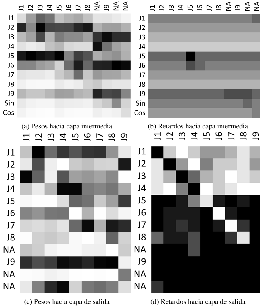
Figura 7.13: Diagramas de conexión del substrato de \tau -HyperNEAT para el robot Quadrotot. La figura muestra cuatro diagramas correspondientes a las magnitudes de los pesos y retardos asociados a las conexiones en el substrato entre la capa de entrada e intermedia, y entre la capa intermedia y de salida. En cada diagrama, el pixel (i, j) representa el peso, o el retardo según sea el caso, de la conexión desde el nodo i -ésimo de la capa origen hacia el nodo j -ésimo de la capa destino, escalados entre cero y el valor máximo ( \omega_{max} o \tau_{max} según corresponda). Las viñetas a la izquierda de cada fila y sobre cada columna indican el motor (joint) ligado a ella, Sin y Cos las entradas senoidales a la red, y NA nodos no asignados.
