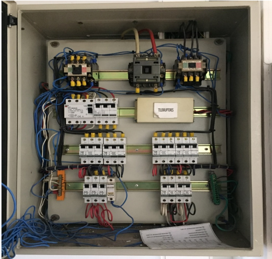
Figura 2-2 Interior del tablero
