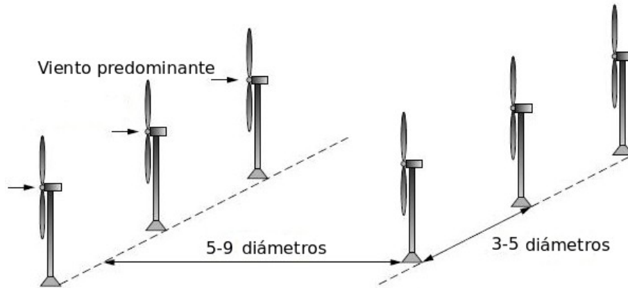
Figura 5.3: Ejemplo emplazamiento turbinas eólicas.
