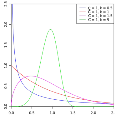
Figura 2.2: Función de distribución de probabilidad de Weibull Fuente: Adaptación propia desde [11].
