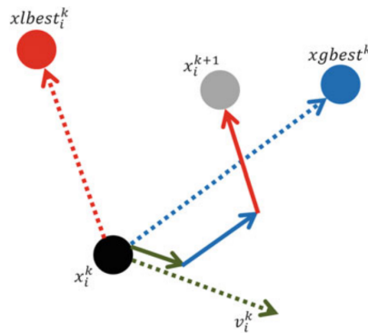
Figura 2.1: Movimiento de una partícula
