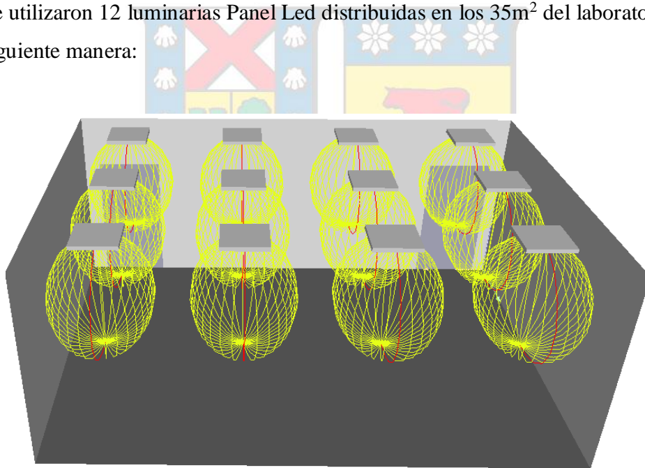
Imagen 22 Representación 3D de la distribución luminosa
