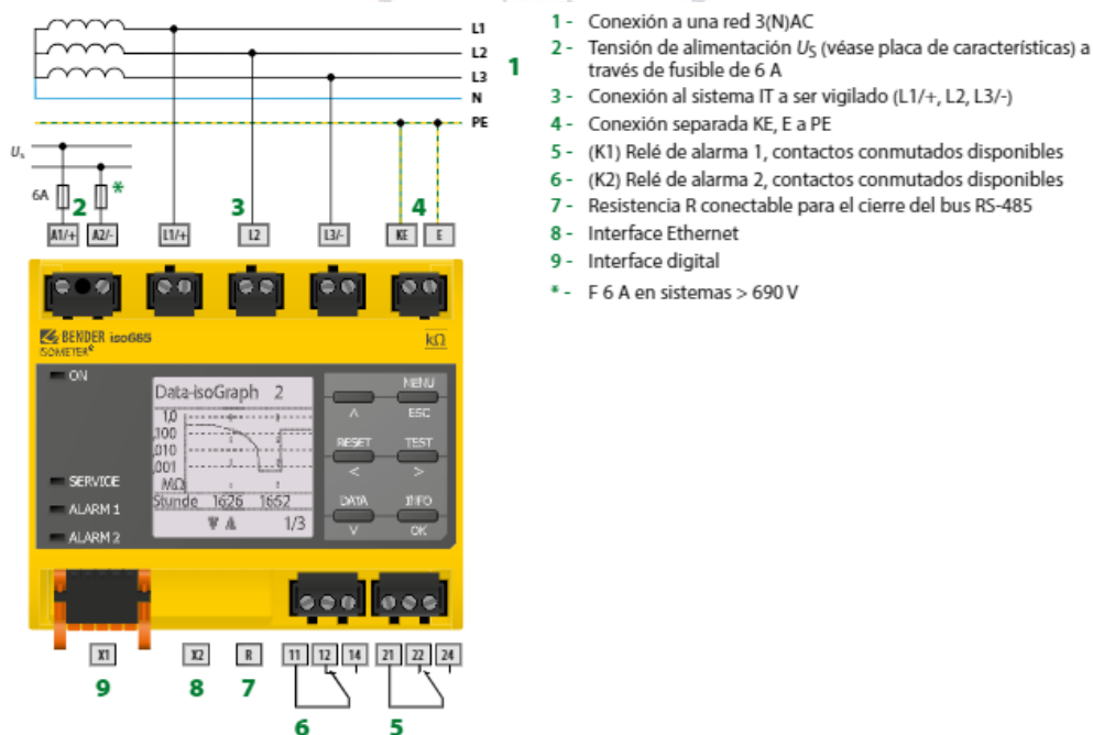
Imagen 19 Esquema de conexionado Vigilante isoNAV685-D
