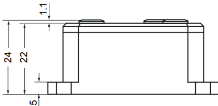
Imagen 31 Medidas físicas del rectificador B6U, PWS-A
