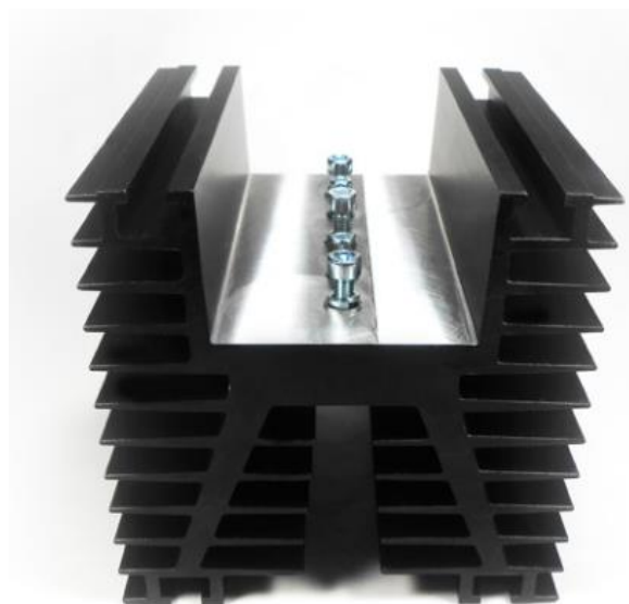
Imagen 33 Vista frontal Disipador de calor
