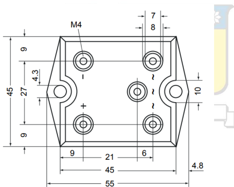
Imagen 32 Medidas físicas del rectificador B6U, PWS-A
