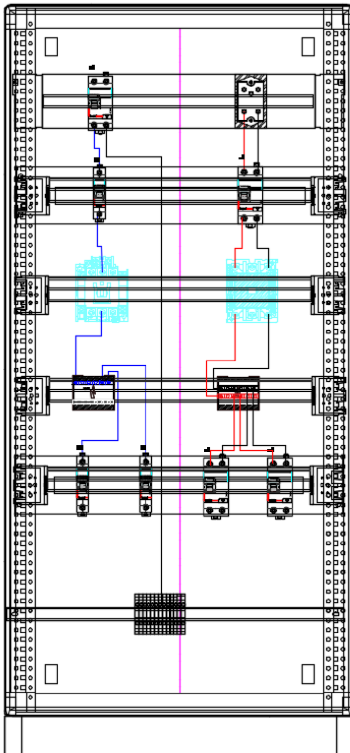
Imagen 38 Tableros 2x220 y 110Vcc
