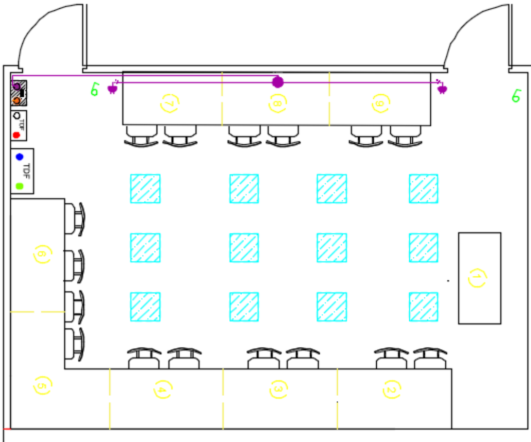
Imagen 7 Distribución de enchufes Alumbrado y S.G
