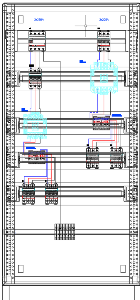
Imagen 37 Tableros circuito 3x380 y 3x220
