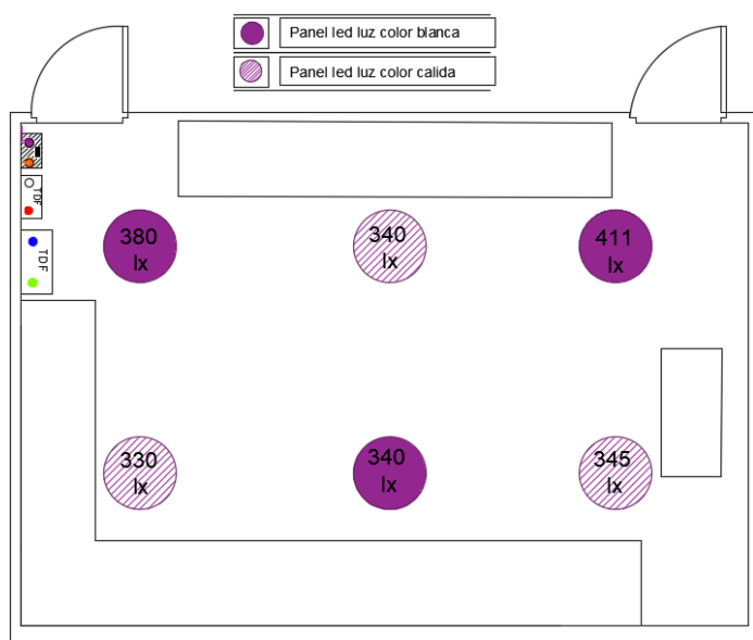
Imagen 4 Medidas de lúmenes L.A.2
