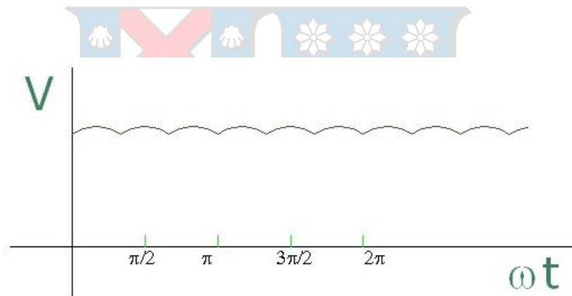
Imagen 28 Grafica de onda rectificada
