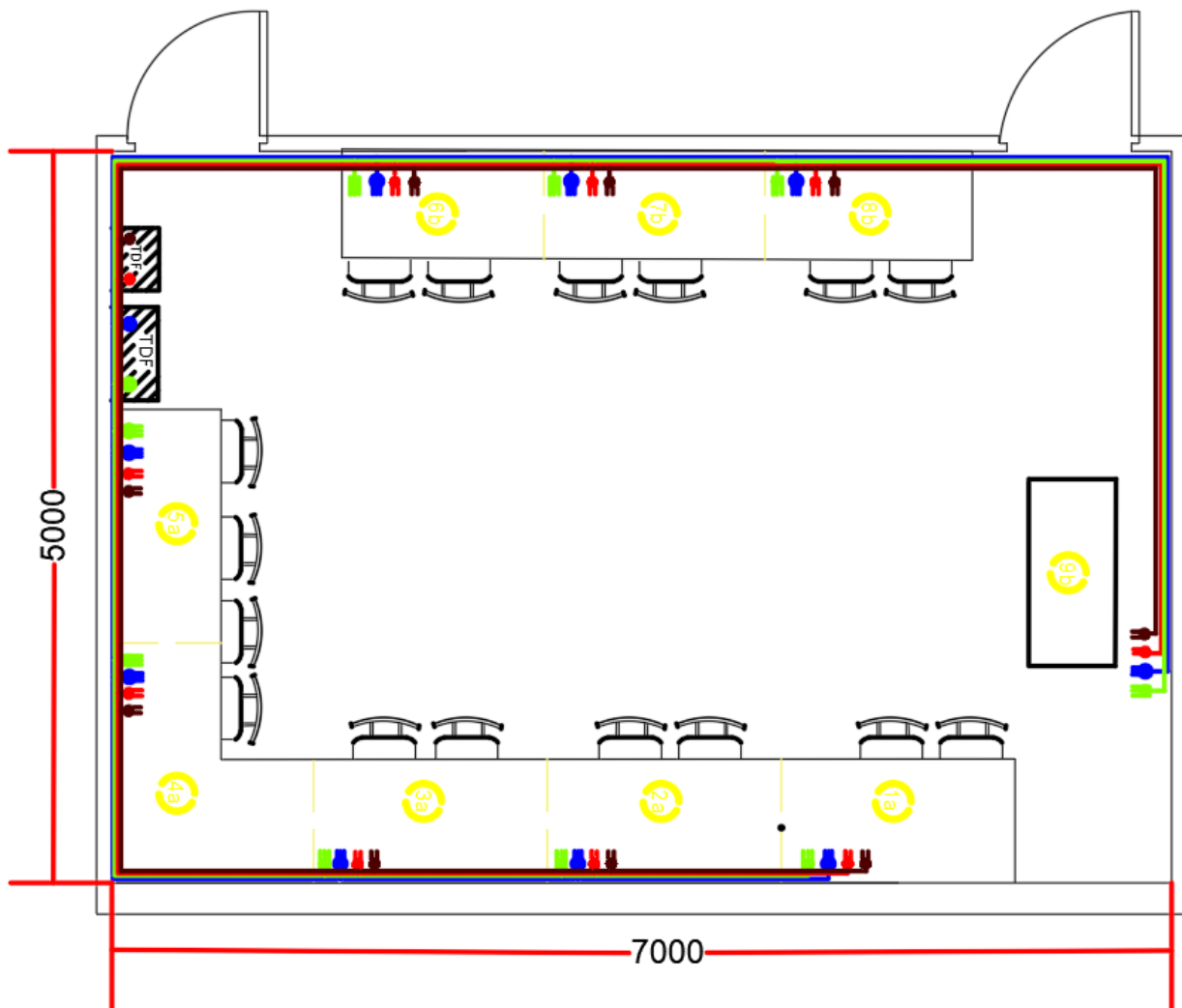
Imagen 34 Distribución enchufes LAB2
