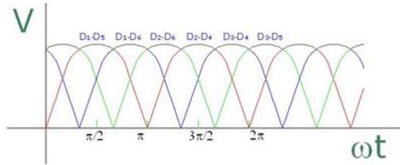
Imagen 27 Sinusoidal de rectificación de onda completa con conmutación de diodos
