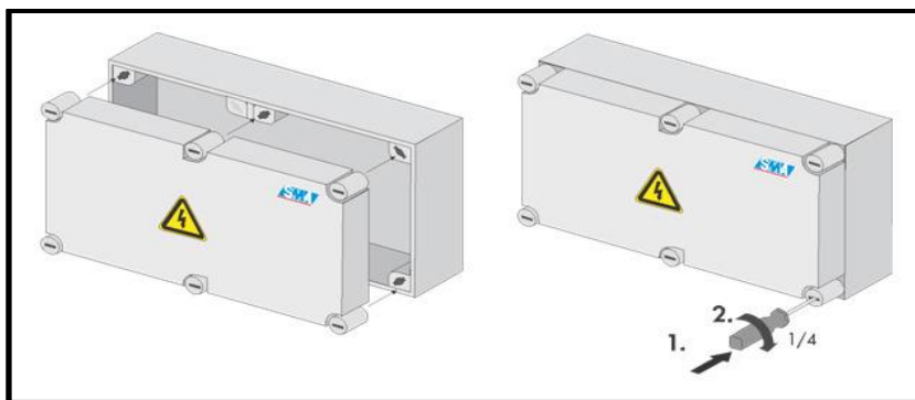
Figura 3-3. Tapa exterior de la caja de campo SSM
