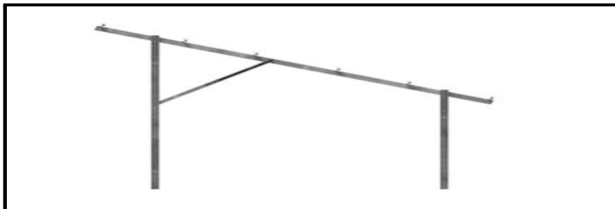
Figura 2-13. Estructura biposte utilizada en planta solar Doña Carmen
