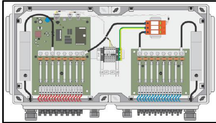
Figura 3-4. Interior de la caja de campo SSM
