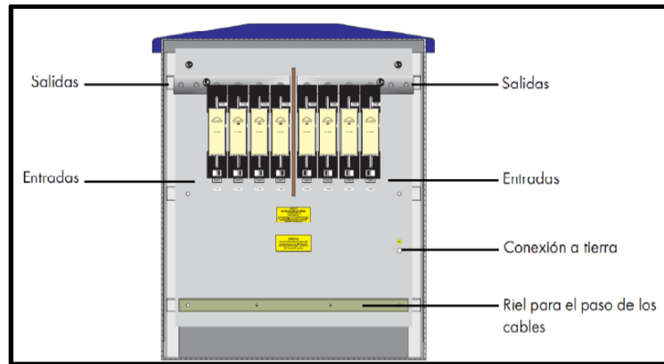
Figura 3-6. Estructura interna de la caja central SMBC
