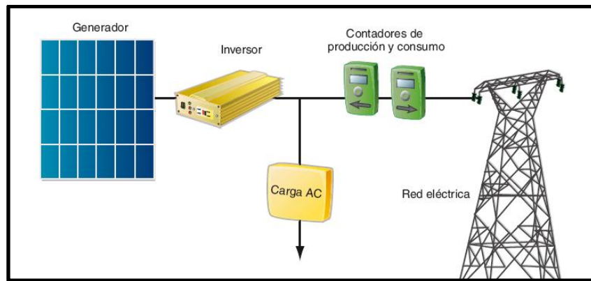
Figura 2-6. Instalación fotovoltaica conectada a la red, Inversor
