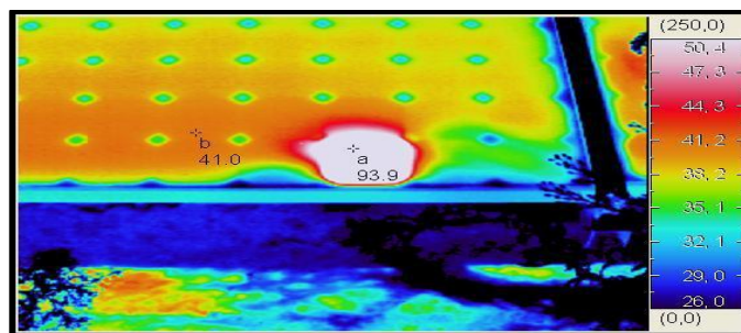
Figura 3-2. Termografía de un panel fotovoltaico
