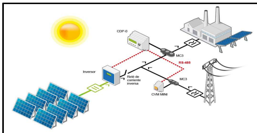
Figura 2-1. Esquema básico de una Planta Solar Fotovoltaica
