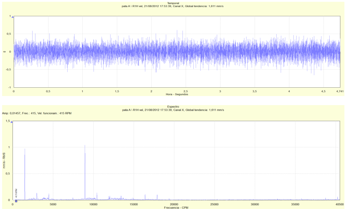
Figura 99: Señal temporal y espectro de vibración para la dirección horizontal de la pata lado succión de la bomba RABI 8 para un flujo impulsado de 988 m 3 /h
