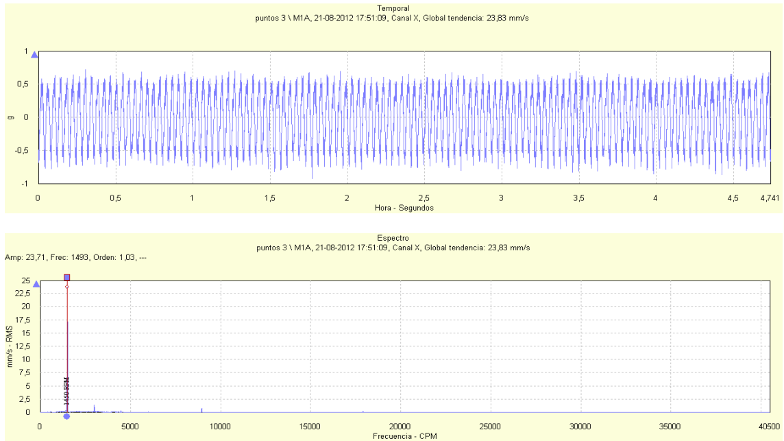
Figura 72: Señal temporal y espectro de vibración para la dirección axial del ducto de descarga de la bomba RABI 8 para un flujo impulsado de 988 m 3 /h
