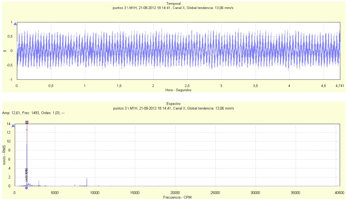
Figura 67: Señal temporal y espectro de vibración para la dirección horizontal del ducto de descarga de la bomba RABI 8 para un flujo impulsado de 610 m 3 /h
