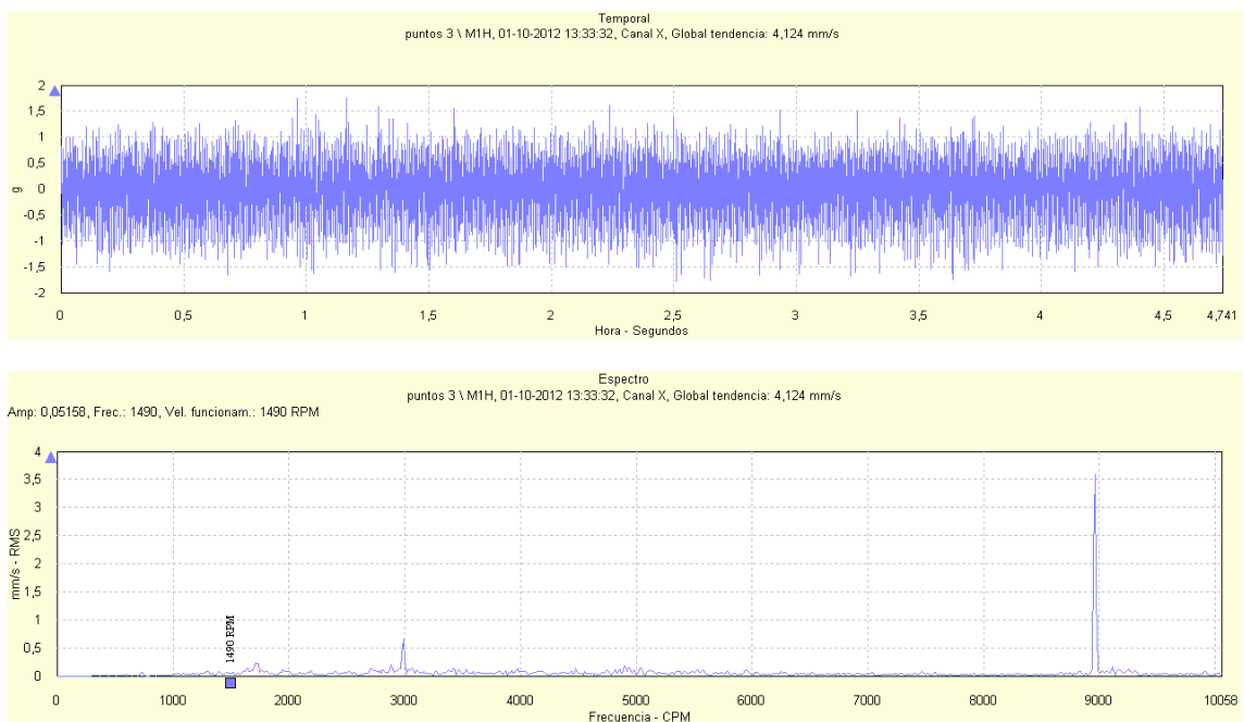
Figura 162: Señal temporal y espectro de vibración para la dirección horizontal del ducto de descarga de la bomba RABI 8 para un flujo impulsado de 650 m 3 /h
