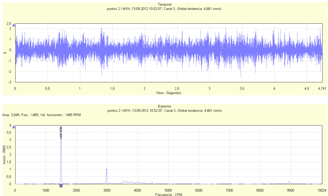
Figura 121: Señal temporal y espectro de vibración para la dirección horizontal del ducto de succión de la bomba RABI 6 para un flujo impulsado de 800 m 3 /h
