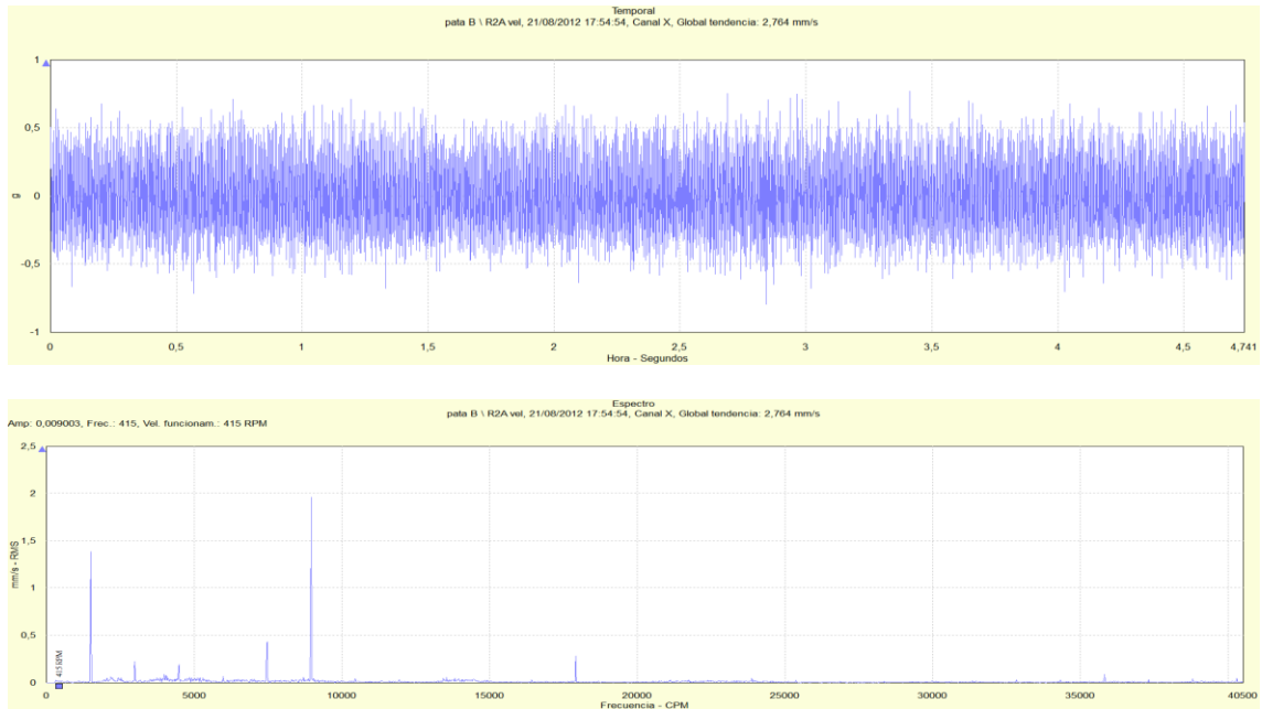
Figura 104: Señal temporal y espectro de vibración para la dirección axial de la pata lado descarga de la bomba RABI 8 para un flujo impulsado de 988 m 3 /h
