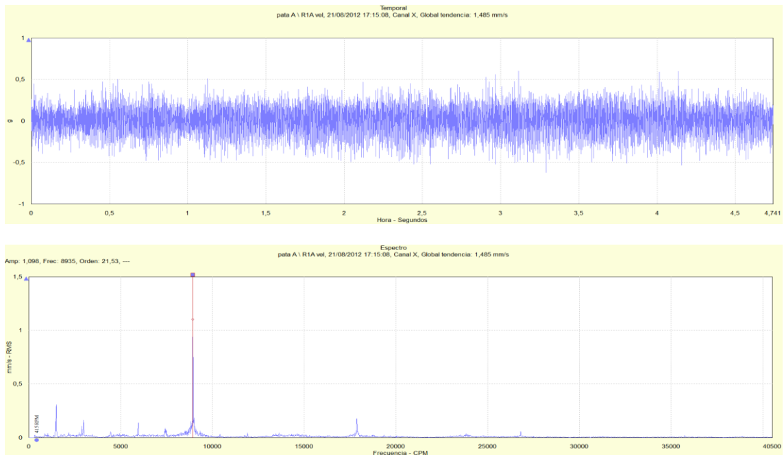
Figura 47: Señal temporal y espectro de vibración para la dirección axial de la pata lado succión de la bomba RABI 7 para un flujo impulsado de 1 030 m 3 /h
