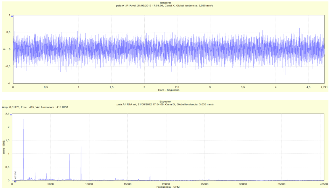
Figura 98: Señal temporal y espectro de vibración para la dirección axial de la pata lado succión de la bomba RABI 8 para un flujo impulsado de 988 m 3 /h
