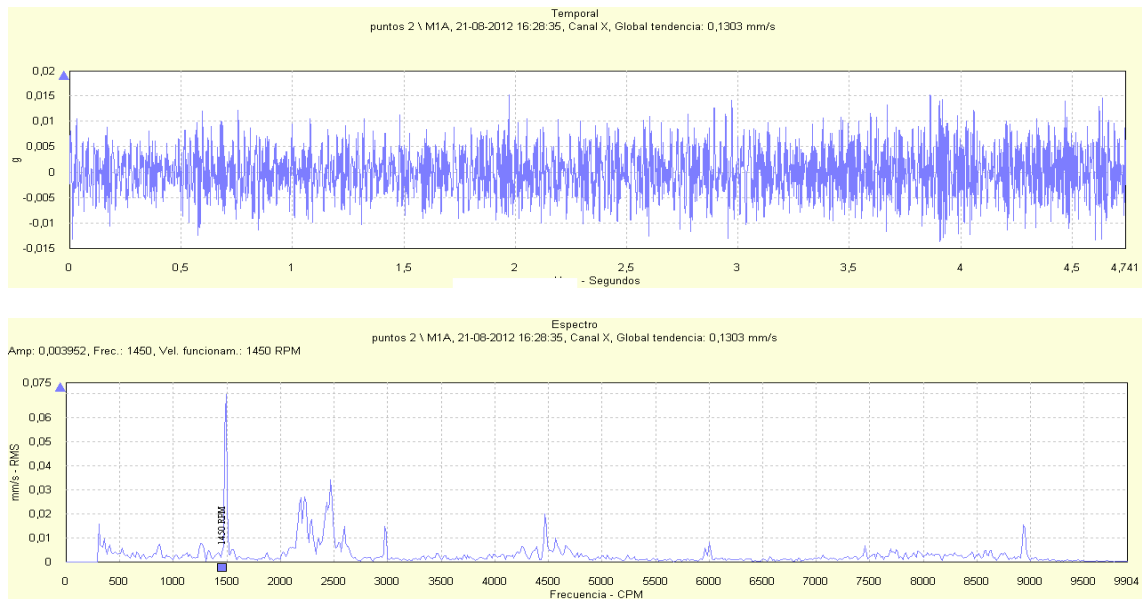
Figura 107: Señal temporal y espectro de vibración para la dirección axial del ducto de succión de la bomba RABI 8 para la condición de operación de la bomba RABI 7.
