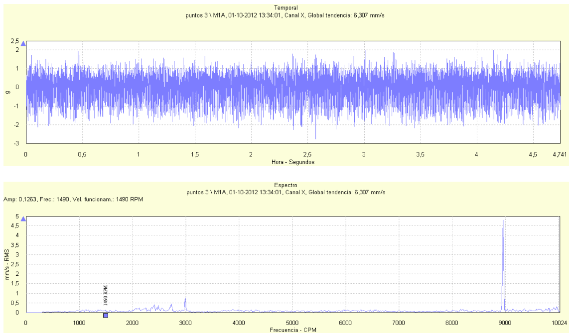
Figura 161: Señal temporal y espectro de vibración para la dirección axial del ducto de descarga de la bomba RABI 8 para un flujo impulsado de 650 m 3 /h
