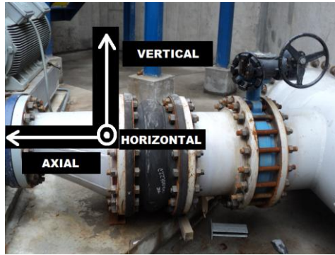
Figura 2, Definición de puntos de medición y direcciones ducto de alimentación
