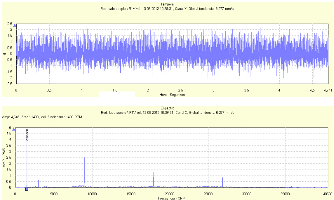
Figura 147: Señal temporal y espectro de vibración para la dirección vertical del porta-rodamientos lado acople de la bomba RABI 6 para un flujo impulsado de 650 m 3 /h
