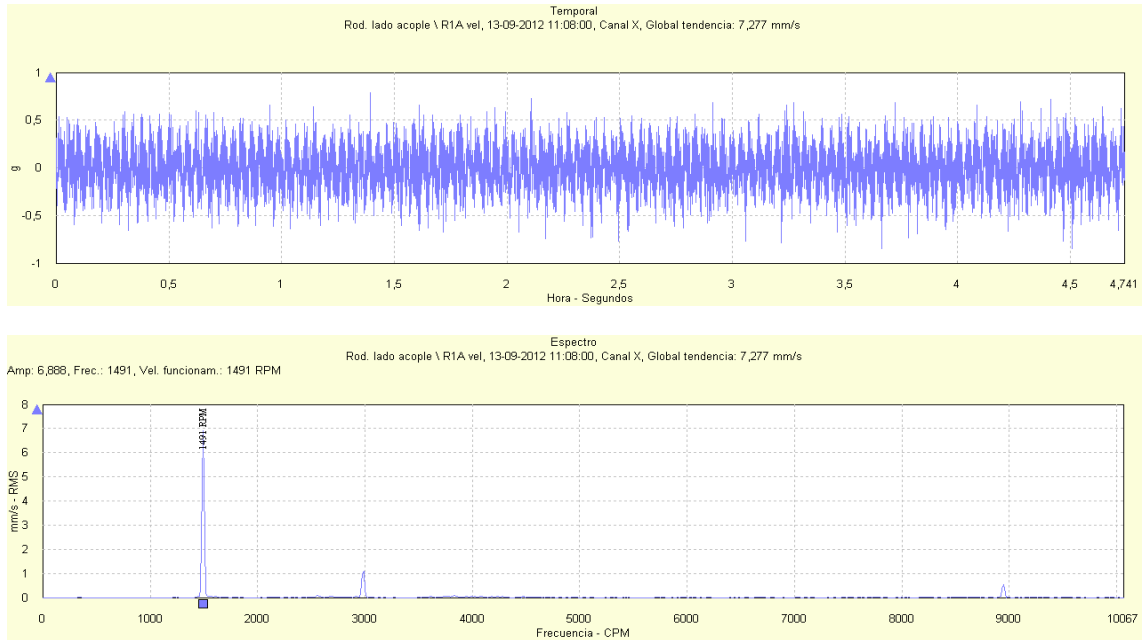
Figura 151: Señal temporal y espectro de vibración para la dirección axial del porta-rodamientos lado acople de la bomba RABI 6 para un flujo impulsado de 1 000 m 3 /h
