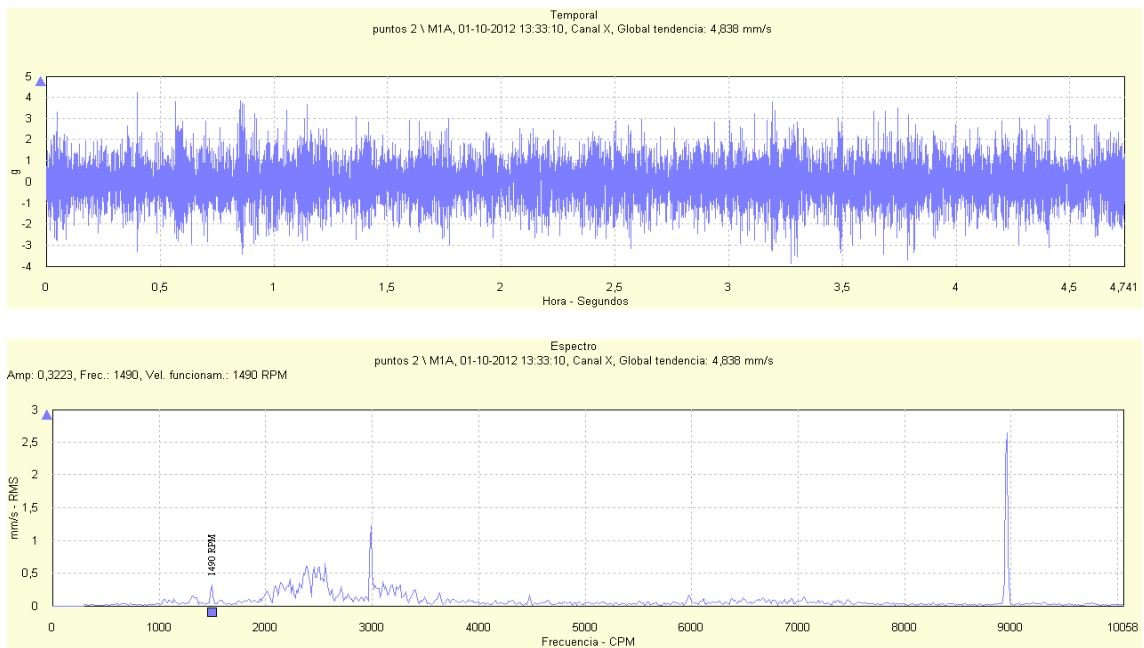
Figura 155: Señal temporal y espectro de vibración para la dirección axial del ducto de succión de la bomba RABI 8 para un flujo impulsado de 650 m 3 /h
