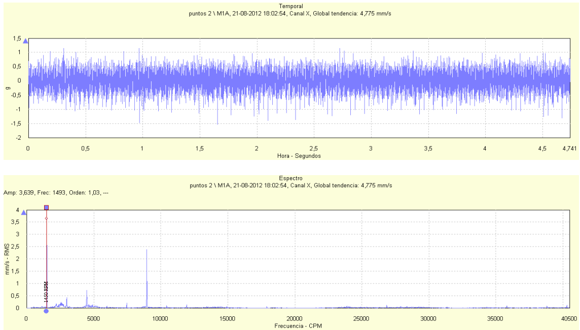
Figura 60: Señal temporal y espectro de vibración para la dirección axial del ducto de succión de la bomba RABI 8 para un flujo impulsado de 760 m 3 /h
