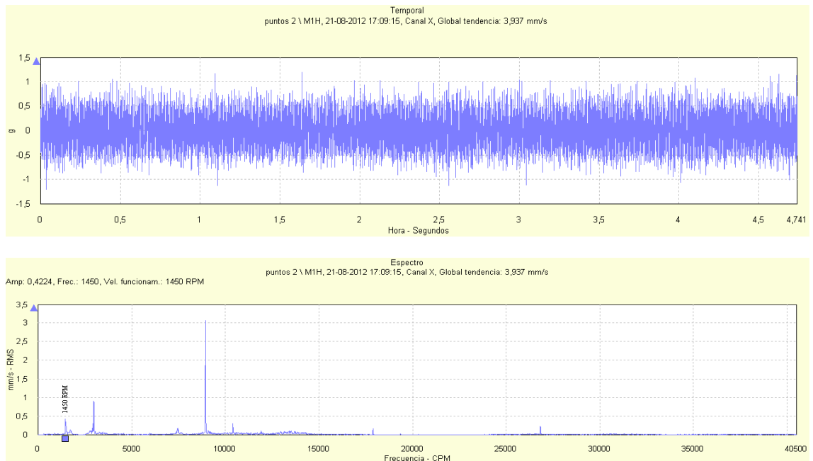
Figura 13: Señal temporal y espectro de vibración para la dirección horizontal del ducto de succión de la bomba RABI 7 para un flujo impulsado de 1 030 m 3 /h
