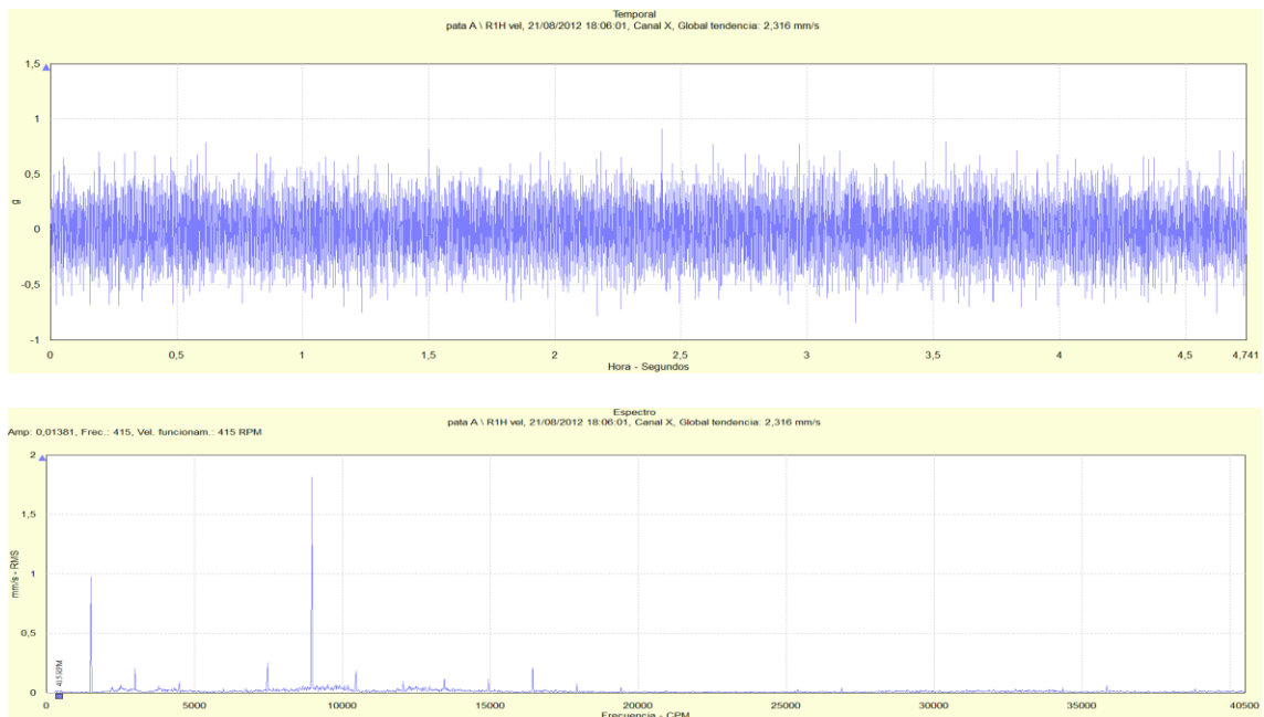
Figura 96: Señal temporal y espectro de vibración para la dirección horizontal de la pata lado succión de la bomba RABI 8 para un flujo impulsado de 760 m 3 /h
