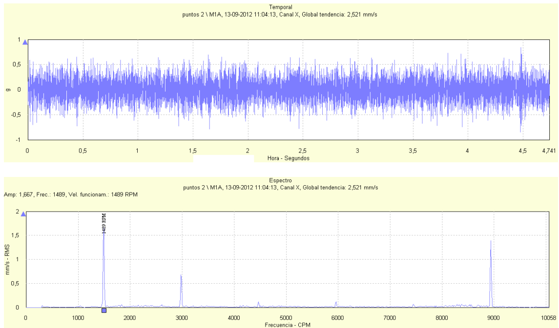
Figura 123: Señal temporal y espectro de vibración para la dirección axial del ducto de succión de la bomba RABI 6 para un flujo impulsado de 1 000 m 3 /h
