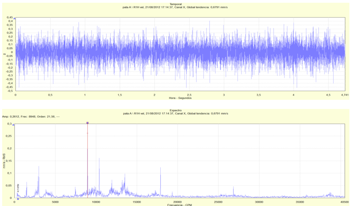
Figura 48: Señal temporal y espectro de vibración para la dirección horizontal de la pata lado succión de la bomba RABI 7 para un flujo impulsado de 1 030 m 3 /h
