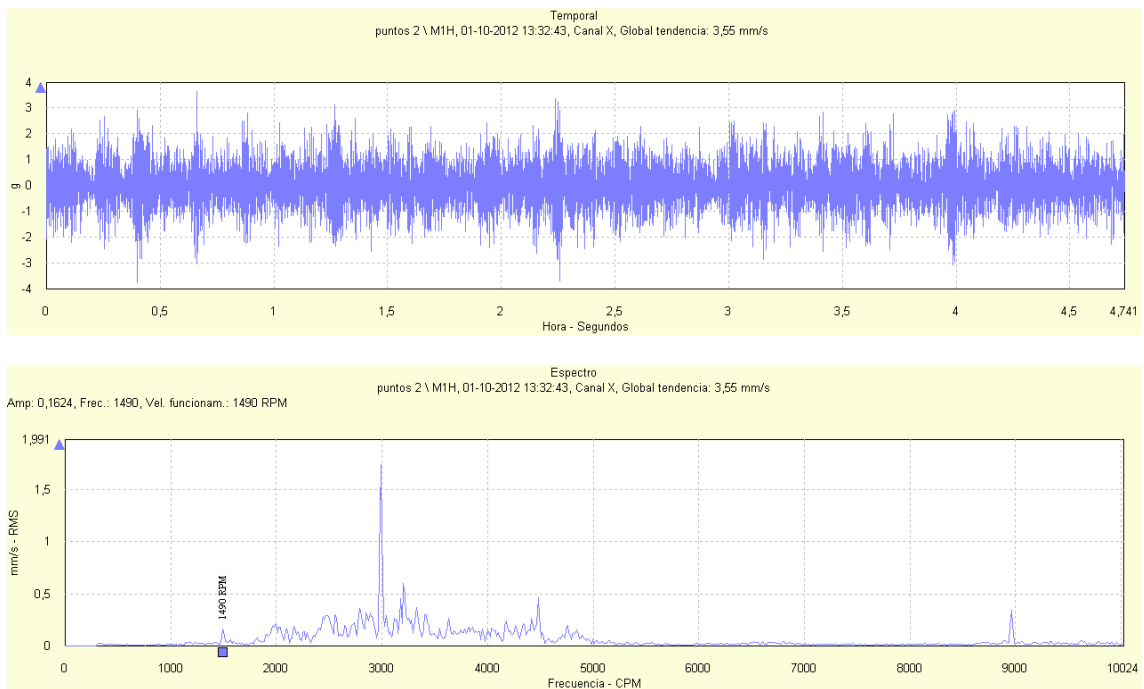
Figura 156: Señal temporal y espectro de vibración para la dirección horizontal del ducto de succión de la bomba RABI 8 para un flujo impulsado de 650 m 3 /h
