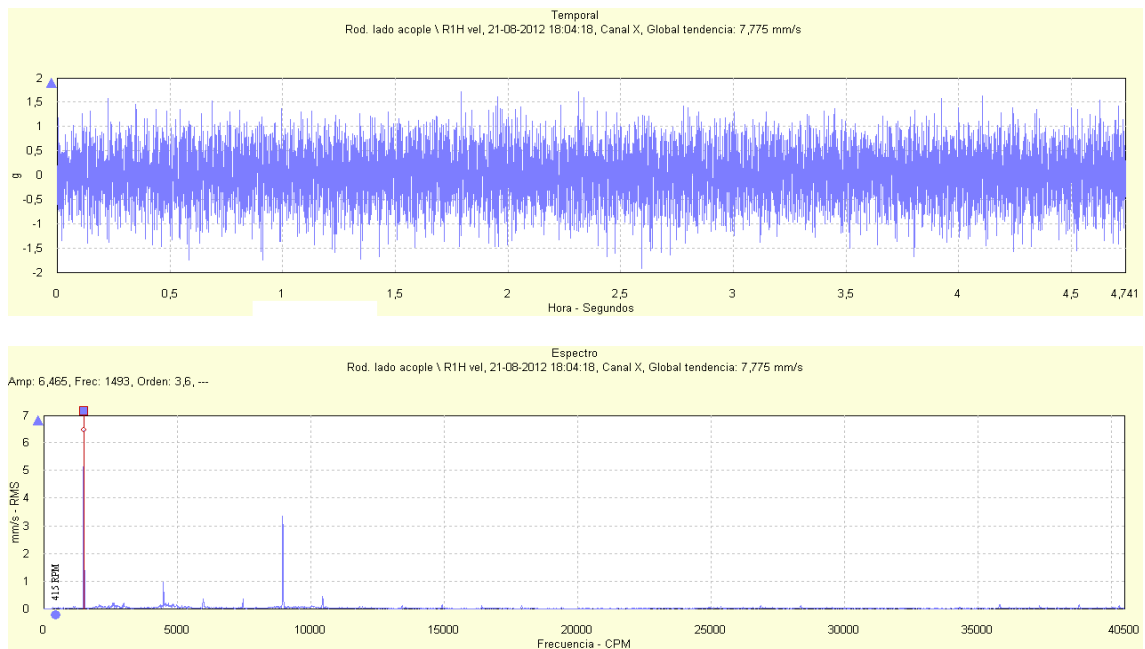
Figura 89: Señal temporal y espectro de vibración para la dirección horizontal del porta-rodamientos lado acople de la bomba RABI 8 para un flujo impulsado de 760 m 3 /h
