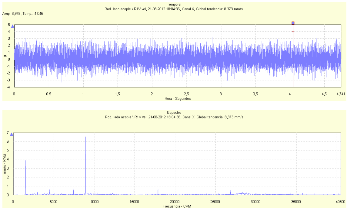
Figura 90: Señal temporal y espectro de vibración para la dirección vertical del porta-rodamientos lado acople de la bomba RABI 8 para un flujo impulsado de 760 m 3 /h
