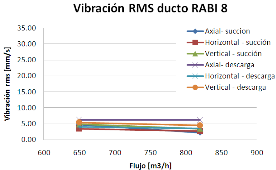
Figura 154, Nivel de vibración rms Ducto RABI 8 posterior a cambio de bomba
