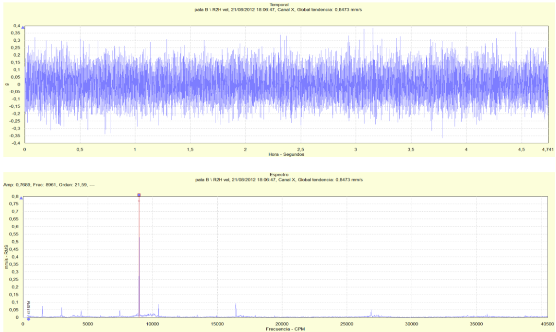
Figura 102: Señal temporal y espectro de vibración para la dirección horizontal de la pata lado descarga de la bomba RABI 8 para un flujo impulsado de 760 m 3 /h
