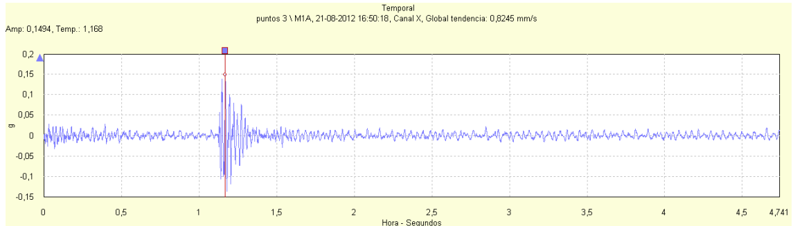
Figura 114: Señal temporal de vibración libre para la dirección axial del ducto de descarga de la bomba RABI 7 ante impacto realizado en un punto cercano.
