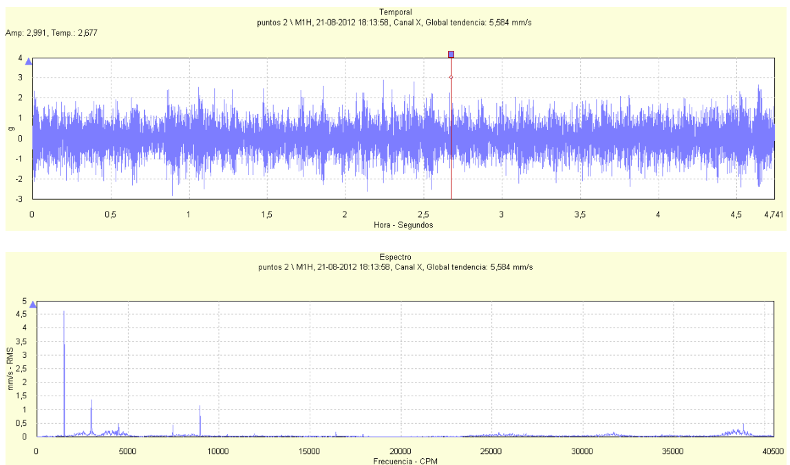
Figura 58: Señal temporal y espectro de vibración para la dirección horizontal del ducto de succión de la bomba RABI 8 para un flujo impulsado de 610 m 3 /h
