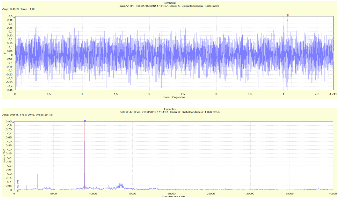
Figura 45: Señal temporal y espectro de vibración para la dirección horizontal de la pata lado succión de la bomba RABI 7 para un flujo impulsado de 770 m 3 /h
