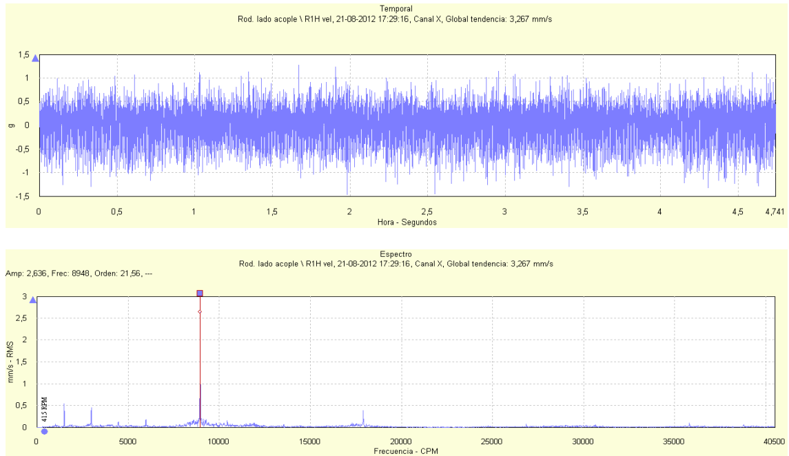
Figura 38: Señal temporal y espectro de vibración para la dirección horizontal del porta-rodamientos lado acople de la bomba RABI 7 para un flujo impulsado de 770 m 3 /h
