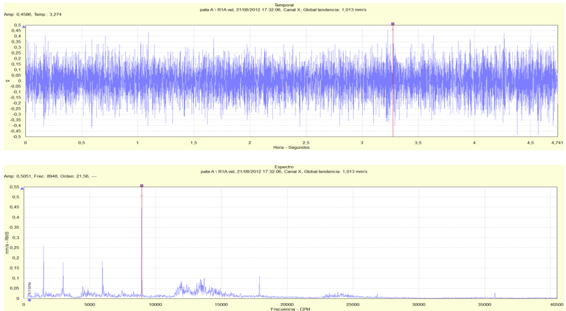
Figura 44: Señal temporal y espectro de vibración para la dirección axial de la pata lado succión de la bomba RABI 7 para un flujo impulsado de 770 m 3 /h
