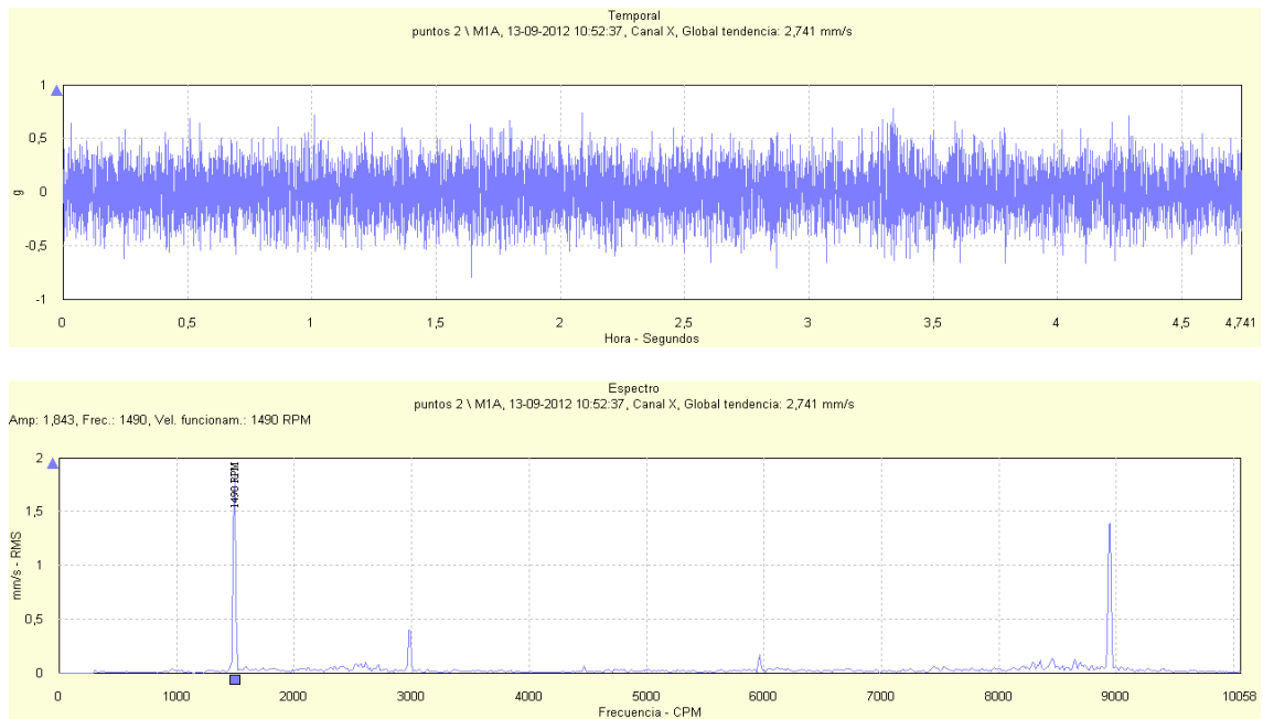
Figura 120: Señal temporal y espectro de vibración para la dirección axial del ducto de succión de la bomba RABI 6 para un flujo impulsado de 800 m 3 /h
