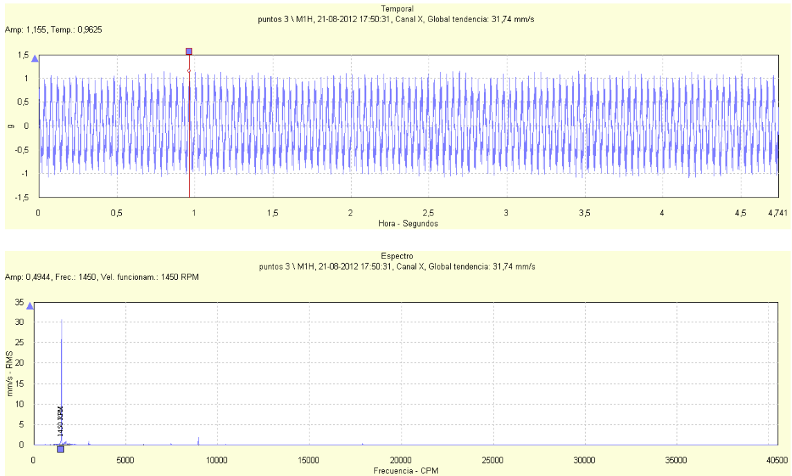
Figura 73: Señal temporal y espectro de vibración para la dirección horizontal del ducto de descarga de la bomba RABI 8 para un flujo impulsado de 988 m 3 /h
