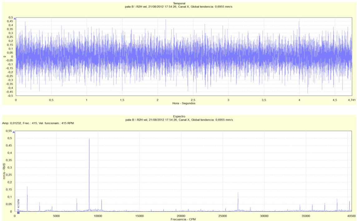
Figura 105: Señal temporal y espectro de vibración para la dirección horizontal de la pata lado descarga de la bomba RABI 8 para un flujo impulsado de 988 m 3 /h
