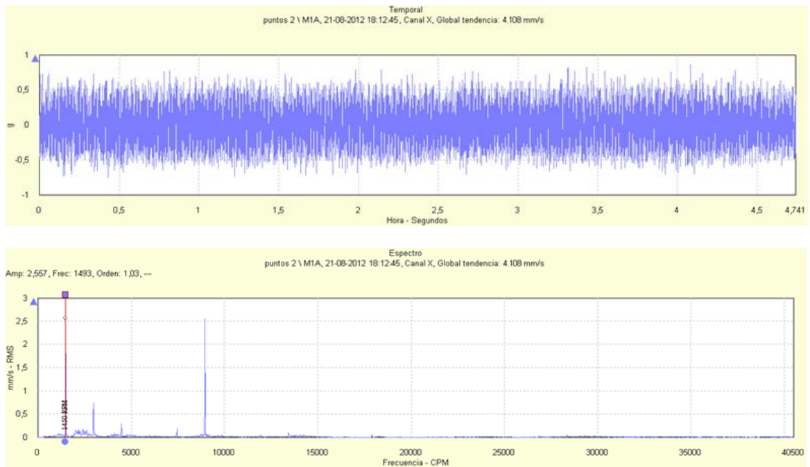
Figura 57: Señal temporal y espectro de vibración para la dirección axial del ducto de succión de la bomba RABI 8 para un flujo impulsado de 610 m 3 /h
