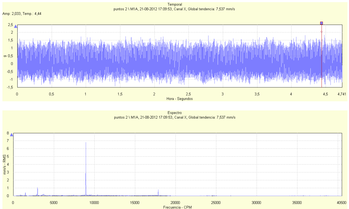
Figura 12: Señal temporal y espectro de vibración para la dirección axial del ducto de succión de la bomba RABI 7 para un flujo impulsado de 1 030 m 3 /h
