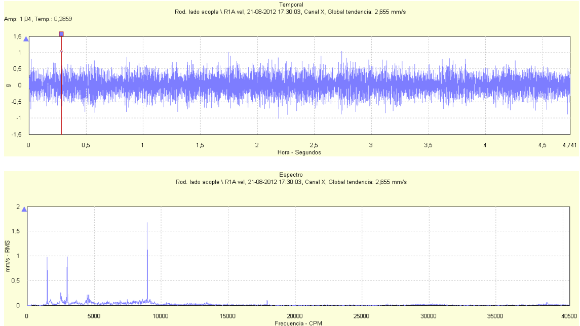
Figura 37: Señal temporal y espectro de vibración para la dirección axial del porta-rodamientos lado acople de la bomba RABI 7 para un flujo impulsado de 770 m 3 /h
