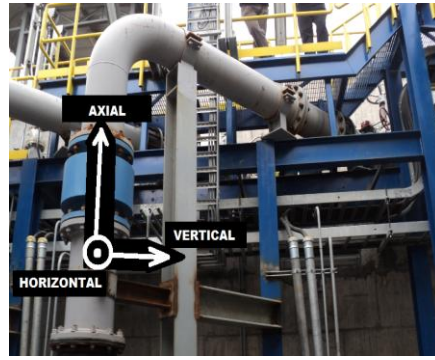
Figura 3, Definición de direcciones y puntos de medición ducto de descarga
