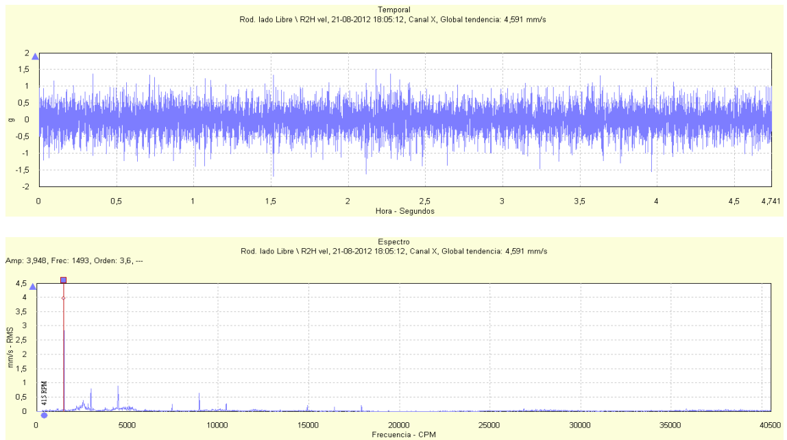
Figura 80: Señal temporal y espectro de vibración para la dirección horizontal del porta-rodamientos lado libre de la bomba RABI 8 para un flujo impulsado de 760 m 3 /h
