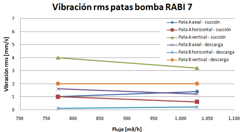
Figura 43, Niveles de vibración rms Patas bomba RABI 7
