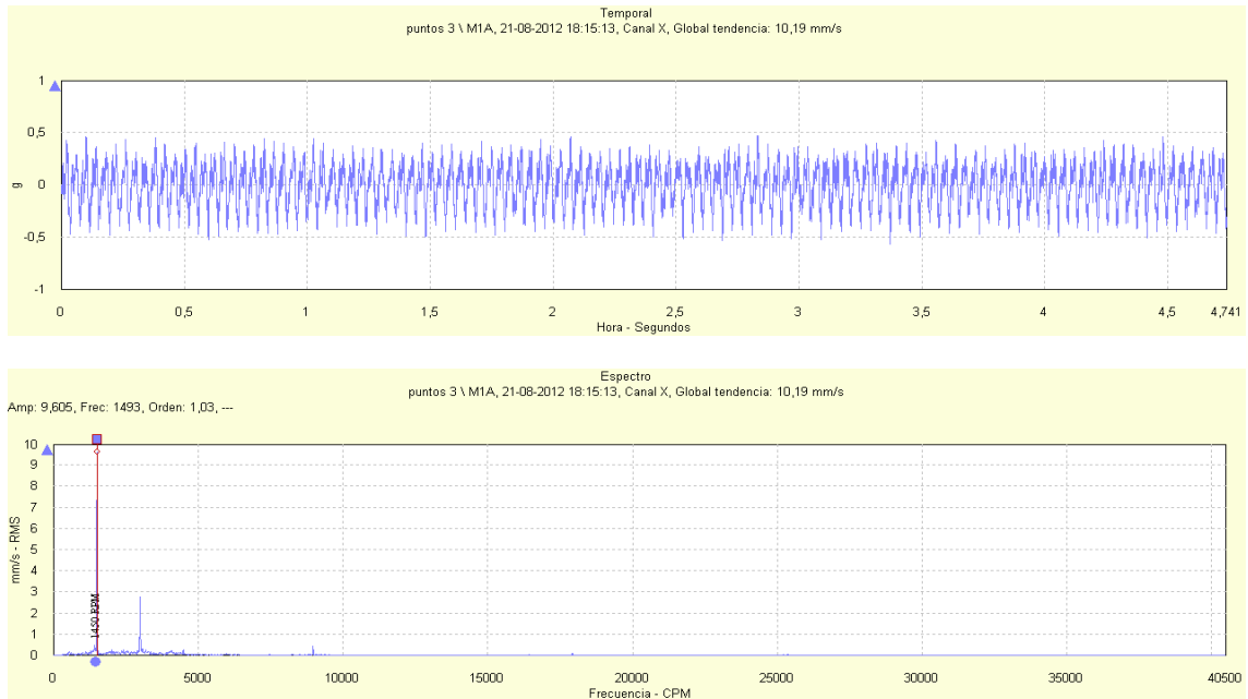
Figura 66: Señal temporal y espectro de vibración para la dirección axial del ducto de descarga de la bomba RABI 8 para un flujo impulsado de 610 m 3 /h
