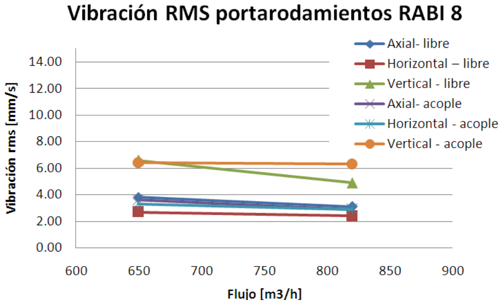
Figura 167, Vibración rms Porta-rodamiento RABI 8, posterior a cambio de bomba.
