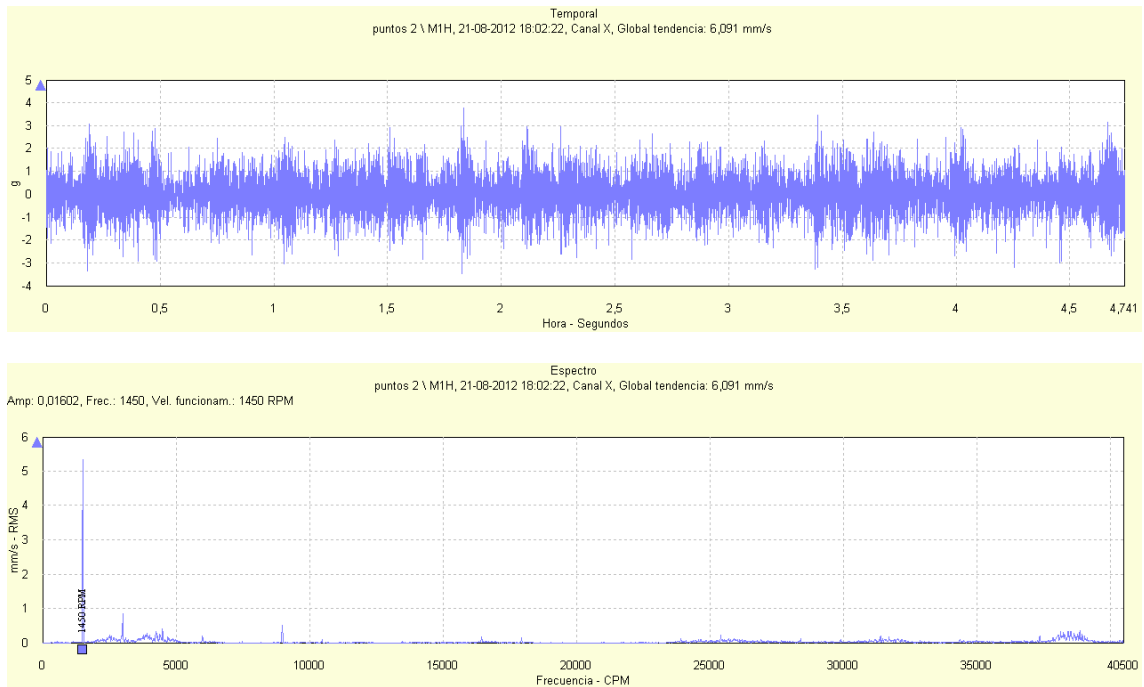
Figura 61: Señal temporal y espectro de vibración para la dirección horizontal del ducto de succión de la bomba RABI 8 para un flujo impulsado de 760 m 3 /h
