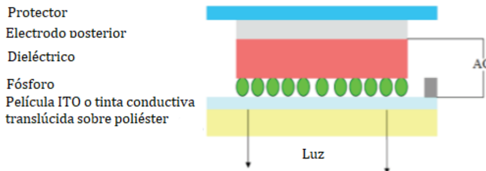
Figura 4: Ejemplo N°1 de secuencia de compilación de una pantalla electroluminiscente Fuente: Kopp & Nixon, 2012
