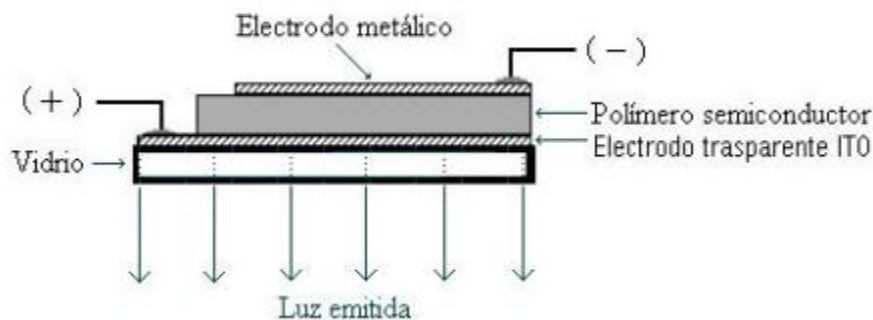
Figura 3: Diagrama esquemático de un dispositivo electroluminiscente
