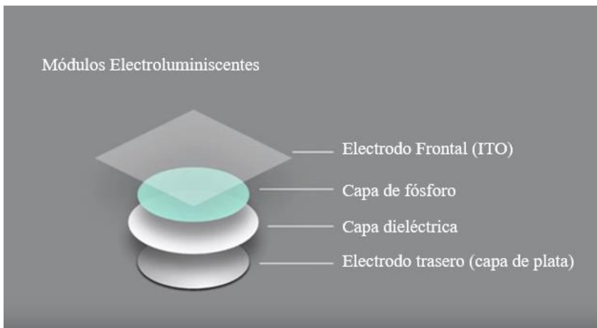
Figura 7: Composición de panel electroluminiscente
