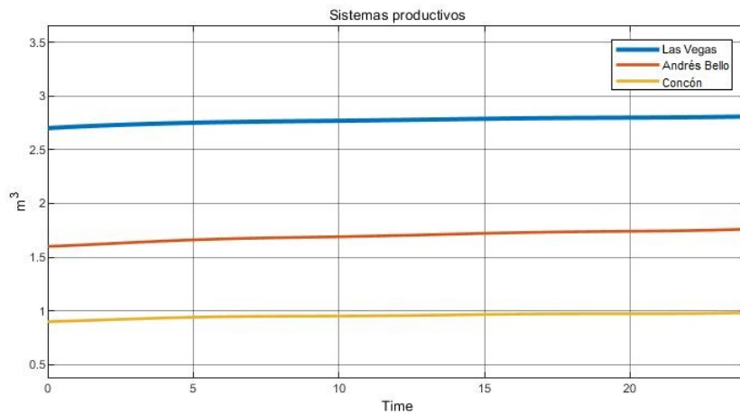
Fig. 5.2: Sistemas productivos en un día de operación
