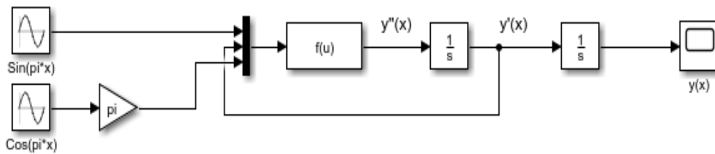
Fig. 2.3: Diagrama de bloques
