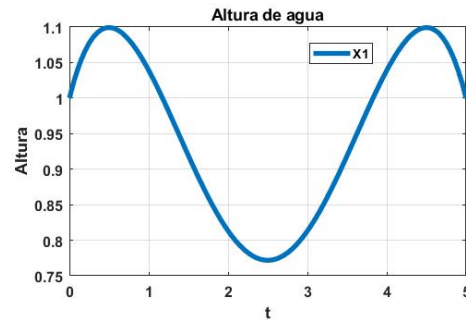
Fig. 2.7: Variación de altura de agua
