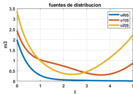
Fig. 3.6: Fuentes de entrada
