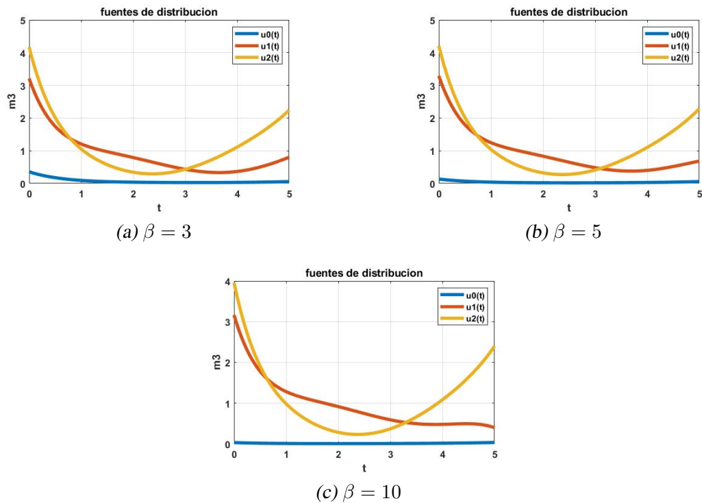
Fig. 3.8: Comportamiento de los caudales con variación de \beta
