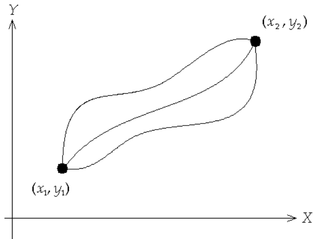
Fig. 2.1: Curvas que pasan por los puntos (x_1, y_1) y (x_2, y_2) en el plano
