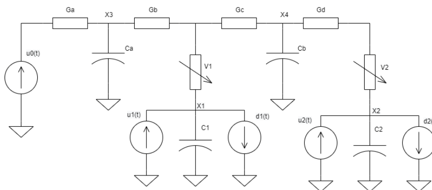
Fig. 3.5: Modelo eléctrico de los estanques
