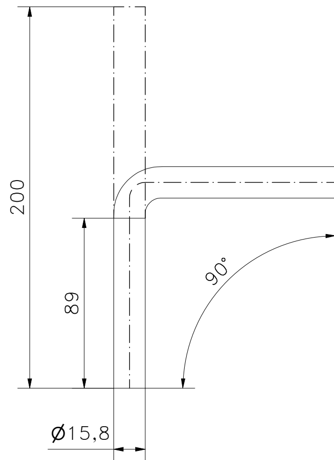
VISTA ALZADO
