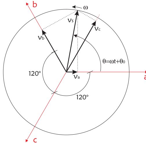
Figura 5.1: Sistema de referencia estático trifásico. Secuencia positiva.
