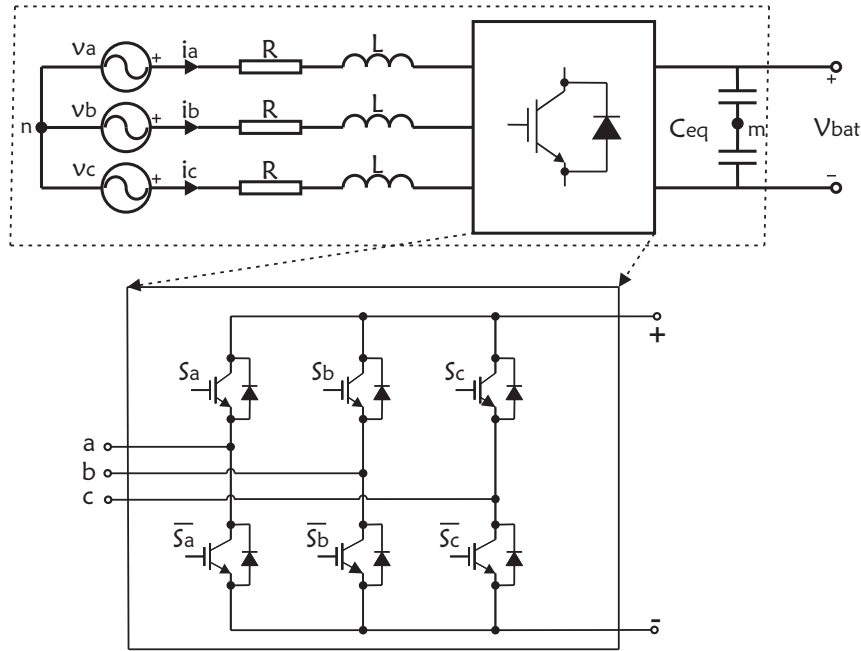
Figura 2.8: Circuito de potencia del rectificador AFE.
