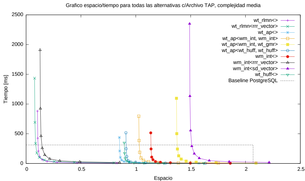
Figura 9: Resultados de espacio v/s tiempo para consultas de complejidad media, utilizando el Archivo TAP como fuente de datos. Las líneas punteadas representan el espacio y tiempo logrados por el baseline.
