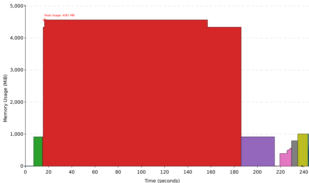
Figura 16: Uso de memoria para la indexación de un archivo de 972 MB, proveniente del Dataset TAP, con un peak de 4.57 GB. Significados de colores, de izquierda a derecha: Par-seo de texto de entrada, construcción SA, construcción BWT, construcción WT, sampleo SA, sampleo ISA.
