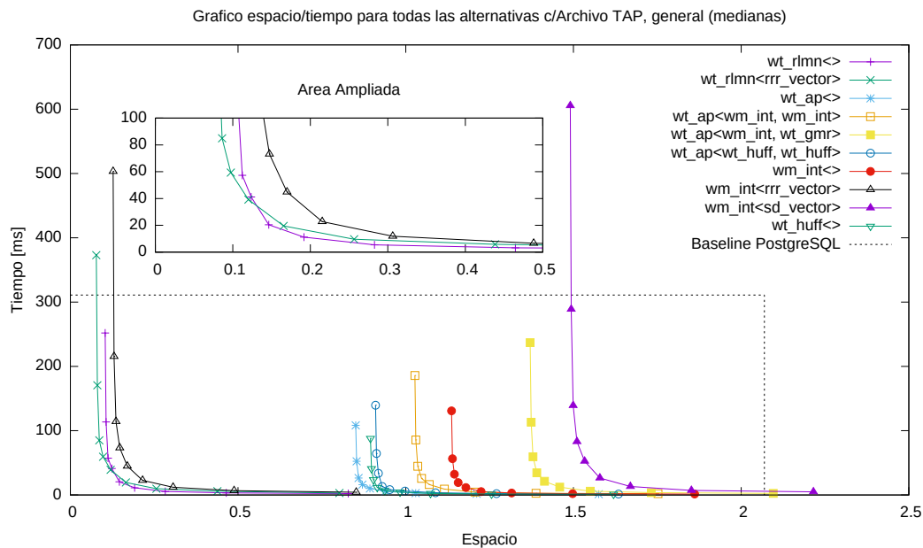
Figura 7: Resultados generales de espacio v/s tiempo para las estructuras probadas, utilizando el Archivo TAP como fuente de datos, y considerando la mediana de los valores de tiempo. Las líneas punteadas representan el espacio y tiempo logrados por el baseline, mientras que el subgráfico dentro de la figura corresponde a un acercamiento en la región de espacio hasta 0.5.
