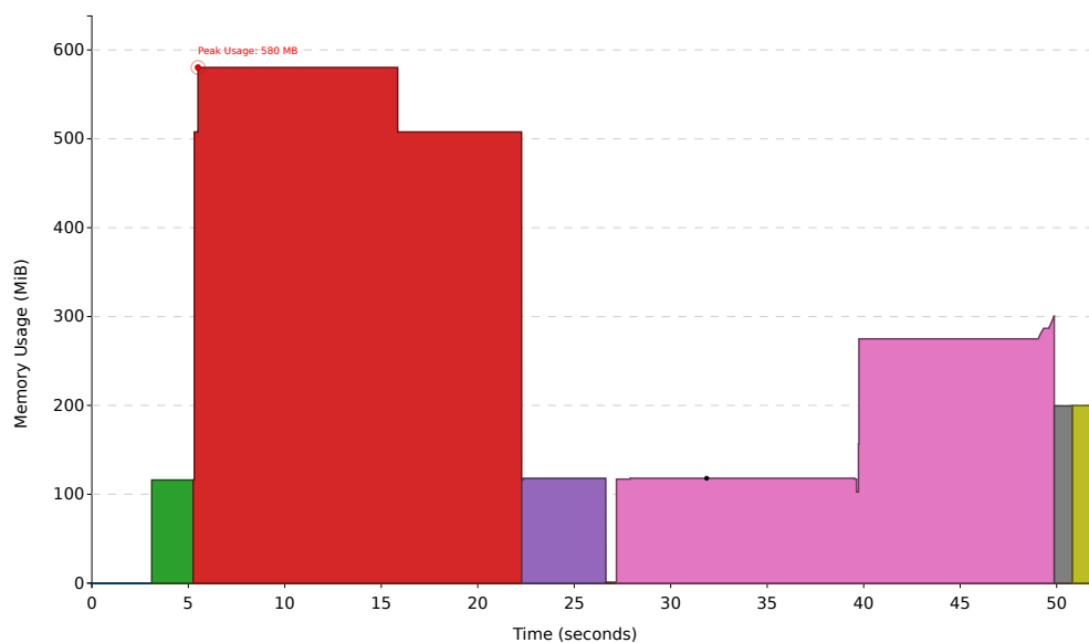
Figura 13: Uso de memoria para la creación de CSA basado en Archivo TAP, utilizando wm_int<sd_vector> y densidad de sampleo 1024, con un peak de 580MB. Significados de colores, de izquierda a derecha: Parseo de texto de entrada, construcción SA, construcción BWT, construcción WT, sampleo SA, sampleo ISA.
