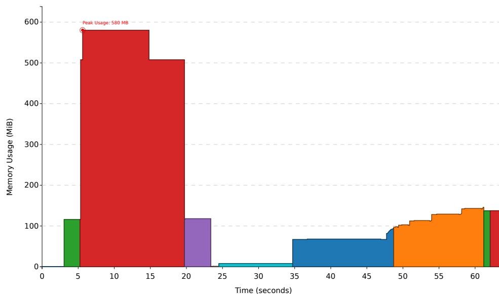
Figura 14: Uso de memoria para la creación de CSA basado en Archivo TAP, utilizando wt_ap<wm_int,wm_int> y densidad de sampleo 2048, con un peak de 580MB. Significados de colores, de izquierda a derecha: Parseo de texto de entrada, construcción SA, construcción BWT, construcción WT, class WT, offset WT's, sampleo SA, sampleo ISA.
