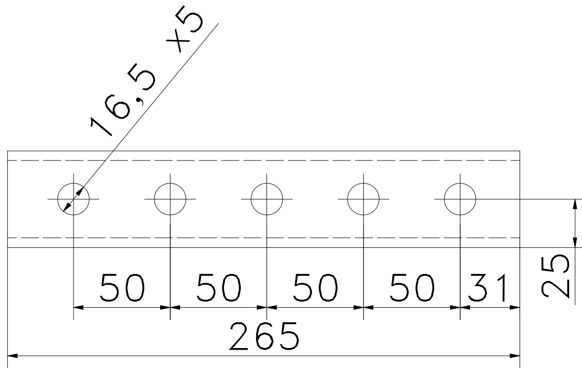
VISTA ALZADO
