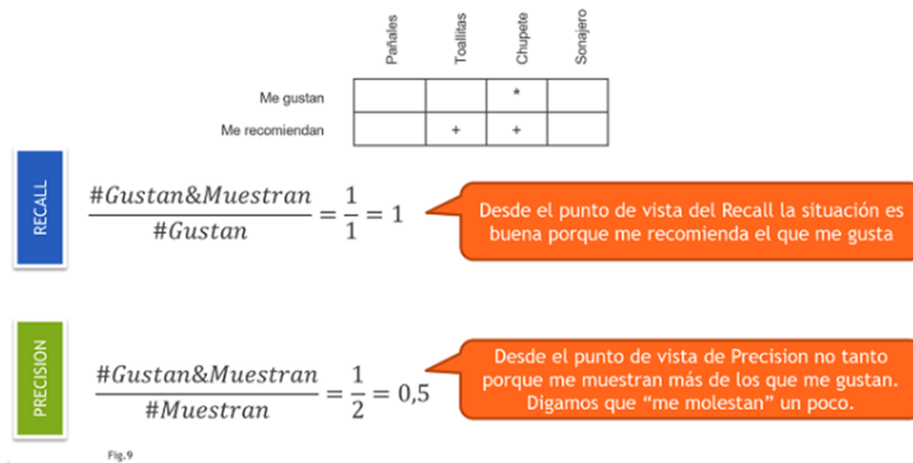
Figura 4.6: Ejemplo del cálculo para Recall y Precisión.
