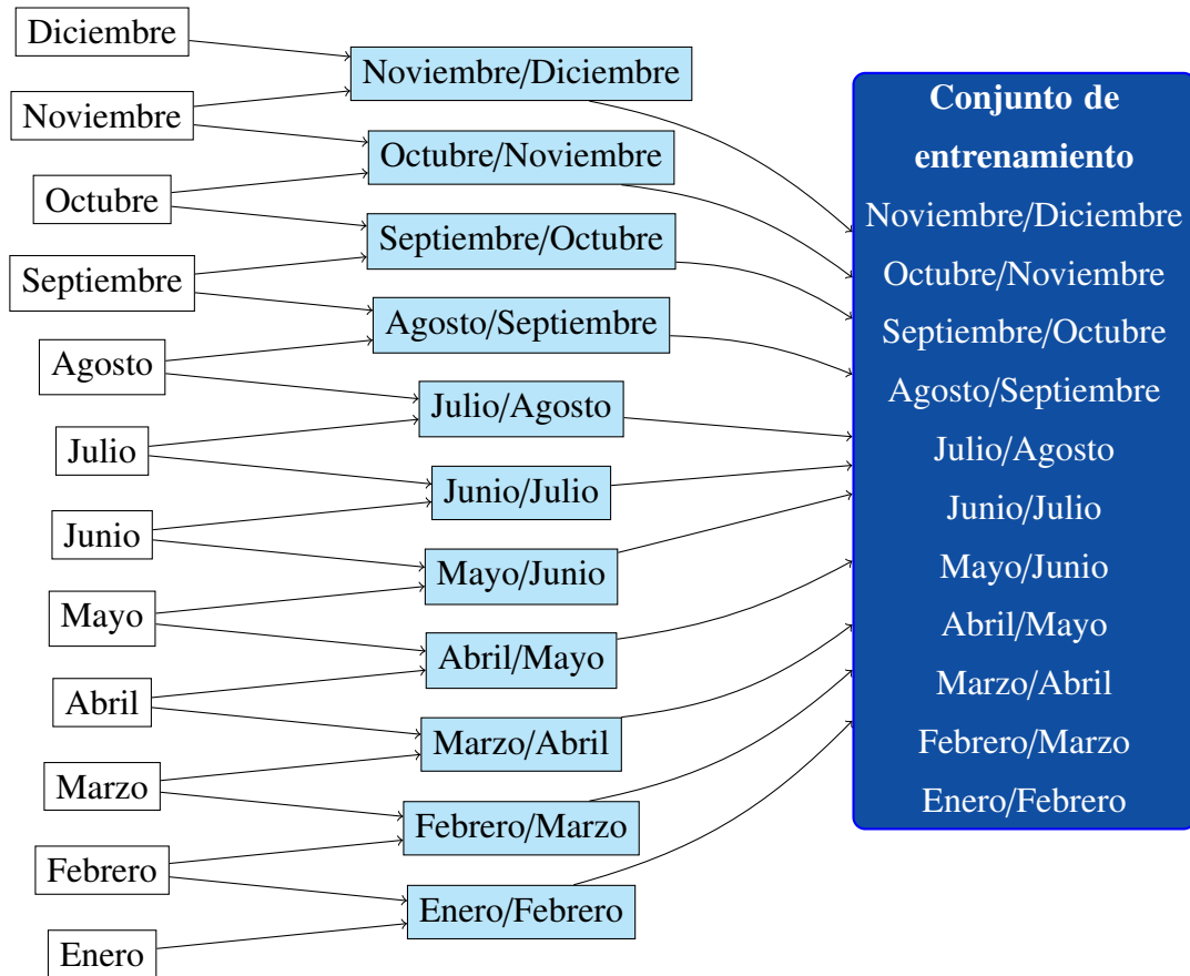
Figura 3.11: Representación del proceso de creación del conjunto de entrenamiento.
