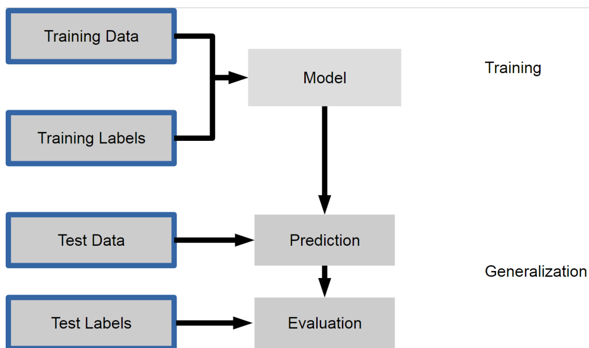
Figura 3.12: El API de un estimador de scikit-learn.
