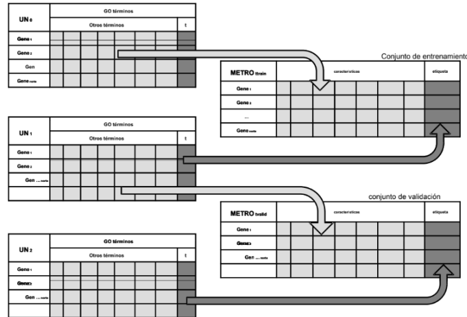
Figura 2.4: Diagrama ilustrativo de la representación de un conjunto de datos de entrenamiento y validación.
