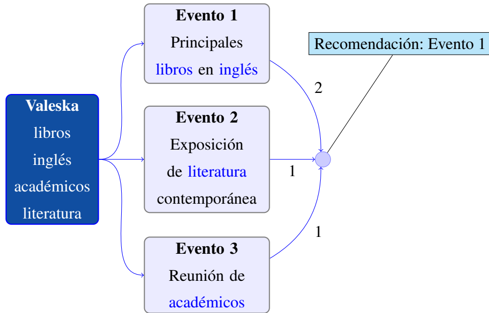
Figura 2.2: Funcionamiento de un Sistema Recomendador Basado en Contenido. Fuente: Elaboración Propia.
