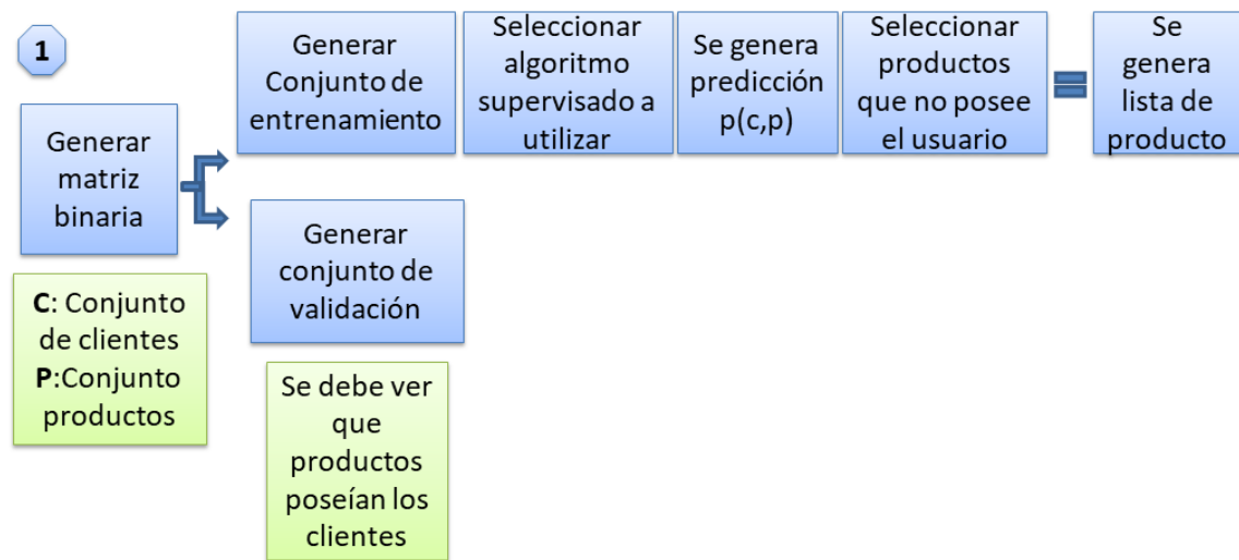
Figura 3.13: Pasos generalizados para la construcción del segundo método.
