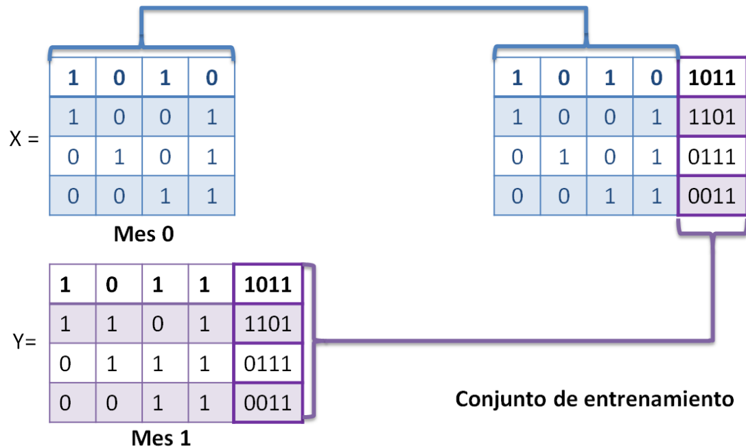
Figura 3.10: Matriz correspondiente al conjunto de entrenamiento.
