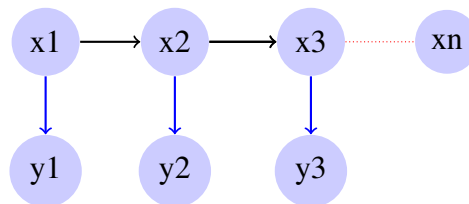
Figura 3.14: Grafo correspondiente a la representación de un modelo simplificado de Markov.
