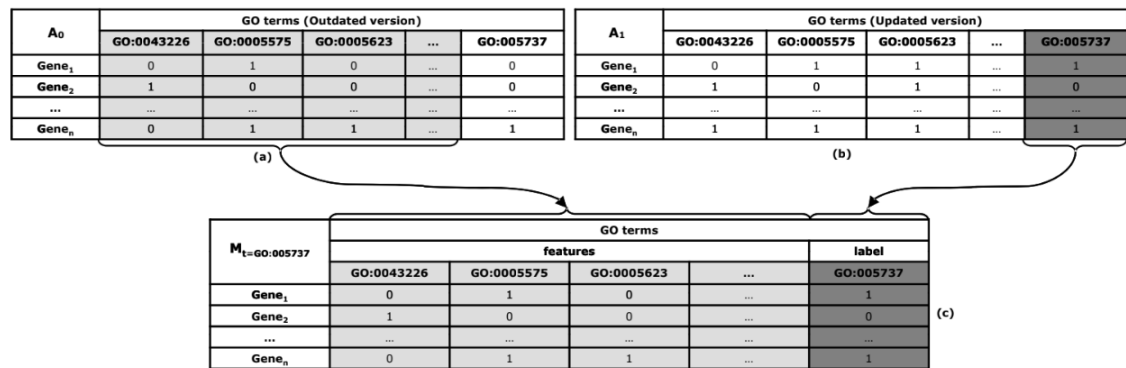
Figura 2.3: Diagrama ilustrativo de la representación de un conjunto de datos para el modelo de predicción de Domeniconi.
