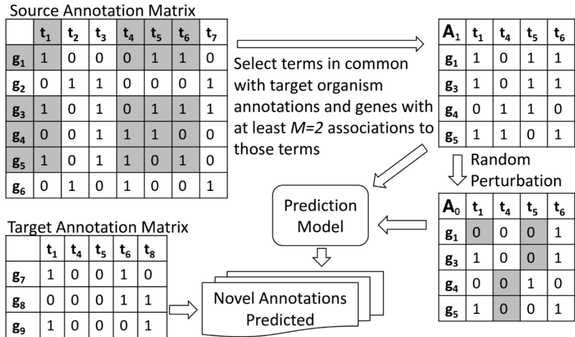
Figura 3.9: Flujo de trabajo para nuevas predicciones de anotación usando para un organismo.
