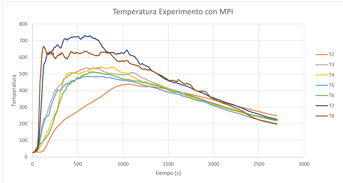
Figura 22: Temperaturas alcanzadas en la cámara de combustión de la estufa BOSCA Spirit 380 a lo largo del tiempo para ensayo de diseño propuesto con MPI
