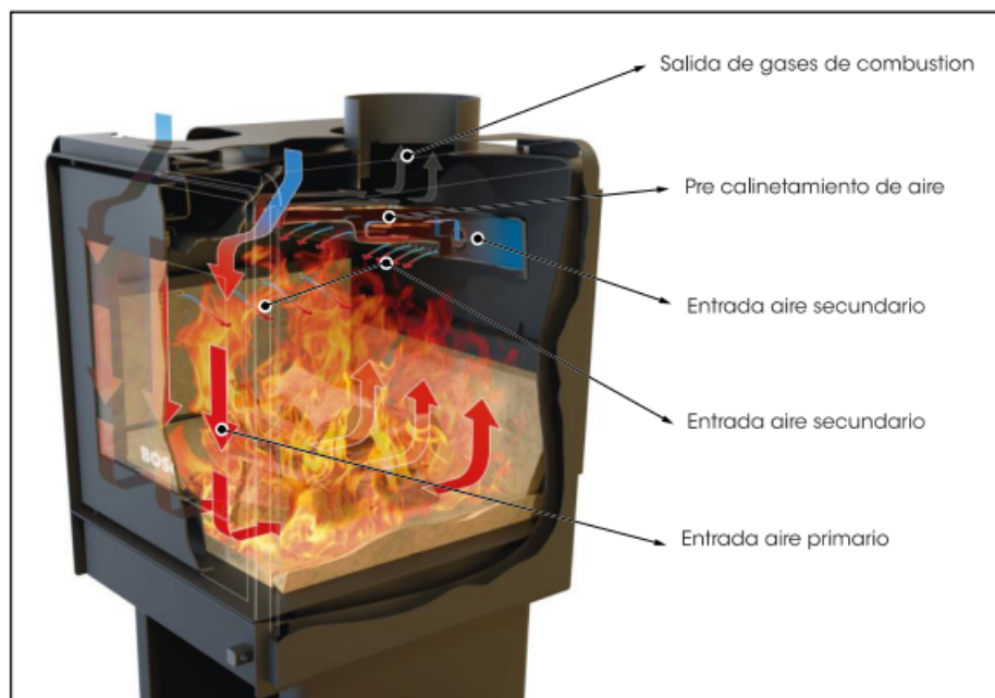
Figura 7: Sistema de funcionamiento de una estufa de combustión doble [25]
