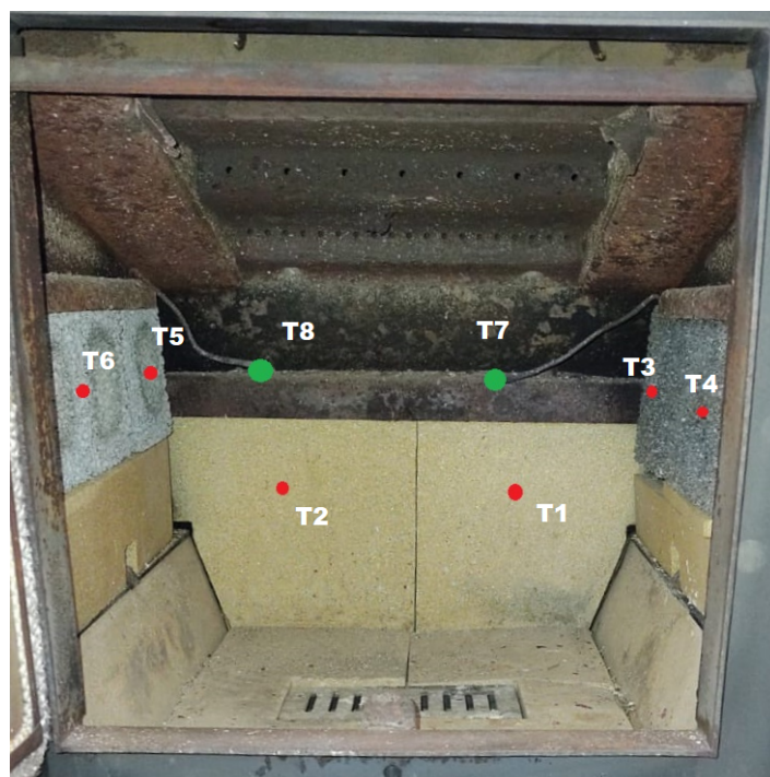
Figura 19: Disposición termocuplas para ensayo con MPI
