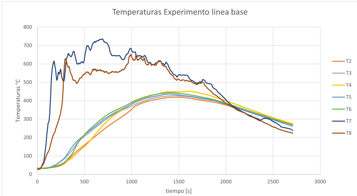
Figura 21: Temperaturas alcanzadas en la cámara de combustión de la estufa BOSCA Spirit 380 a lo largo del tiempo para ensayo de Línea base
