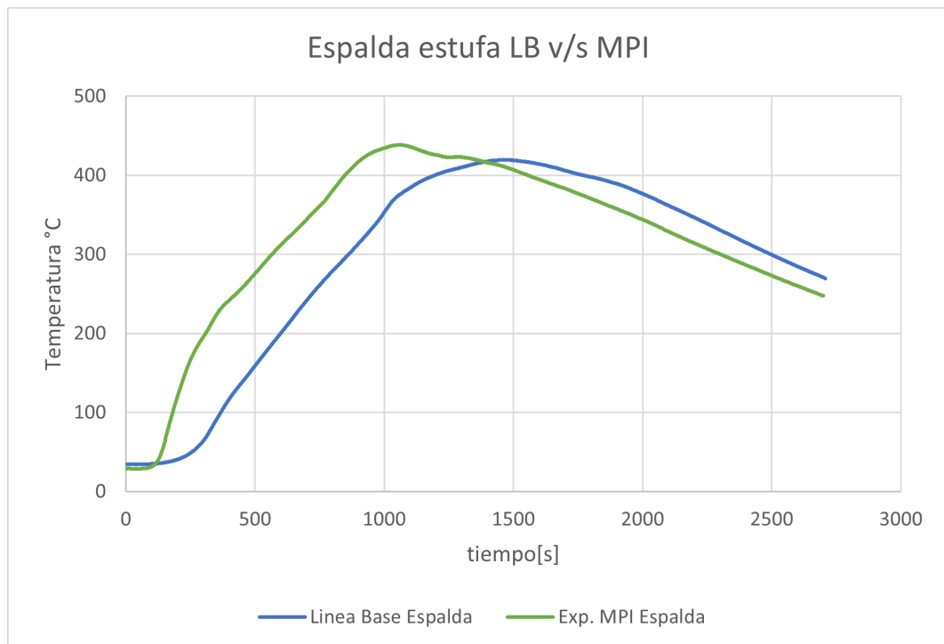
Figura 32: Diferencias entre los promedios de pared trasera obtenidos en experimentos de linea base y medio poroso
