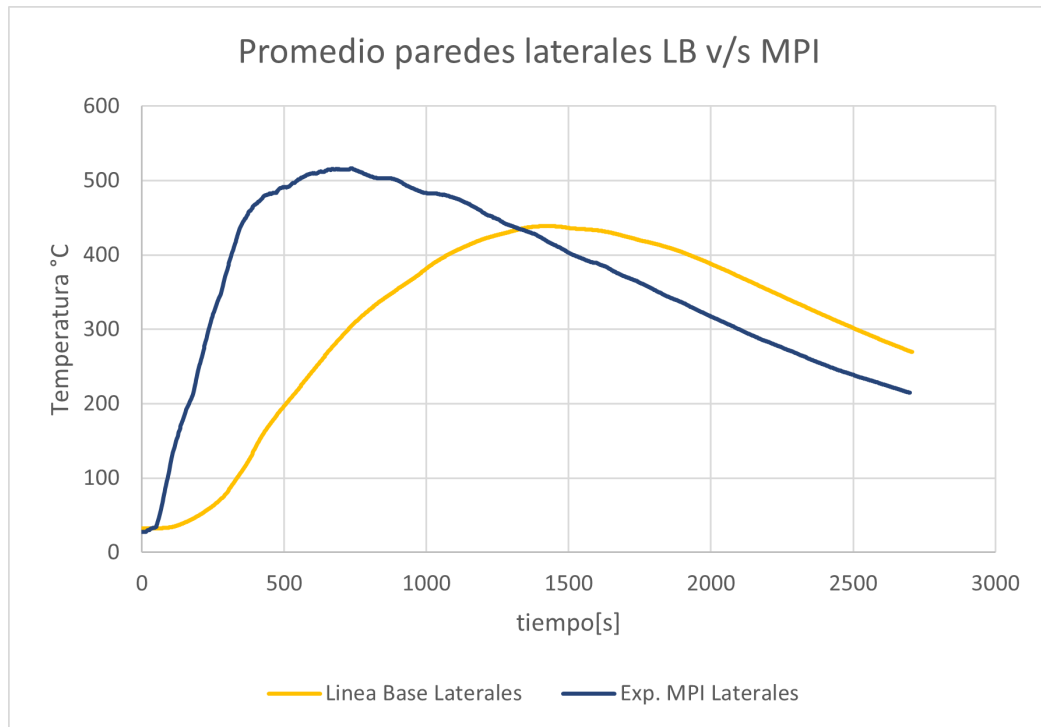
Figura 31: Diferencias entre los promedios de paredes laterales obtenidas en experimentos de linea base y medio poroso
