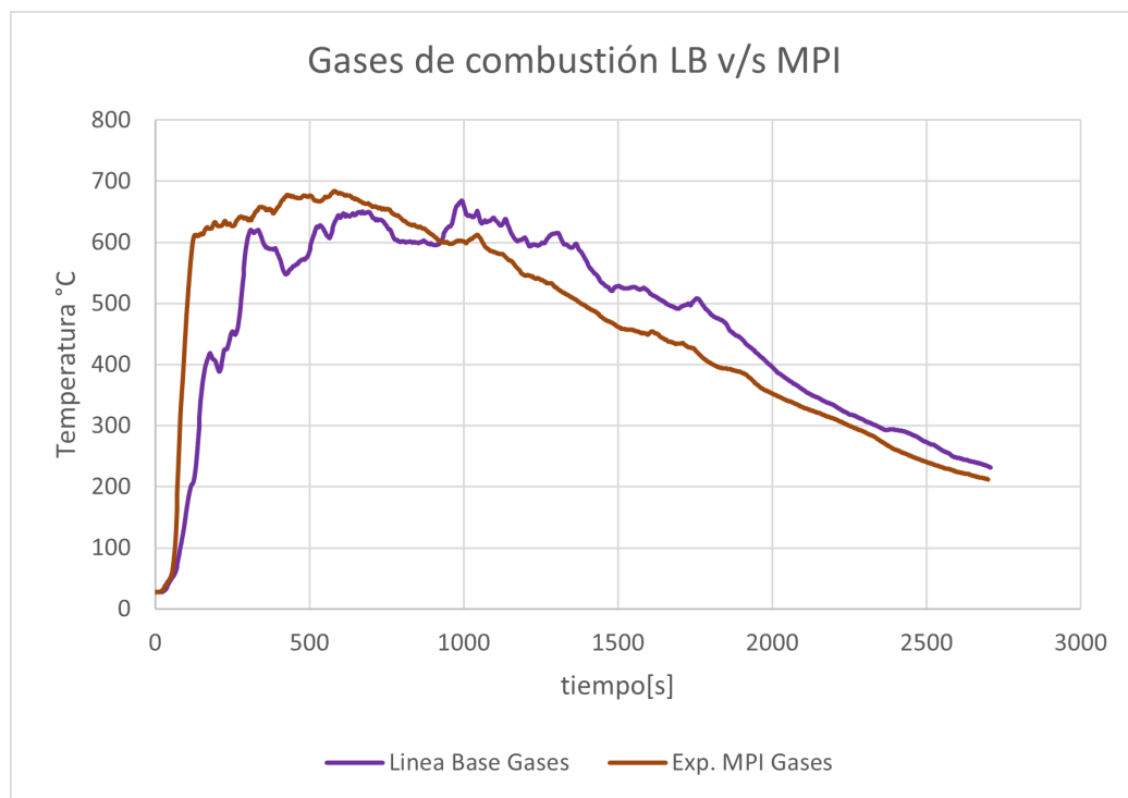
Figura 30: Diferencias entre los promedios de gases obtenidos en experimentos de linea base y medio poroso
