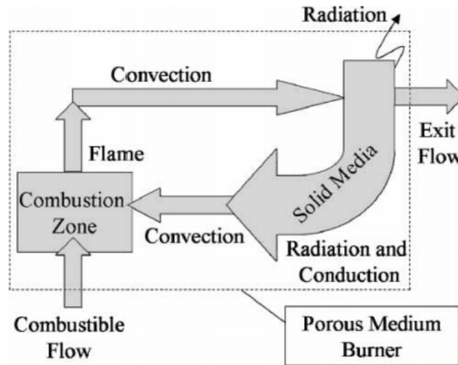
Figura 9: Teoría de llama con exceso de entalpía [17]
