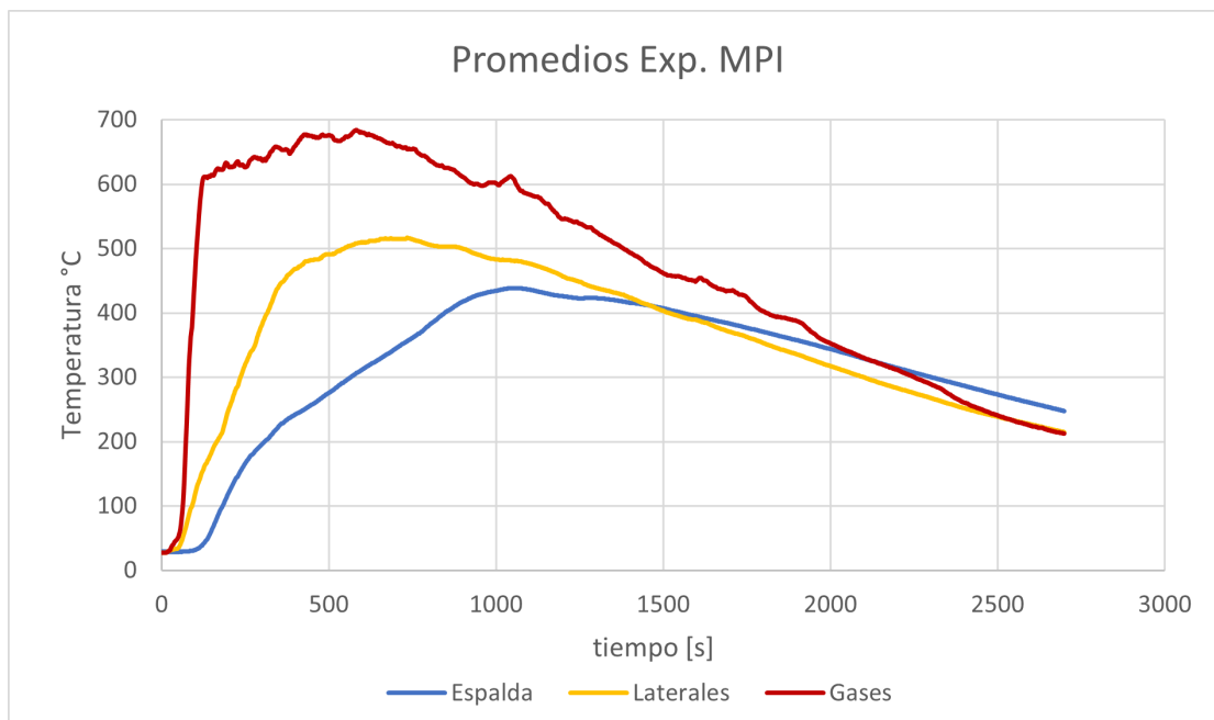
Figura 24: Promedios de temperaturas para diseño propuesto
