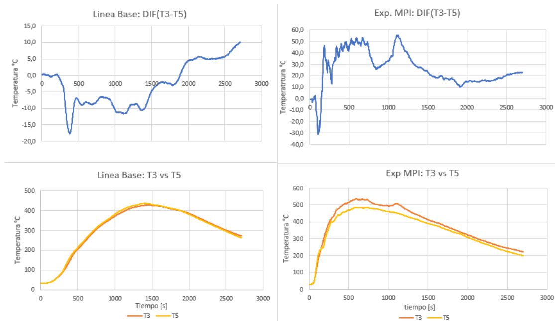
Figura 26: Diferencias de temperaturas entre termocupla frontal para T3 y T5
