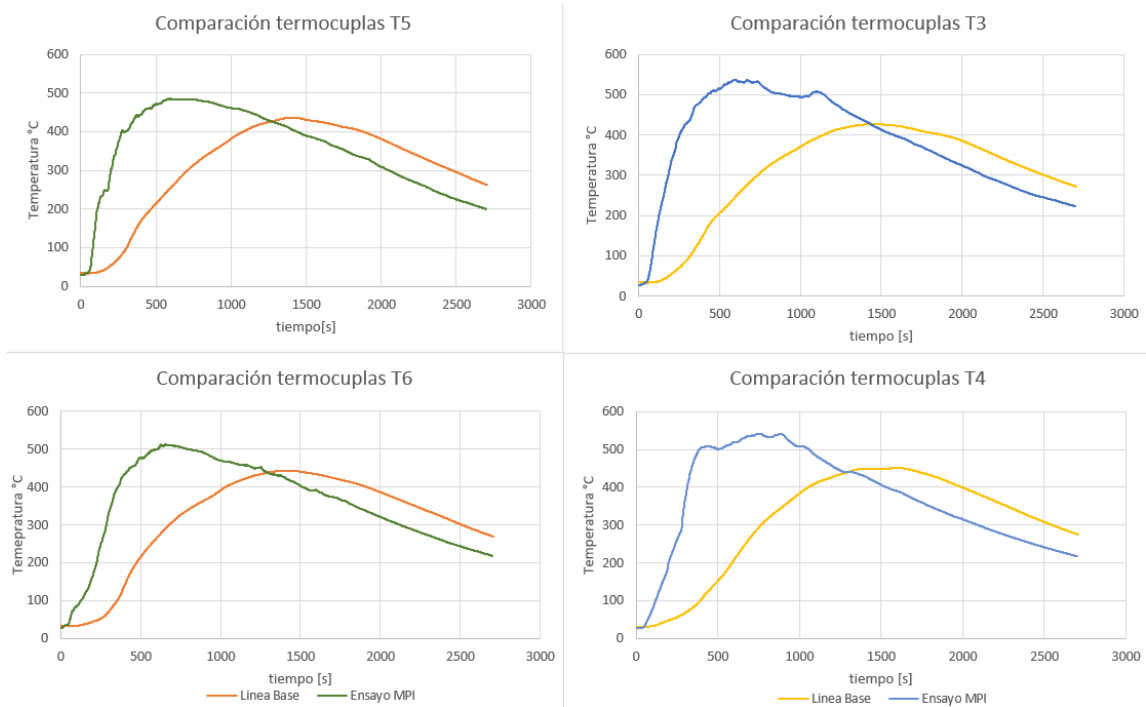
Figura 25: Comparación termocuplas de pared laterales dentro de la estufa, diferenciando entre linea base y ensayo con medio poroso inerte
