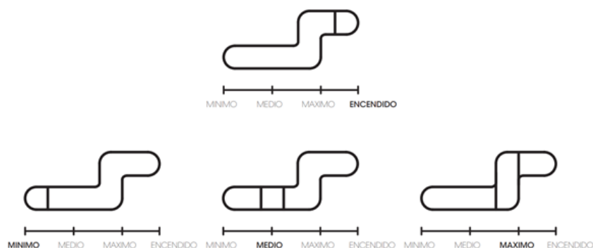
Figura 20: Niveles de regulación de aire primario que posee la estufa BOSCA Spirit 380
