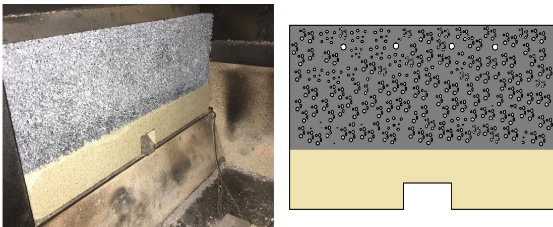
Figura 16: Fotografía y esquema de pared lateral del conjunto vermiculita y medio poroso al interior de la cámara de combustión
