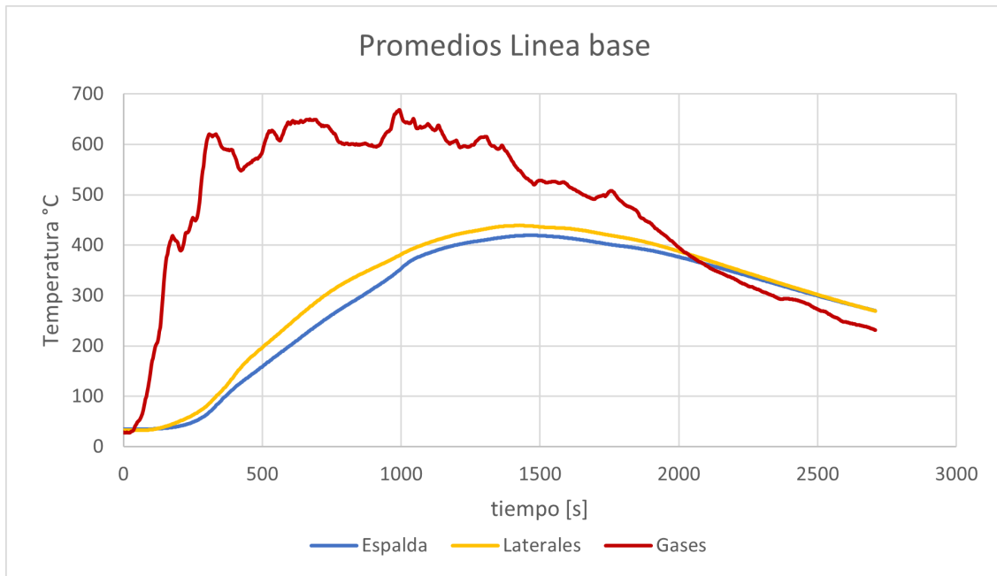
Figura 23: Promedios de termocuplas para Linea base
