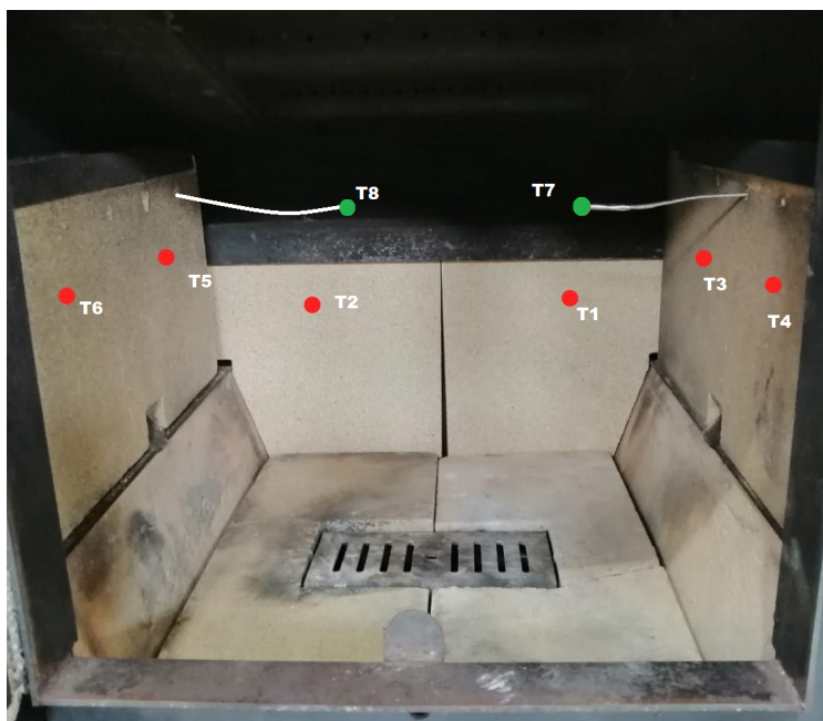
Figura 18: Disposición termocuplas para ensayo linea base
