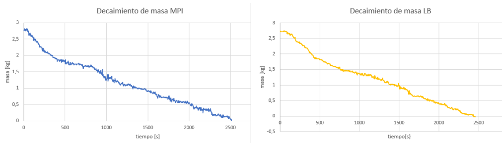
Figura 29: Decaimiento de masa para experimento linea base y prototipo de estufa
