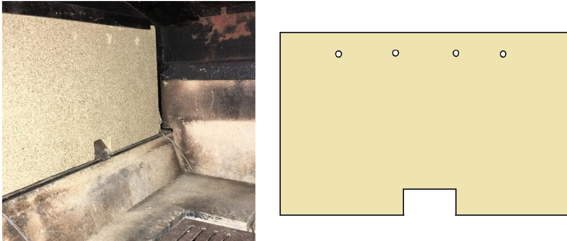
Figura 15: Fotografía y esquema de pared lateral de vermiculita al interior de la cámara de combustión, correspondiente a los ensayos de línea base
