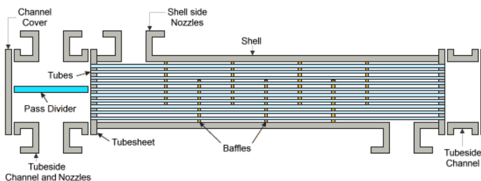
Figura IV.58: Esquema de intercambiador de tubo y carcasa convencional.
