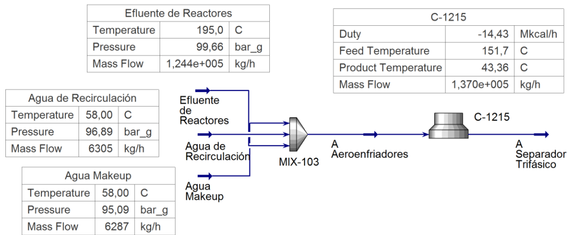
Figura IV.39: Simulación de intercambiadores C-1215 nuevos para carga de 2.548 m 3 /d de gasoil..
