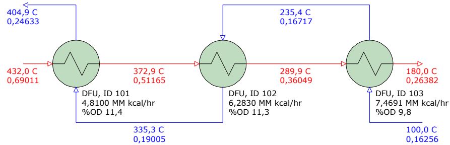
Figura V.8: Rediseño de intercambiador de tubo y carcasa con tubos twisted .
