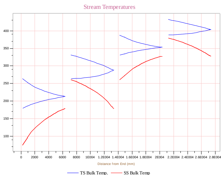
Figura IV.14: Perfil de temperatura de diseño de intercambiadores C-1201.
