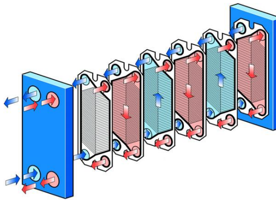
Figura IV.59: Funcionamiento de un intercambiador de placas.
