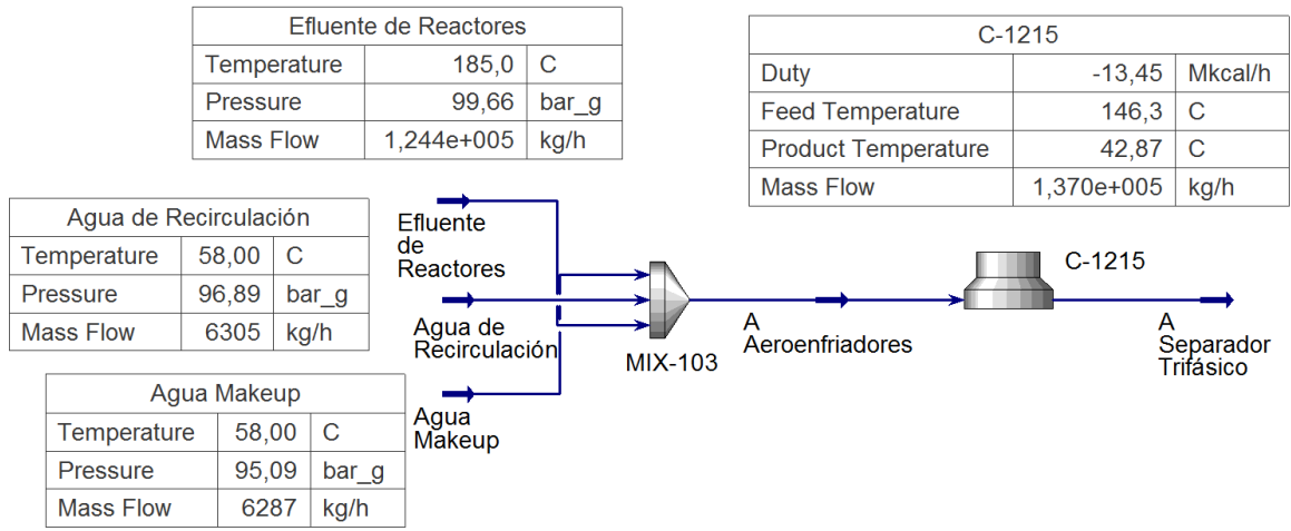
Figura IV.41: Simulación de intercambiadores C-1215 nuevos para carga de 2.548 m 3 /d de gasoil..
