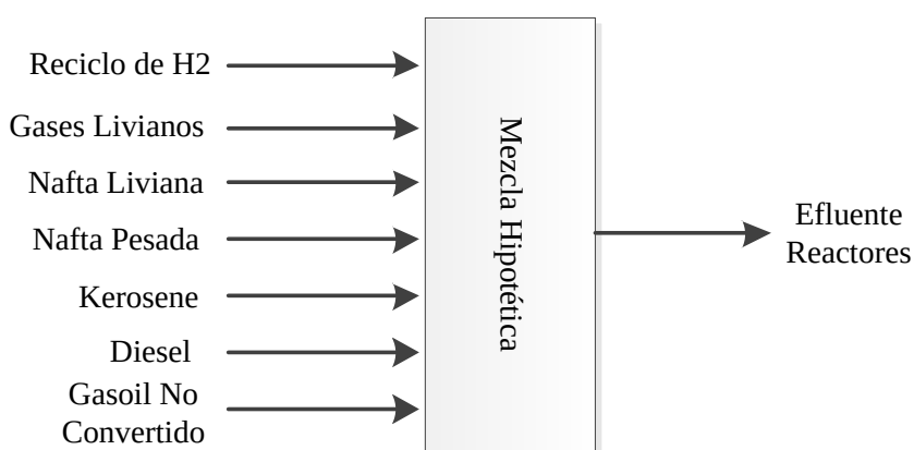
Figura IV.6: Caja negra para balance de masa de efluente de reactor. Fuente: Elaboración propia
