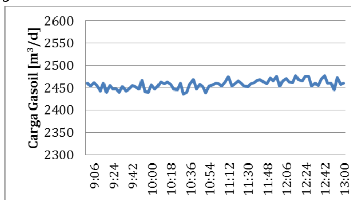
Figura XI.5: Oscilación de carga de Gasoil durante el caso operacional analizado 25/5/16. Fuente: Elaboración propia en base a PI.
