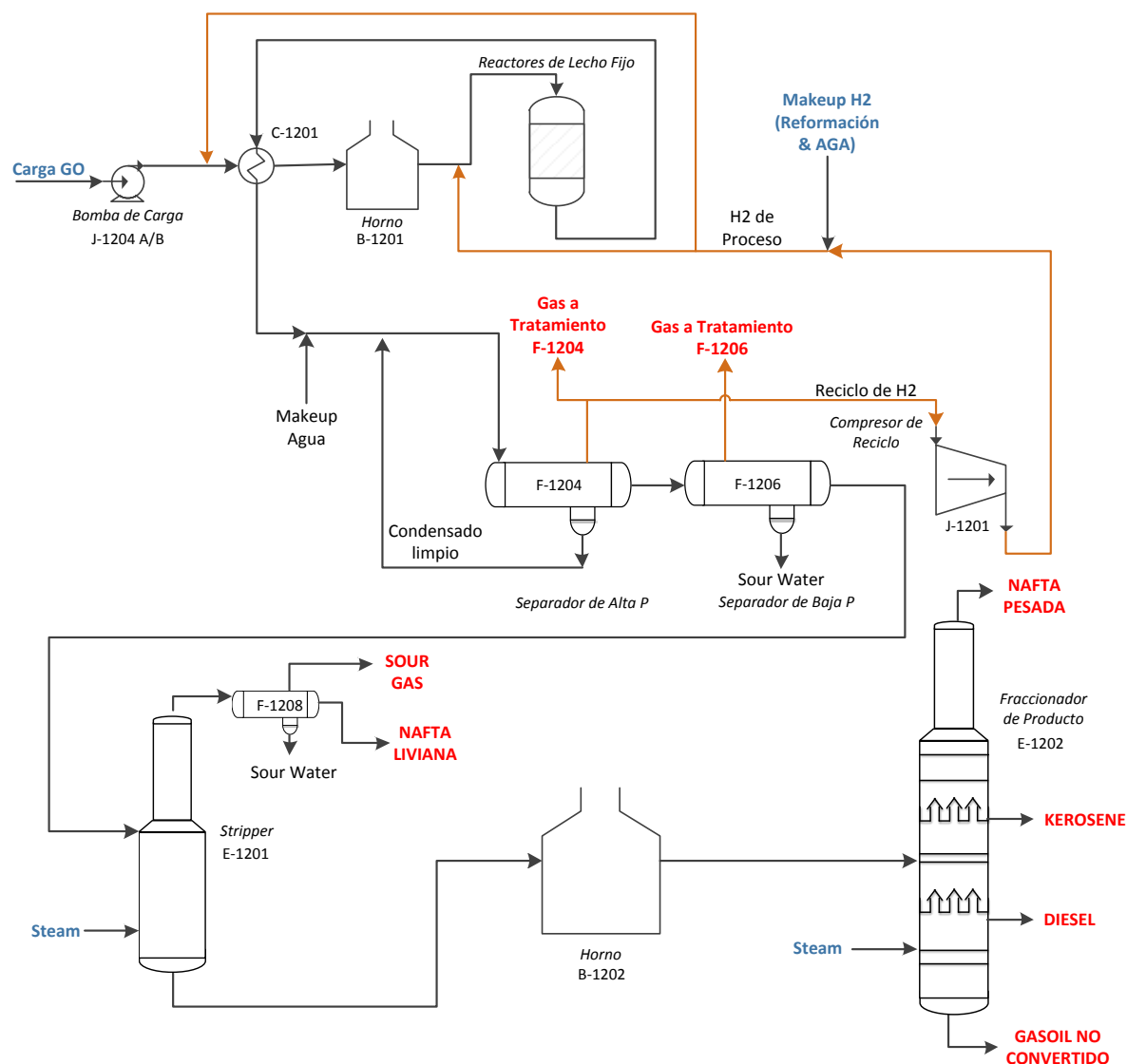
Figura IV.2: Diagrama de planta de Hydrocracking simplificado.
