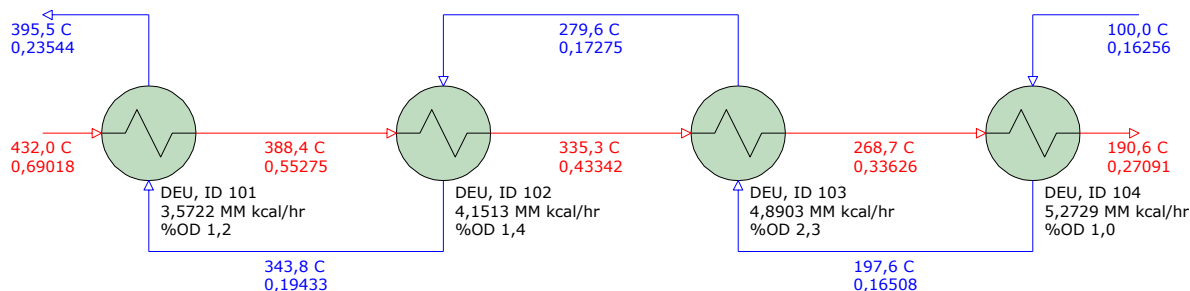
Figura V.4: Diseño de haces tubulares trenzados Koch en HTRI.
