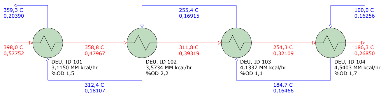
Figura IV.44: Simulación C-1201 limpios en HTRI para carga de 3200 m 3 /d de gasoil.
