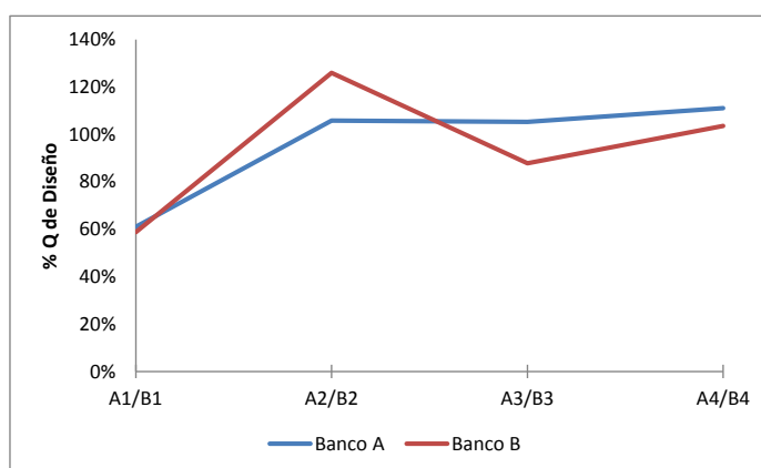
Figura IV.29: Estimación pérdida de intercambio de energía.
