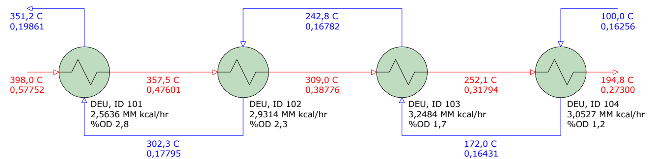
Figura IV.34: Simulación C-1201 sucios en HTRI.
