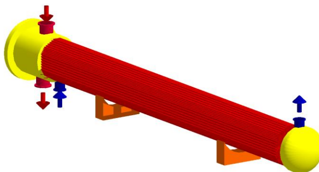
Figura V.5: Esquema del diseño obtenido para recambio de haces tubulares por tubos twisted .
