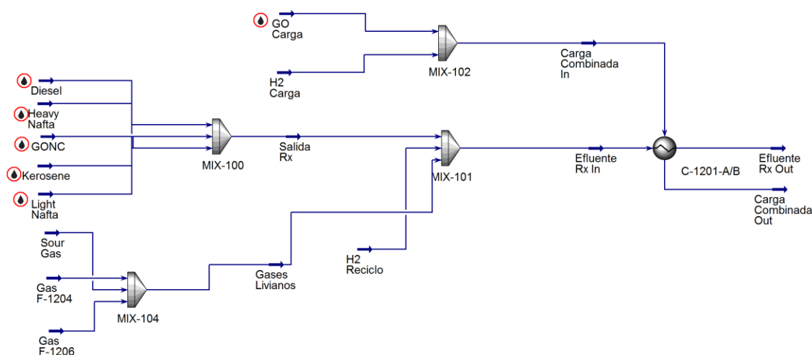
Figura IV.16: Esquema de la simulación realizada.
