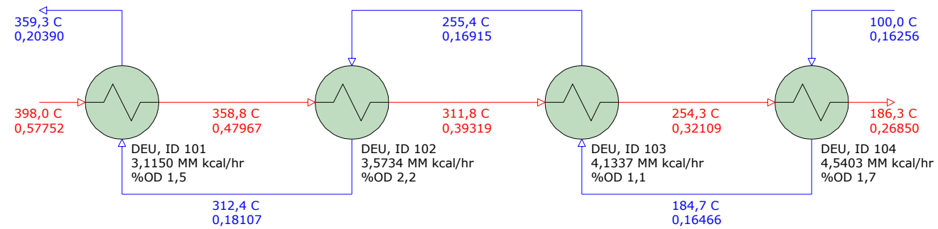
Figura IV.48: Simulación C-1201 limpios en HTRI para carga de 3200 m 3 /d de gasoil.
