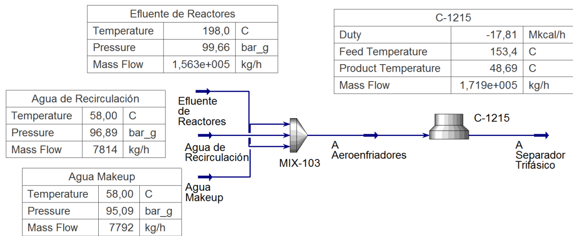
Figura IV.47: Simulación de intercambiadores C-1215 nuevos para carga de 3200 m 3 /d de gasoil..
