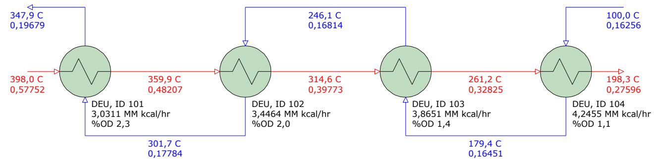
Figura IV.42: Simulación C-1201 sucios en HTRI para carga de 3200 m 3 /d de gasoil..
