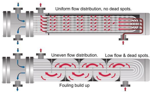
Figura IV.55: Distribución del fluido de la carcasa para un intercambiador de calor con haz de tubos trenzados.
