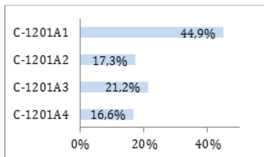
Figura V.1: Distribución del ensuciamiento tren C-1201A
