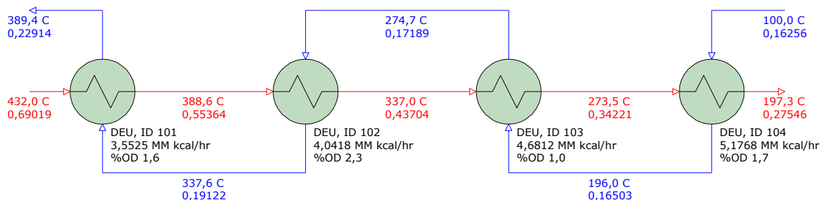
Figura IV.52: Simulación de los intercambiadores C-1201 limpios.
