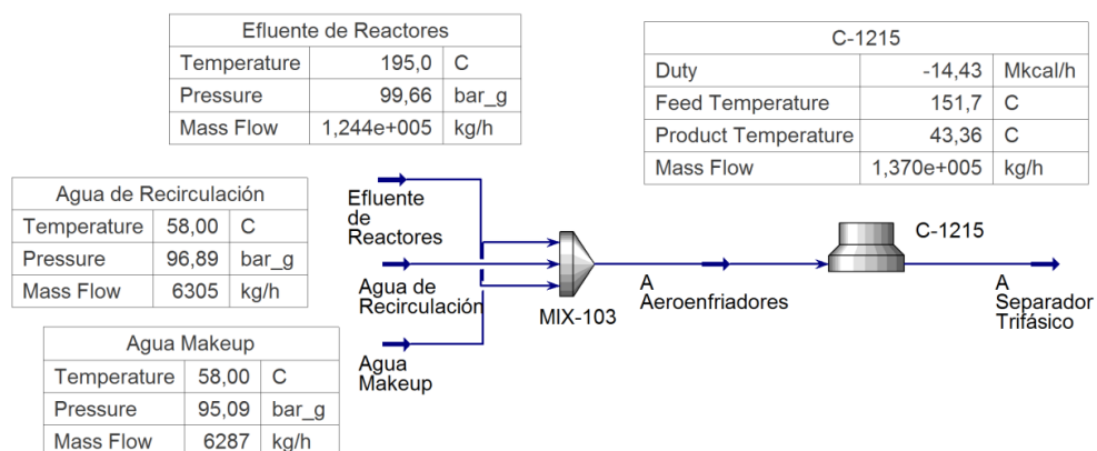
Figura IV.22: Simulación de operación C-1215 en escenario futuro (optimista).
