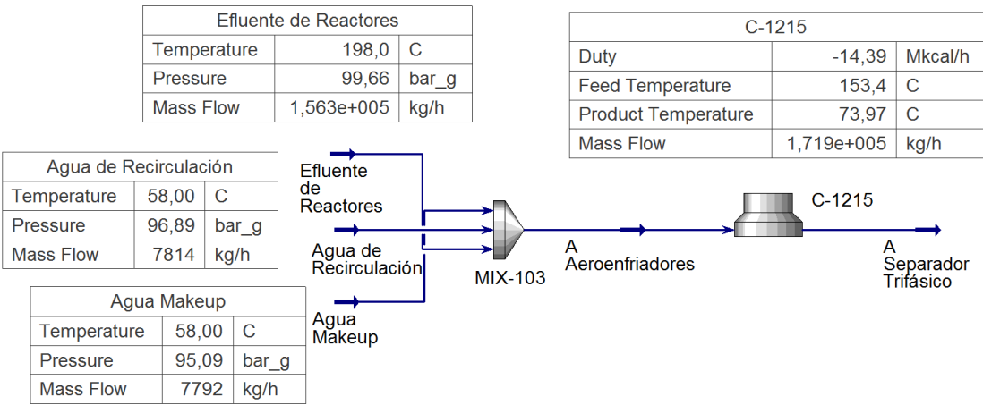
Figura IV.43: Simulación de intercambiadores C-1215 actuales para carga de 3200 m 3 /d de gasoil..
