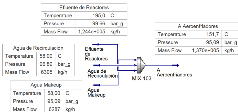
Figura IV.17: Simulación de las corrientes aguas debajo de C-1201.
