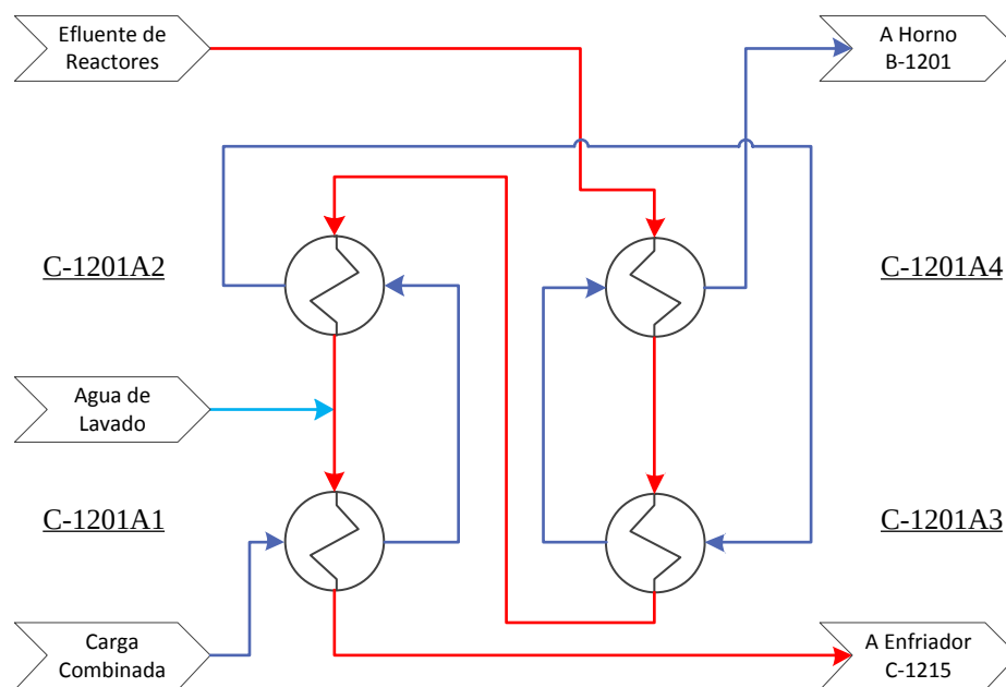
Figura IV.54: Esquema de inyección de agua como mejora del proceso en Banco A.
