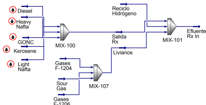
Figura IV.8: Mezclado de corrientes en Hysys para simulación de efluente de reactores.
