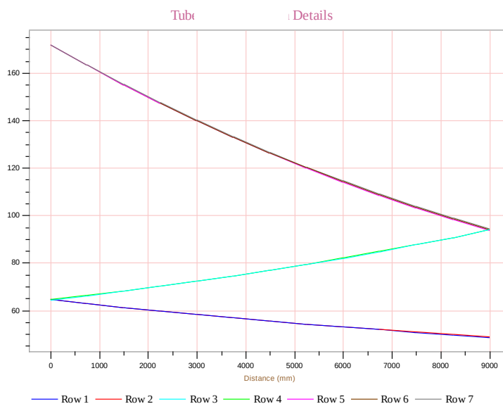
Figura IV.15: Perfil de temperatura de diseño C-1215
