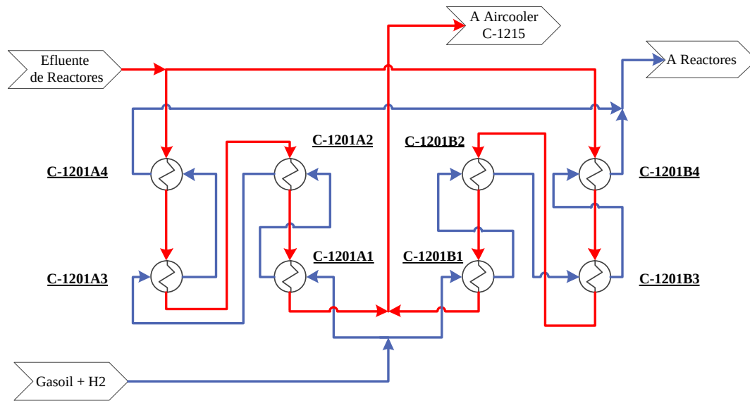
Figura IV.12: Disposición de los intercambiadores de carga combinada C-1201A y C-1201B.
