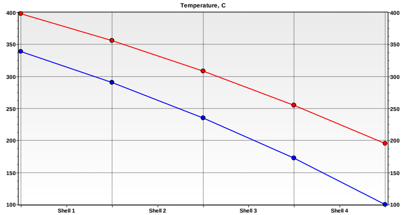
Figura IV.26: Perfil de temperatura de los intercambiadores C-1201 con ensuciamiento. Fuente: Elaboración propia en base a simulación en HTRI.
