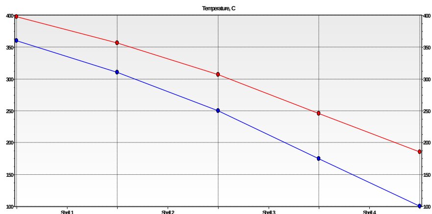
Figura IV.21: Perfil de temperatura de intercambiadores de calor C-1201 en condiciones de operación para desempeño por diseño.
