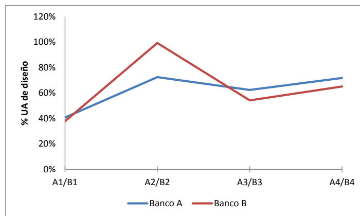
Figura IV.28: Estimación pérdida de capacidad de transferencia de calor.
