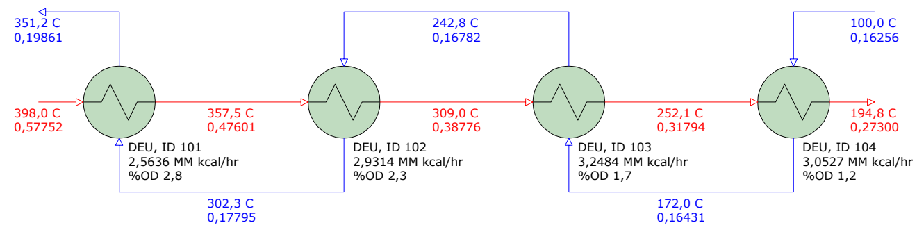
Figura IV.38: Simulación C-1201 sucios en HTRI para carga de 2.548 m 3 /d de gasoil..
