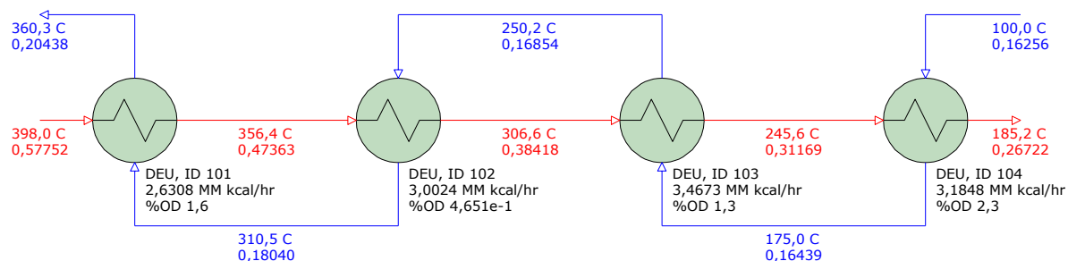
Figura IV.20: Simulación de la operación actual por diseño de C-1201.
