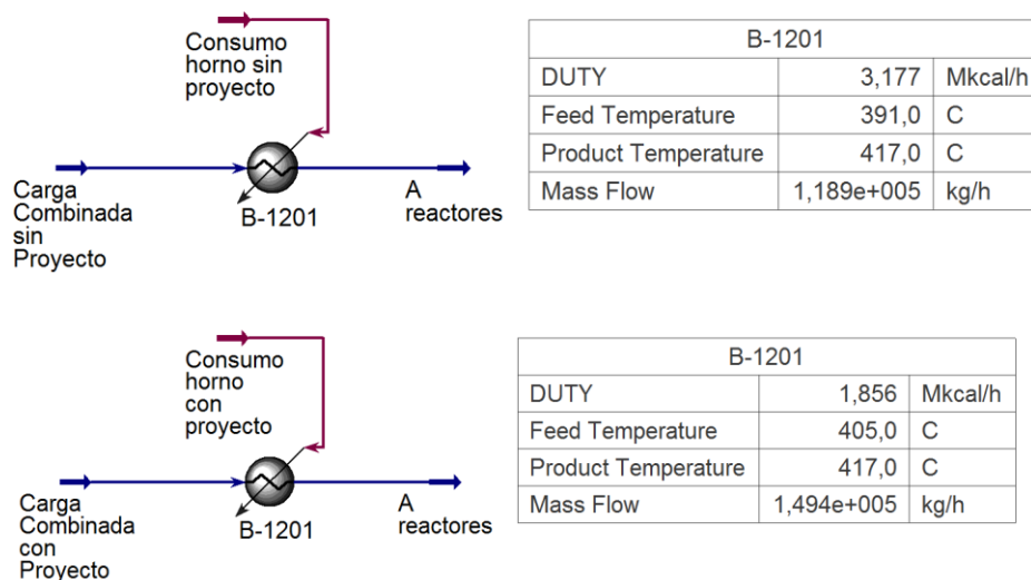
Figura VIII.2: Comparación del consumo energético del horno B-1201 sin proyecto y con proyecto
