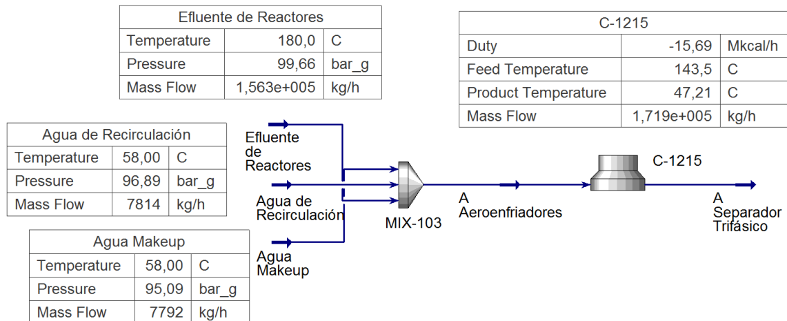
Figura IV.50: Simulación para la obtención de la temperatura de diseño de salida del efluente de reactores de los intercambiadores C-1201.
