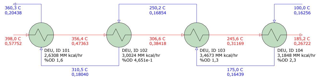
Figura IV.40: Simulación C-1201 limpios en HTRI para carga de 2.548 m 3 /d de gasoil.
