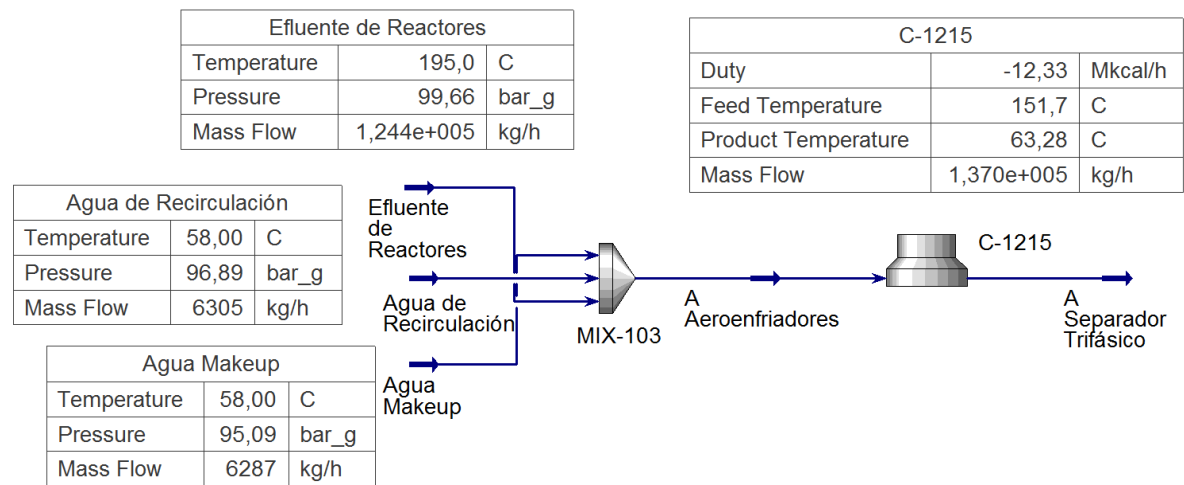
Figura IV.35: Simulación de intercambiadores C-1215 actuales para carga de 2.548 m 3 /d de gasoil.
