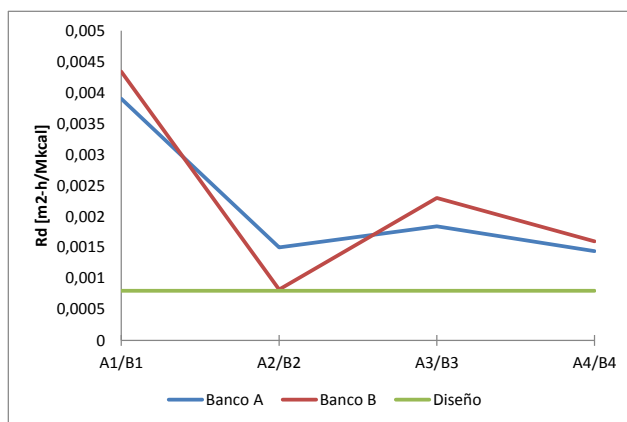
Figura IV.27: Ensuciamiento C-1201
