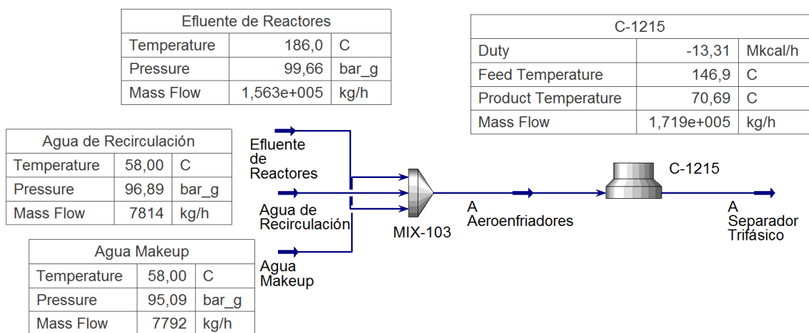
Figura IV.45: Simulación de intercambiadores C-1215 actuales para carga de 3200 m 3 /d de gasoil..
