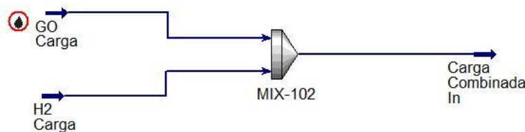
Figura IV.7: Mezclado de corrientes en Hysys para simulación de carga combinada.
