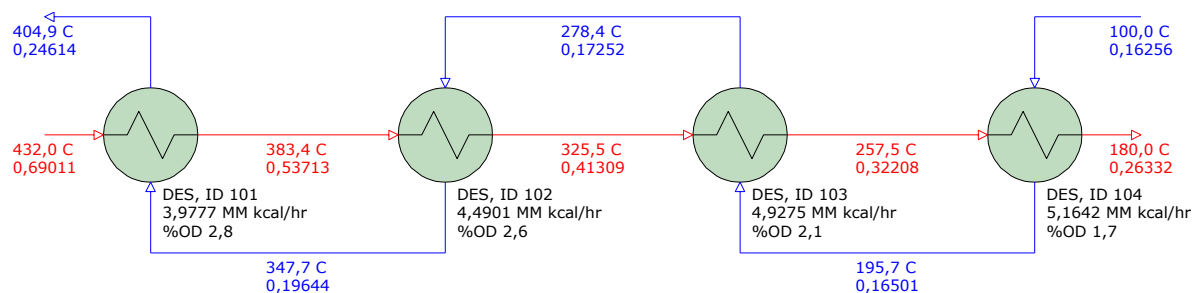
Figura V.6: Rediseño de intercambiador convencional de tubo y carcasa. Fuente: Elaboración propia en base a simulación en HTRI.
