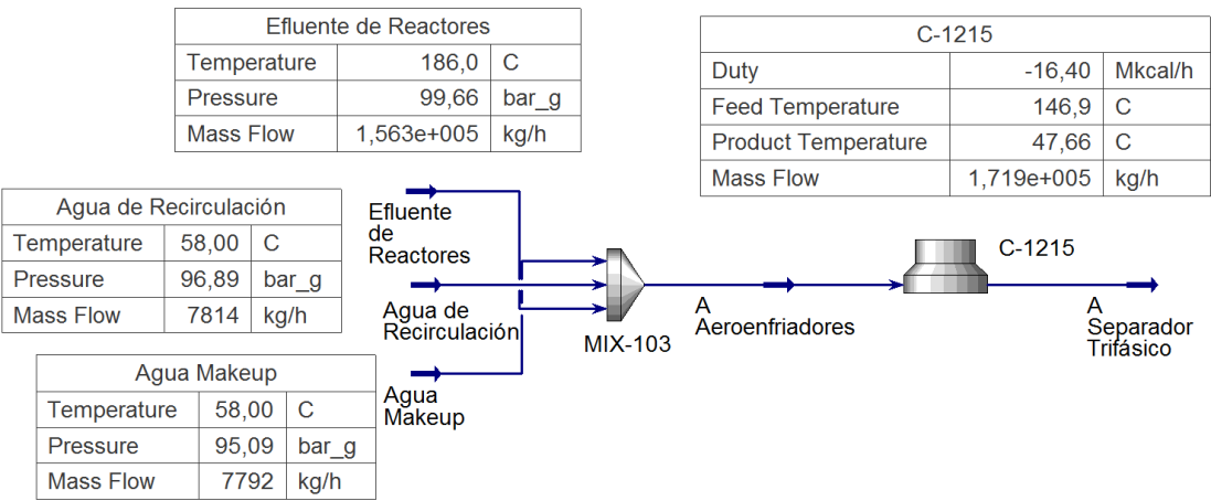
Figura IV.49: Simulación de intercambiadores C-1215 nuevos para carga de 3200 m 3 /d de gasoil.
