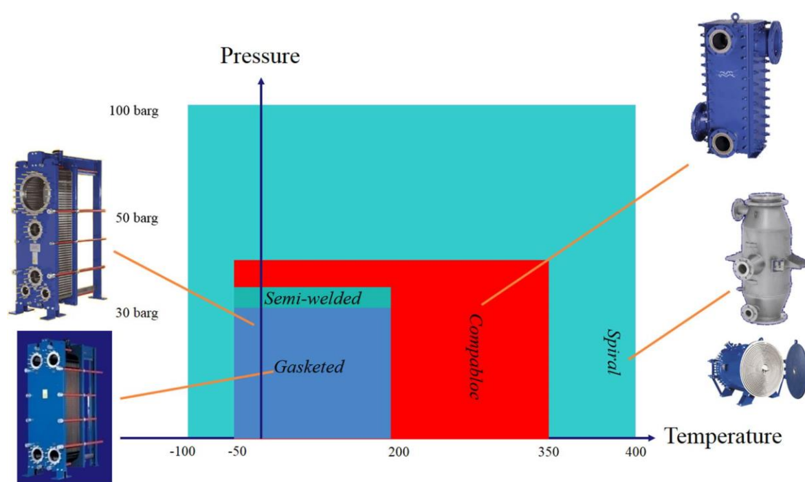
Figura V.10: Rangos de operación para la selección de intercambiadores de placas disponibles en AlfaLaval.
