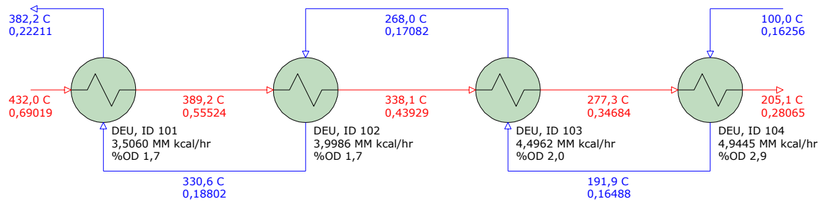
Figura V.3: Simulación de intercambiadores con inyección de agua de lavado en intercambiadores C-1201A1 y C-1201B1.
