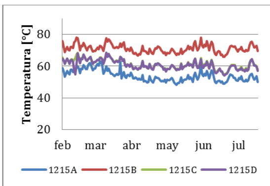
Figura IV.18: Perfil de temperatura por fecha de C-1215 previo al reentubamiento de C-1215D.
