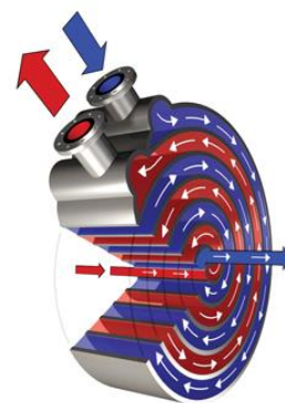
Figura IV.62: Dibujo esquemático de un Spiral Heat Exchanger.
