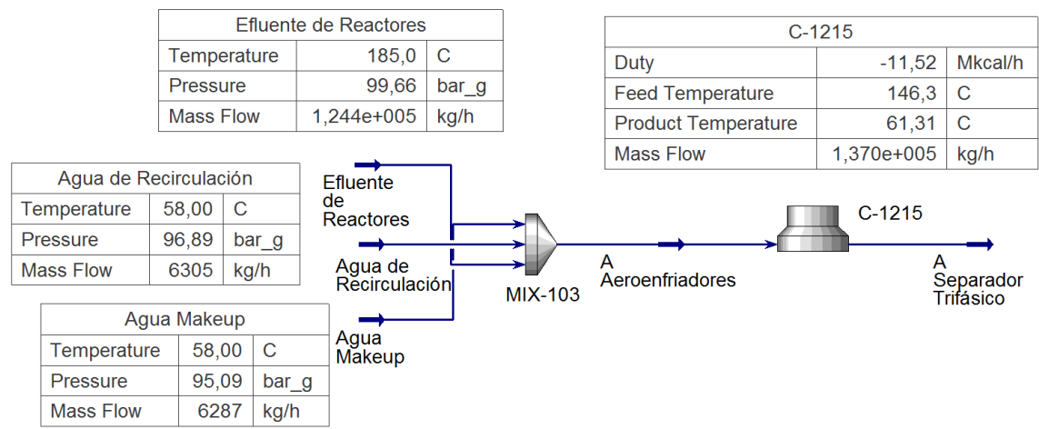
Figura IV.37: Simulación de intercambiadores C-1215 actuales para carga de 2.548 m 3 /d de gasoil..
