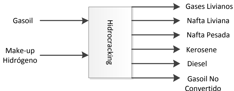
Figura IV.3: Caja negra de Hydrocracking para balance de masa
