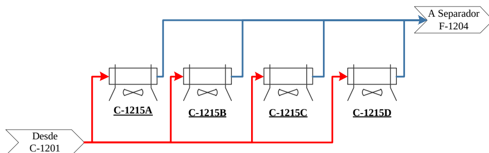
Figura IV.13: Disposición de los intercambiadores C-1215.
