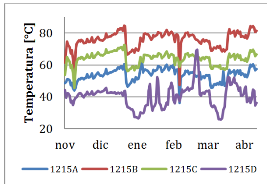
Figura IV.19: Perfil de temperatura por fecha de C-1215 desde el término del paro de planta en octubre del 2015.
