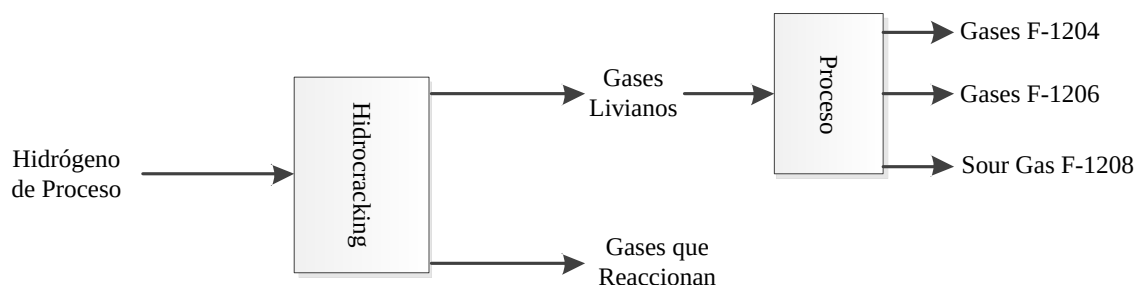
Figura IV.4: Caja negra de la planta para balance de masa de gases livianos.
