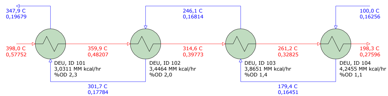
Figura IV.46: Simulación C-1201 sucios en HTRI para carga de 3200 m 3 /d de gasoil.
