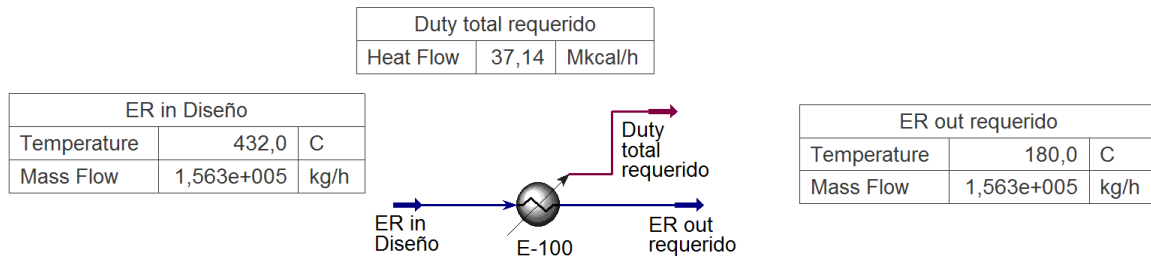
Figura IV.51: Obtención de duty requerido por diseño.
