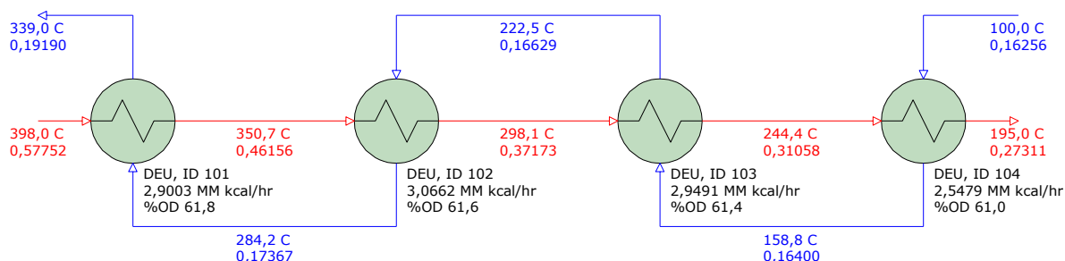
Figura IV.25: Simulación de intercambiadores C-1201 con ensuciamiento.
