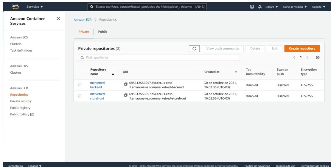
Fig. 4.15: Respositorios ECR
