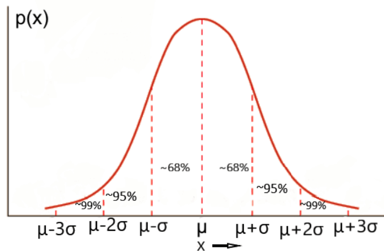
Figura 2.3: Gráfico genérico para una PDF con distribución gaussiana ( Bell-Curve ).
