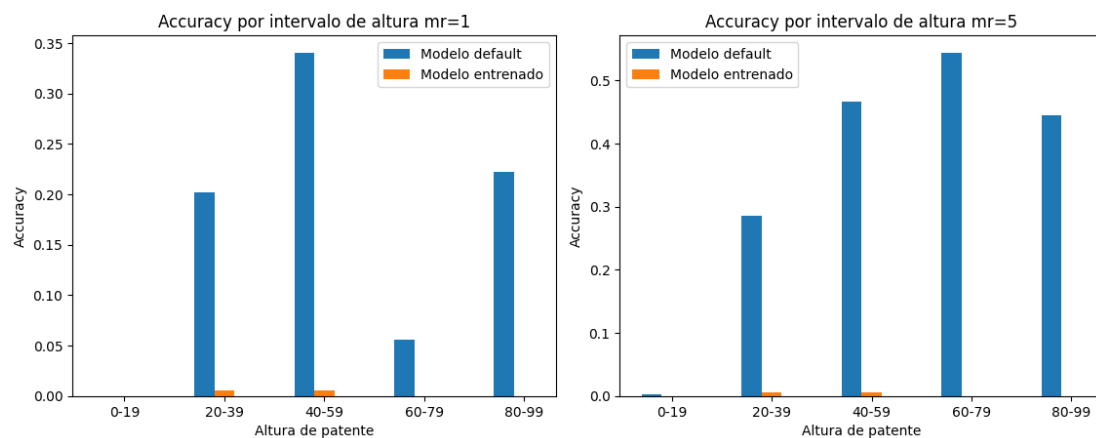
Figura 5.15: Accuracy con 'magnification ratio' de 1 y 5.
