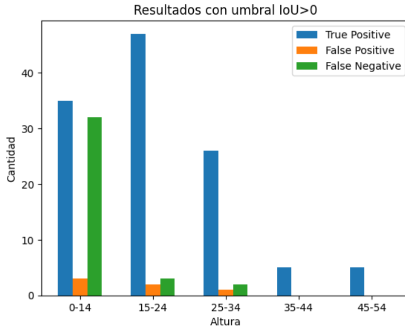
Figura 5.4: Resultados por grupo.
