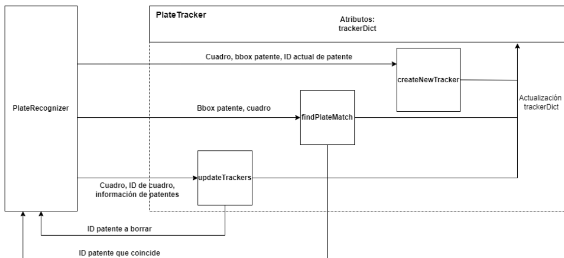
Figura 4.10: Diagrama de bloques del módulo de seguimiento.
