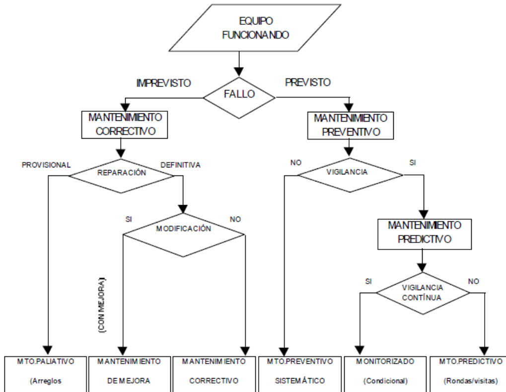
Figura 2: Diagrama de Decisión de tipo de mantenimiento, Técnicas de mantenimiento industrial, Juan Díaz Navarro
