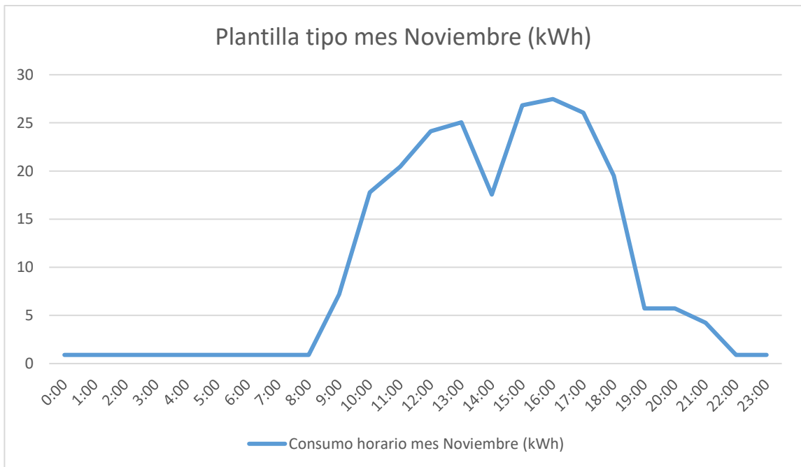
Gráfico 1-11. Consumo horario tipo del mes de noviembre.
