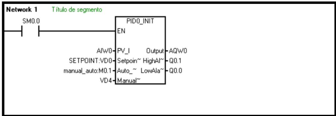
Figura 1-2. Programación PLC parte uno.
