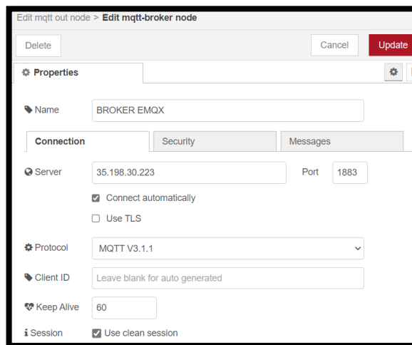
Figura 2-17. Configuración del bróker dentro de Node-RED.
