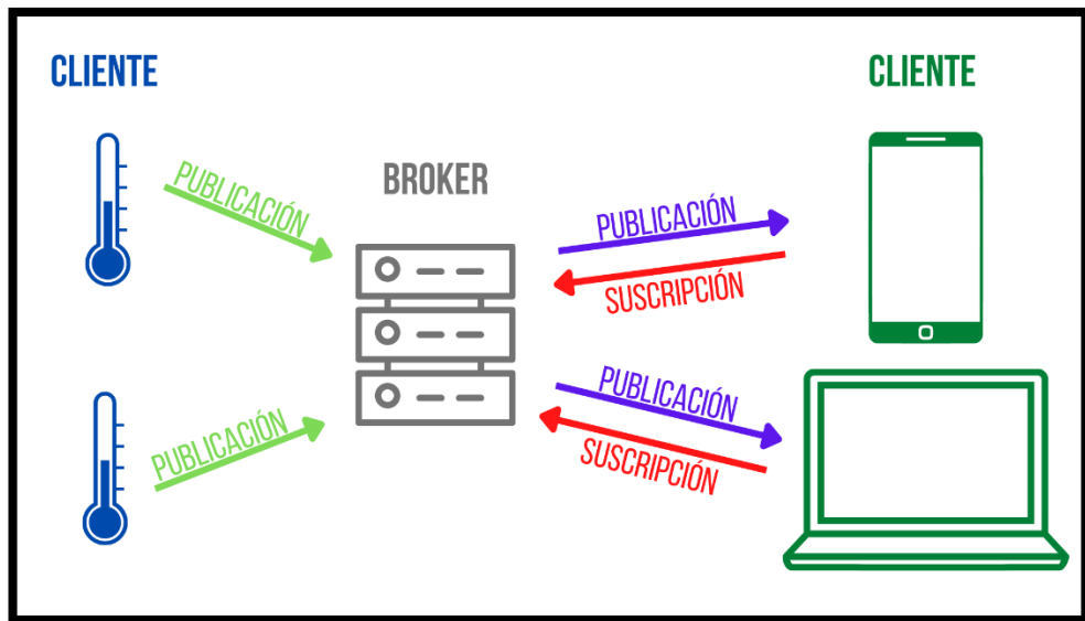
Figura 1-8. Arquitectura MQTT.
