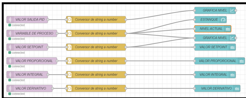
Figura 2-22. Programación dashboard.
