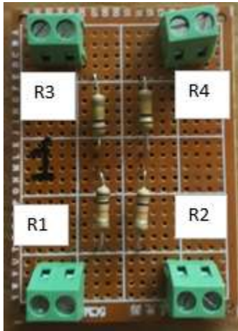
Figura 3.7 Divisor de tensión diferencial
