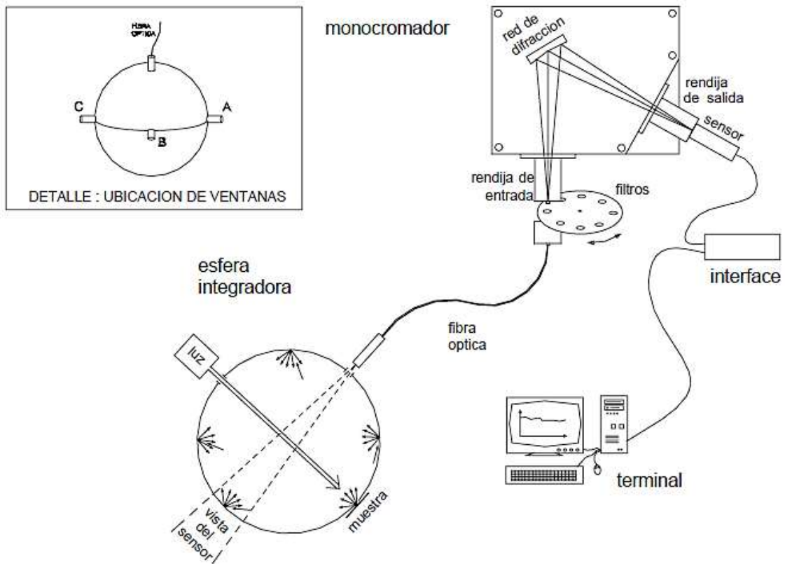
Figura 2.18 Esquema del montaje experimental [10].
