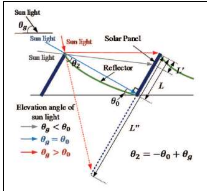
Figura 2.8 Caso (c), panel PV con reflector curvo [7].
