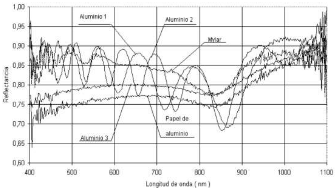
Figura 2.19 Reflectancias espectrales de aluminio de alta reflectividad, papel aluminio y papel Mylar [10]
