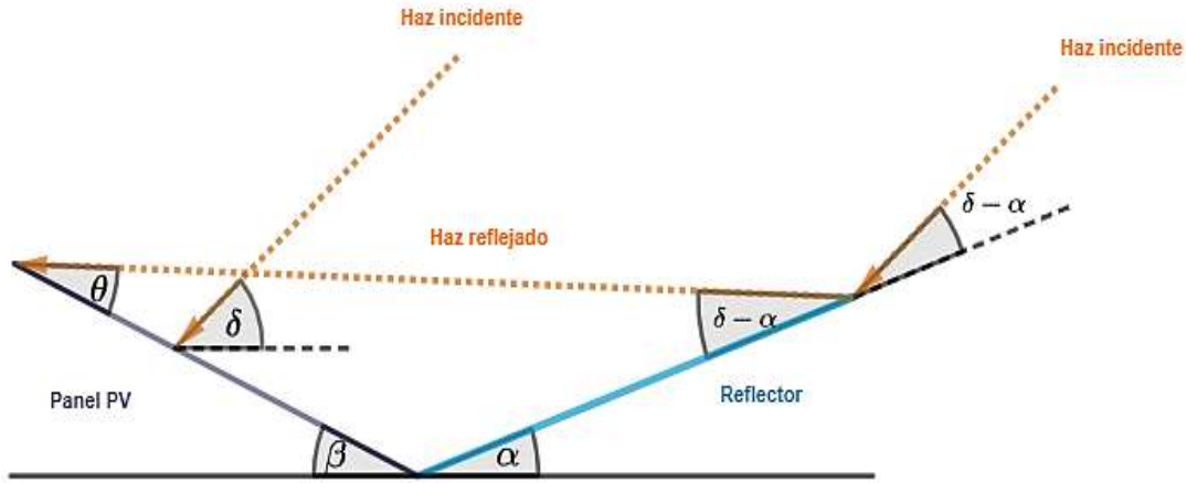
Figura 4.12 Esquema Panel PV-Reflector para la optimización de la inclinación del reflector.
