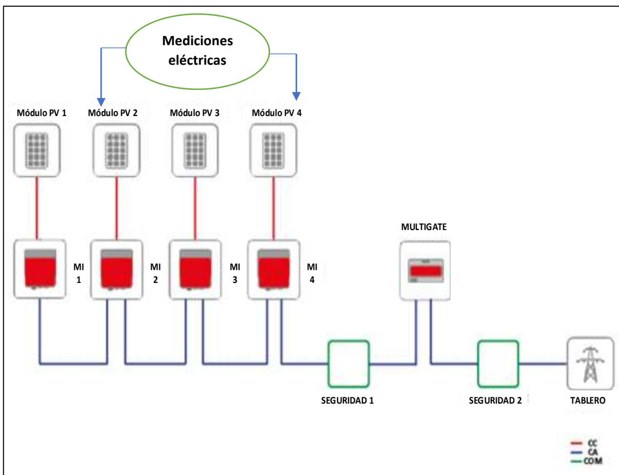
Figura 4.2 Esquema de conexiones eléctricas planta de generación.
