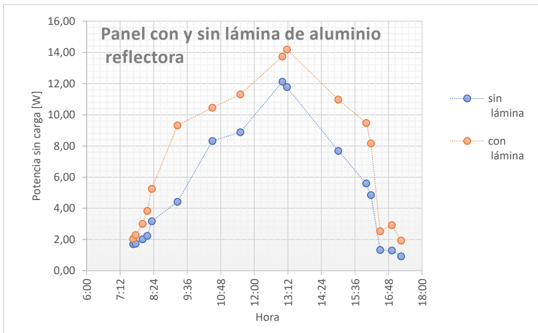
Figura 2.4 Gráfico de potencia de panel con y sin lámina de aluminio reflectora
