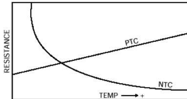
Figura 3.2 Curva característica de termistor PTC y NTC [13].
