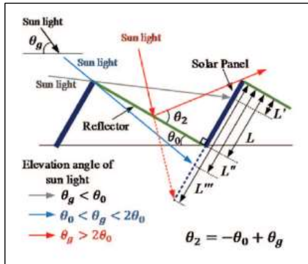
Figura 2.7 Caso (b), panel PV con reflector plano [7].
