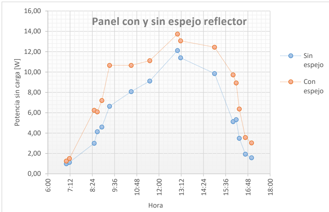
Figura 2.3 Gráfico de potencia para panel con y sin espejo reflector
