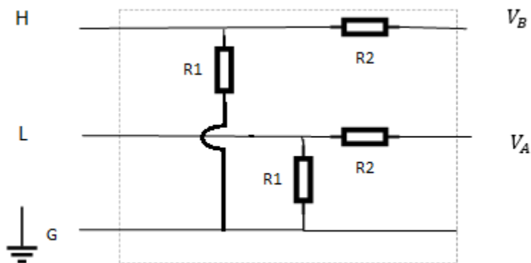
Figura 3.6 Esquema divisor de tensión diferencial.
