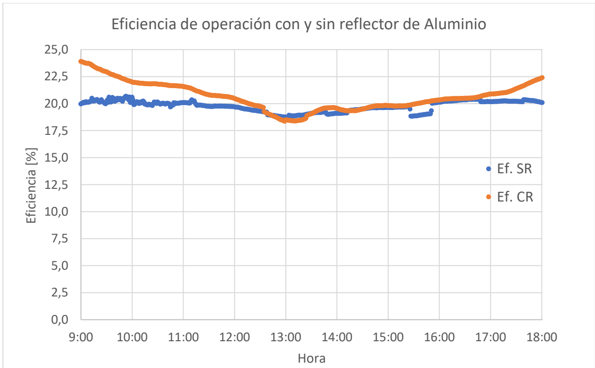
Figura 5.4 Eficiencia de operación de panel CR y sin reflector de aluminio, para aun día despejado.
