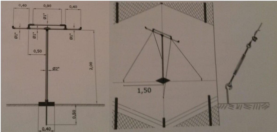
Figura 4.1: Bosquejo de estructura y disposición de vientos en estructura.-
