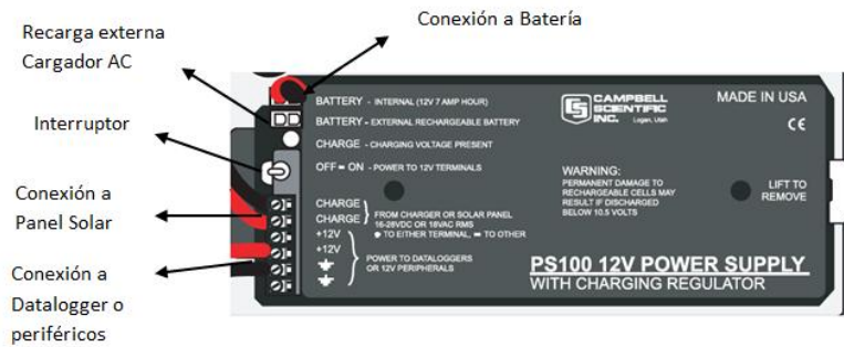
Figura 4.2: PS150, Campbell Scientific.-
