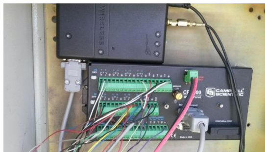
Foto 8: Datalogger CR100 EMA La Platina.-
