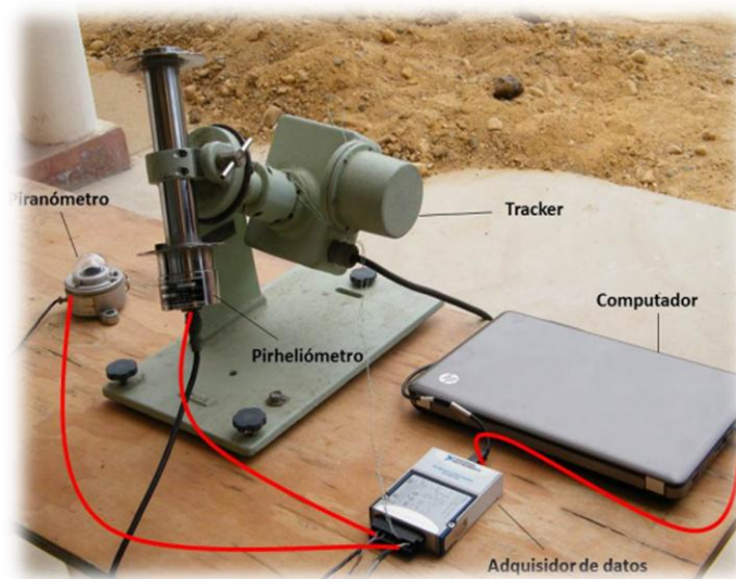
Figura 1.19: Instalación y ensamblaje de equipos.-
