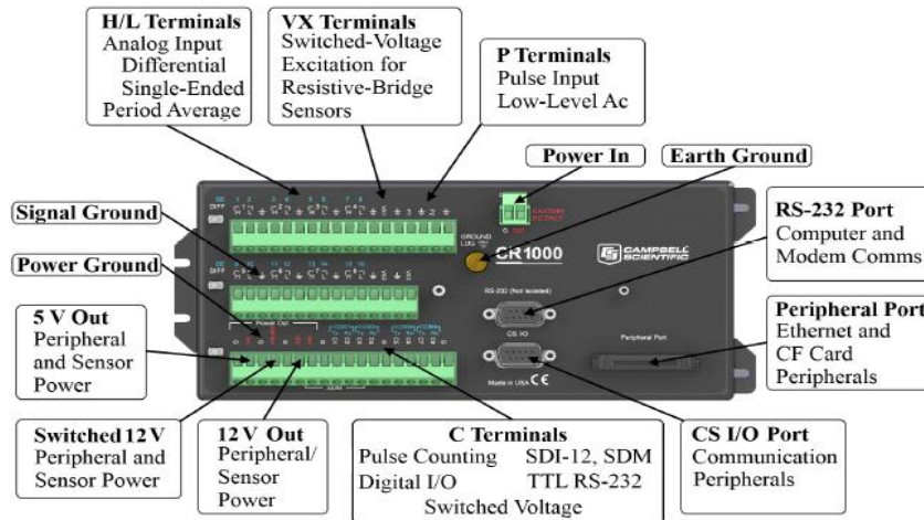
Figura 4.3: Panel de cableado del CR1000 (Manual CR1000, Campbell Scientific).-
