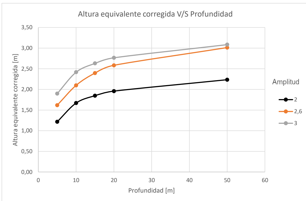
Grafico 8.5 Altura equivalente corregida respecto a la profundidad
