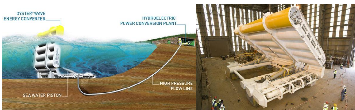
Figura 3.9 OYSTER
