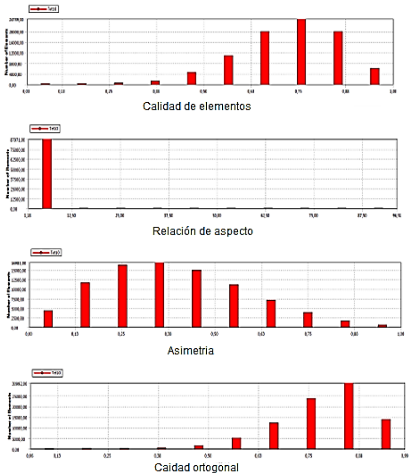
Figura 67. Histogramas de los parámetros de calidad de los elementos de la malla de la espuma d).
