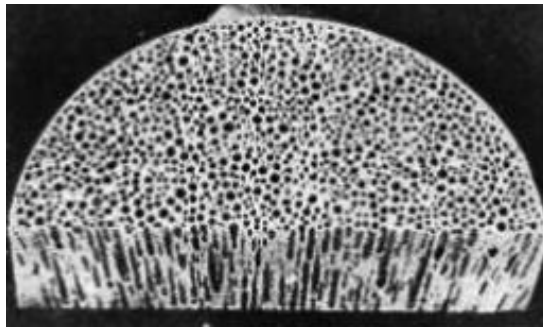
Figura 10. Espuma metálica obtenida mediante método Gasar [8].
