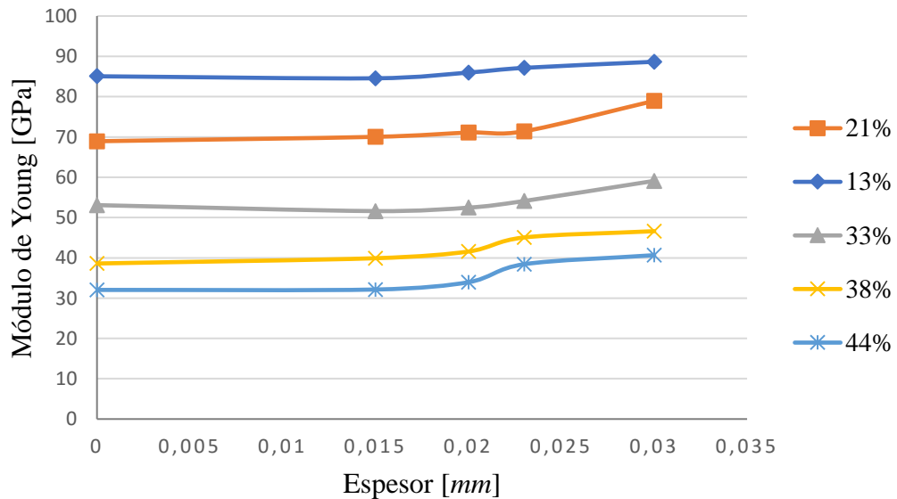
Figura 61. Comportamiento en la variación de espesores de esferas para probetas de diferente porosidad y tamaño de 8 mm.
