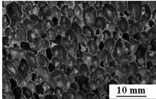
Figura 5. Espuma de aluminio de poro cerrado [6].
