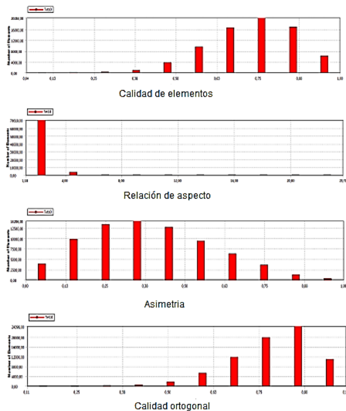
Figura 65. Histogramas de los parámetros de calidad de los elementos de la malla de la espuma b).
