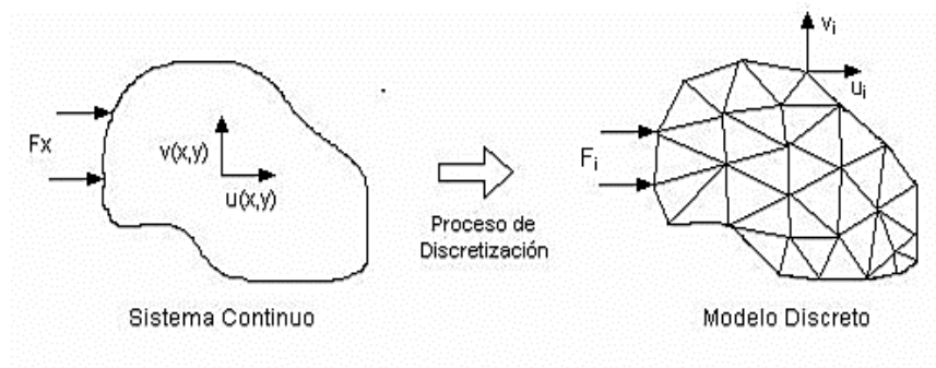
Figura 27. Proceso de discretización [41].
