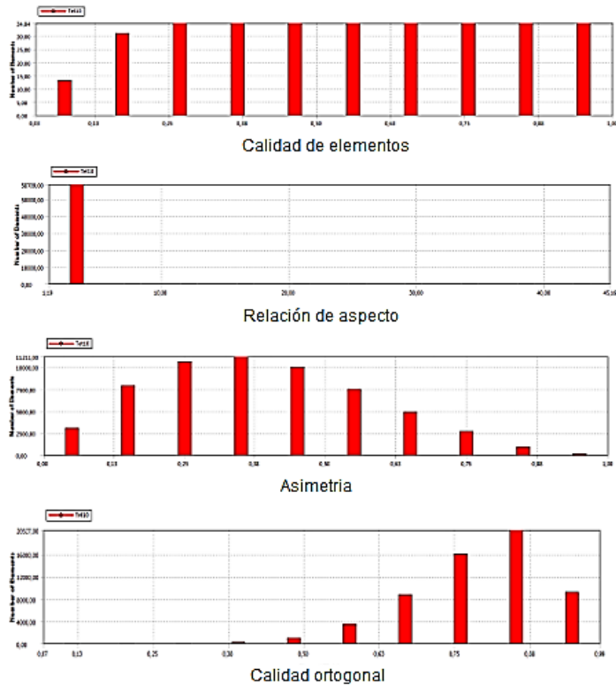
Figura 64. Histogramas de los parámetros de calidad de los elementos de la malla de la espuma a).
