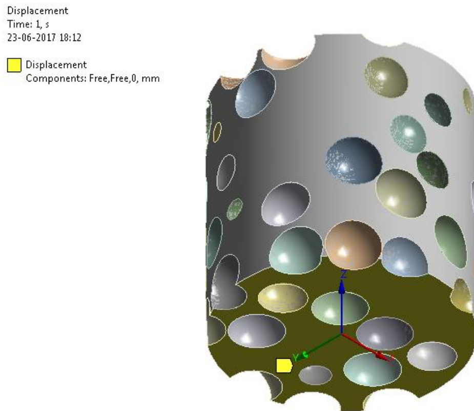
Figura 49. Condición de desplazamiento de la cara inferior de la probeta.
