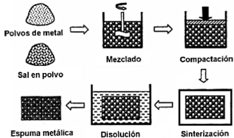
Figura 11. Fabricación de espuma por sinterización de mezcla de polvos metálicos [9].
