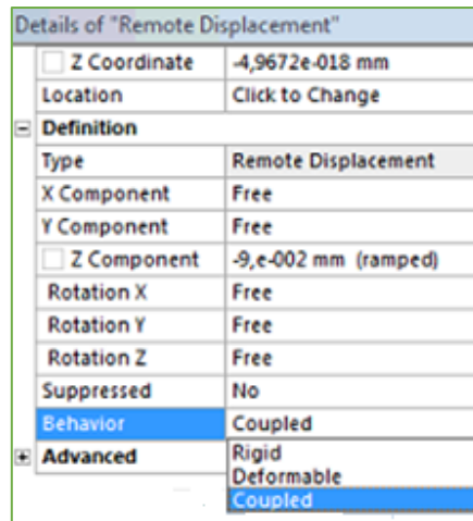
Figura 52. Detalle de la condición de desplazamiento remoto.
