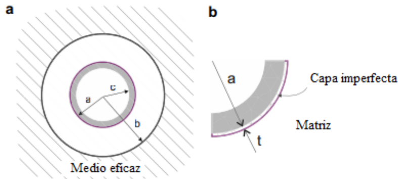
Figura 37.(a) Modelo trifásico con espuma sintáctica con interfaz imperfecta. (b) Aproximación de la capa de resorte lineal de la imperfección de la interfaz con t \ll a [53].
