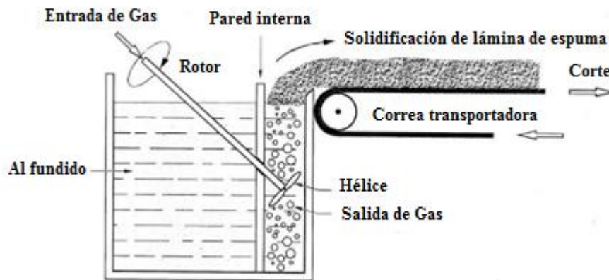
Figura 6. Esquema del método de espumante de líquido por inyección de gas [2].
