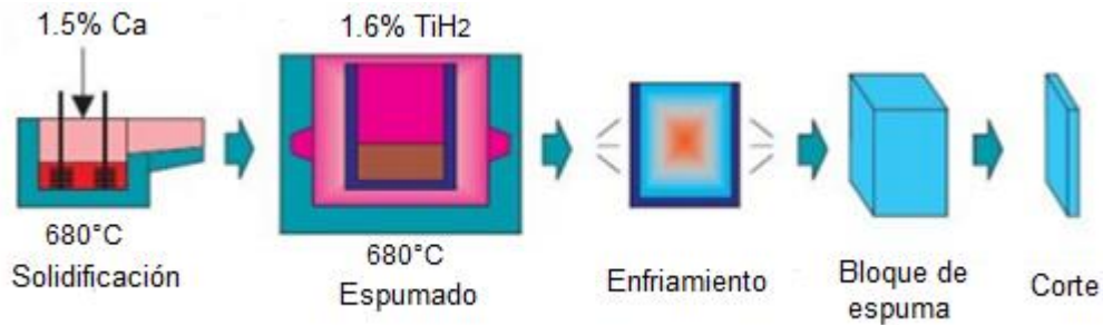
Figura 9. Esquema del método de espumado de líquidos con agentes soplantes [8].
