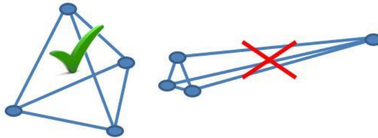
Figura 31. a) Relación de aspecto deseada contrapuesta con b) un elemento que no cumple las características. [50]
