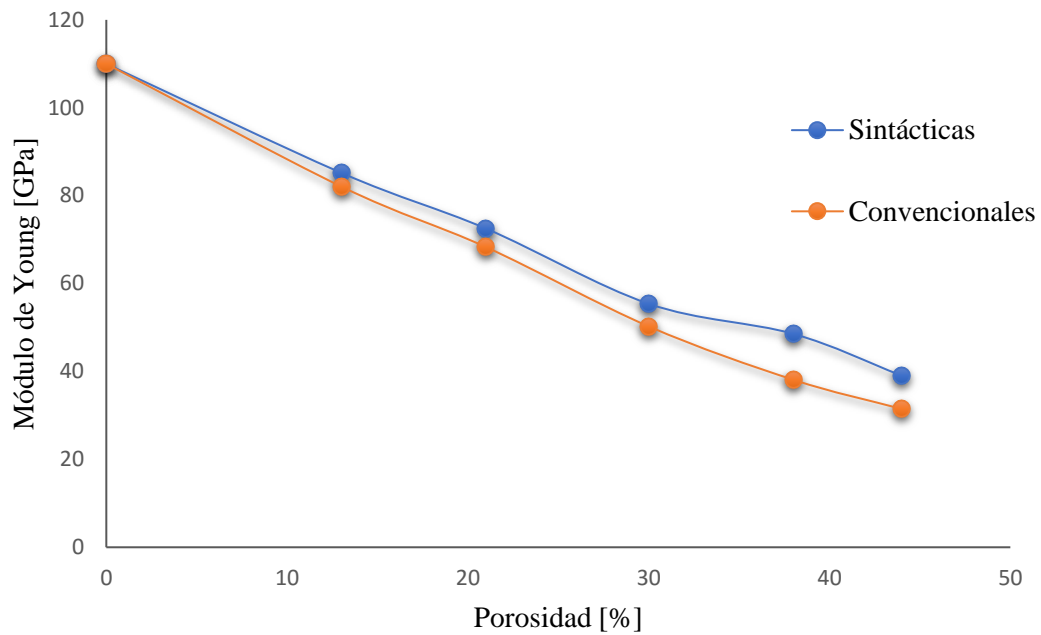
Figura 56. Gráfico para el estudio del comportamiento del Módulo de Young versus la porosidad para probetas de 9 mm, con esferas y con poros.
