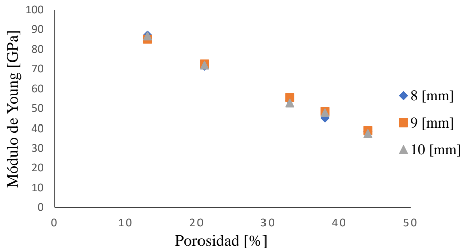
Figura 58. Gráfica del módulo de Young vs. Porcentaje de porosidad de los distintos tamaños de espuma con esfera hueca.
