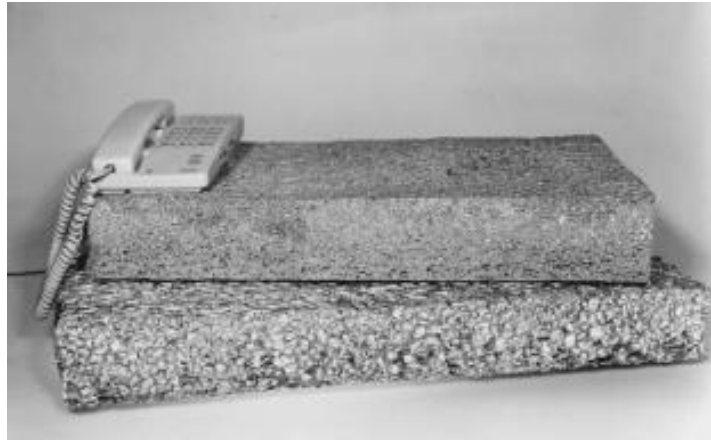
Figura 8. Planchas de espuma de dos diferentes densidades y tamaños de celda producidas mediante el método de inyección de gas (muestra: Hydro Aluminium, Noruega) [2].
