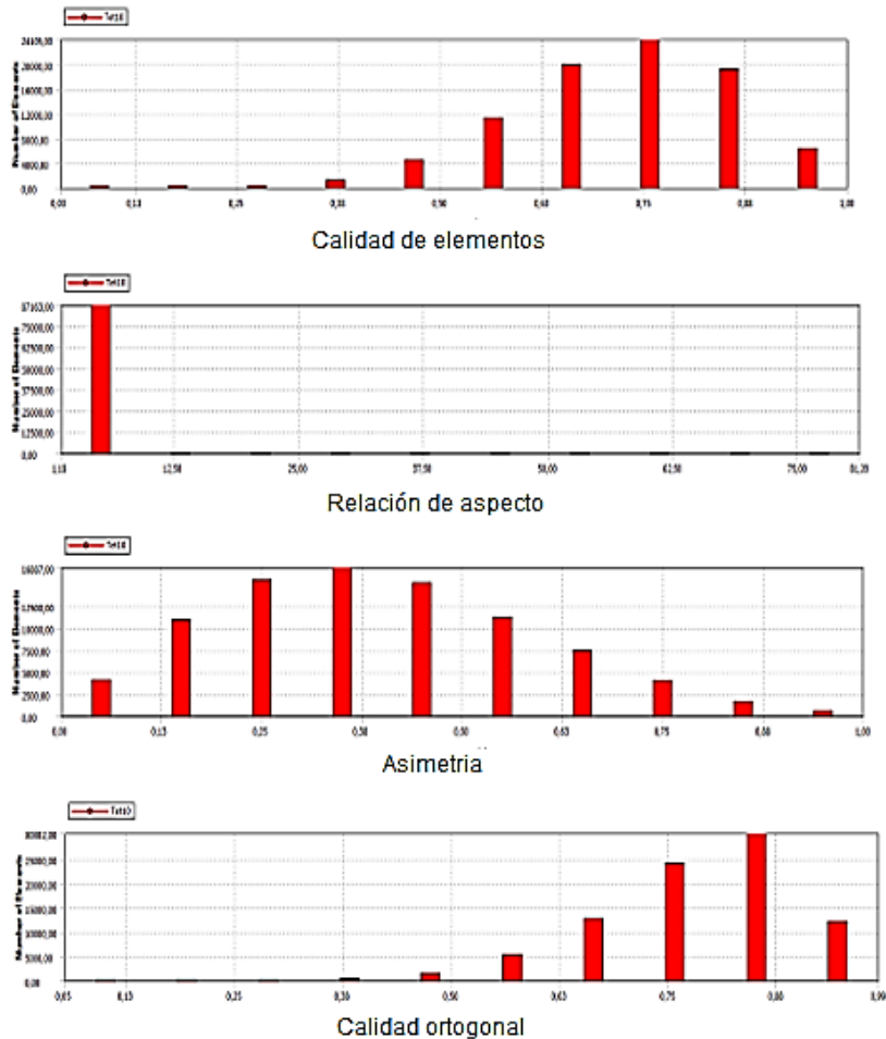
Figura 66. Histogramas de los parámetros de calidad de los elementos de la malla de la espuma c).
