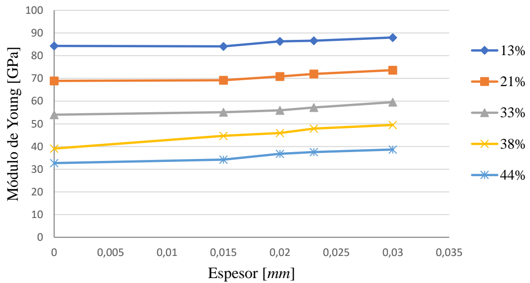
Figura 63. Comportamiento en la variación de espesores de esferas para probetas de diferente porosidad y tamaño 10 mm.
