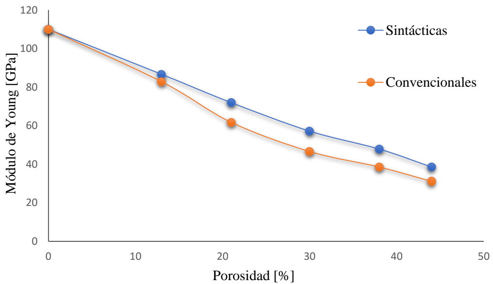
Figura 57. Gráfico para el estudio del comportamiento del Módulo de Young versus la porosidad para probetas de 10 mm, con esferas y con poros.
