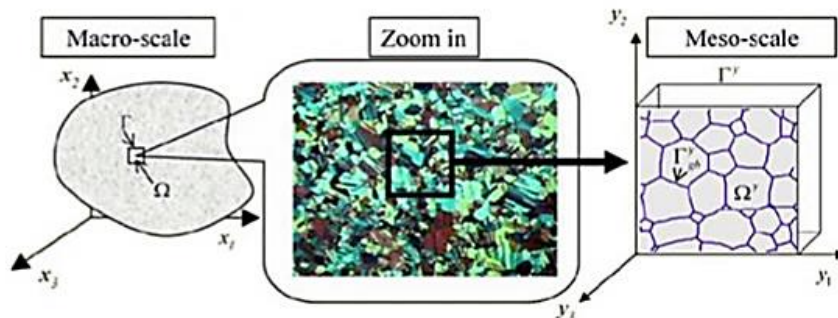
Figura 22. Escalas de homogenización [40].
