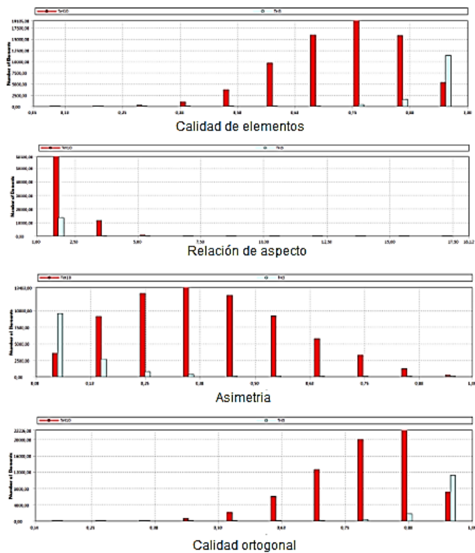
Figura 70. Histogramas de los parámetros de calidad de los elementos de la malla de la espuma g).
