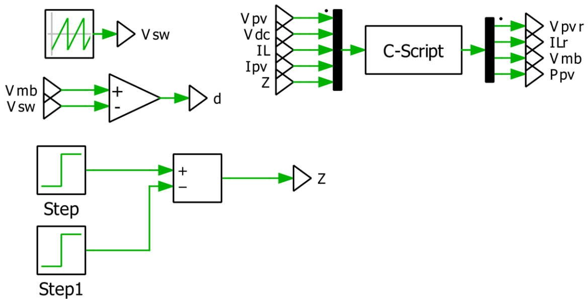
Figura A.2 Control convertidor Boost en PLECS.
