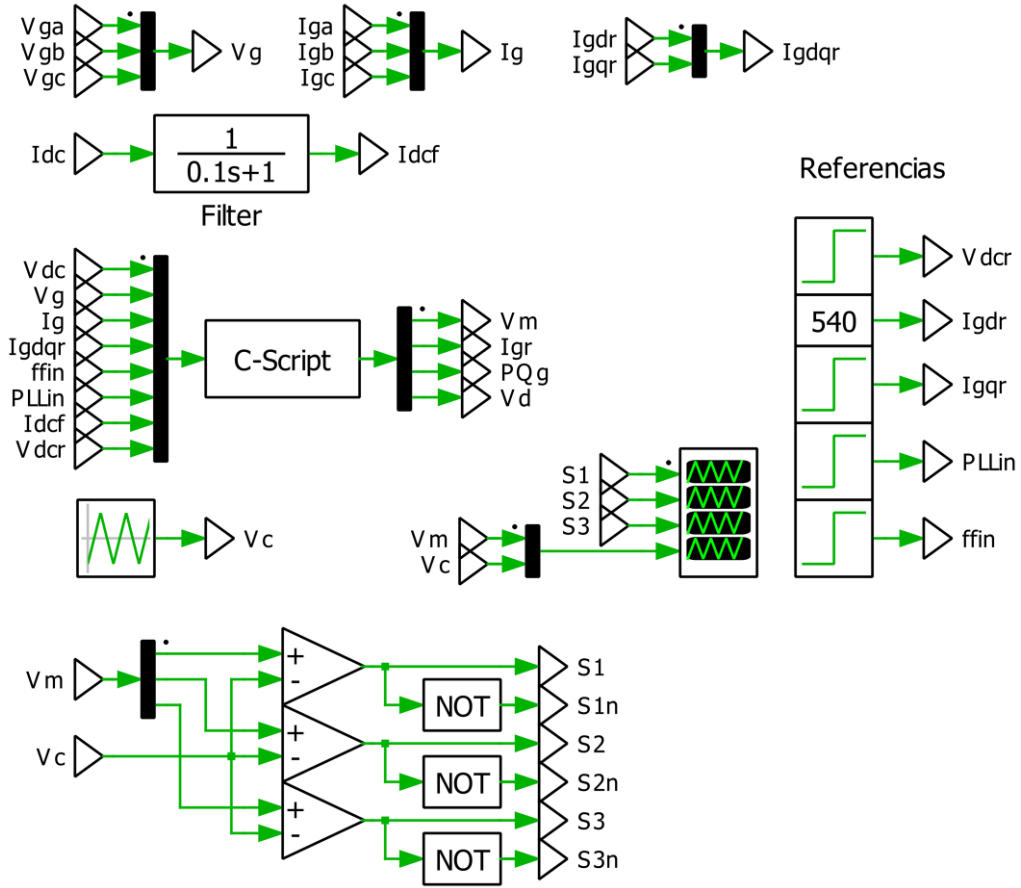
Figura A.3 Control convertidor Puente H en PLECS.
