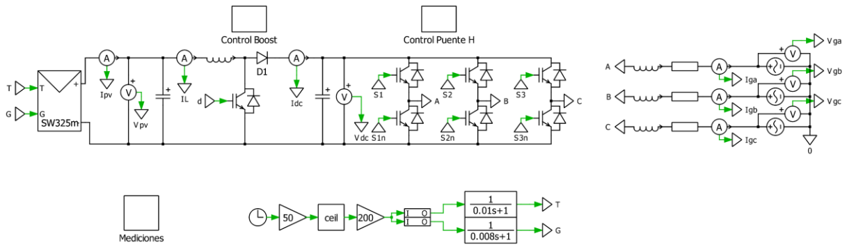
Figura A.1 Circuito general del convertidor en PLECS.
