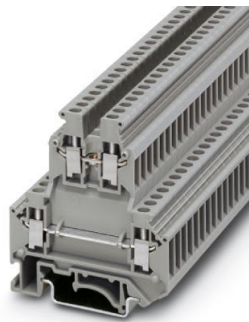
Figura 6.2: Bornera DIN
