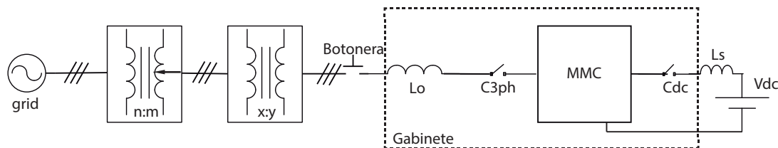
Figura 5.1: Diagrama unilineal de conexión a red
