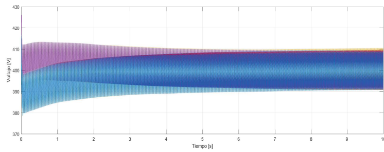
Figura 3.13: Evolución del control de balance en las celdas de fase A
