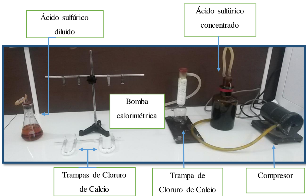
Ilustración 38: Esquema de instalación de ensayo para determinar agua total producida en la combustión y posteriormente el poder calorífico inferior.
