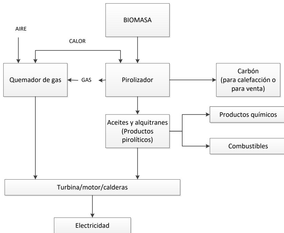
Ilustración 15: Diagrama de alternativas de conversión de energía en Pirólisis. [8]
