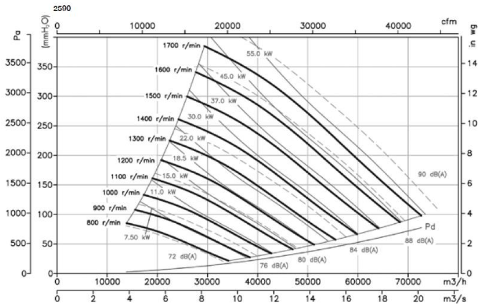
Ilustración 29: Curvas características ventilador Sodeca, modelo CMR-2590.
