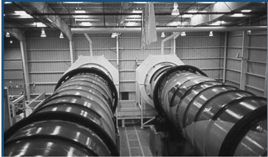
Ilustración 26: Vista de un sistema de Tambor rotativo de compostaje estándar. [14]
