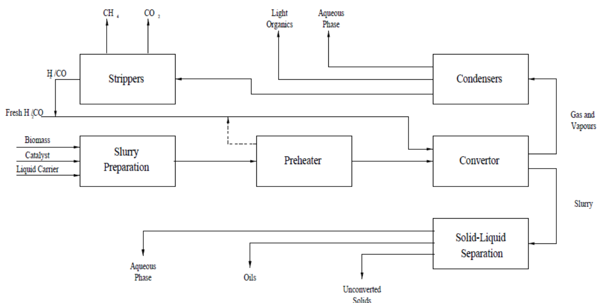
Ilustración 16: Diagrama de flujo del proceso de Licuefacción. [1]
