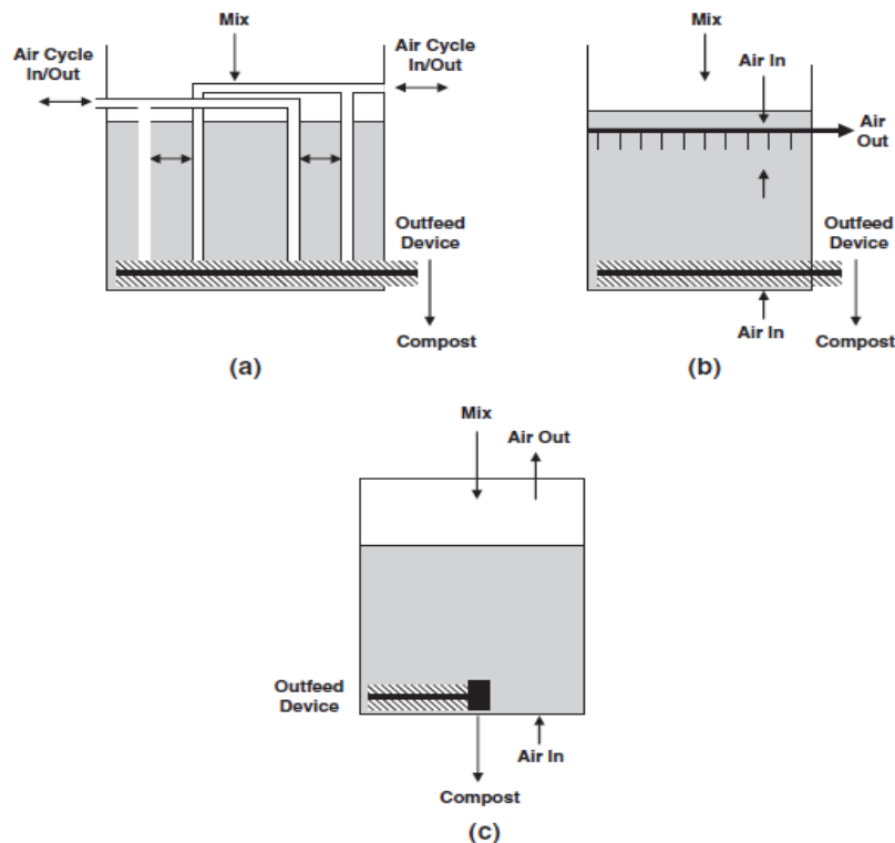
Ilustración 23: Diagrama esquemático de los reactores verticales. [13]
