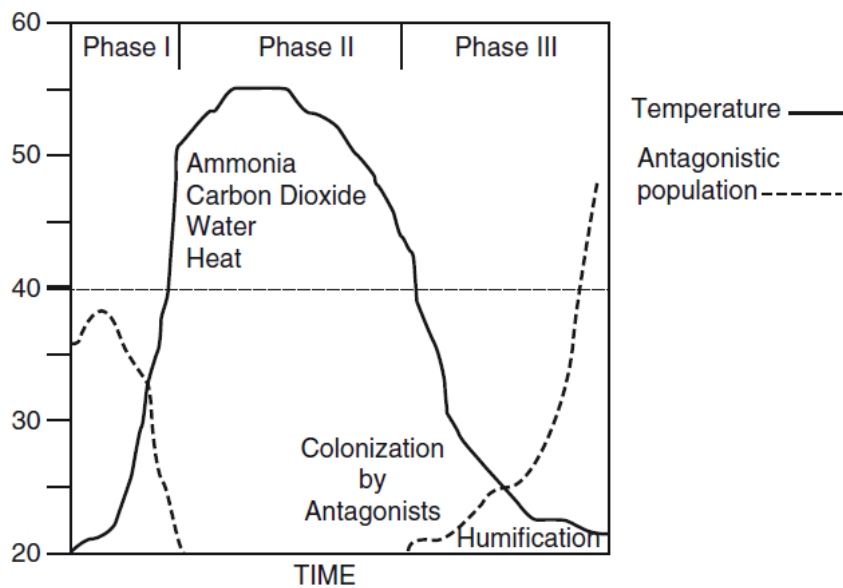
Ilustración 18: Diagrama de Temperatura en las fases del proceso de compostaje. Smith 1992 [12]
