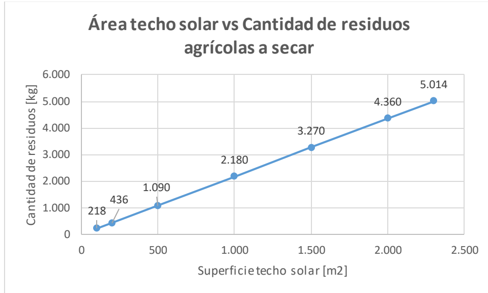
Gráfico 3: Área de techo solar activo vs cantidad de residuos agrícolas a secar en un período de 14 horas. (Los residuos agrícolas poseen una humedad inicial de 85% y tienen un consumo energético específico de 3 [MJ/kg]).
