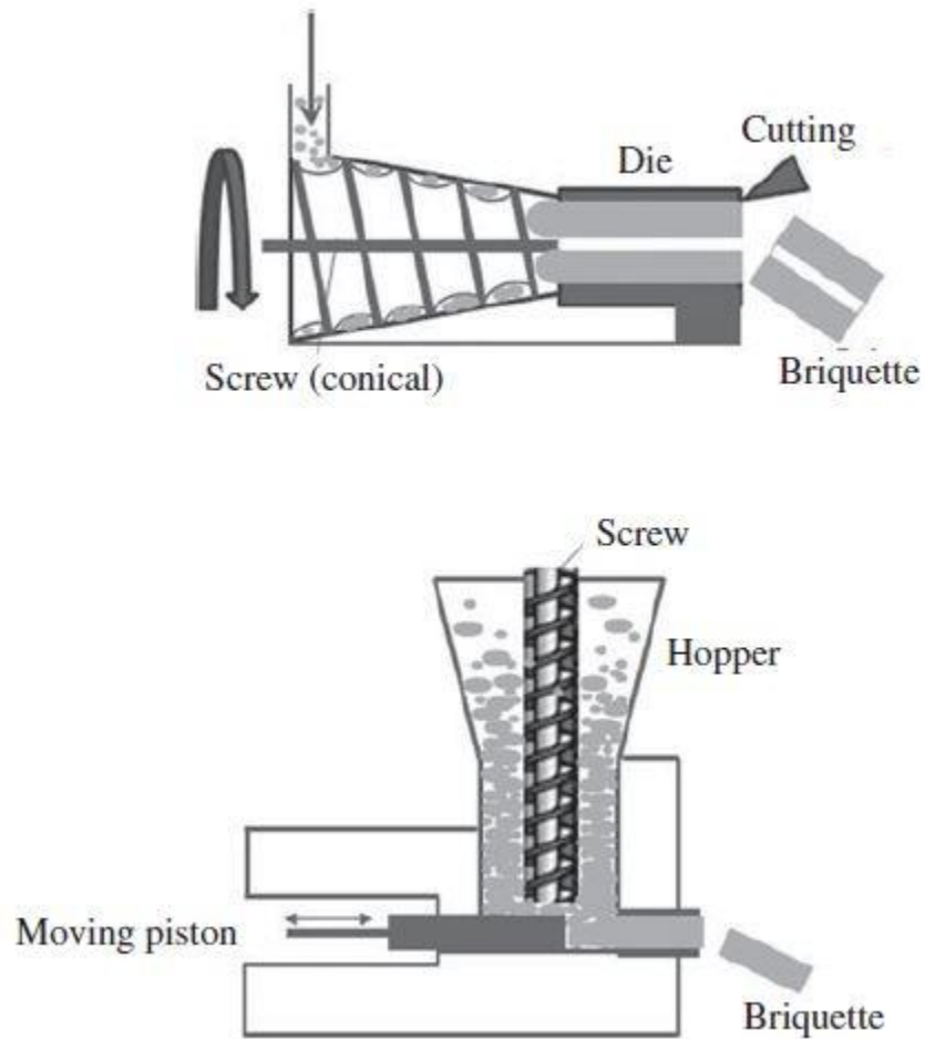
Ilustración 7: Tecnologías para la producción de briquetas. Extrusor de tornillo (arriba) y "Piston press" (abajo).
