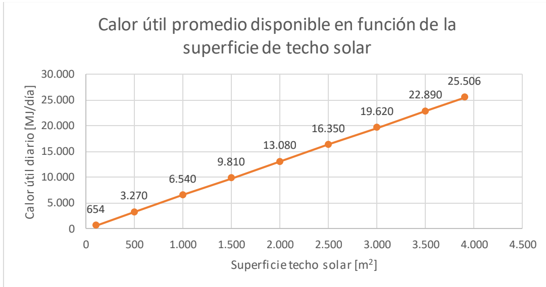
Gráfico 2: Calor útil promedio disponible en función de la superficie de techo solar.
